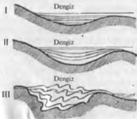
49-rasm. Geosinklinal taraqqiyot bosqichlari:
