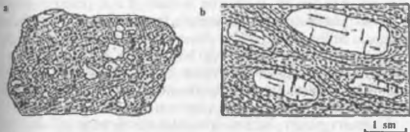
31-rasm. Effuziv tog' jinslarining struktura va teksturalari:
