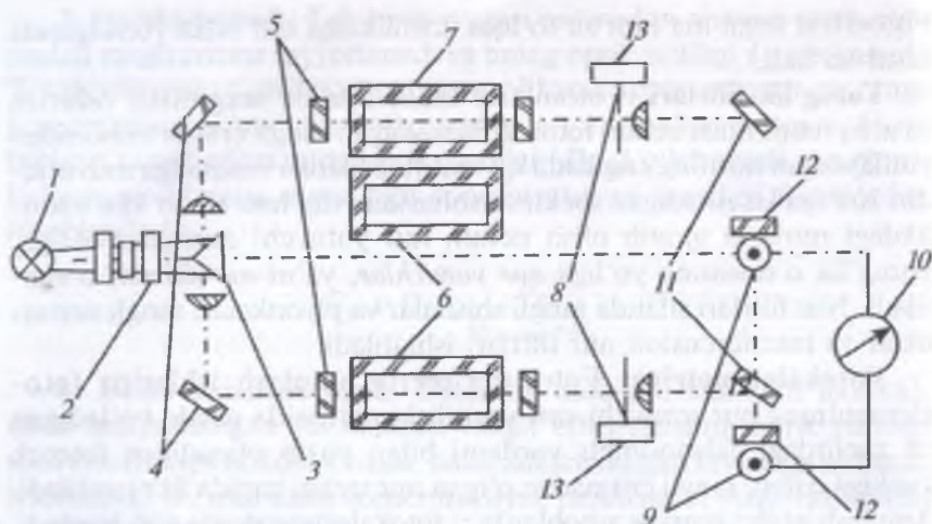
6-rasm. ФЭК-56M fotoelktroklorimetrlning optik sxemasi.
