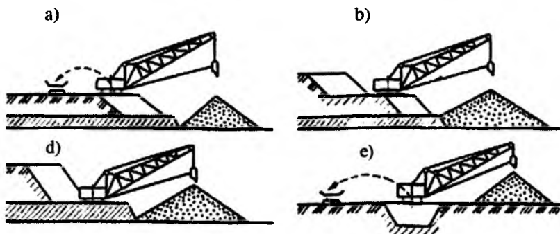
29-rasm. Draglaynning ishlash sxemalari: a,b,d – mos ravishda draglayn pog‘ona ustida, pog‘ona usti bilan osti o‘rtasidagi maydonchada va pog‘ona ostki maydonida turganda; e–draglayn pog‘ona ustki maydonida turganda.
