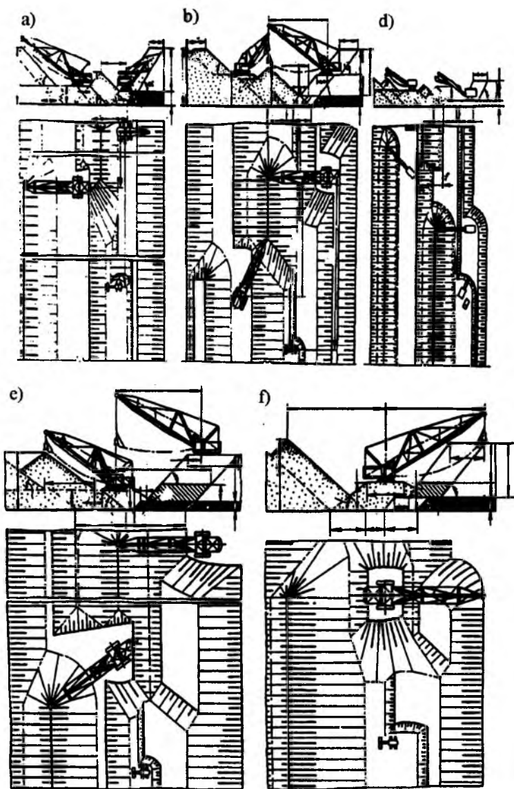
76 - rasm. Bir cho'michli ekskavatorlar bilan qoplama jinslarni qazishdan bo'shagan maydonga qayta-qayta ekskavatsiyalashda ochish ishlari texnologiyasining variantlari.
