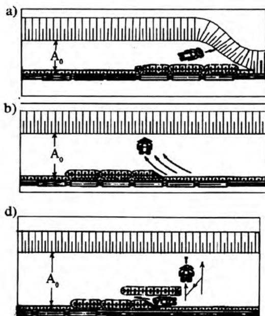
51- rasm. Temiryoʻl transporti qoʻllanganda buldozer bilan agʻdarma hosil qilishning texnologik sxemalari: a – toresli (koʻndalang); b – boʻylama (frontal); d – aralash.
