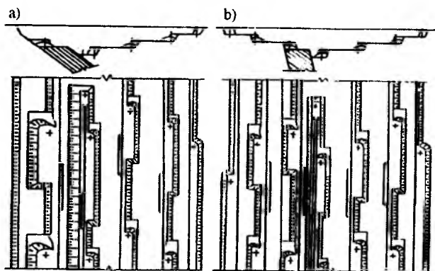
87 - rasmlar. Qoplama jinslarni temiryoʻl transporti bilan tashqi agʻdarmaga tashishda qiya (a) va oʻta qiya (b) konlarni qazib olish texnologik sxemalari.
