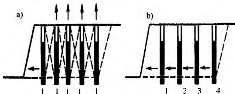
14-rasm. Zaryadlarni oniy (a) va qisqa kechiktirilgan (b) portlatishda zaryadning ta'sirini aniqlash sxemalari (sonlar bilan zaryadlarni portlatish navbatini ko'rsatilgan).
