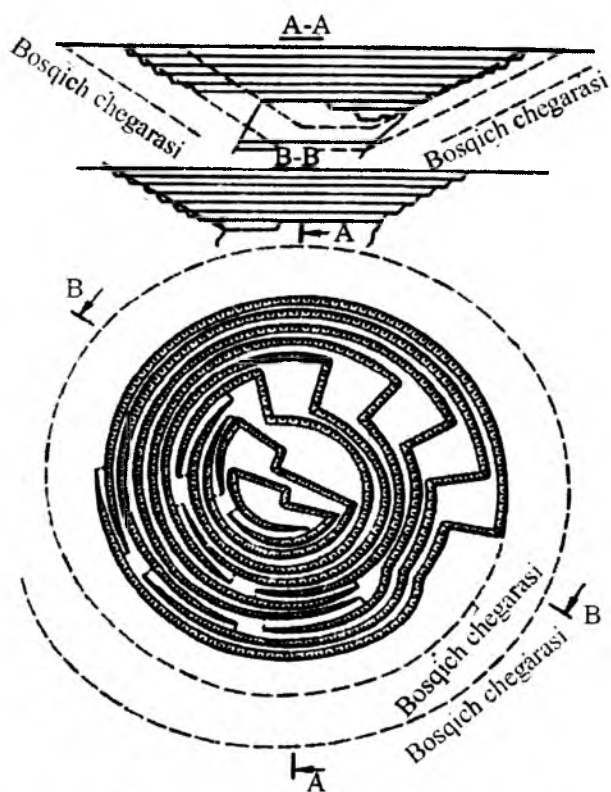
90 - rasm. Qiya qatlamsimon (a) va shtoksimon (b) konlarni pollarga ajratib qazib olish texnologik sxemalari.
