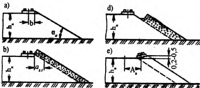
50-rasm. Plug bilan ag'darma hosil qilish sxemasi: a – lokomotiv sostavlarini to'kishdan oldingi ag'darma qiyaligining holati; b – bu ham jinslar to'kilgandan keyin; d – profillashtirilgandan keyin; e – ikkinchi marta to'kilgandan va yo'lni surilgandan so'ng.
