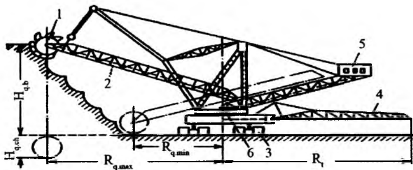
32-rasm. Rotorli ekskavator sxemasi: 1 – rotor g'ildiragi; 2 – strela; 3 – gusenitsalar; 4 – to'kish konsoli; 5 – posangi; 6 – burilish platformasi.
