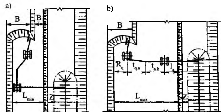
79 - rasm. Konsolli ag'darma hosil qiluvchi uskuna qo'llaganda minimal (a), maksimal (b) ochilgan foydali qazilma zaxirasini qazib olish texnologik sxemalari.
