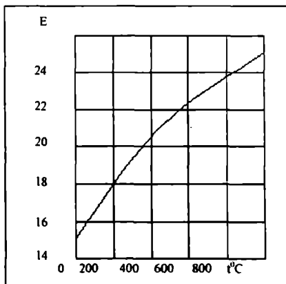
11.7-rasm. (11.20) tenglamadagi E koeffitsiyentini aniqlash uchun grafik.
