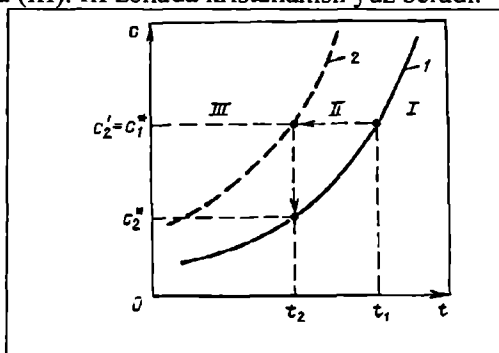
19.1-rasm. Muvozanat va to'yingish konsentratsiyalarining haroratdan bog'liqligi:
