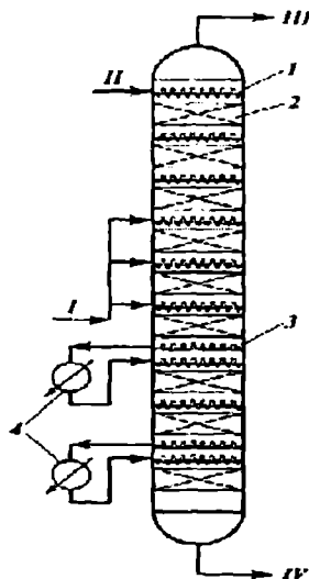
17.9 -rasm. Nasadkali ekstraksiya kolonnaning sxemasi: 1—taqsimlovchi tarelka; 2—nasadka qatlami; 3—bo'g'iq tarelka; 4—oraliq sovitgichlar. Oqimlar: I—xomashyo; II—erituvchi; 3—rafinat eritmasi; ekstrakt eritmasi.
