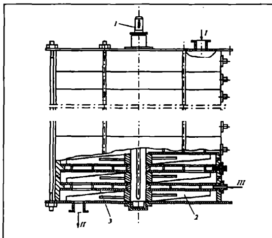
19.6-rasm. Diskli kristallizator sxemasi:
