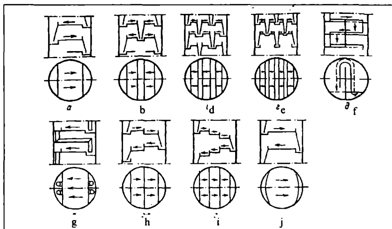
15.2-rasm. Quyilish moslamasi bo'lgan tarelkalarining ustida suyuqlik oqimining sxemalari:
