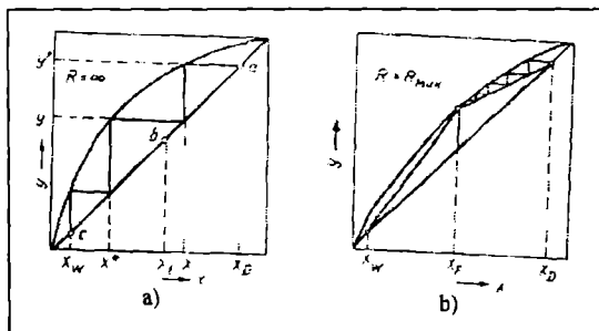
13.12-rasm. Flegma soni bilan rektifikatsion kolonna balandligining o'zaro bog'lanishi:
