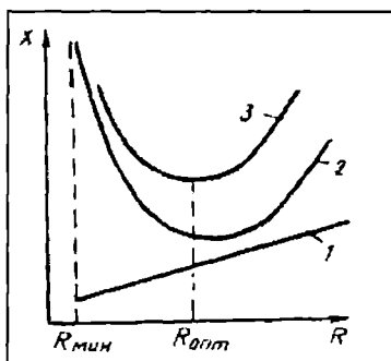
13.11-rasm. Flegma sonining maqbul qiymatini aniqlashga doir: 1–qurilmani ishlatish bilan bog'liq bo'lgan sarflar; 2–kapital xarajatlar; 3–umumiy xarajatlar.
