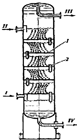
17.10 - rasm. Elaksimon tarelkali ekstraktorning sxemasi:
