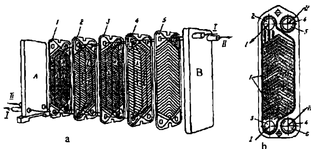
10.10-rasm. Plastinali issiqlik almashgich:
