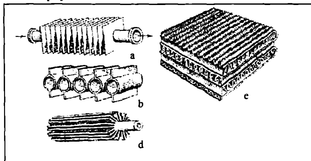
10.13-rasm. Qirrali issiqlik almashgichlarning elementlari: a–qirralari ko'ndalang kesim bo'yicha joylashtirilgan; b,d–qirralari o'q kesimi bo'yicha joylashtirilgan; e–qirralari qat-qat burmali qilib tayyorlangan.
