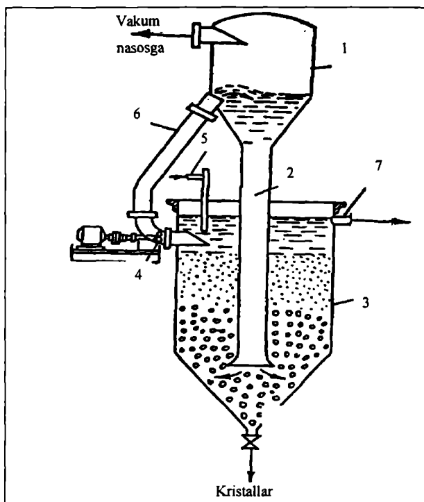
19.4-rasm. Vakuum-kristallizator:
