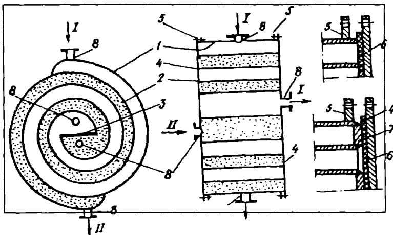
10.11-rasm. Spiralsimon issiqlik almashgich:
