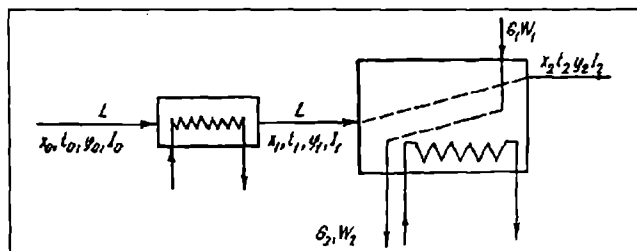
18.8-rasm. Haqiqiy quritgichni hisoblashga doir.
