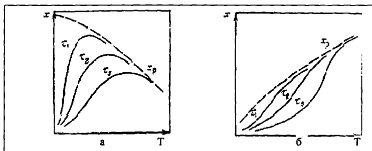
20.1-rasm. Qaytaruvchi egzotermik (a) va endotermik (b) reaksiyalar uchun jarayonning turlicha davomiyligi \tau paytdagi o'zgartirish darajasi x ning harorat T dan bog'liqligi ( \tau_1 > \tau_2 > \tau_3 ; x_r —muvozanat holatdagi qiymat).
