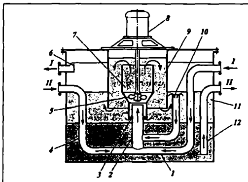
17.8- rasm. Aralashtirgich-tindirgich rusumidagi ekstraktorning sxemasi:
