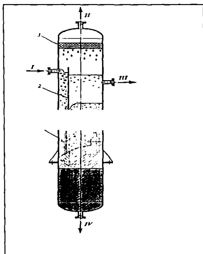
4.4-rasm. Gazoseparator – suv ajratgichning sxemasi:
