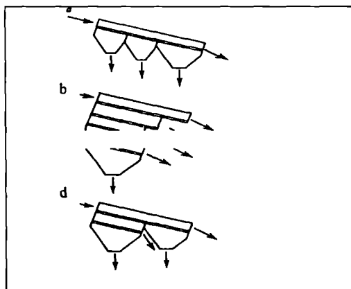
8.1-rasm. Sochiluvchan qattiq materiallarni katta sim g'alvir bilan eish usullari:
