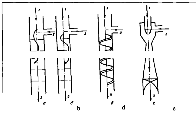
5.6-rasm. Oqimda aralashtirish uchun ishlatiladigan uskunalarning sxemalari:
