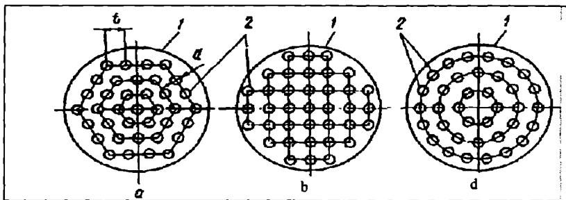
10.6-rasm. Quvurlarni quvur to'rlariga joylashtirish usullari:
