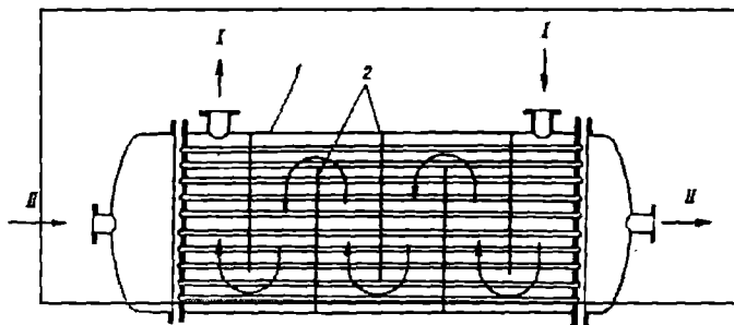
10.4-rasm. Ko‘pli yo‘lli (quvurlar tashqarisidagi bo‘shliq bo‘yicha) issiqlik almashgich:
