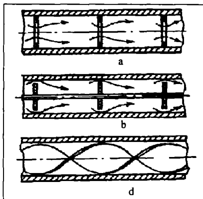
10.15-rasm. Turbulizatsiya qiladigan qo'shimcha quvurlar: a) diafragmali; b) diskli d) spiralli.
