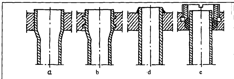
10.2-rasm. Quvurlarni quvur to'rlariga biriktirish usullari:
