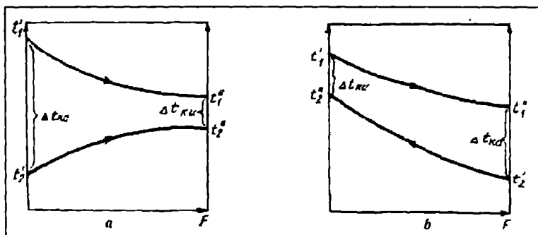
9.6-rasm. Issiqlik tashuvchi agentlar haroratining yuza bo'yicha o'zgarishi:
