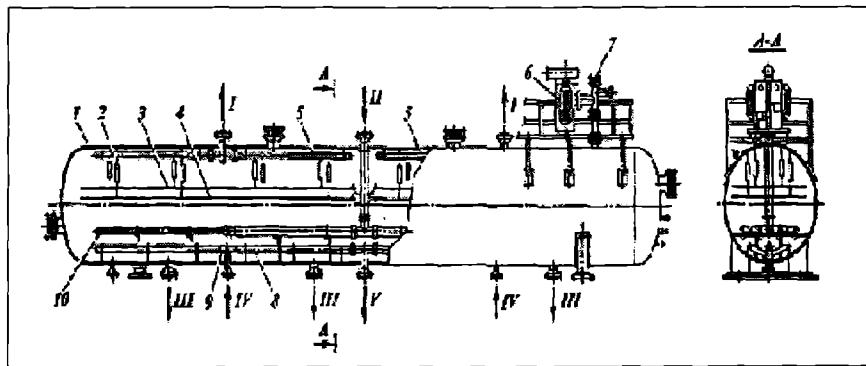
2.11-rasm. Gorizontaal elektrodegidratator EG200-10:
