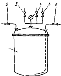
3.15-rasm. Montejoyu:
