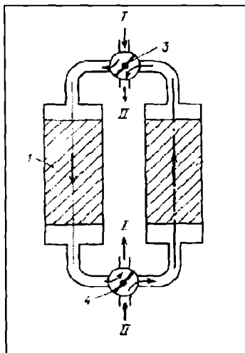
10.18-rasm. Qo'zg'almas qatlamli regenerativ issiqlik almashgichning ishlash sxemasi:
