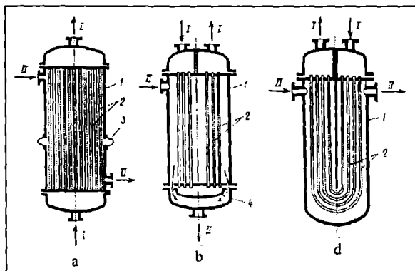
10.5-rasm. Qobiq va quvurlarning turlicha uzayishini kompensatsiya qiladigan qobiq-quvurlari issiqlik almashgichlar:
