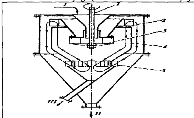
8.5-rasm. Markazdan qochma havo separatorining sxemasi:
