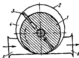
3.10- rasm. Plastinkali nasos: 1 – rotor; 2 – qobiq; 3 – plastinalar; 4 – boʻshliq; 5 – soʻruvchi trubka; 6 – uzatuvchi trubkasi.
