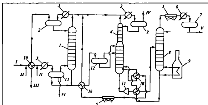
14.6-rasm. Tabiiy va neftga yo'ldosh gazlarni ajratishga mo'ljallangan absorbsion – desorbsion qurilmaning sxemasi:
