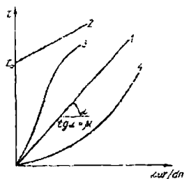
2.3-rasm. Oqish egri chiziqlari. Suyuqliklar: 1- nyuton; 2- bingam; 3- mavhum plastik; 4- dilatant.
