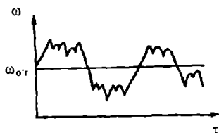
2.8- rasm. Oqim tezliklarining pulsatsiyasi ( \omega_{0,i} = \omega \pm \Delta\omega ).
