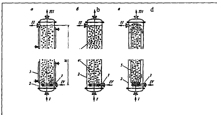
5.3-rasm. Barbotajli aralashtirgichli uskunalarning sxemalari: a—ichi bo'sh; b—seksiyali; d—gazliftli; 1—barbolyor; 2—qobiq; 3—sovitish g'illofi; 4—seksiya hosil qiluvchi to'siqlar; 5—sirkulatsiya quvuri. Oqimlar: I—dastlabki suyuqlik; II—chiqayotgan suyuqlik; III—chiqayotgan gaz; IV—kirayotgan gaz.
