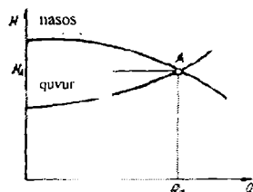
3.6-rasm. Nasos va quvurning o‘zaro bog‘lanish xarakteristikasi.
