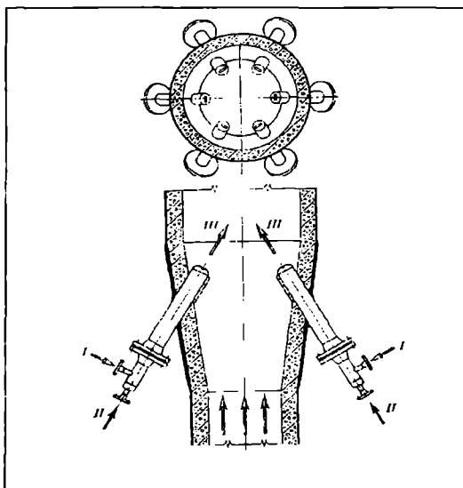
21.9- rasm. Reaktor liftingning pastki qismiga «Atomax» soplosini o'rnatish sxemasi:
