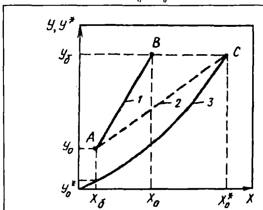
14.2-rasm. Absorbsiya jarayonining ish va muvozanat chiziqlari:
