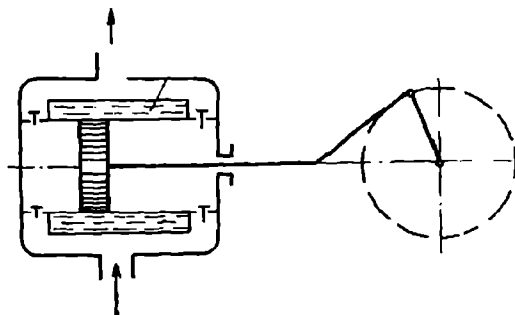
3.24- rasm. Ikki tomonlama harakatlanuvchi bir silindrlı kompressor.
