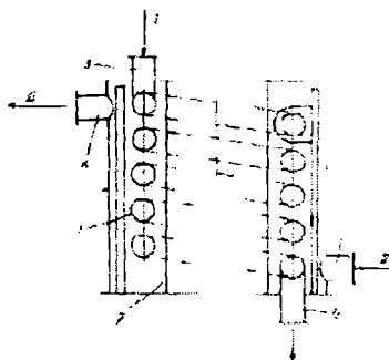
10.9-rasm. Zmeevikli issiqlik almashgich:
