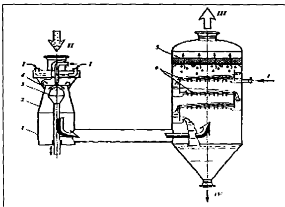
4.15-rasm. «Kox» firmasi gaz tozalash qurilmasining sxemasi: 1–Venturi quvuri; 2–diffuzor; 3–boshqaruvchi konus; 4–konfuzor; 5–toʻrli qaytargich (demister); 6–klapanli tarelkalar. Oqimlar: I–suv; II–dastlabki gaz; III–tozalangan gaz; IV–chiqindilar.
