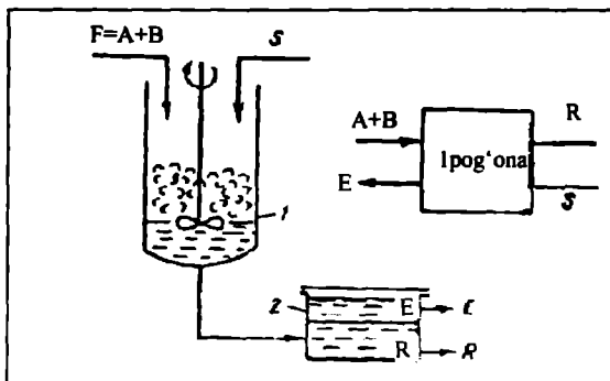
17.5-rasm. Bir pog'onali ekstraksiyalashning sxemasi: 1–aralashtirgich; 2–tindirgich; F–dastlabki eritma; A,V–aralashma komponentlari; S–ekstragent; E–ekstrakt; R–rafinat.
