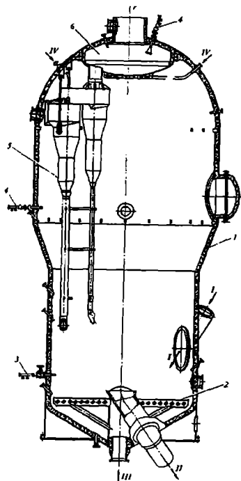
21.6 rasm. Changsimon katalizatorli regeneratori:
