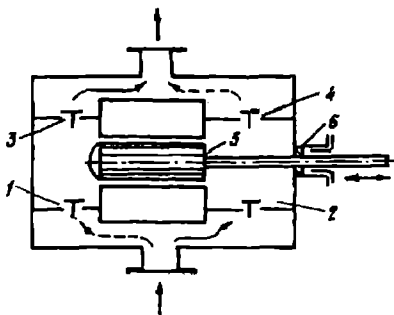
3.8-rasm. Ikki tomonlama ishlaydigan plunjerli nasos: 1, 2 – so‘ruvchi klapanlar; 3, 4-uzatuvchi klapanlar; 5 – so‘rish quvuri; 6-salnik.
