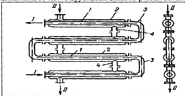
10.7-rasm. Qo'sh quvurli issiqlik almashgich:
