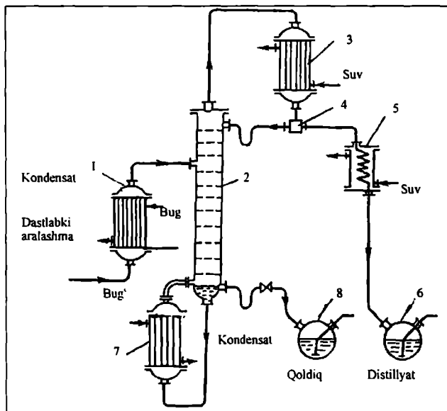
13.7-rasm. Uzluksiz ishlaydigan rektifikatsion qurilma sxemasi: 1—isitkich; 2—rektifikatsion kolonna; 3—deflegmator; 4—ajratgich; 5—sovitkich; 6—distillyat uchun yig'gich; 7—qaynatgich; 8—qoldiq mahsulot uchun yig'gich.
