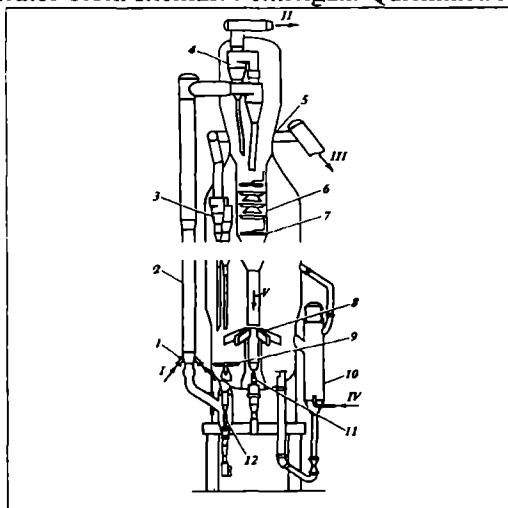
21.10-rasm. «Kellog» firmasi katalitik kreking qurilmasining reaktor-regenerator bloki:
