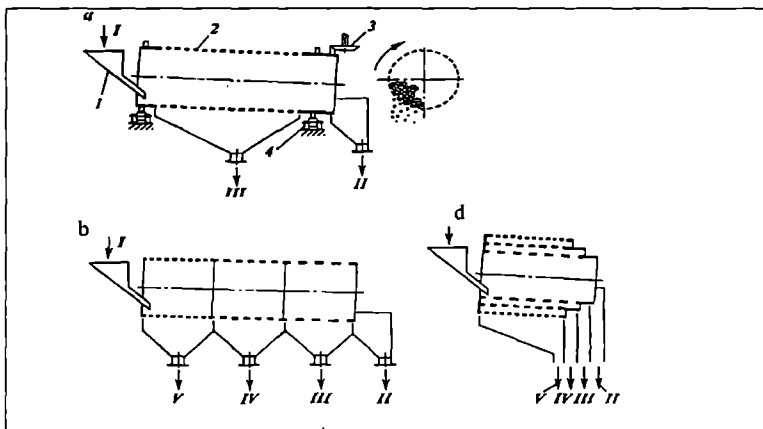
8.2-rasm. Barabanli sim g'alvirli uskunalarining sxemalari: a–bitta g'alvirli: 1–dastlabki materialni berish uchun tarnov; 2–baraban; 3–uzatma moslamasi; 4–tayanch roligi; b–g'alvirlarning ketma-ket joylanishi; d–g'alvirlarning markaziy o'qqa parallel joylanishi. Oqimlar: I–dastlabki material; II–katta o'lchamli fraksiya; III, IV, V–zarrachalarning o'lchami kichrayib boradigan fraksiyalar.
