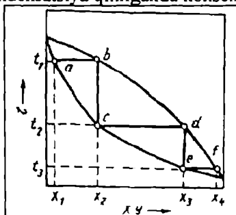
13.5-rasm. Binar aralashmalarni rektifikatsiya usuli bilan ajratishning diagrammada tasvirlanishi.
