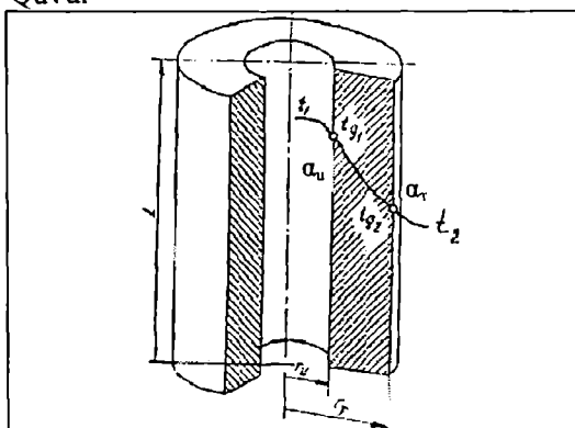
9.2-rasm. Silindrsimon yuzadan issiqlik o'tishining sxemasi.
