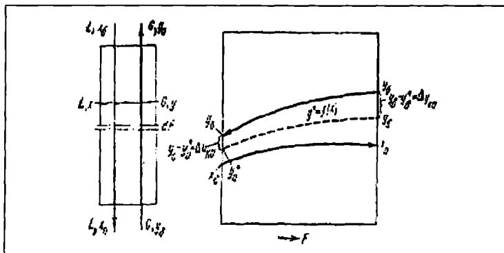
12.2-rasm. Modda o'tkazishning harakatlantiruvchi kuchini aniqlashga doir.
