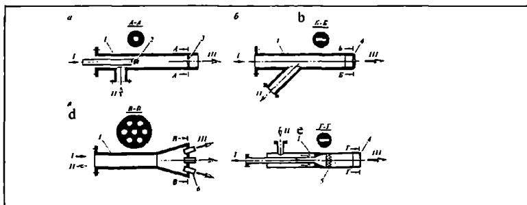
21.8-rasm. Katalitik kreking qurilmalari uchun mo'ljallagan sochib beruvchi soplolarning turlari:
