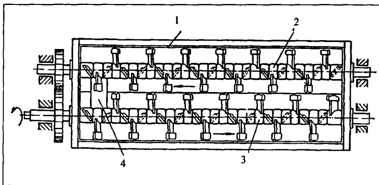
8.8-rasm. Ikkita vali bo'lgan qarama-qarshi oqimli aralashtirgichning sxemasi: 1-qobiq; 2,3-shnekli vallar; 4-tushirish teshigi.
