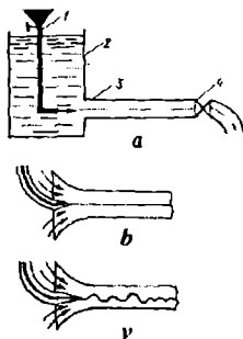
2.7-rasm. Reynolds tajribasi: a ) uskuna sxemasi; 1- rangli suyuqlik yuboriladigan naycha; 2- suyuqlik to'ldirilgan idish; 3- suyuqlik oqadigan quvur; 4- suyuqlik harakatini rostlab turuvchi kran; b ) quvurdagi suyuqlikning laminar harakati; d ) quvurdagi suyuqlikning turbulent harakati.
