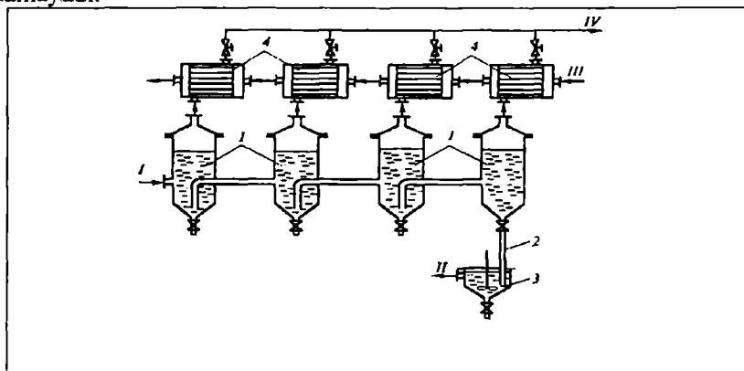
19.10-rasm. Ko'p korpusli vakuum-kristallanish qurilmasining sxemasi: 1–kristallizatorlar(korpuslar); 2–barometrik quvur; 3–gidravlik zatvor; 4–kondensatorlar; I–dastlabki eritma; II–kristallizat; III–sovituvchi suv; IV–kondensat.
