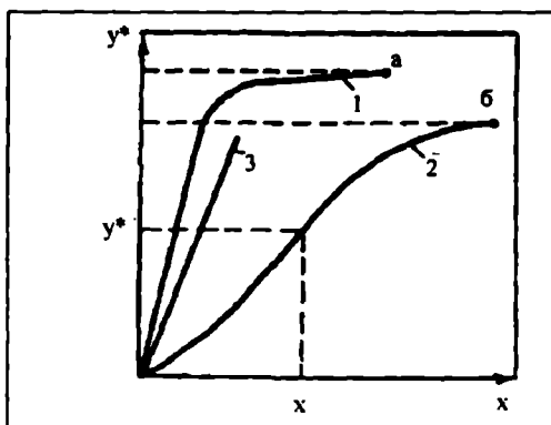
17.1-rasm. Ekstraksiyalash izotermalari: 1, 2 - u^* = f(x) ; 3 - u^* = mx .
