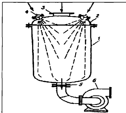
10.16-rasm. To‘g‘ri yo‘nalishli aralashtiruvchi kondensator: 1—kondensator qobig‘i; 2—qopqoq; 3—bug‘ning kirishi uchun patrubka; 4—sochib beruvchi soplo; 5—suv, kondensat va havoni chiqarish uchun patrubka; 6—nasos.
