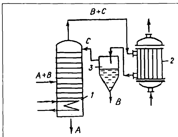
13.14-rasm. Azeotrop rektifikatsiyalash qurilmasi: 1–kolonna; 2–deflegmator; 3–cho'ktirish uskunasi.
