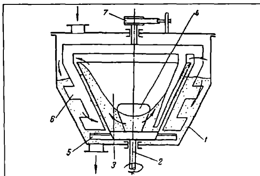
8.9-rasm. Aylanuvchi konusli aralashtirish uskunasi sxemasining 1-qobiq; 2-val; 3-konus; 4-oynak; 5-parrakli aralashtirgich; 6-rama; 7-to'xtatish uchun moslama.
