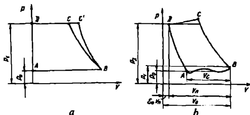
3.26-rasm. Bir bosqichli porshenli kompressorning indikator diagrammasi:
