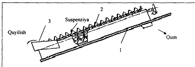
8.4-rasm. Spiralli sinflash uskunasiining sxemasi:
