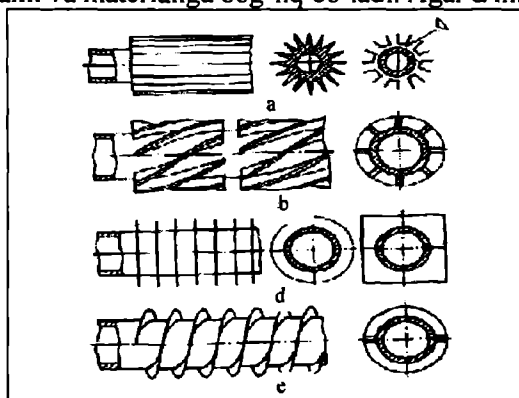
10.14-rasm. Qirrali quvurlar: a) bo'ylama qirrali; b) kesilgan qirrali; d) ko'ndalang qirrali; e) spiralsimon qirrali.
