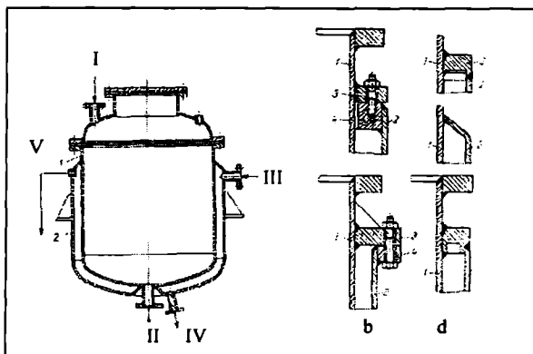
10.12-rasm. G'ilofli issiqlik almashgich(a) va g'ilofni uskunaga biriktirish usullari (b—flanes yordamida; d—payvandlash yo'li bilan): 1—idishlarning qobiqlari; 2—isitiuvchi g'iloflar; 3—halqalar; 4—flaneslar. Oqimlar: I—sovuq suyuqlik; II—issiq suyuqlik; III—bug'; IV—kondensat; V—havo.
