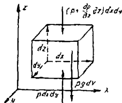
2.5-rasm. Harakatdagi suyuqlikning Eylér tenglamasini aniqlashga doir.
