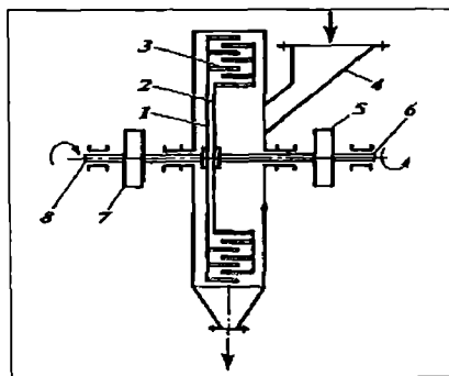
7.6-rasm. Dezintegratorning tuzilish sxemasi:
