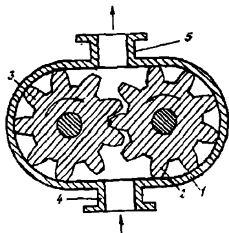
3.9- rasm. Shesternyali nasos: 1-qobiq; 2, 3-bir-biriga ilashgan tishli shesternyalar; 4 – soʻruvchi patrubka; 5 – haydash trubka.
