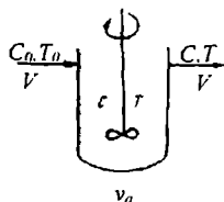
2.15- rasm. Ideal siqib chiqarish uskunasi-ning sxemasi.
