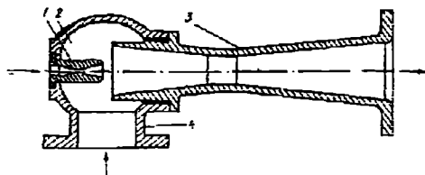
3.30-rasm. Ingichka oqimli bug' vakuum-nasosi:
