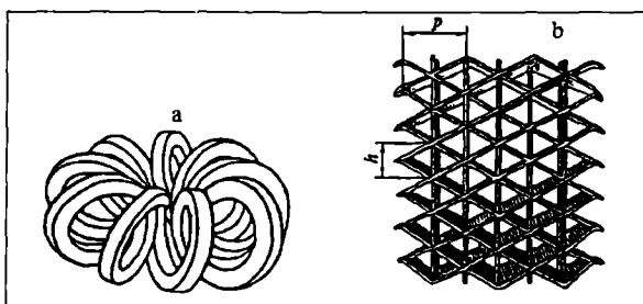
15.11-rasm. Gidravlik qarshiligi kichik va yuqori samaradorlikka ega bo'lgan nasadkalar:
