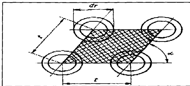
10.20-rasm. Bitta quvur uchun to'ringning foydali maydonini aniqlashga doir.
