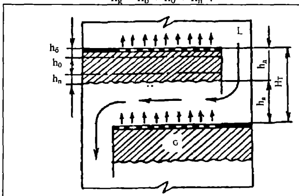
17.14-rasm. Tirgovuch balandligini va tarelkalar orasidagi masofani aniqlash.
