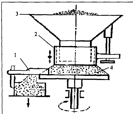
8.7-rasm. Tarekali ta'minlagichning sxemasi: 1–buriluvchi pichoq; 2–manjeta(qadama eng); 3–qabul qiluvchi bunker; 4–tarekka.
