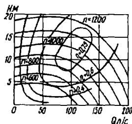
3.5-rasm. Markazdan qochma nasosning universal xarakteristikasi.
