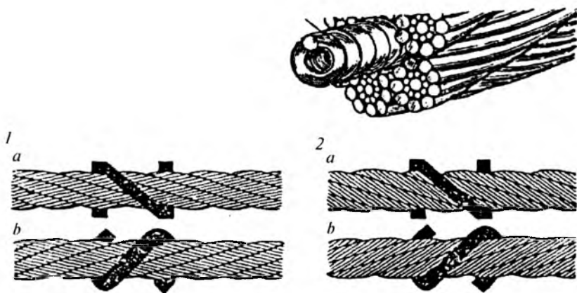
3.7-rasm. Har xil o'ramli po'lat arqonning ko'rinishi: 1 – xoch o'ramli; 2 – bir tomonlama o'ramli; a – o'ng; b – chap.
