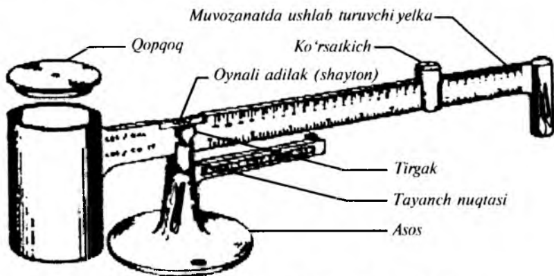
7.2- rasm. Yulkali tarozining umumiy ko'rinishi.
