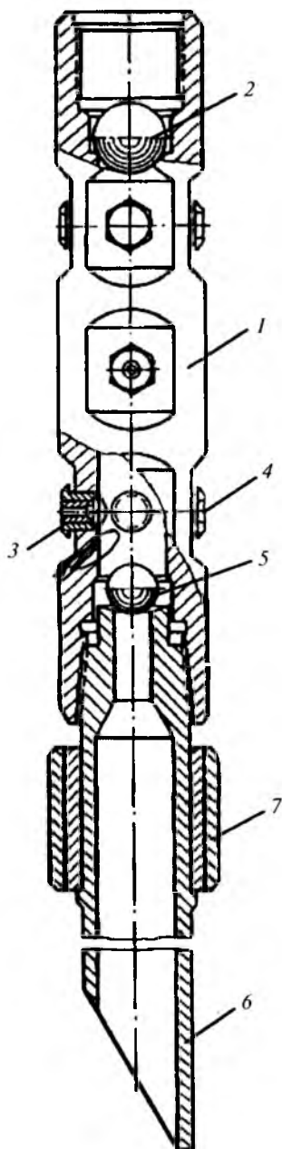
13.2- rasm. Qum aralash oqimli API6M perforatori:
