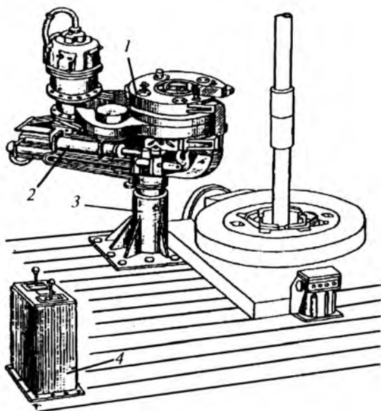
3.10-rasm. AKB-3M turdagi avtomatik burg'ilash kalitining umumiy ko'rinishi:
