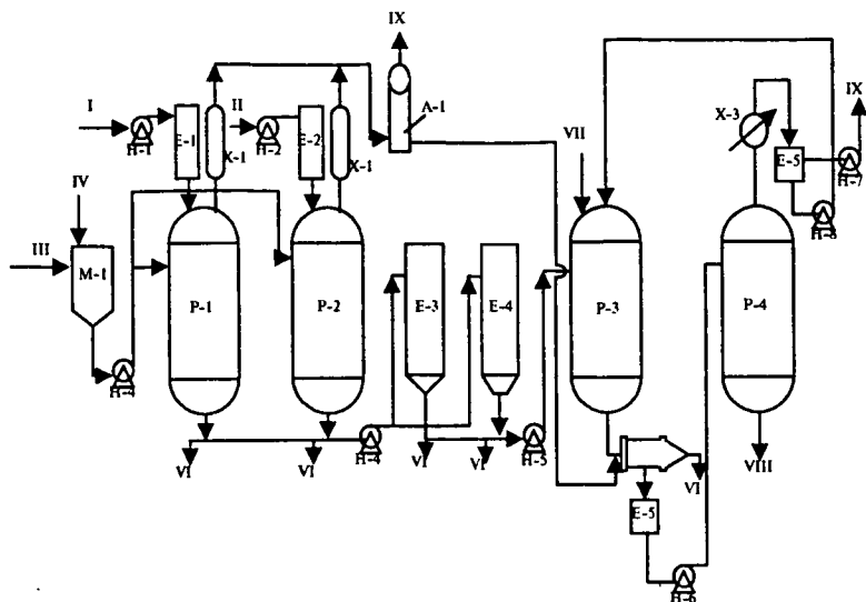
10-rasm. DF – 11 qo‘ndirmani olish texnologiyasi:
