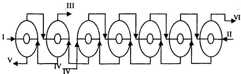
3-rasm. Aralashtirgich – tindirgichlardagi oqimlarning chizmasi:
