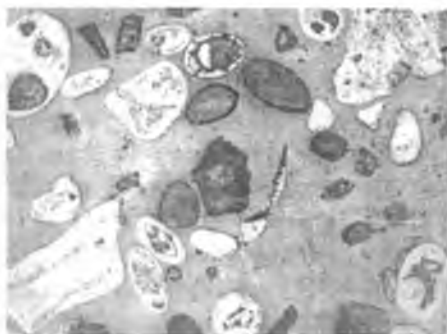
67-rasm. Donali fosforitlar organogen strukturasiining fotosurati. Paleogen. Qizilqum
