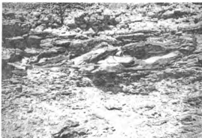
65-rasm. Qatlamli temirli jinslarning fotosurati. Yuqori bo'r. Sulton Uvays tog'lari
