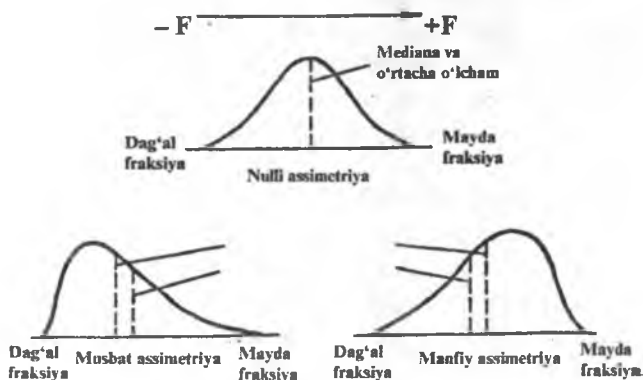
18-rasm. Granulometrik tarkibning musbat va manfiy asimmetriyalari egri chizig'i
