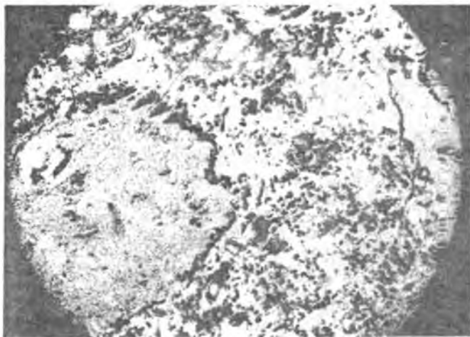
43-rasm. Tufolava strukturasiining mikrofotosurati. Zarra binda 30 marta kattalashtirilgan
