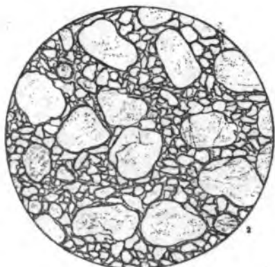
40-rasm. Kvarsitga aylangan qumtoshning mikrofotosurati. Zarrabinda 30\times kattalashtirilgan
