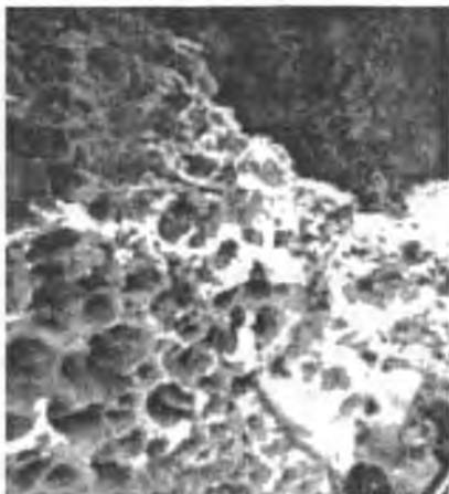
2-rasm. Karbonatli jinslarning erishi tufayli hosil bo'lgan o'yiqliklar
