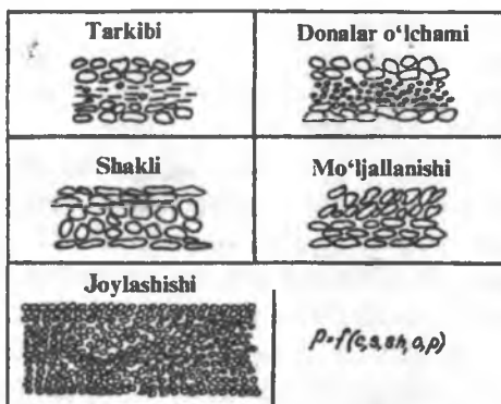
29-rasm. Struktura hosil qiluvchi donalarning tarkibi, o'lchami, shakli, mo'ljallanishi va joylashish tartibi bo'yicha qat-qatlanish
