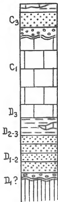
71-rasm. Ikkinchi fatsial zonallik qonunini tushuntiruvchi stratigrafik ustun. Qo'shaloq to'liqlik chiziq cho'kindi hosil bo'lishdagi uzilishni bildiradi. Boshqa shartli belgilar 70-rasmga berilgan
