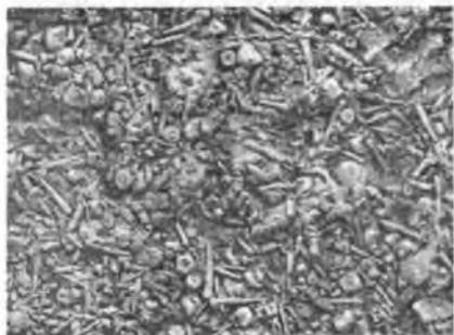
57-rasm. Organogen ohaktoshlarda dengiz nilufarlari qoldiqlarining mikrofotosurati
