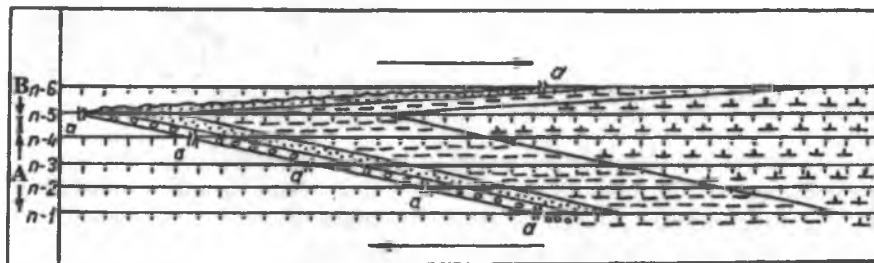
74-rasm. To'rtinchi fatsial zonallik qonunini tushuntiruvchi chizma. To'liqlik chiziqlar – yuvilish yuzasi. Shartli belgilar 72-rasmda berilgan
