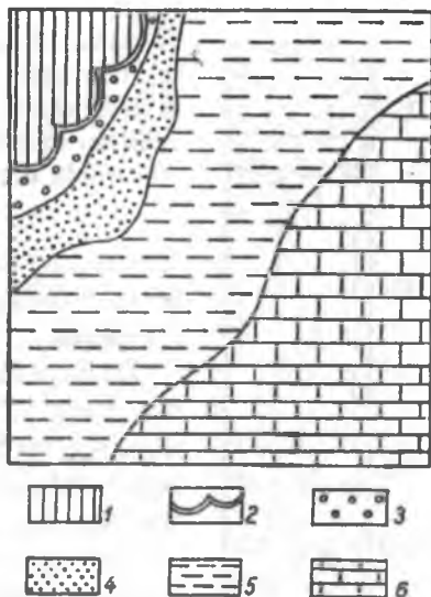
70-rasm. Birinchi fatsial zonallik qonunini tushuntiruvchi chizma.
