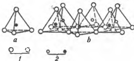
45-rasm. Gil minerallari kristall panjarasida oktayedr (a) va oktayedr to'ring (b) sxematik tasviri. 1-gidroksillar; 2-alyuminiy, magniy va b.
