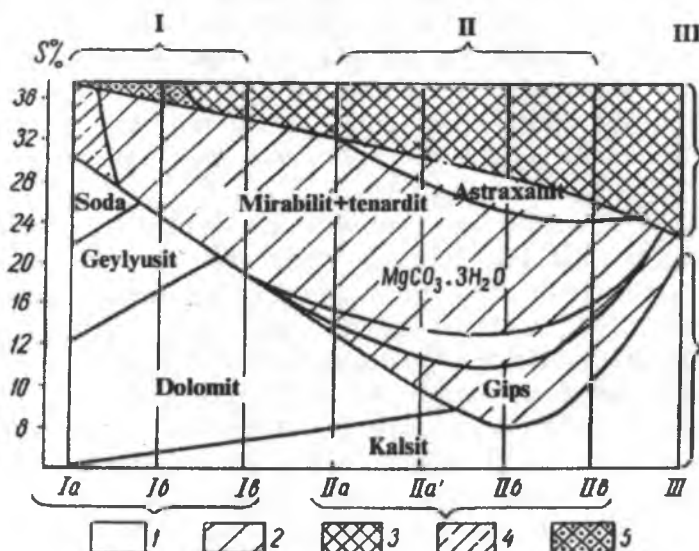
68-rasm. Qurg'oqchil zonalaridagi hozirgi ko'llarda galogenezning umumiy chizmasi (N.M.Straxov bo'yicha). I-sodali ko'llar; Ia-kuchli sodali (Shk>30%); Ib-mo'tadil sodali (Shk 30-3%); kuchsiz sodali (Shk <3%); II-sulfatli ko'llar; IIa-natriy-magniyli; IIa"-magniy-natriyli; IIb-natriy-magniy-kalsiyli; IIv-magniy-kalsiyli; III-NaCl, MgCl 2 , CaCl 2 ga ega bo'lgan xloridli ko'llar. 1-karbonatli bosqich; 2-sulfatli bosqich; 3-xloridli bosqich; 4-soda qo'shimchasi ko'p bo'lgan sulfatli cho'kindilar; 5-natriy sulfatlari qo'shimchalari ko'p bo'lgan galit
