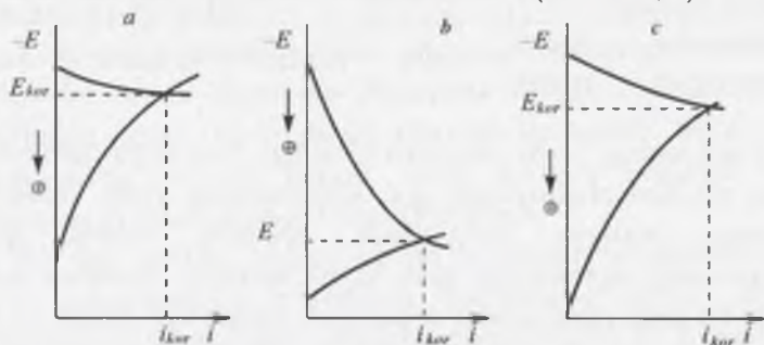
6.5-rasm. Tuproq korroziyasi sharoiti turlicha bo'lgan holatlar uchun korroziya jarayonining nazorat turlari.
