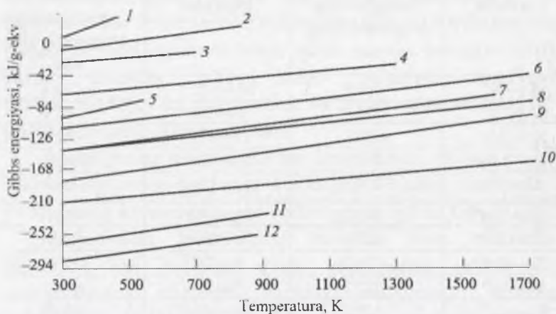
3.1-rasm. Ba'zi metall oksidlarining hosil bo'lishiga \Delta G^0 haroratning ta'siri:
