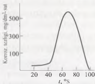
7.16-rasm. Haroratning distillangan suvdagi Zn korroziyasi tezligiga ta'siri
