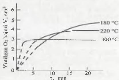
3.7-rasm. Kislorodning turli haroratlarda kumushda adsorbsiyalanish kinetikasi ( P_{O_2} = 200 mm sm ust).
