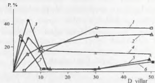
9.1-rasm. Turli himoyalash usullari R solishtirma og'irligi bilan po'lat konstruksiyalarining talab qilinadigan ishlash muddati D ga bog'liq holda korroziyaga qarshi qo'llaniladigan vositalar hajmida taqsimlanishi.
