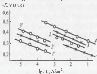
4.17-rasm. Parsial erish tezliklarining potentsialga bog'liqligi. Fe-0,85% Cr qotishmadagi temir (1—4) va xrom (1'—3') uchun, rNning turli qiymatlarida: 1, 1'—0,03; 2, 2'—1,84; 3, 3'—3,01; 4, 4'—3,91;
