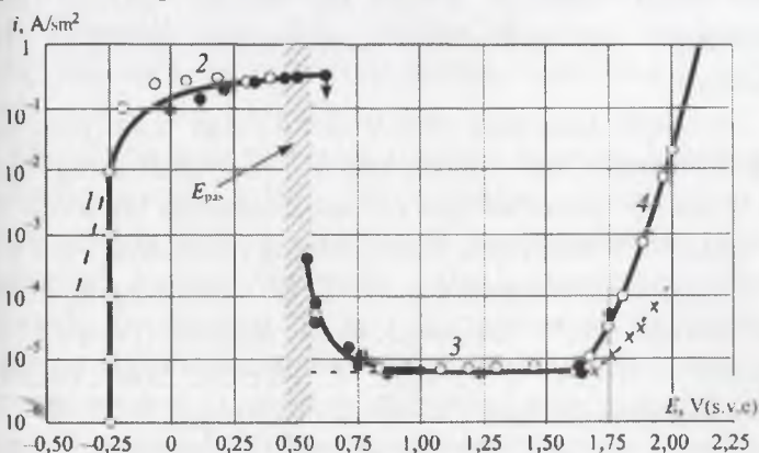
4.22-rasm. Deaeratsiyalangan 0,5 M H_2SO_4 eritmasida 25°C uchun temirning statsionar anod qutblanish egriliklari.
