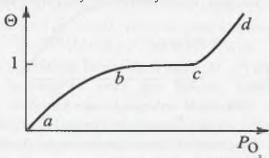
3.5-rasm. Kislorod uchun adsorbsiya izotermasi.
