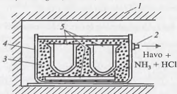
9.3-rasm. Termoalumiylash jarayonining sxemasi.
