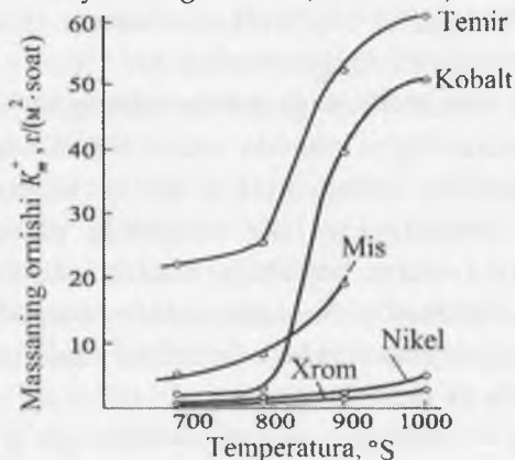
3.16-rasm. Kislorod atmosferasida ba'zi metallarning oksidlanish tezligi
