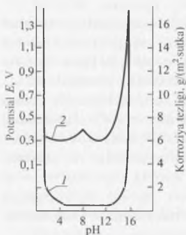
7.11-rasm. Alumiiniy uchun 24 soatda korroziya tezligining – (1) va elektrod potensialining xloridli eritma pH ga bog'liqligi
