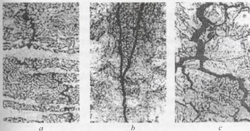
5.5-rasm. 200 mg/l Sl^- konsentratsiyali, 320°S haroratli suvdagi po'latlarning tipik korroziyon yorilishi ( \times 900 ):
