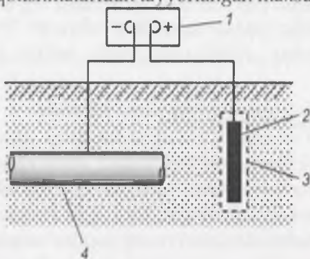
10.2-rasm. Katod himoyasi qurilmasining sxemasi.
