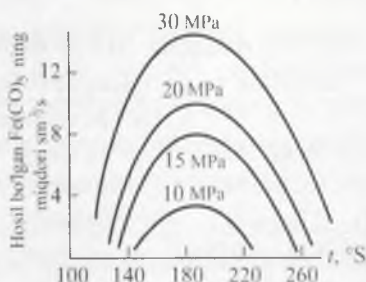
6.12-rasm. Turli bosimlarda temir pentakarbonili hosil bo'lish tezligi-ning haroratga bog'liqlik grafigi
