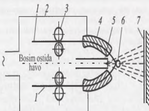
9.6-rasm. Elektrometallizator qurilmasining sxemasi.
