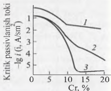
7.5-rasm. Fe-Cr qotishmasidagi xrom miqdorining eritmalar-dagi passivlanish kritik tokiga ta'siri:
