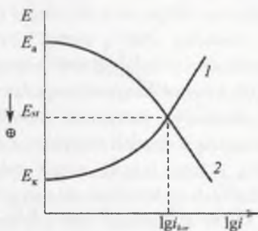
4.7-rasm. Depolyarizator razryadi (1) va metall ionizatsiyasi (2) reaksiyalari tezliklarining potensialga bog'liqligi.
