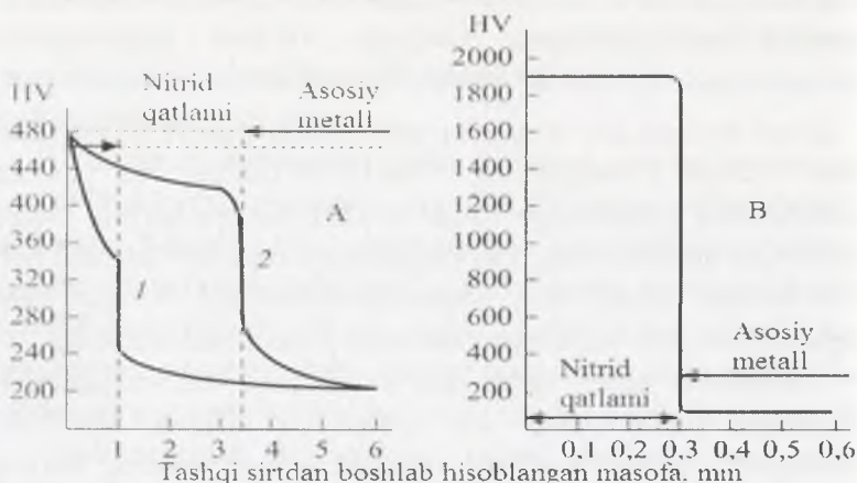
6.11-rasm. HV qattiqligining qalinlik bo'yicha o'zgarishi. A – ammiak sintezi kolannasidagi 18XZMB po'latdan tayyorlangan termopara cho'ntagi devori, 1 – 500–550 °S da 14000 soat ishlaganda; 2 – 51840 soat ishlaganda. B – ammiak sintezi kolannasidagi X18N10T po'latdan tayyorlangan Fild trubkasi devori, ≈ 500 °S da 30800 soat ishlaganda.
