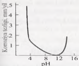
7.15-rasm. pH miqdorining Zn korroziyasiga ta'siri.
