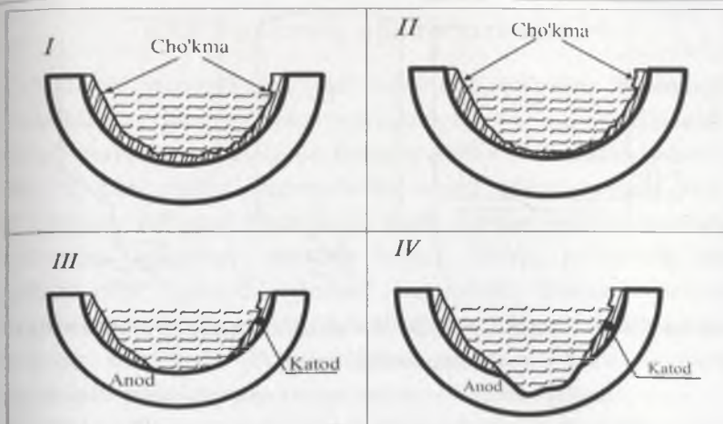
6.7-rasm. Ariqchali korroziya hosil bo'lishning asosiy bosqichlari:
