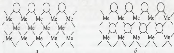
3.8-rasm. Metallda xemosorblangan qatlam (a) va metall oksidining (b) tuzilish sxemasi.
