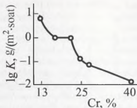
7.6-rasm. Xrom konsentratsiya-sining 10% li \text{FeCl}_3 \cdot 6\text{N}_2\text{O} eritmasidagi Fe-Cr qotishma-larining pitting korroziyasi tezligiga ta'siri
