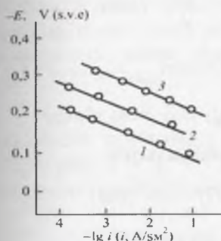
4.14-rasm. Sulfat konsentratsiyasi 1 n va turlicha pH da H_2SO_4 + Na_2SO_4 eritma-larida temir uchun anod qutblanish chiziqlari. pH: 1-0,2; 2-1,2; 3-2,3
