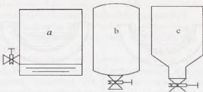
6.8-rasm. Suyuqligi pastdan bo'shatiladigan apparatlarning konstruksiyalari.
