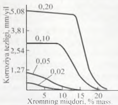
6.13-rasm. Neft bug'larida (650°C) xromli po'latlar korroziya tezligining xrom miqdoriga bog'liqligi.
