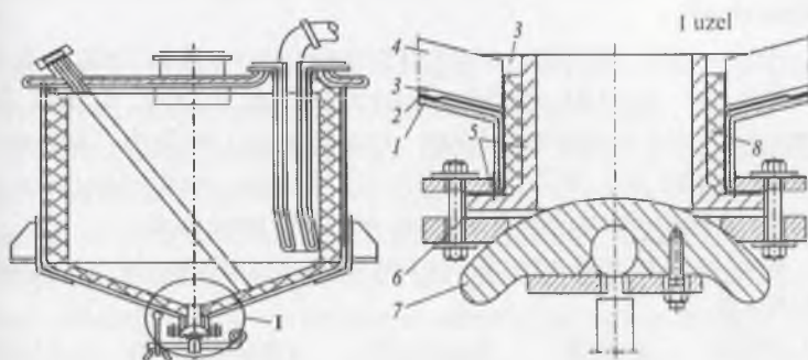
7.14-rasm. Yuvuvchi kislota to'plagichining antikorrozion himoyasi.
