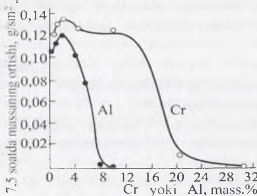
7.10-rasm. Havoda, 1200°S haroratda Fe–Cr va Fe–Al Qotishmalari oksidlanish tezligining qotishmadagi legirlovchi komponentlar miqdoriga bog'liqligi
