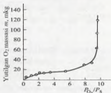
3.6-rasm. 77 K haroratda aluminiydagi kislorod adsorbsiyasining izotermasi (Skorchelletti ma'lumotlari bo'yicha).
