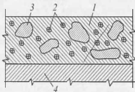
9.7-rasm. Lok-bo'yoq plyonkasi tuzilishining sxemasi.
