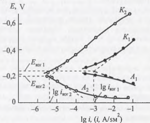
10.6-rasm. Ingibitor ta'sirining effektiv-ligini tushuntiruvchi qutblanish egriliklari.
