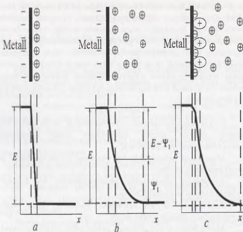
4.1-rasm. Qo'sh qavatda zaryadlar taqsimoti va potensialning o'zgarishi.
