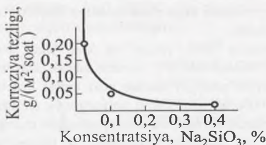
10.8-rasm. Neytral suvli eritmalarida po'lat korroziyalanish tezligining Na 2 SiO 3 konsentratsiyasiga bog'liqligi
