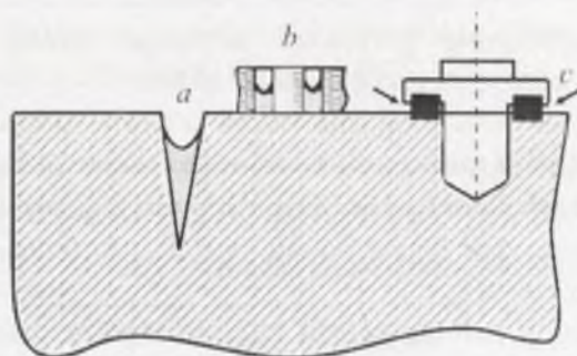
6.3-rasm. Buyum konstruktiv xususiyatlari ning kapllyar kondensatsiya markazlariga markaz-lariga ta'siri va atmosfera korro-ziyasining kuchayishi.
