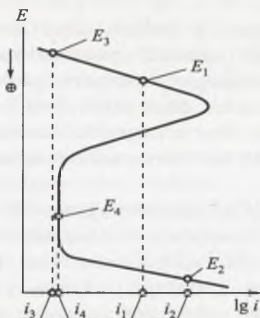
10.1-rasm. Elektrokimyoviy himoyada metall erish tezligini pasaytirish usullari.
