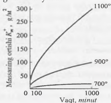
3.11-rasm. Yuqori haroratlarda temirning havoda oksidlanish parabolik egriliklari.
