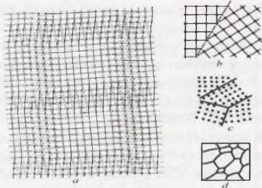
2.2-rasm. Oddiy kub panjarada chegaralarning ko'rinishi. a – buralish chegarasi; b – kogerent qo'shloq chegara; c, d – katta burchak ostida joylashgan orientirlashgan donalar chegaralari (d – umumiy ko'rinish).
