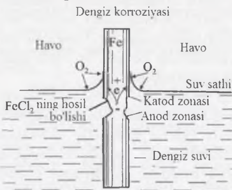
6.6-rasm. Dengiz suviga botgan temirning korroziyalanish sxemasi.
