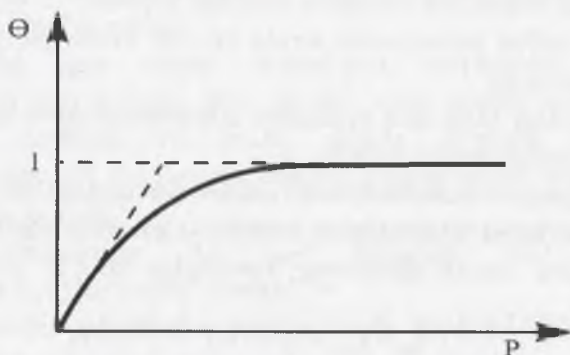
3.3-rasm. Lengmyur izotermasi
