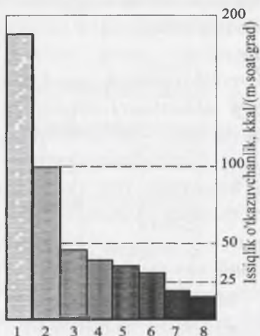
8.3-rasm. Uglerod-grafitli materiallar va metallarning issiqlik o'tkazuvchanligi.
