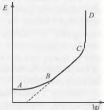
4.6-rasm. Qutblanish egriligining umumiy ko'rinishi
