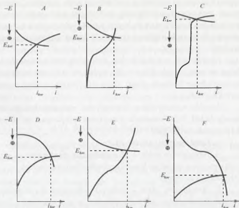
4.12-rasm. Korroziya jarayoni nazoratining ko'rinishlari.
