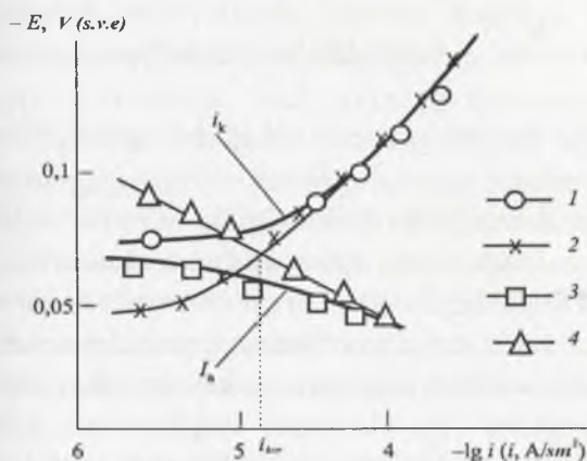
4.9-rasm. 1 n. \text{H}_2\text{SO}_4 dagi nikelda o'lchangan katod (1) va anod (3) qutblanish egriliklari.
