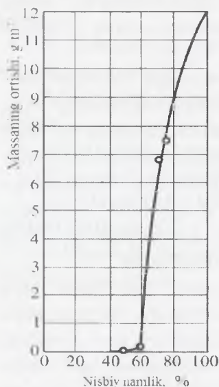
6.1-rasm. Temirning tarkibi-da 0,01% (hajm) SO 2 bo'lgan havodagi korroziozitalanishi. Saqlanish muddati 55 kun.
