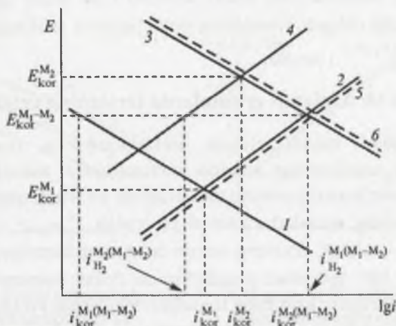
4.13-rasm. M_1(1,2) va M_2(3,4) metallar uchun E - \lg i_a (1,3) va E - \lg i_k (2,4) bog'lanish-larning grafiklari. Shuningdek M_1 (1, 2) va M_2 (3, 4) kontaktlashuvchi metallar tizimi uchun katod (5) va anod (6) yig'indi tok zichliklarining potensialga bog'liqligi.
