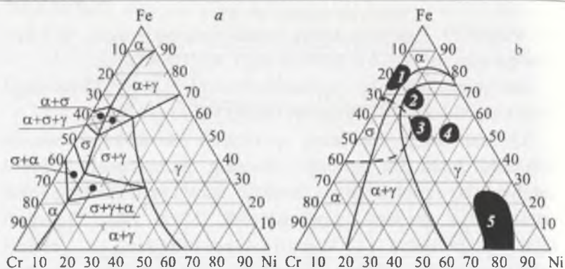
7.8-rasm. Fe-Ni-Cr sistemasi uchun 400 °S (a) va xona (b) haroratida fazaviy muvozanat qirgimi.
