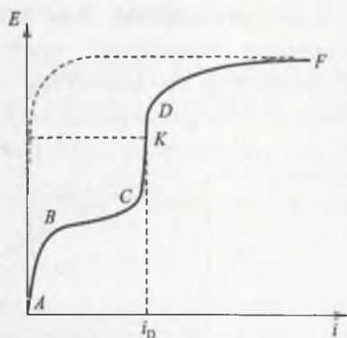
4.10-rasm. Kislorod-vodorod depolyarizatsiya jarayoni uchun umumiy qutblanish egriligi
