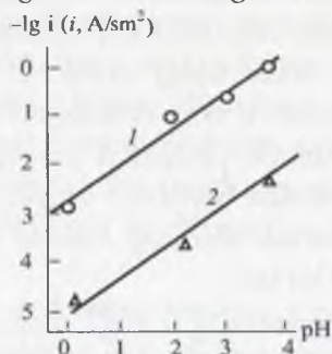
4.18-rasm. Eritma pH ning parsial erish tezligiga ta'siri. E = -0,34 V bo'lganda \text{N}_2\text{SO}_4 + \text{Na}_2\text{SO}_4 eritmalaridagi Fe-0,85% Cr qotishmasidagi temir (1) va xrom (2) uchun.
