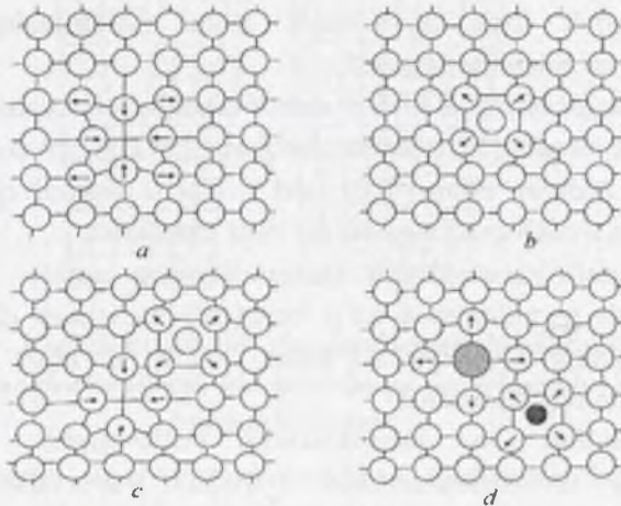
2.1-rasm. Kristallardagi nuqtaviy defektlarning ko'rinishlari.
