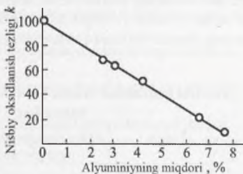
3.19-rasm. Temirni aluminiiy bilan 900°S haroratda legirlashning oksidlanish nisbiy tezligiga bog'liqligi
