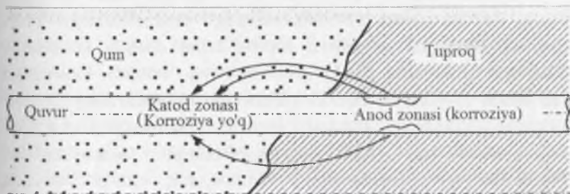
6.4-rasm. Turli aeratsiyali tuproq sharoitida yotqizilgan quvur o'tkazgichning korroziyalanish sxemasi.
