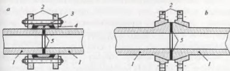
8.1-rasm. Sitall quvurlarni ulash usullari.
