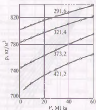
Рис. 2.10. Зависимость плотности конденсата Астраханского месторождения от давления при различных температурах, К
