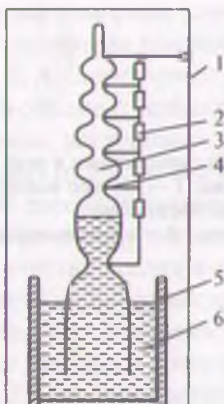
Рис. 2.4. Пьезометр Михельса: 1 — камера высокого давления; 2 — сопротивление; 3 — стеклянный пьезометр; 4 — платиновые контакты; 5 — стакан с ртутью; 6 — ртуть
