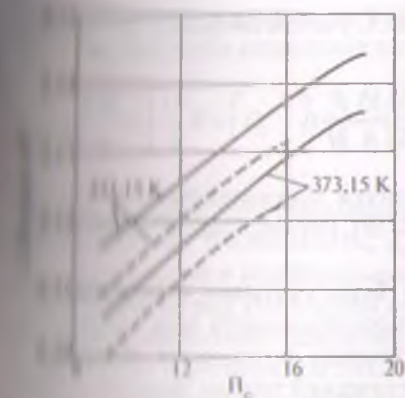
Рис. 4.11. Зависимость коэффициента теплопроводности нормальных парафинов (пунктирная линия) и олефинов (сплошная линия) от числа атомов углерода в молекуле [8]
