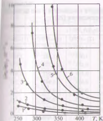
Рис. 3.15. Температурная зависимость величины (\partial\eta/\partial P)_T для фракций газового конденсата Опoшнинского месторождения: 1 — фракция н.к.—95°C; 2 — 122—150 °C; 3 — 175—200 °C; 4 — 225—250 °C; 5 — 275—300 °C; 6 — 325—к.к.
