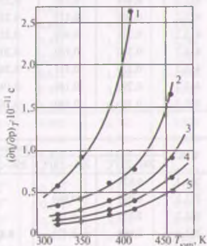
Рис. 3.18. Зависимость величины (\partial\eta/\partial P)_T от средней температуры кипения для фракций газового конденсата Оренбургского месторождения при температурах: 1 — 250 K; 2 — 300 K; 3 — 350 K; 4 — 400 K; 5 — 450 K
