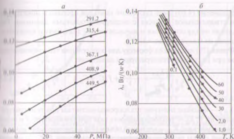
рис. 4.26. Экспериментальные значения коэффициента теплопроводности тяжелого конденсата астраханского месторождения: а) изотермы теплопроводности при различных давлениях; б) изобары теплопроводности при различных температурах
