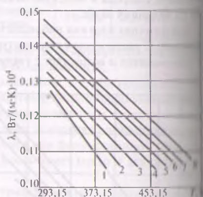
Рис. 4.10. Температурная зависимость коэффициента теплопроводности олефинов при атмосферном давлении [8]: 1 — n -нонен-1; 2 — n -децен-1; 3 — n -ундецен-1; 4 — n -додецен-1; 5 — n -тридецен-1; 6 — n -тетрадецен-1; 7 — n -пентадецен-1; 8 — n -гептадецен-1
