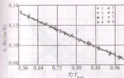
Рис. 4.18. Зависимость \lambda = f(T/T_{кип}) для олефиновых углеводородов [8]: 1 — нонен-1; 2 — децен-1; 3 — ундецен-1; 4 — додэцен-1; 5 — тридецен-1; 6 — тетрадецен-1; 7 — пентадецен-1; 8 — гексадецен-1
