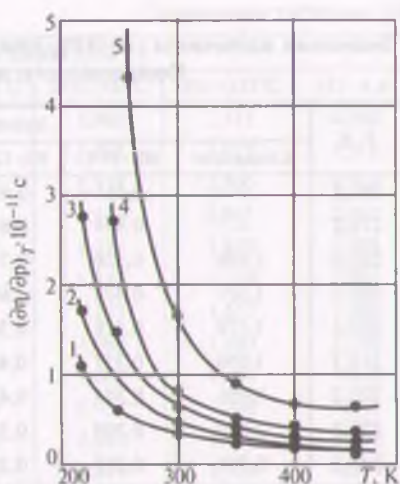
Рис. 3.16. Температурная зависимость величины (\partial\eta/\partial P)_T для фракций газового конденсата Оренбургского месторождения: 1 — фракция н.к.—60°C; 2 — 60—95°C; 3 — 95—122 °C; 4 — 122—150 °C; 5 — 150—к.к.
