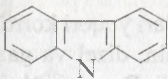
karbazol
