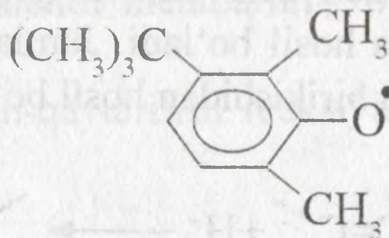
2,4,6-tritretbutilfenoksil
