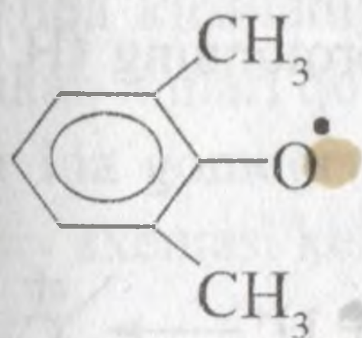
o,o-dimetilfenoksil
