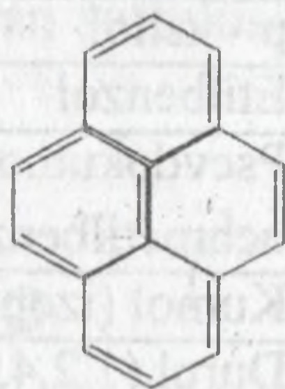
piren
