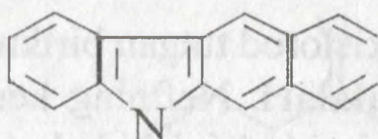
benzkarbazol
