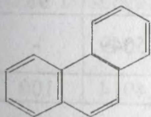
fenantren
