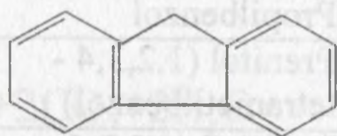
Fluoren
