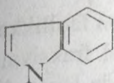
indol
