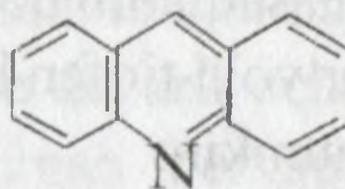
akridin
