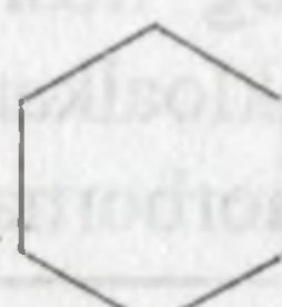
Siklogeksan
