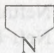
pirrol
