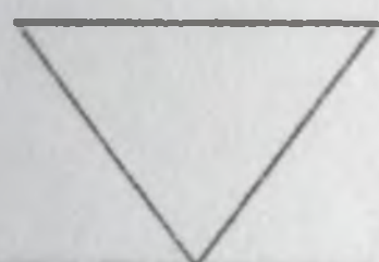
Siklopropan
