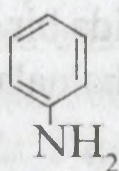
anilin
