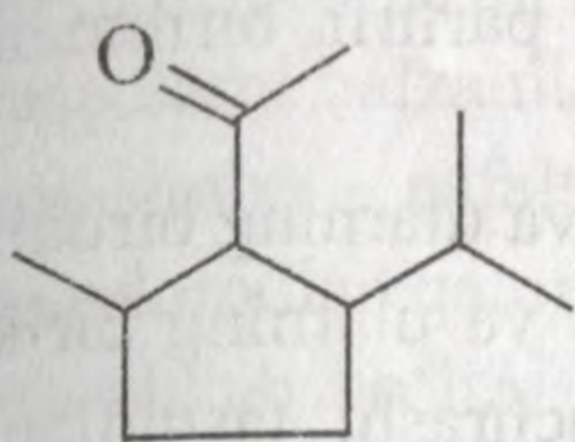
atsetilizopropil- metilsiklopentan
