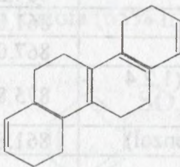
xrizen
