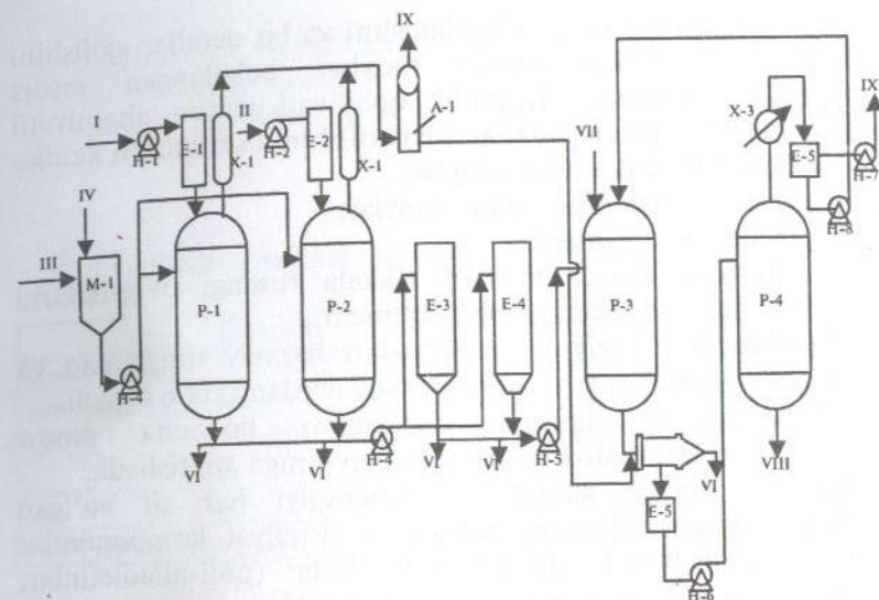
10-rasm. DF – II qo'ndirmaning olish texnologiyasi: I – izobutil spirt, II – izooktil spirt, III – mineral moy, IV – P_2S_5 , V – butil spirt, VI – chiqindilar, VII – ZnO, VIII – tayyor qo'ndirma, IX – kondensirlangan gazlar.
