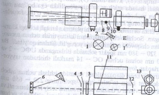
2.7-rasm. CΦ – 4 spektrofotometrning optik chizmasi.
