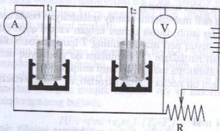
3.4-rasm. Moddaning solishtirma issiqlik sig'imini aniqlash uchun tajriba chizmasi (2-usul).
