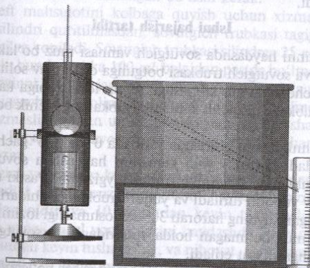
1.1- rasm. Suyuq yoqilg'i, erituvchilar va tiniq neft mahsulotlarini haydovchi standart qurilmaning ko'rinishi.
