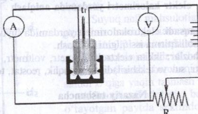
3.3-rasm. Moddaning solishtirma issiqlik sig'imini aniqlash tajriba chizmasi (1-usul).
