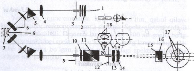
2.5-rasm. CФ — 18 spektrofotometrining optik chizmasi.
