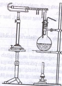
4.1-rasm. Yuqori haroratlardagi zichlikni aniqlashga mo'ljallangan qo'shimcha qurilmali Vestfal-Mor tarozisi.
