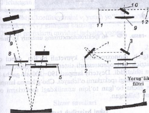
2.3-rasm. CФ — 46 spektrofotometrning optik chizmasi.
