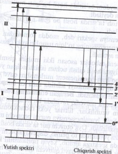
2.9 -rasm. Elektron sathlardagi nurlanishlar.
