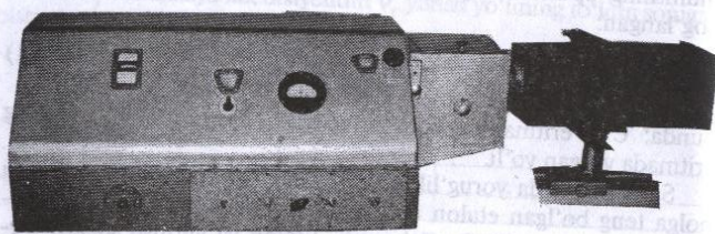
2.8-rasm. СФ — 4 markali spektrofotometrning umumiy ko'rinishi.
