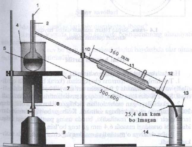
1.3-rasm. Suyuq bitum mahsulotlarini haydash uchun mo'ljallangan standart qurilma.
