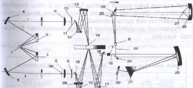
2.1-rasm. ИКC – 14 spektrofotometrining optik chizmasi.
