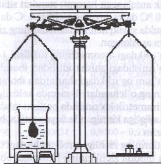
4.3-rasm. Gidrostatik tortish yo'li bilan zichlikni aniqlovchi qurilma.
