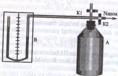
4.4-rasm. Tajriba qurilmasi.
