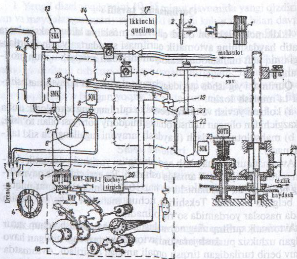
1.2 -rasm. Fraksiyalarga ajratib haydashning avtomatik qurilmasi.
