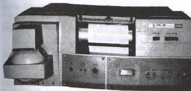
2.6 -rasm. CФ — 18 spektrofotometrining umumiy ko'rinishi.
