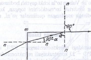
3.11 -rasm. Havo/shisha/neft mahsuloti chegarasidagi to'la ichki qaytish.
