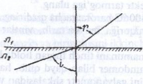
3.10-rasm. Ikki muhit chegarasidan o'tayotgan yorug'lik nurining sinishi.
