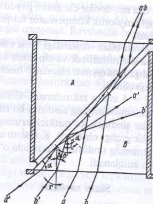
3.13 -rasm. АББЕ rusumidagi refraktometr prizmalaridagi nurlarning yo'li.
