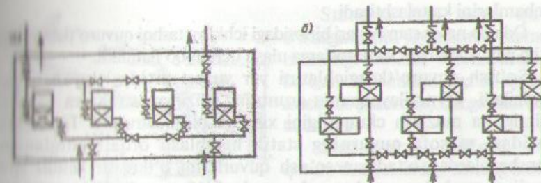
3.4-rasm. So'rish va siquv quvurlaridagi kollektorli ulanishlar. a) - suv ikki so'rish quvuri orqali 4 ta nasosga olib borilishi; b- 4 ta nasosning turli tizimda ham ishlashini ta'minlovchi 6 ta nasosning 3 so'rish quvurini kollektorli ulash
