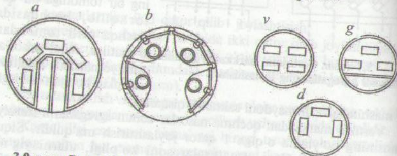
3.9-rasm. Doira shaklidagi mashinalar binosida agregatlarning joylashishi
