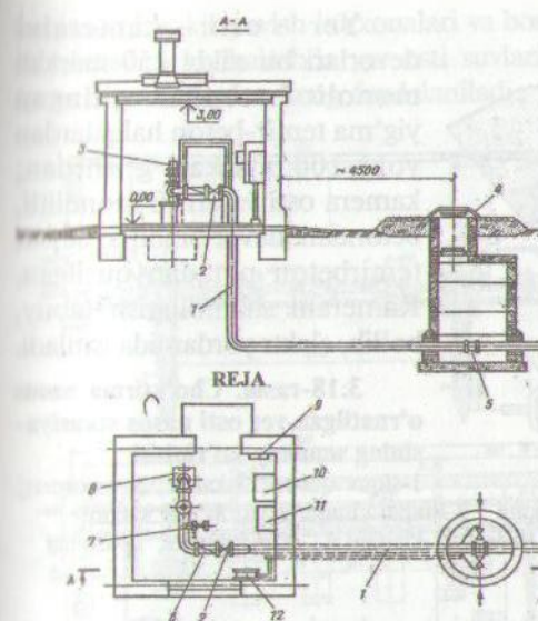
3.17-rasm. Cho'ktirma nasos bilan jihozlangan, yer ustida joylashgan nasos stansiyasi.
