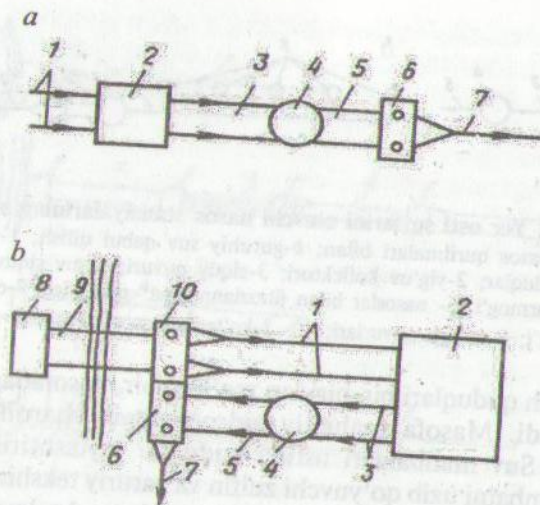
1.3-rasm. II-ko'taruv nasos stansiyalarining prinsipial sxemalari a -aloqida joylashgan; b -birlashgan; 1-I-ko'taruv nasoslarining siquv quvurlari; 2-tozalash inshootlari; 3-tozalash inshootlaridan toza suv rezervuarigacha bo'lan quvurlar; 4-toza suv rezervuarlari; 5-II-ko'taruv nasoslarining so'rish quvurlari; 6-II-ko'taruv nasos stansiyasi; 7-II-ko'taruv nasoslarining siquv quvurlari; 8-I-ko'taruv nasos stansiyasi; 9-o'zloqar quvurlar; 10- suv oluvchi inshootlar
