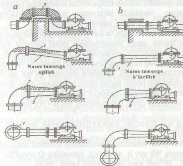
3.1-rasm. So'rish quvurlarini to'g'ri (a) va noto'g'ri (b) joylashishi 1 - havoli xalta; 2-to'g'ri o'tish; 3-qiya o'tish.
