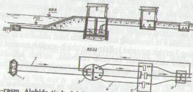
3.3 -rasm. Alohida tipdagi 1-ko'taruv nasos stansiyaning olib boruvchi va so'ruvchi quvurlari sxemasi. 1-kallak; 2-o'zi oqar tizim; 3-suv qabul qigich; 4-so'rish quvurlari; 5-stansiya; 6-o'chirib-yoqish kamerasi
