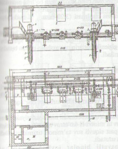
3.19-rasm Ikki quduqli birlashgan I, II ko'taruv nasos stansiyalari
