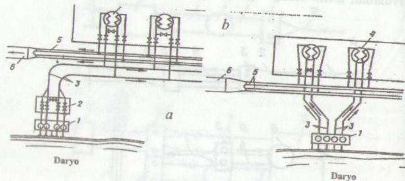
1.5-rasm. Issiqlik elektr stansiyalar (IES) ni suv bilan ta'minlash tizimi nasos stansiyalar chizmasi:
