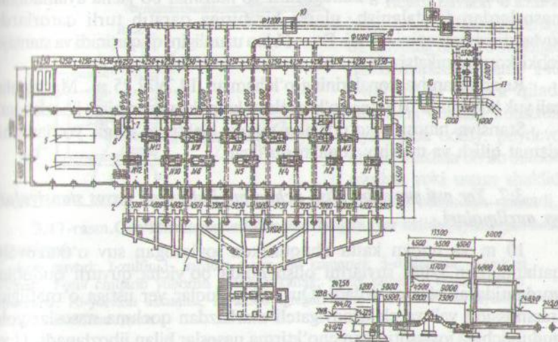
3.16-rasm. Braziliyaning yirik sanoat markazi suv ta'minoti tizimiga kiruvchi nasos stansiya
