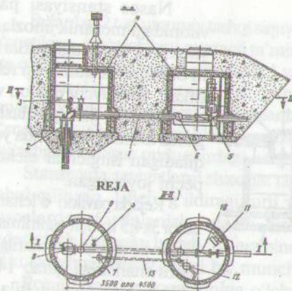
3.18-rasm. Cho'ktirma nasos o'rnatilgan yer osti nasos stansiyasining umumiy ko'rinishi
