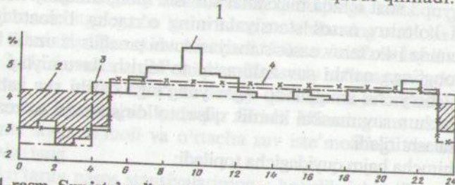
2.1-rasm. Suv iste'moli va nasos stansiyasining bir tekisda hamda pog'onali uzatishining birlashtirilgan grafi
