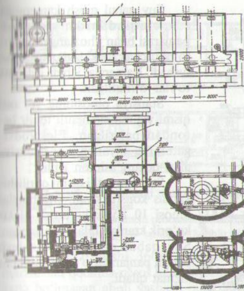
3.12-rasm. Tokio shahridagi suv ta'minoti tizimidagi 1-ko'taruv nasos stansiyasi
