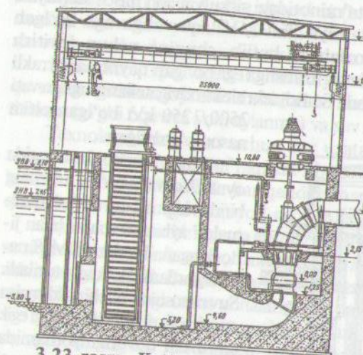
3.23-rasm. Katta quvvatli GRESning to'g'ridan-to'g'ri oquvchi suv ta'minoti tizimining sirkulyatsion nasos stansiyasi
