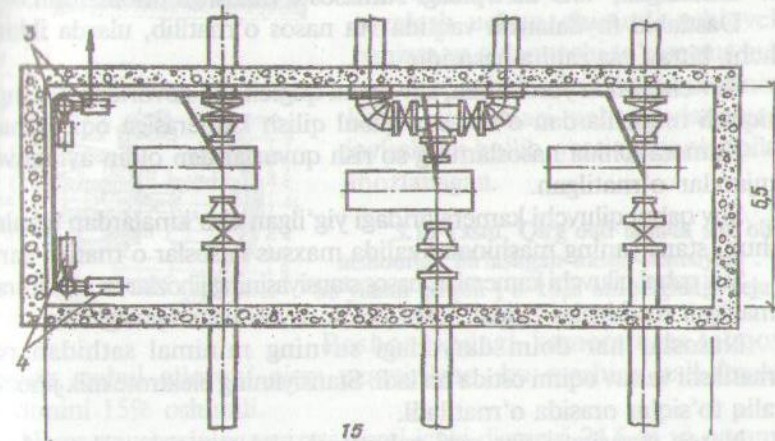
3.10-rasm. Alohida turdagi I-ko'taruv nasos stansiyasi
