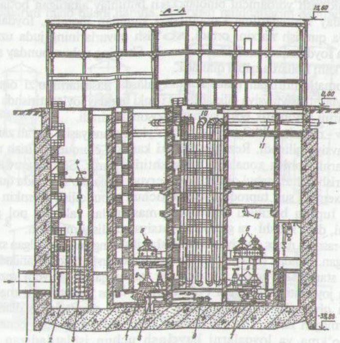
4.2-rasm. Shaxtali kanalizatsiya nasos stansiyasi
