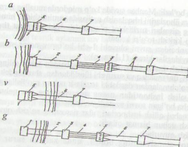
1.1.-rasm. Ochiq suv manbaidan foydalanadigan I-chi ko'taruv nasos stansiyalari inshootlari kompanovkasining prinsipial sxemalar
