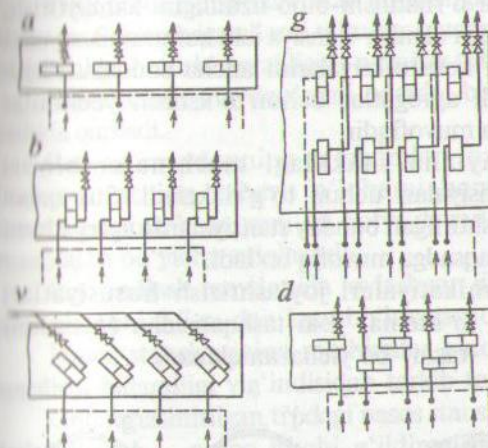
3.7-rasm. Gorizontall markazdan qochma nasosli agregatlarning joylashishi.
