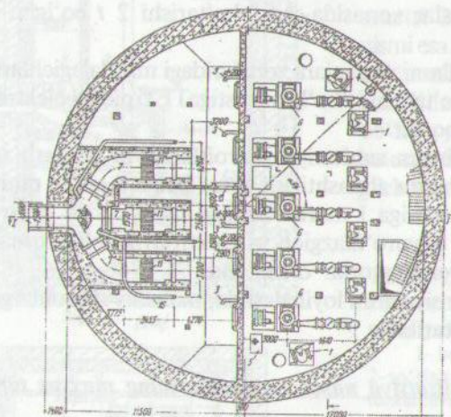
4.7-rasm. FV2700/26,5 tipidagi nasoslar bilan jihozlangan yirik kanalizatsiya nasos stansiyasining namunaviy loyihasi (902-1-10/70)
