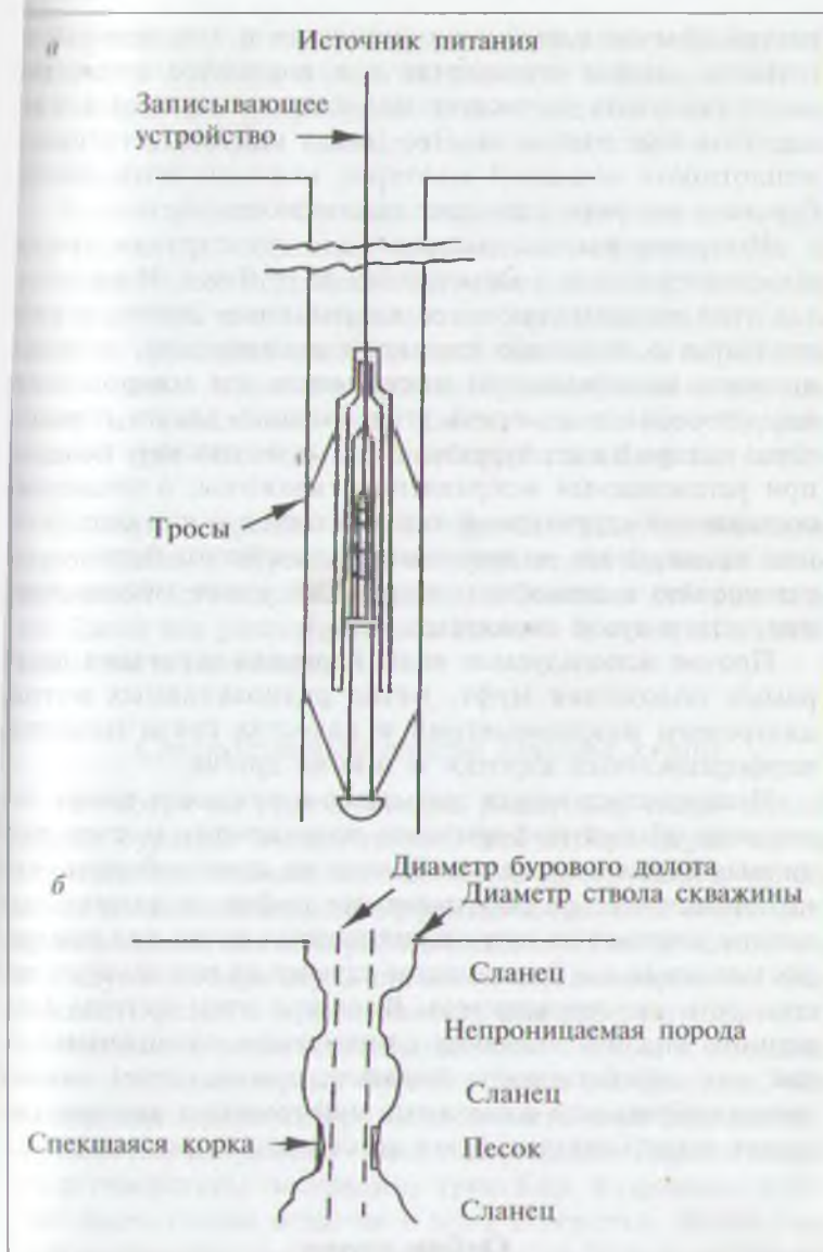
Рис. 6.7. Инструмент для регистрации диаграммы диаметра ствола скважины (а) и типовой ствол скважины (б), где показаны изменения диаметра
