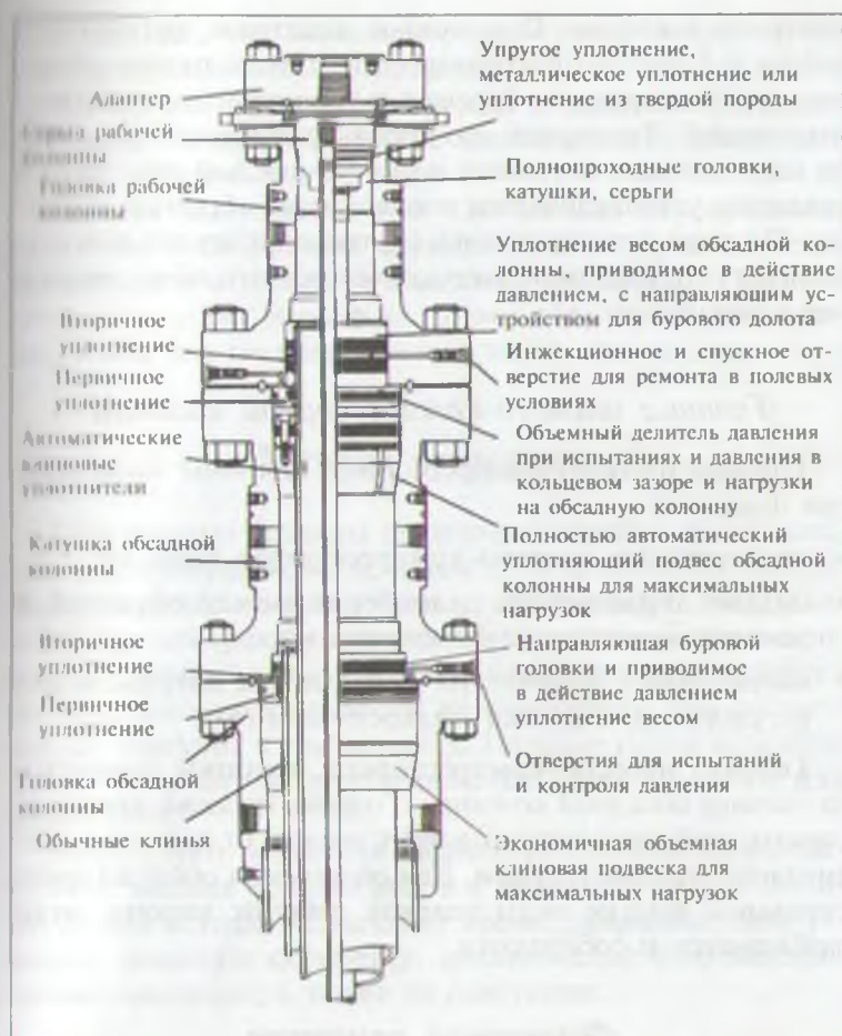
Рис. 11.2. Части оборудования устья скважины (предоставлено Gray Tool Co.)
