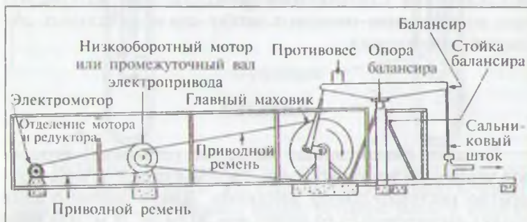
Рис. 10.15. Старинная качалка
