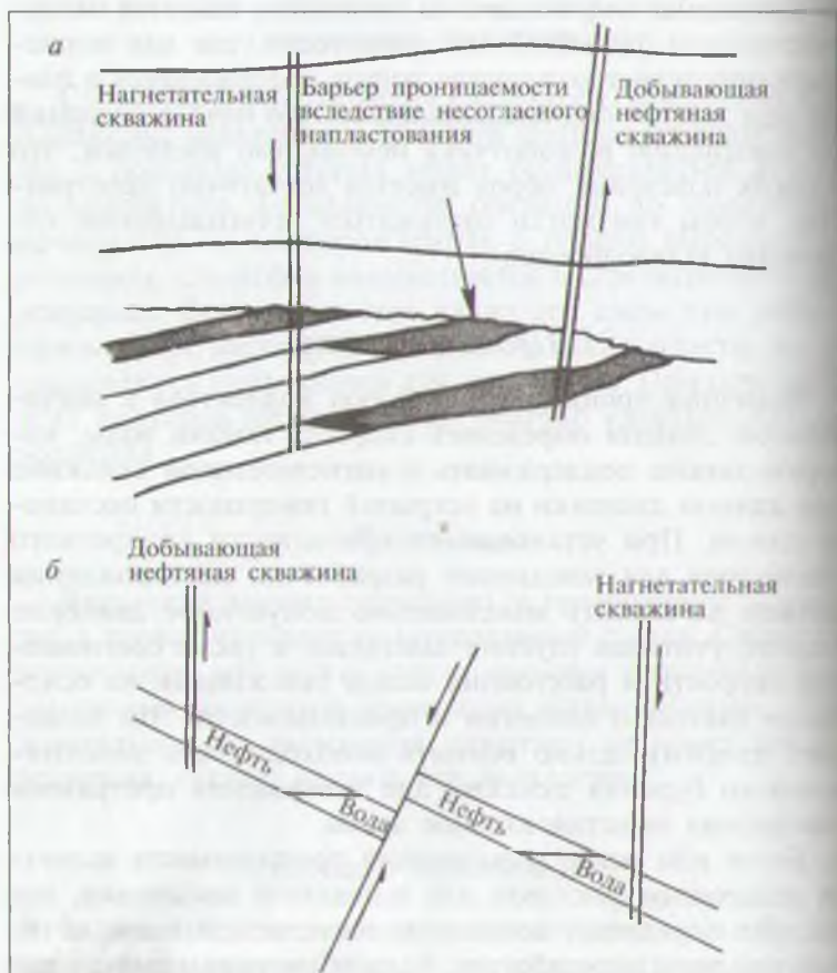
Рис. 14.1. Барьеры проницаемости, связанные с несогласным напластованием (а) и сбросом (б).
