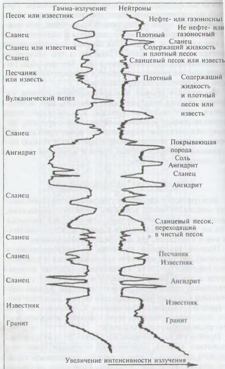
Рис. 6.6. Каротажная диаграмма по радиоактивности
