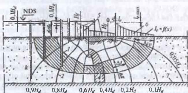
3.10-rasm. Gidrodinamik to'r:
