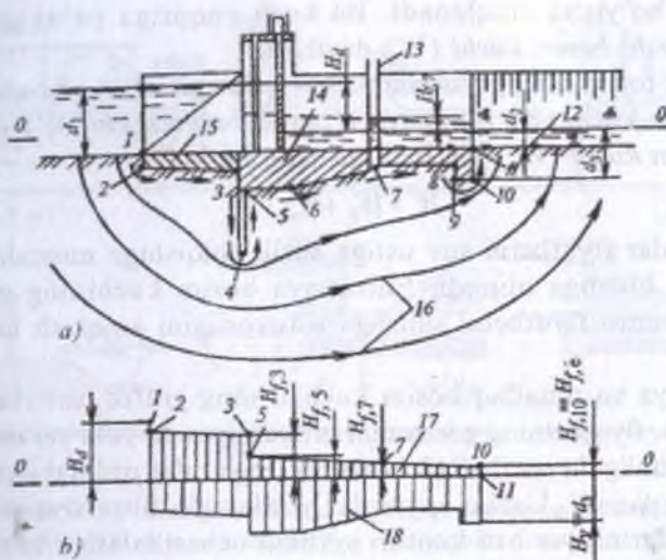
3.24 - rasm. Suv dimlovchi inshoot yer osti konturiga filtratsiya oqimi kuchi ta'siri sxemasi: a -- suv dimlovchi inshoot kesimi; b -- flyutbet gorizontali proyeksiyasidagi bosim epyuralari; 1 - 11-flyutbet yer osti chiziqlari bo'yicha filtratsiya oqimining aylanib o'tishi; 12 - risberman; 13 - pezometr; 14 - suv urilma; 15 - ponur; 16 - grunt suvlarining tok chiziqlari; 17, 18 - flyutbet gorizontali proyeksiyasidagi muallaq va filtratsiyaga qarshi bosim epyuralari.
