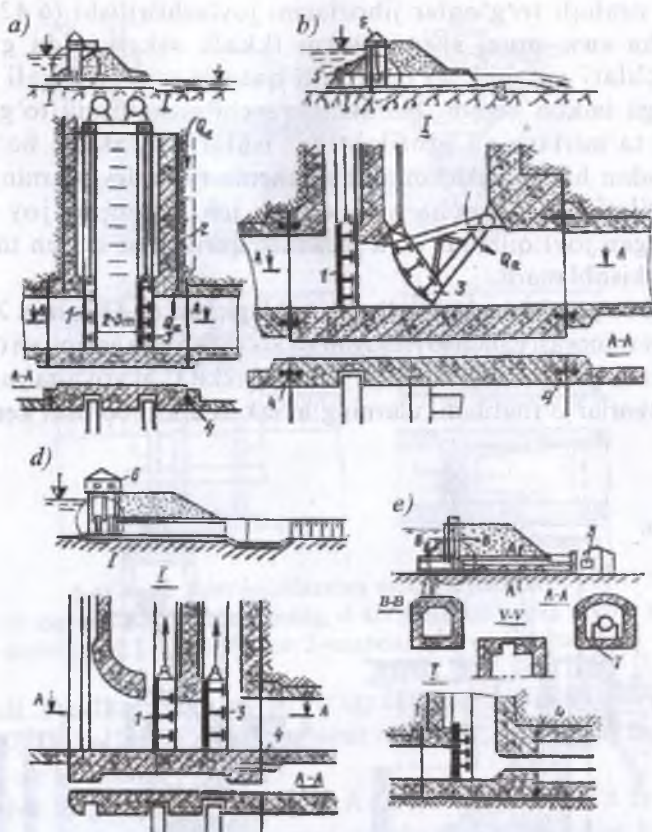
6.43-rasm. Gruntli to'g'onlardagi quvurli suv tashlagichlar mexanik jihozlari: a, b—to'g'ondagi minora bilan; d—kirishdagi minora bilan; c—quvurdagi asosiy zatvor bilan; 1—avariya-ta'mirlash zatvorlari; 2—havo yuboruvchi quvur; 3—asosiy zatvor; 4—choklar zichlagichlar bilan; 5—ta'mirlash zatvori; 6—xodimlar binosi; 7—galereya quvurlar bilan.
