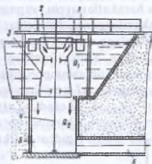
6.49-rasm. Suv bilan o'zaro ta'sir etuvchi zatvor-avtomat sxemasi: 1–po'kak; 2–trapetsial vodostivli voronka; 3–avtorostlagich korpusi; 4–yo'naltiruvchi o'q; 5–quduq; 6–quvur.
