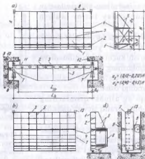
6.12-rasm. Yassi zatvor sxemalari: a—ko'ndalang tizim to'plami; b—bo'yлама tizim to'plami (yaxlit diafragma ko'rinishdagi ko'ndalang bog'lovchilar); d—ko'ndalang kesim va yon tomondan ko'rinishi.
