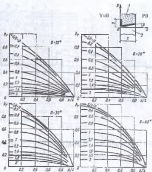
3.47-rasm. V turdagi tutashgan yon devor fragmenti sxemasi va tutashgan devor bo'ylab keltirilgan bosim h_r ning x o'qiga nisbatan uning turli qiyalik burchaklari \theta da va shpora S li uzunliklarida aniqlash grafiklari: 1 – gruntli to'g'on; 2 – suv tashlash inshooti.
