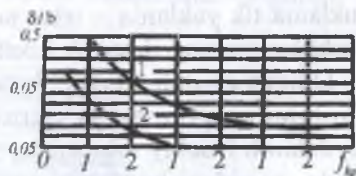
5.56-rasm. Bosimsiz tunnel nisbiy qalinligi \delta/b ni oldindan aniqlash grafiqi: 1 - betondan; 2 - temir-betondan.
