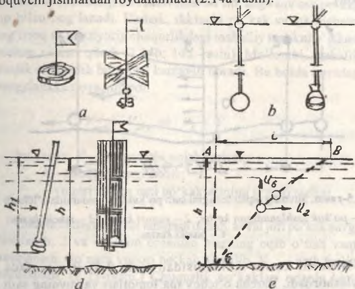
2.14-rasm. Suvning oqish tezligini o'lchash uchun qo'llaniladigan po'kaklarining turlari.
