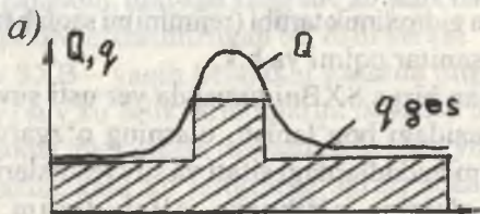
3.7. (a)-rasm. Oqimni oddiy rostlash gidrografi
