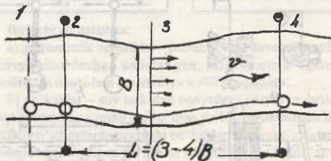
2.15-rasm. Suvning oqish tezligini sath po'kaklari yordamida o'lchash 1 – po'kak tashlanadigan kesim; 2 – yuqori kesim; 3 – ishchi kesim; 4 – pastki kesim
