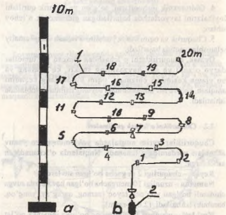
2.6-rasm. Reyka (a) va ko'l loti (b)
