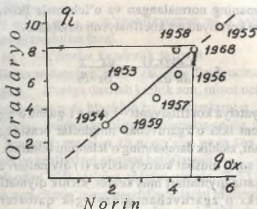
3.6-rasm. q_i = f(q_{o,x}) grafigi
