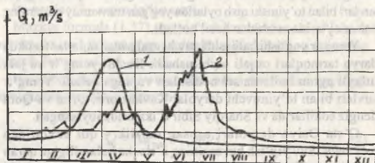
1.10-rasm. Tekislik (1) va tog'li (2) daryolar uchun tipik gidroagraflar
