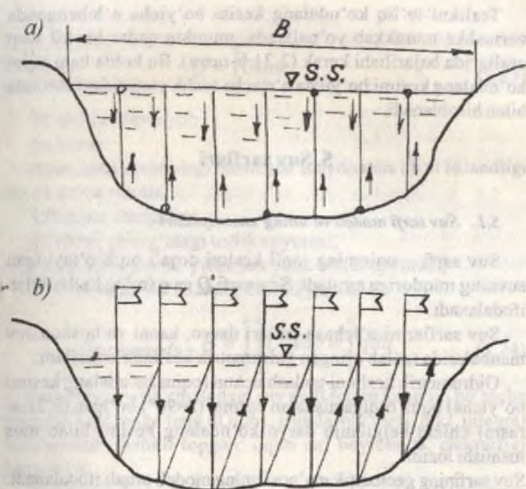
2.20-rasm. Integratsiya usuli bo'yicha oqim tezliklarini o'lchash a – vertushkani vertikalalar bo'yicha harakatlantirib tezlikni o'lchash; b – vertushkani oqim ko'ndalang kesim bo'yicha harakatlantirish; → – vertushkaning tezlik o'lchash mobaynida harakat yo'nalishi
