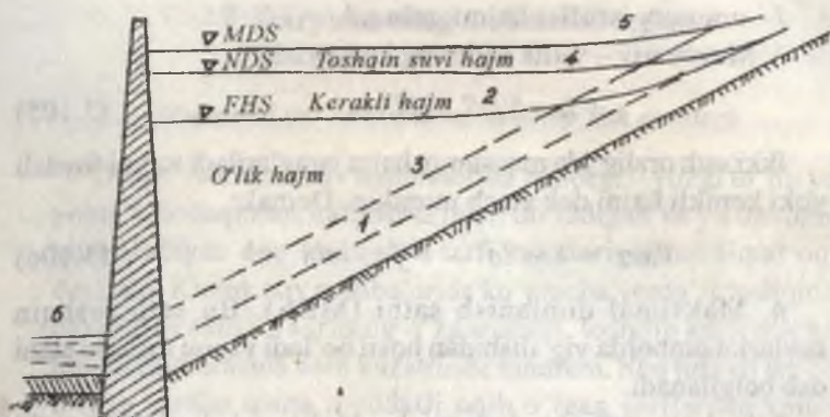
3.9-rasm. Suv omborining asosiy sathlari va hajmlari
