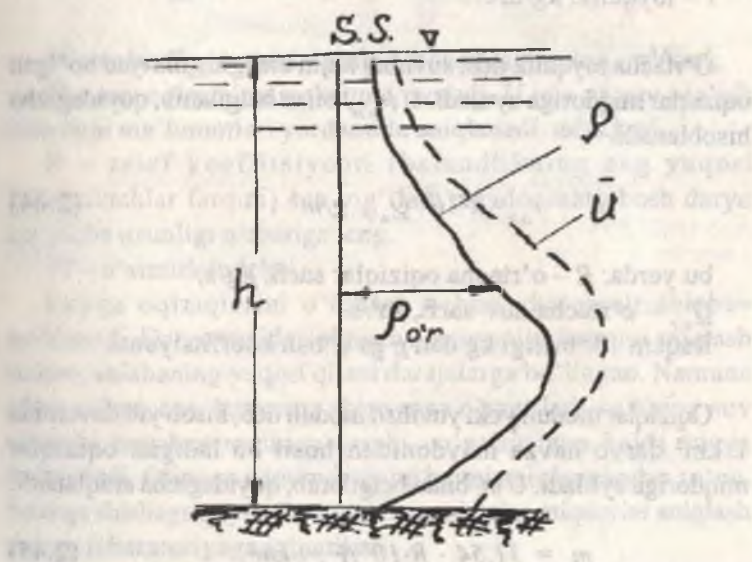
2.27-rasm. Oqiziqilarni chuqurlik bo'yicha taqsimlanishi:
