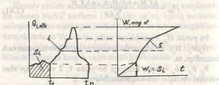
2.24-rasm. Suv sarfi gidrografi (4) va oqim hajmi grafigi (5)
