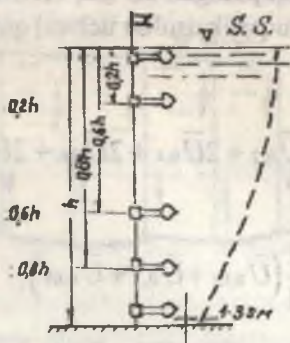
2.19-rasm. Batafsil usul bilan suvning o'rtacha tezligini aniqlash
