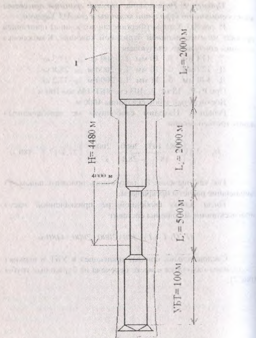
Рис.2. Расчетная схема прихвата в скважине 3 Хартум. 1-промежуточная колонна 219 x 245 мм, спущенная на глубину 4000 м.
