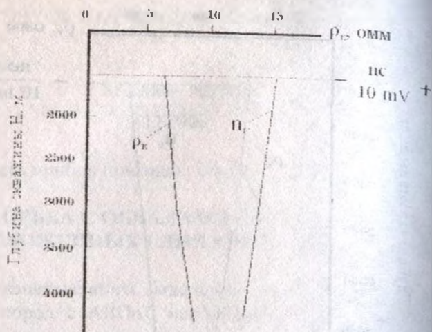
Рис. 6. Диаграмма стандартного каротажа при отсутствии зон обвалов глин.
