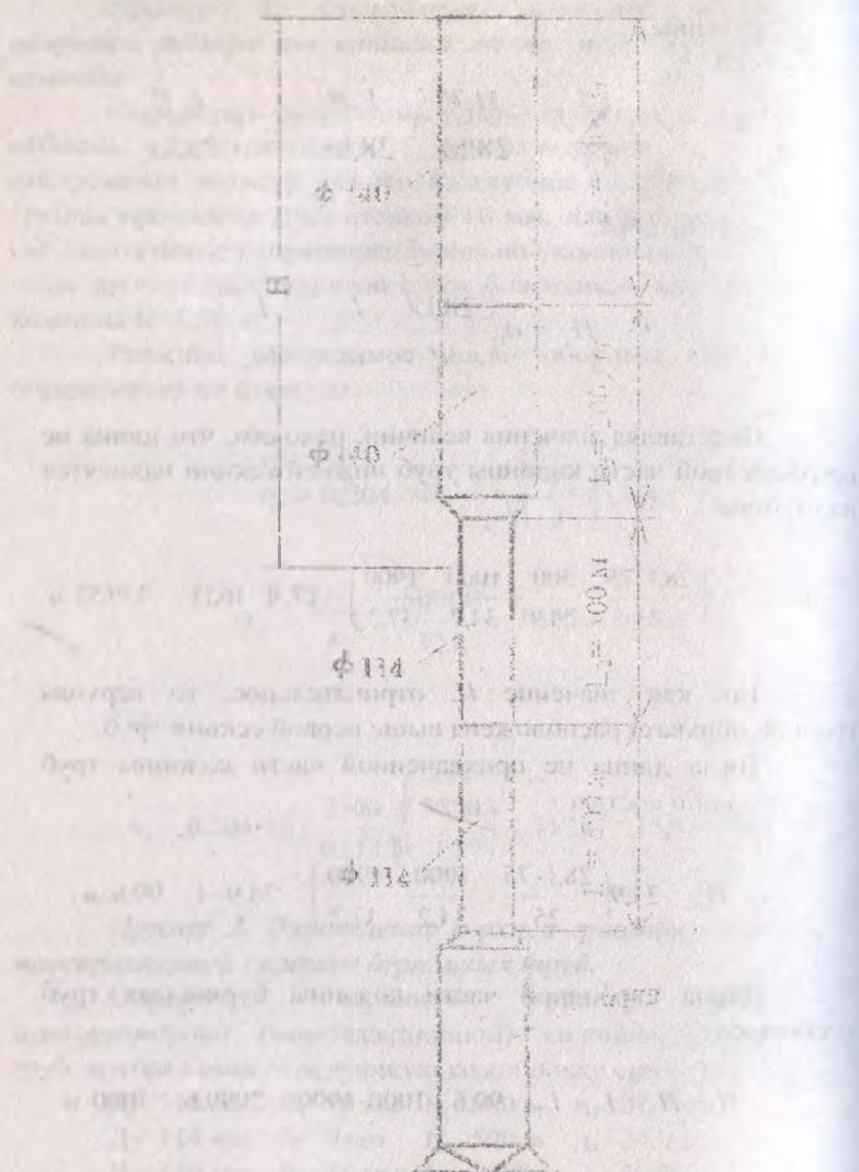
Рис. 1. Расчетная схема места прихвата.
