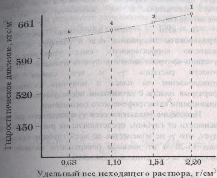
Рис.8. График падения гидростатического давления столба раствора в зависимости от удельного веса исходящего раствора. Точки 3, 5, 7 и 8 на графике не показаны.
