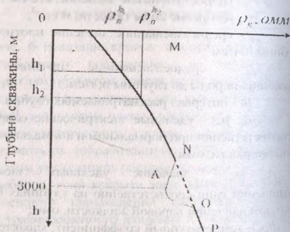
Рис.7. Расчетная схема для определения P_n по методике нормально уплотненных глин.
