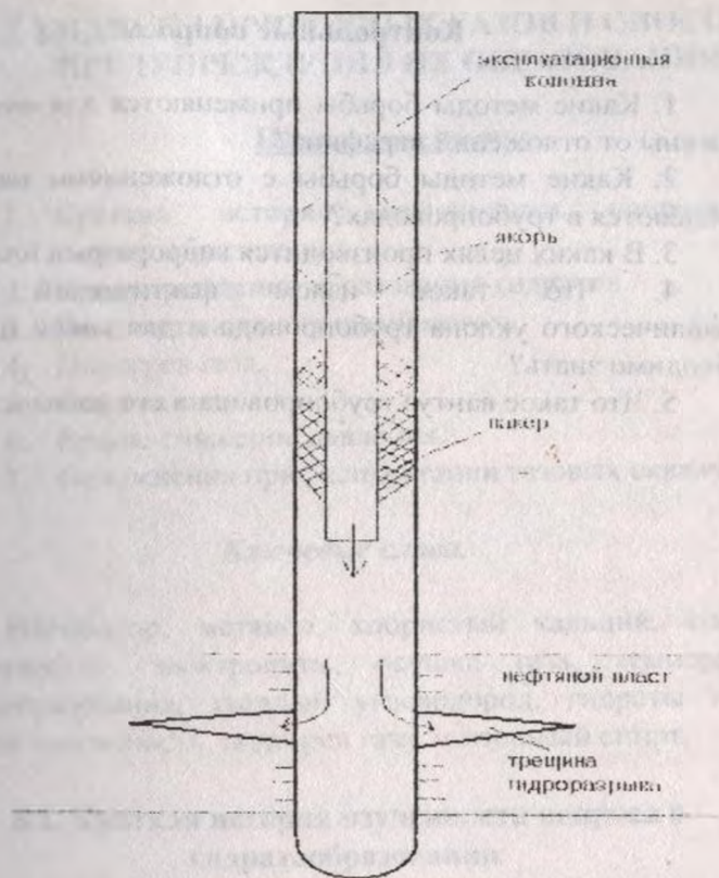
Рис. 9. Схема гидроразрыва пласта.
