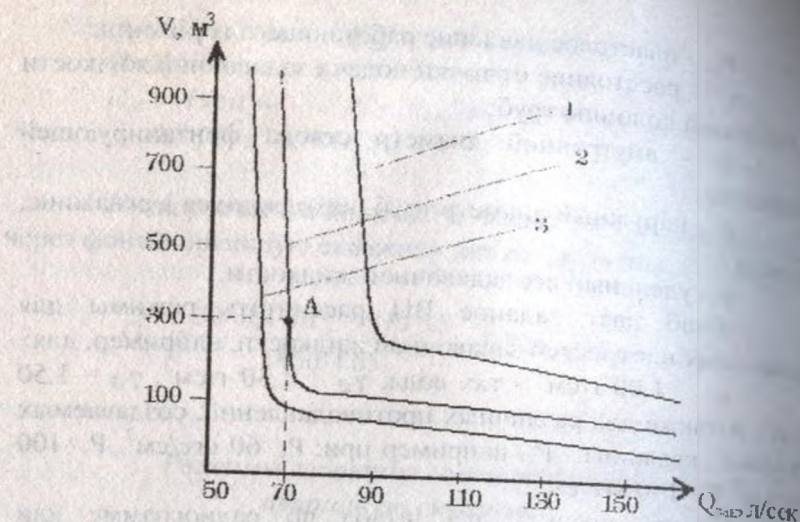
Рис.13. Режимы глушения газового фонтана. График зависимости V=f(Q_{зак}) .
