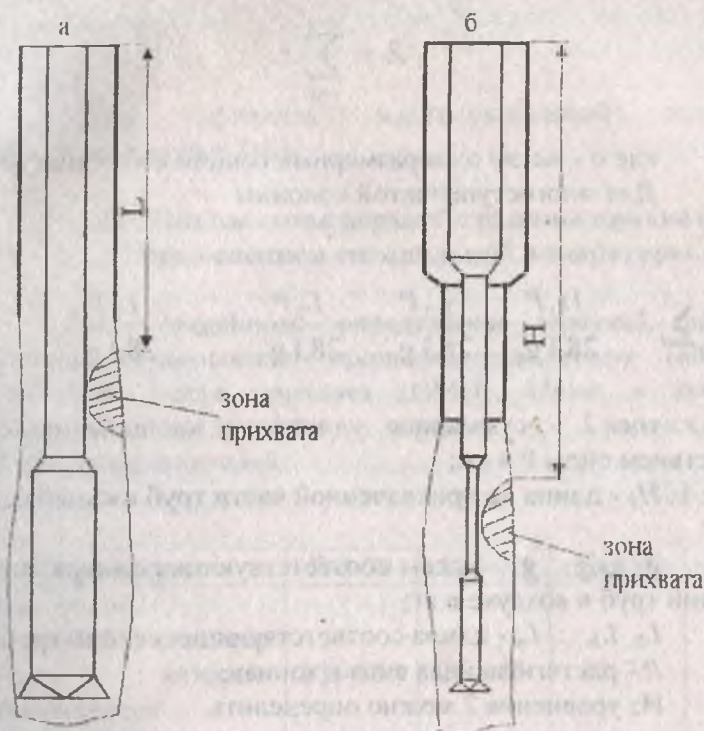
Рис.1. Схема прихвата: а) одноразмерная буровая колонна; б) многомерная буровая колонна.
