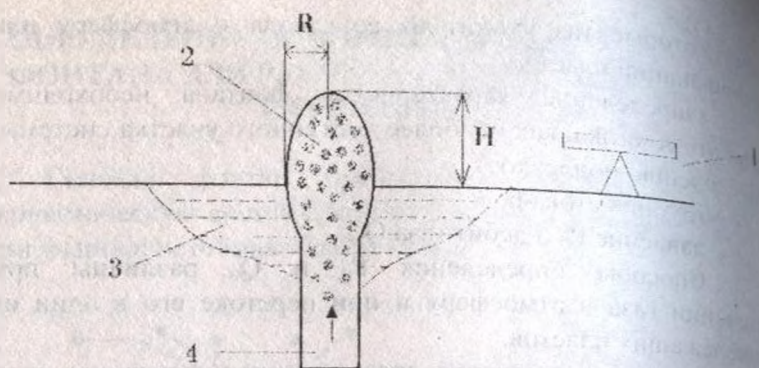
Рис.11. Схема измерений буруна. 1-нивелир; 2-газожидкостый бурун; 3-кратер фонтигаирующей скважины; 4-скважина.
