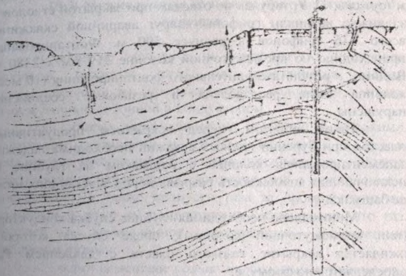
Рис. 12. Принципиальная схема возникновения грифонов при прорыве газа из скважины с коротким кондуктором.
