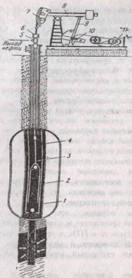
Рис. 11. Схема глубиннонасосной установки.
