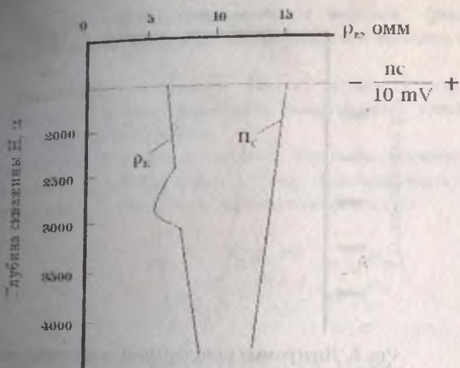
Рис. 5. Диаграмма стандартного каротажа для выделения зоны АВІПоД.
