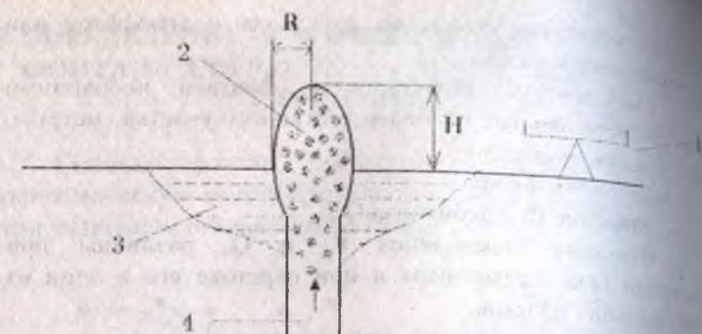
Рис.11. Схема измерений буруна. 1-нивелир; 2-газожидкостный бурун; 3-кратер фонтанирующей скважины; 4-скважина.
