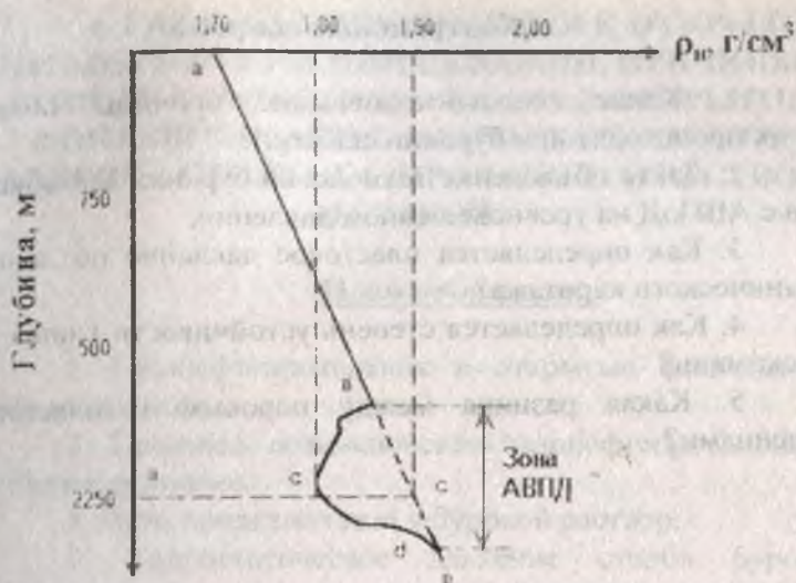
Рис.4. Кривая функции \rho_{\text{ф}}=f(H) . Кривая а, b, c, d, e - фактическая плотность глин, при этом участок ab - подчиняется закону нормального уплотнения глин, согласно уравнению (1); участок кривой вcd - фактическая плотность глины в зоне обвала; пунктирная линия вд - мысленно проведенная линия несуществующей в скважине нормального уплотнения глин в зоне АВП/Д.
