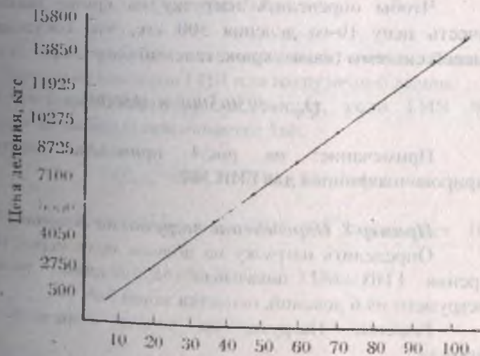
Рис.4. Нагрузочная (тарировочная) линия ГИВ №1 на канате диаметром 28 мм.
