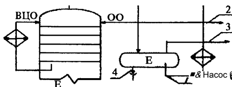
Рис. 3.14. Принципиальная схема КВС вакуумной колонны с использованием вакуумного гидроциркуляционного агрегата (ВГУ):
