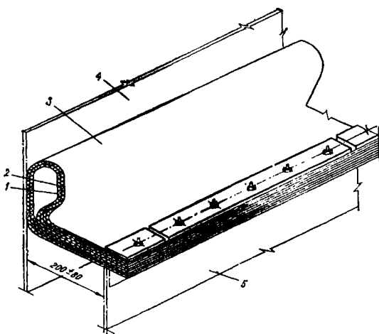
Рис. 2.130. Петлевой затвор: 1 — внутренняя петля; 2 — прокладка; 3 — наружная петля 4 — стенка резервуара; 5 — понтон
