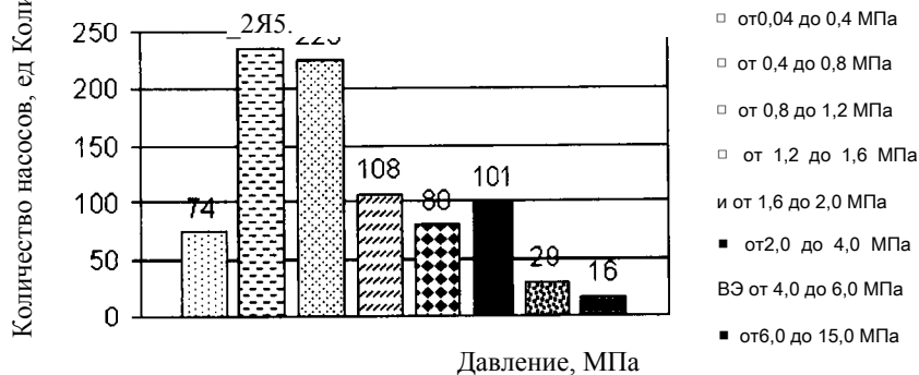
Рис. 2.195. Распределение центробежных насосов по давлению
