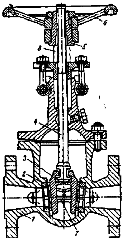
Рис. 2.155. Задвижка с упругим клином и выдвижным шпинделем: 1 — корпус; 2 — седло; 3 — затвор; 4 — шпindelь; 5 — ходовая гайка; 6 — маховик; 7 — клин; 8 — стойка
