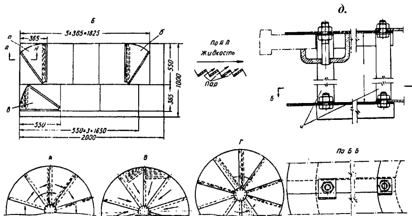
Рис. 2.15. Ситчатая тарелка с радиально-круговой организацией потока жидкости:
