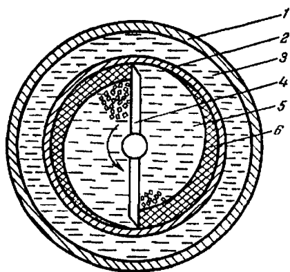
Рис. 4.16. Схема сечения скребкового кристаллизатора: 1 — наружная труба; 2 — внутренняя труба; 3 — хладагент; 4 — скребок; 5 — суспензия сырья; 6 — слой твердой фазы
