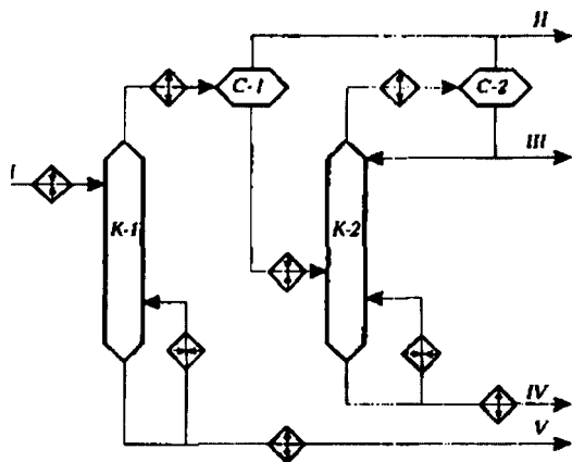
Рис. 3.1. Принципиальная схема установки стабилизации нефти:
