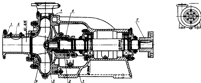
Рис. 2.203. Насос фекальный типа ФГ:
