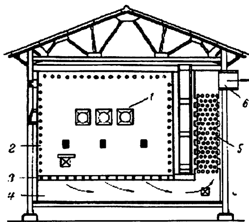
Рис. 2.124. Кубовая печь:
