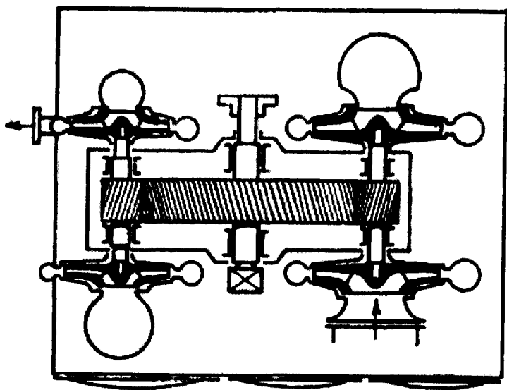
Рис. 2.223. Схема двухроторного четырехступенчатого нагнетателя фирмы «Демаг» (Германия)
