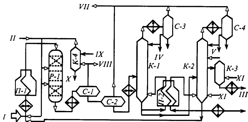
Рис. 8.15. Принципиальная технологическая схема установки одноступенчатого гидрокрекинга вакуумного газойля: I — сырье; II — ВСГ; III — дизельное топливо; IV — легкий бензин; V — тяжелый бензин; VI — тяжелый газойль; VII — углеводородные газы на ГФУ; VIII — газы отдува; IX — регенерированный раствор МЭА; X — раствор МЭА на регенерацию; XI — водяной пар
