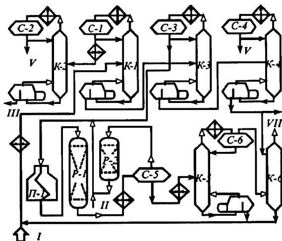
Рис. 8.9. Принципиальная технологическая схема установки изомеризации пентанов и гексанов: I — сырье; II — ВСГ; III — изопентановая фракция; IV — бутановая фракция; V — изогексановая фракция; VI — гексановая фракция на изомеризацию; VII — жирный газ
