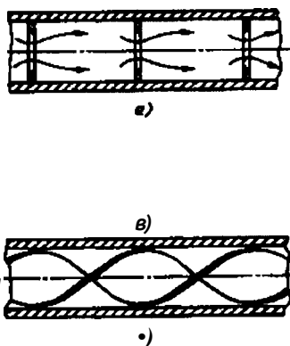
Рис. 2.44. Трубы с турбулизирующими вставками
