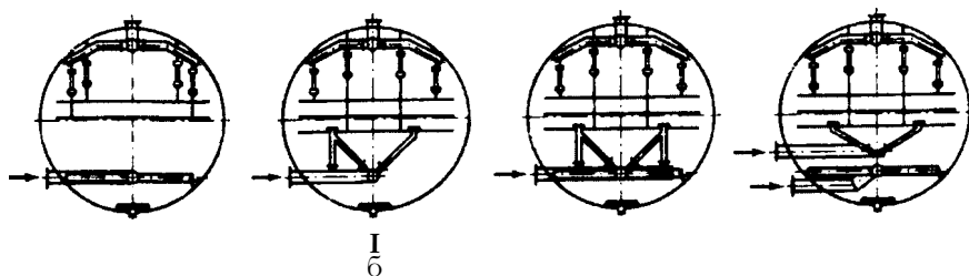
Рис. 3.25. Модификации горизонтальных электродегидраторов: а - 2ЭГ160; б - 2ЭГ160/3; в — 2ЭГ160-2; г - 2ЭГ160-2М
