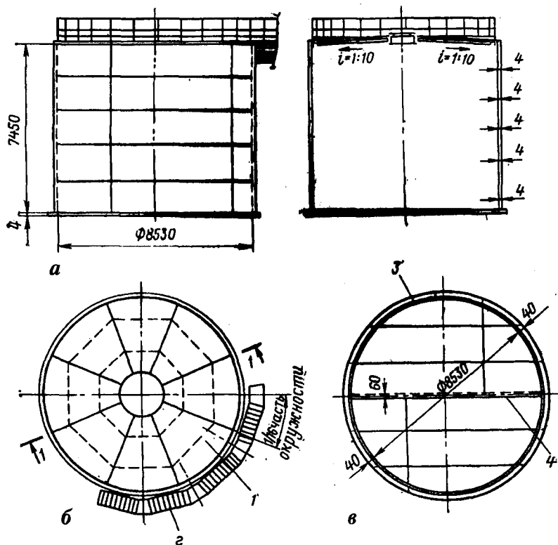
Рис. 2.126. Резервуар объемом 400 м³:
