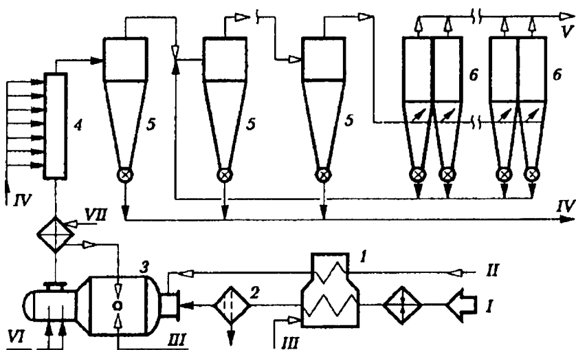
Рис. 5.11. Принципиальная технологическая схема печной активной сажи:
