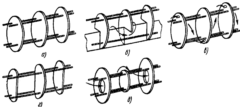
Рис. 2.40. Поперечные перегородки:
