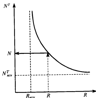
Рис. 3.6. Зависимость числа теоретических тарелок NT в колонне от флегмового числа R при заданной четкости разделения смеси
