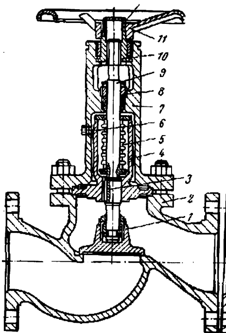
Рис. 2.168. Сифонный запорный вентиль: 1 — золотник; 2 — корпус; 3 — шпонка; 4 — промежуточный корпус; 5 — сифон; 6 — контрольное отверстие; 7 — крышка; 8 — аварийный сальник; 9 — шпиндель; 10 — ходовая гайка; 11 — маховик; 12 — разжимное кольцо
