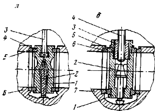
Рис. 2.159. Затвор двухдисковых параллельных задвижек: а) ШУЮ ИЗ двух Грибков, СИМ-
