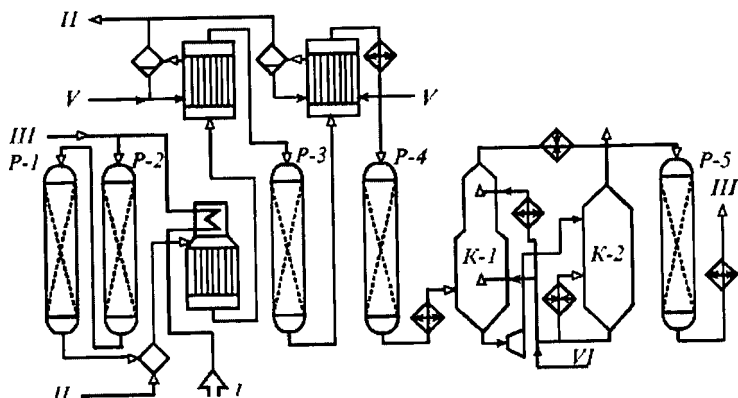
Рис 7 1 Принципиальная технологическая схема установки для производства водорода. I - сырье; II - водяной пар; III - водород; IV - диоксид углерода; V - вода; VI - водный раствор карбоната калия
