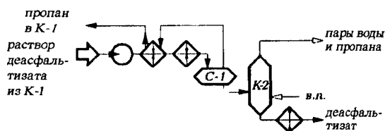
Рис. 4.7. Принципиальная схема узла регенерации пропана в сверхкритическом режиме из деасфальтизатного раствора
