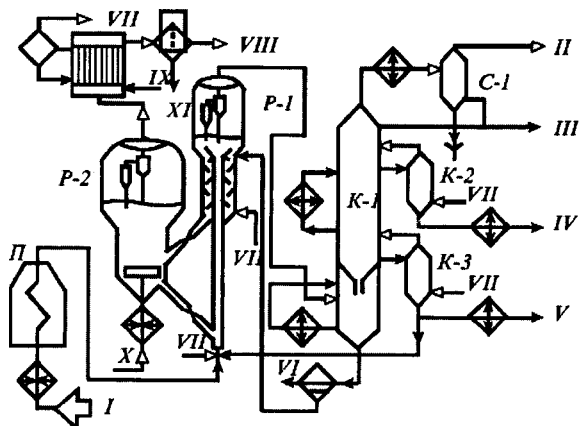
Рис. 6.6. Принципиальная технологическая схема установки каталитического крекинга Г-43-107:
