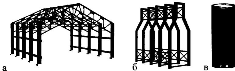
Рис. 2.74. Форма каркаса печи:
