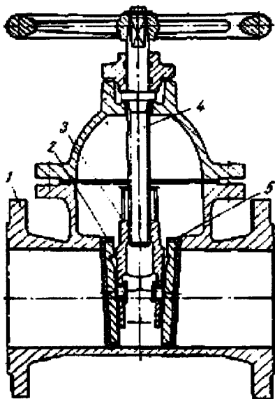
Рис. 2.160. Задвижка
