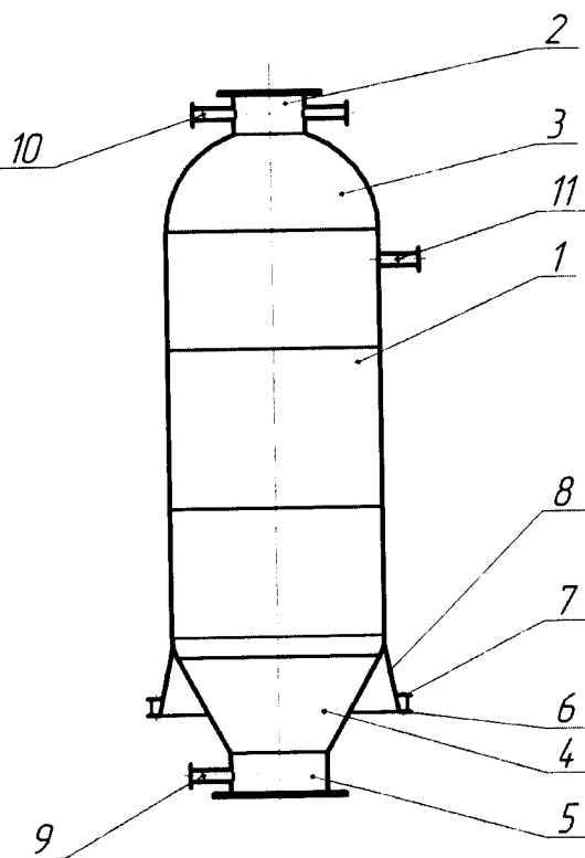
Рис. 5.13. Реактор установки замедленного коксования: 1 — корпус; 2,5 — верхняя и нижняя горловины; 3,4 — полушаровое и конические днища; 6 — фундаментное кольцо; 7 — опорное кольцо, 8 — опора, 9 — штуцер для ввода сырья; 10 — штуцер для выхода паров; 11 — штуцер для ввода антипенной присадки
