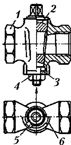
Рис. 2.163. Натяжной муфтовый кран с резьбовой затяжкой:
