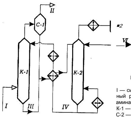
Рис. 3.5. Принципиальная схема установки этаноламиновой очистки горючих газов:
