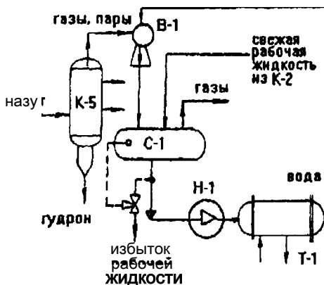
Рис. 3.30. Схема создания вакуума вакуумсоздающей системы СТВв П а С СИВНОГО Т ела фирмы «Техновакуум»
