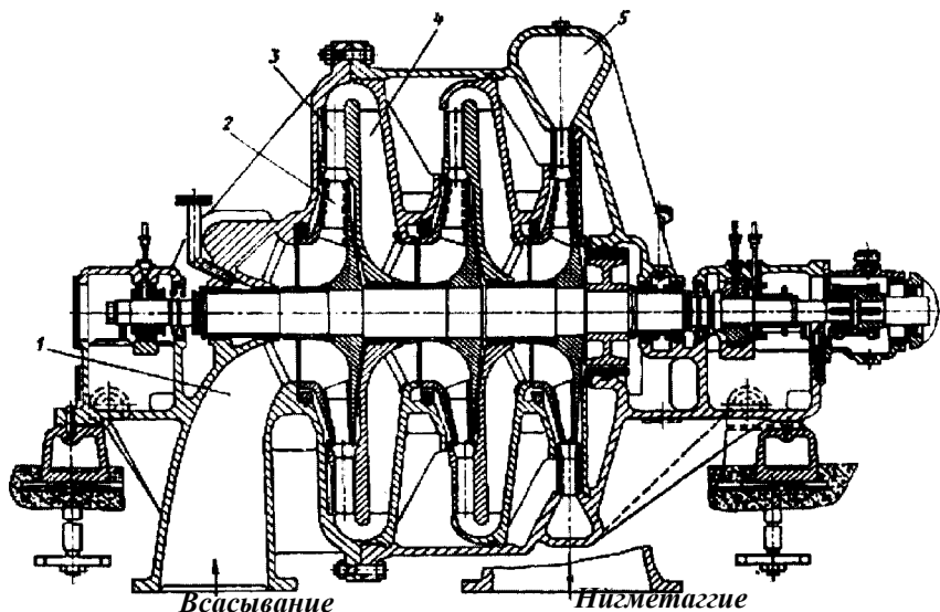
Рис. 2.219. Трехступенчатый нагнетатель типа 1200-25-1 НЗЛ:
