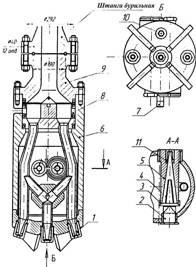
Рис. 5.16. Гидрорезак универсальный ГРУ-ЗР-250:
