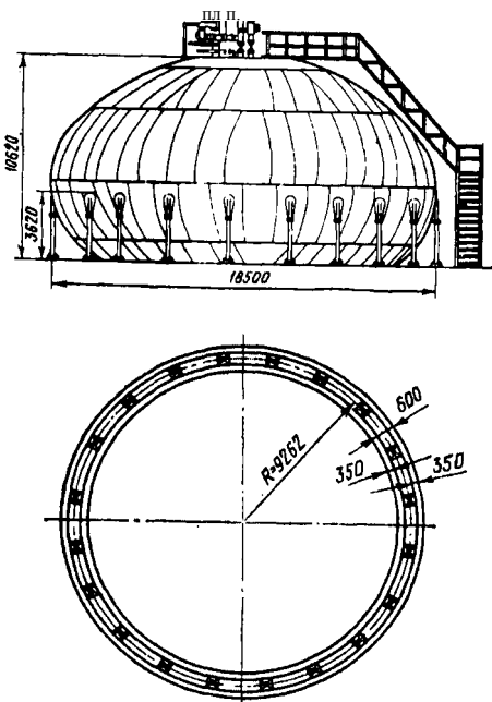
Рис. 2.135. Каплевидный резервуар с экваториальной опорой
