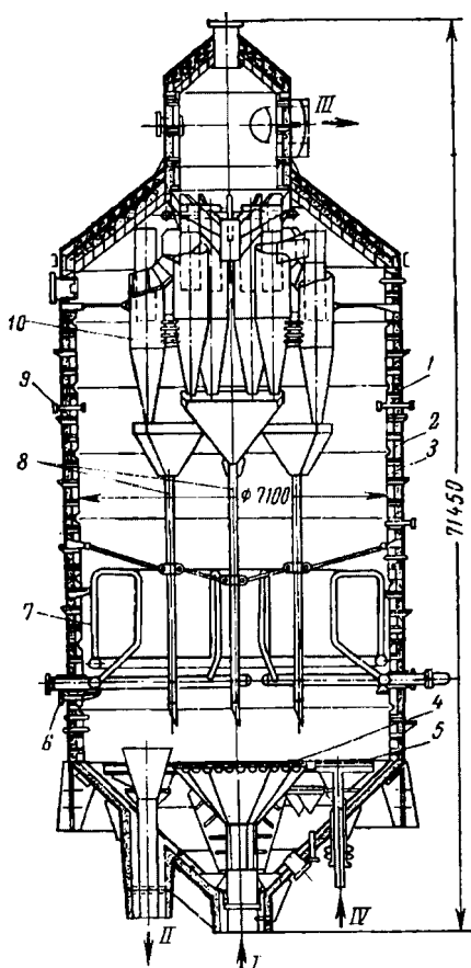
Рис. 6.23. Регенератор установки крекинга с пылевидным катализатором:
