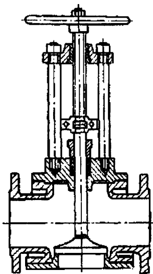
Рис. 2.170. Смесительный вентиль
