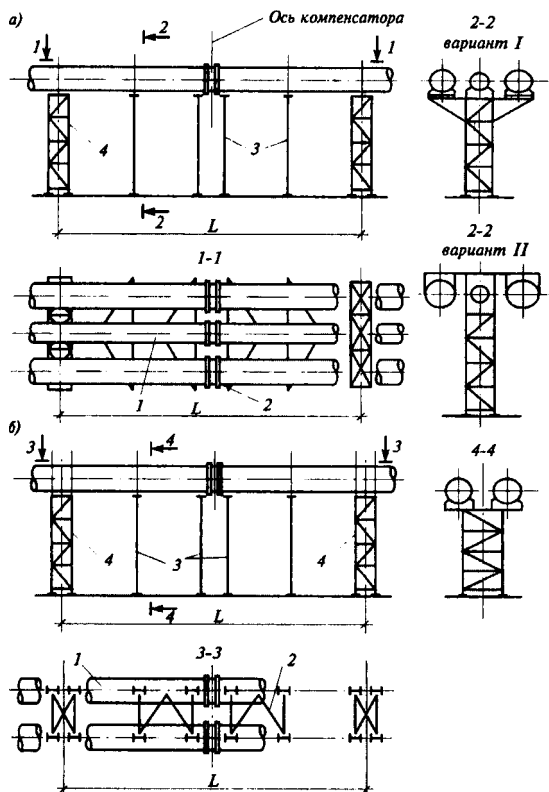
Рис. 2.145. Конструктивная схема при поперечном сечении типа III: 1 — трубопровод-распорка; 2 — подкос; 3,4 — соответственно промежуточные и неподвижная опоры; а — при осевом положении «ведущей» трубы; б — при боковом положении
