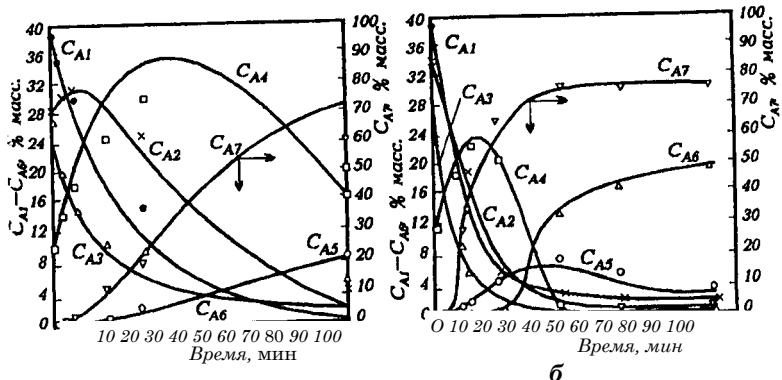
Рис 5.2. Изменение концентрации групповых компонентов дистиллятного крекинг-остатка Красноводского НПЗ от продолжительности термолиза при давлении 0,1 МПа и температуре 420 (а) и 490°C (б):
