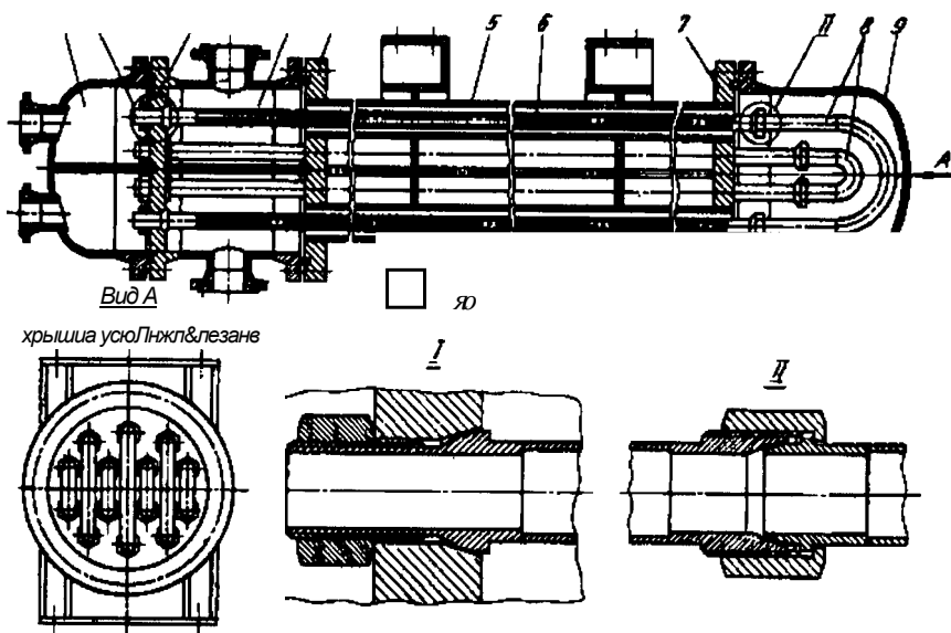
Рис. 2.50. Разборный двухпоточный теплообменник типа «труба в трубе»
