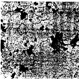
Рис. 2.228. Ковкий чугун на ферритной (в) и перлитной (г) основе x 200
