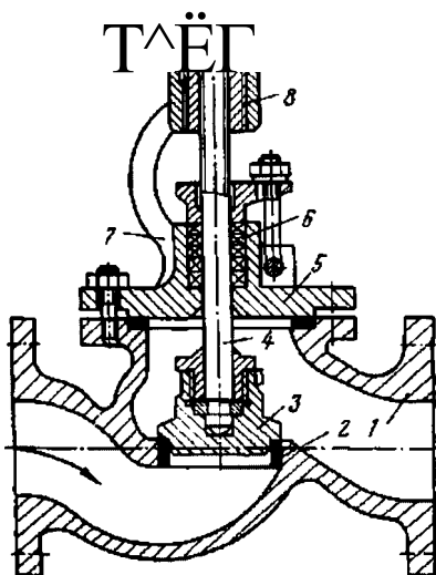
Рис. 2.161. Проходной вентиль
