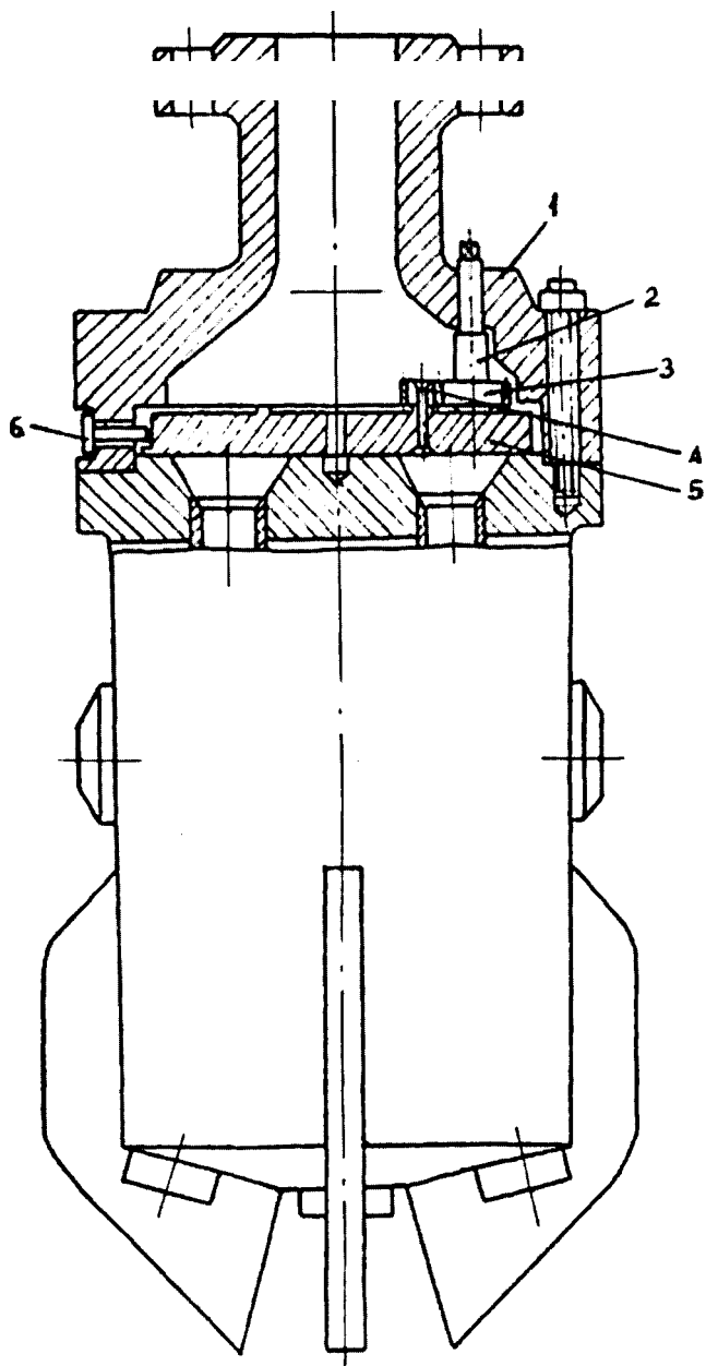
Рис. 5.17. Узел механического переключения режимов гидрорезака ГРУ-ЗР: 1 — фланец гидрорезака; 2 — ступенчатый вал; 3 — шестерня; 4 — зубчатый сектор; 5 — золотник; 6 — фиксатор
