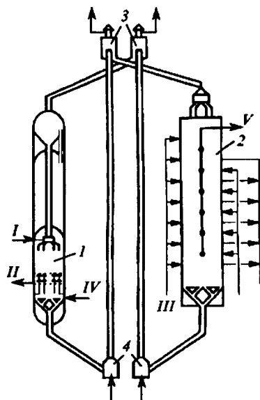
6.3. Схема реакторного блока установки каталитического крекинга с движущимся слоем шарикового катализатора (43-102): 1 — реактор; 2 — регенератор; 3 — сепараторы; 4 — дозеры; I — сырье; II — продукты крекинга; III — воздух; IV — водяной пар; V — дымовые газы; VI — вода
