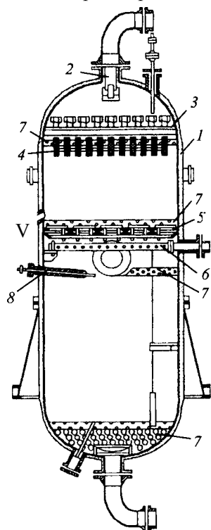
РИС. 8.12. Реактор гидроочистки дизельного топлива
