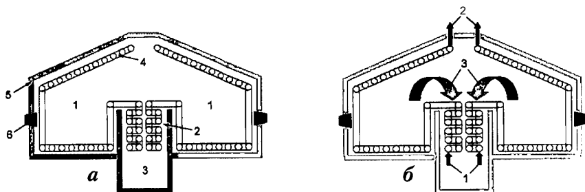
Рис. 2.109. Схема работы печи:
