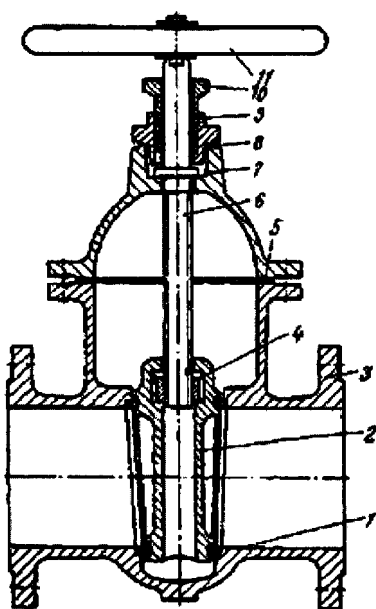
Рис. 2.151. Задвижка:
