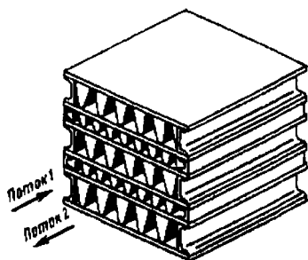
Рис. 2.67. Пакет противоточного теплообменника
