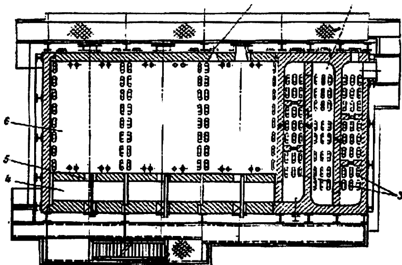
Рис. 2.122. Многокамерная печь типа Р:
