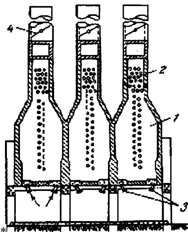
Рис. 2,123. Схема МНОГОКМВРной печи
