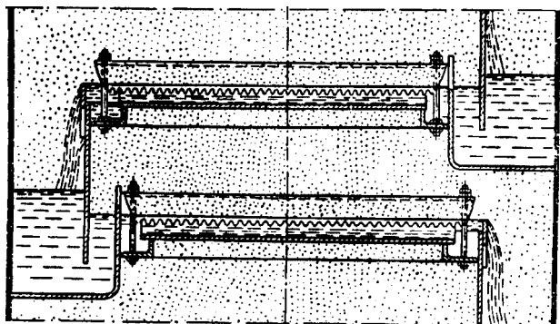
Рис. 2.10. Гидравлический затвор в переливных устройствах
