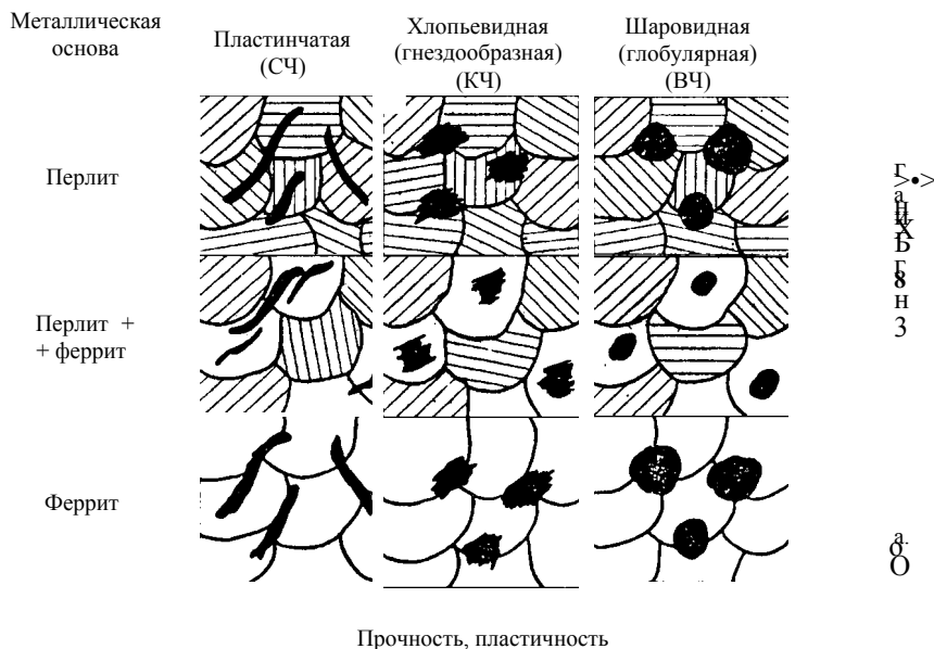
Рис. 2.225. Влияние металлической основы и формы включения графита на свойства чугунов
