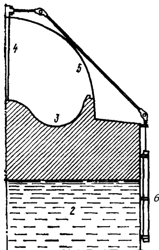
Рис. 2.133. Резервуар с мембранной «дышащей» крышей:
