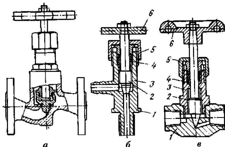
Рис. 2.171. Запорно-регулирующие вентили:
