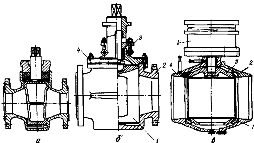
Рис. 2.172. Краны:
