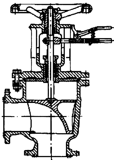
Рис. 2.1 77. Двухходовый угловой кран с подъемом пробки
