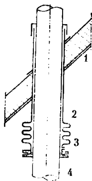
Рис. 6.22. Соединение трубопровода большого диаметра с корпусом аппарата: 1 — корпус; 2 — линзовый компенсатор; 3 — ввод пара на продувку катализатора; 4 — трубопровод
