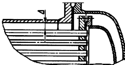
Рис. 2.33. Вариант размещения крышки плавающей головки в кожухе меньшего диаметра
