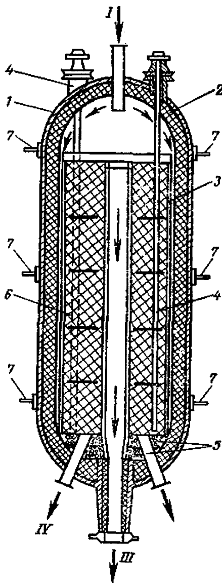
Рис. 8.19. Схема реактора каталитического риформинга с радиальным вводом газосырьевой смеси: 1 — корпус; 2 — футеровка; 3 — кожух; 4 — многослойная термopapa; 5 — фарфоровые шары; 6 — катализатор; 7 — поверхностная термopapa. Линии: I — газосырьевая смесь; II — продукты реакции; III — выгрузка катализатора; IV — вывод продуктов при эжектировании системы во время регенерации катализатора
