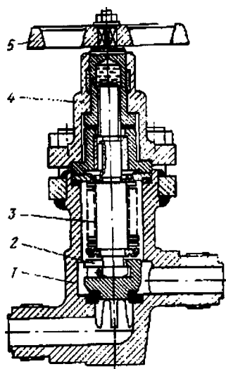
Рис. 2.169. Сифонный стальной вентиль:
