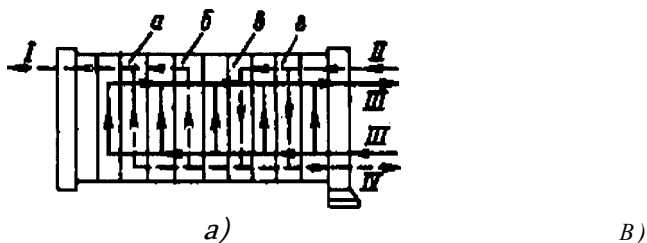
Рис. 2.58. Схемы специальных пластинчатых аппаратов: а — конденсатор; б — теплообменник для трех теплоносителей
