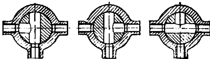
Рис. 2.175. Схема работы трехходового крана
