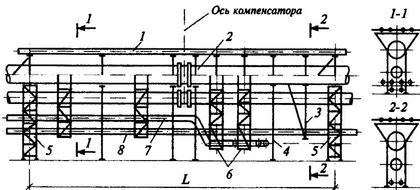
Рис. 2.144. Конструктивная схема при поперечном сечении типа II:
