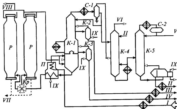
Рис. 5.5. Принципиальная технологическая схема двухблочной установки замедленного коксования:
