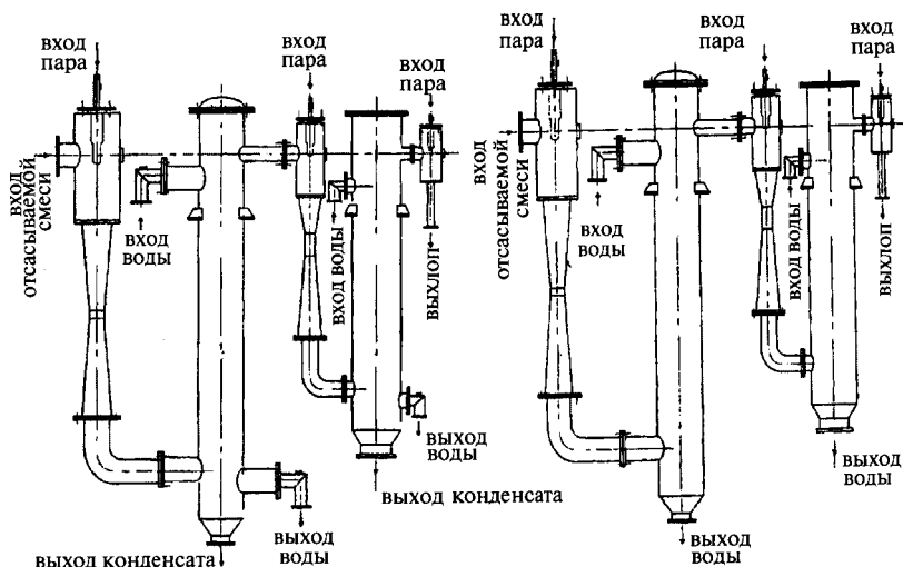
Рис. 3.29. Вакуум-насосы парозжекторные трехступенчатые с конденсаторами смешения (а) и с поверхностными конденсаторами (б)
