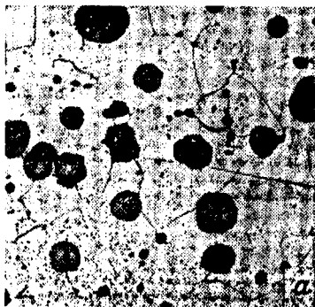
Рис. 2.227. Высокопрочный чугун на ферритной (а) и ферритно-перлитной (б) основе x 200
