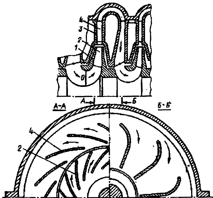
Рис. 2.215. Схема ступени центробежного компрессора: 1 — рабочее колесо; 2 — лопатки; 3 — кольцевой отвод; 4 — диффузорные лопатки
