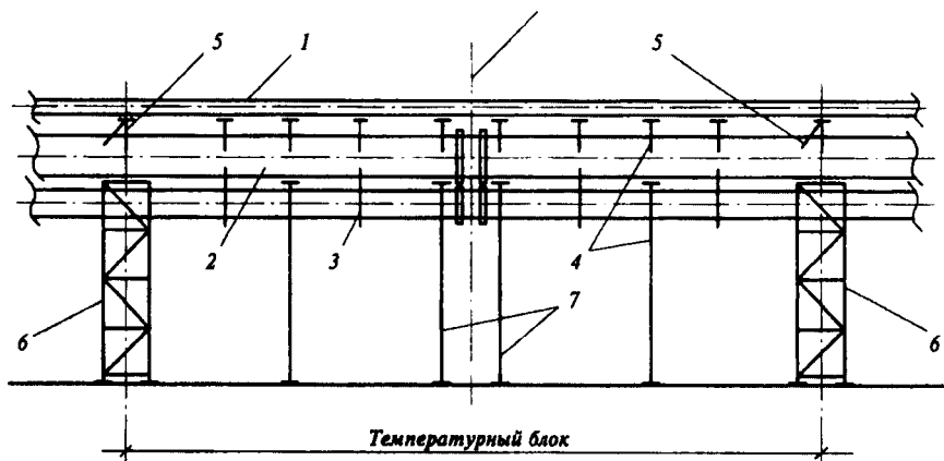
Рис. 2.139. Трубопроводная система балочной прокладки:
