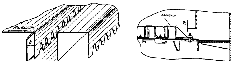
Рис. 2.18. Размещение Э-образных элементов тарелки
