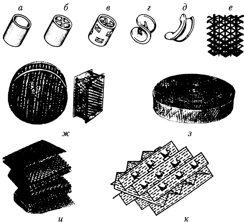
Рис. 3.12. Типы насадок:
