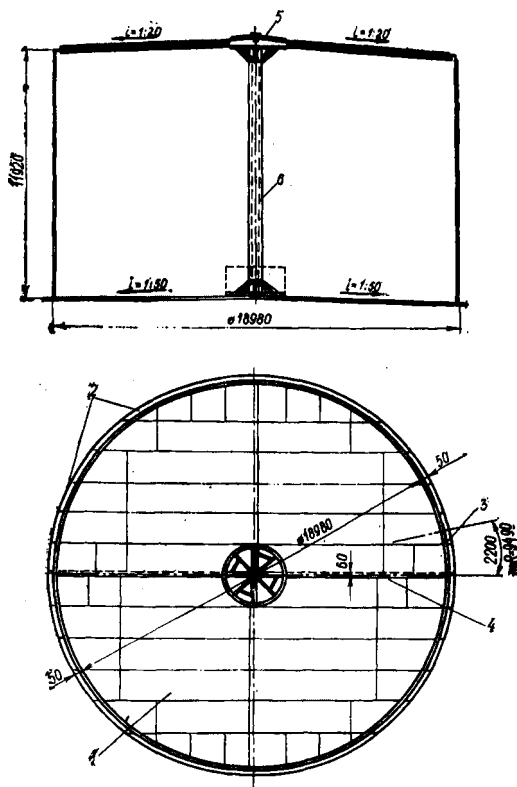
Рис. 2.127. Резервуар объемом 3000 м 3 с центральной стойкой:
