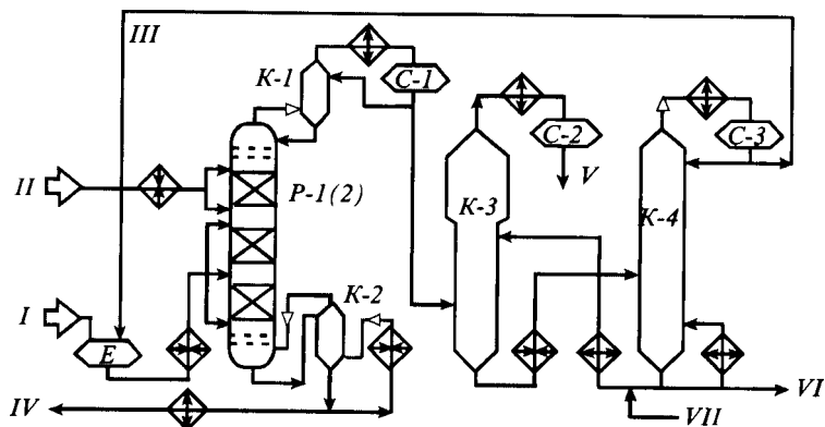
Рис. 6.13. Принципиальная технологическая схема установки получения метил-грег-бутилового эфира:
