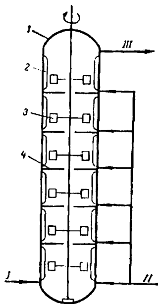
Рис. 4.17. Схема кристаллизатора смешения:
