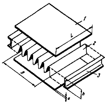
Рис. 2.66. Детали элемента пластинчато-ребристого теплообменника
