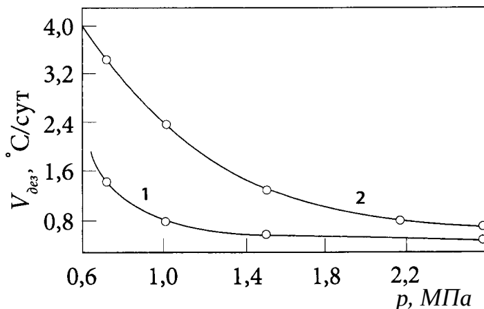
Рис. 8.4. Зависимость скорости дезактивации V катализатора КР-108 от давления при различных октановых числах риформата (ММ) (массовая скорость — 3 \text{ ч}^{-1} ; отношение водород : углерод = 5:1 ): 1 — 87; 2 — 90
