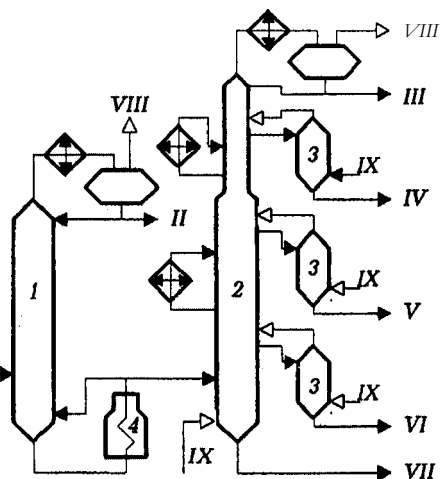
Рис. 3.15. Принципиальная схема блока атмосферной перегонки нефти установки ЭЛОУ-АВТ-6: 1 — отбензинивающая колонна; 2 — атмосферная колонна; 3 — отпарные колонны; 4 — атмосферная печь; I — нефть с ЭЛОУ; II — легкий бензин; III — тяжелый бензин; IV — фракция 180...220°C; V — фракция 220...280°C; VI — фракция 280...350°C; VII — мазут; VIII — газ; IX — водяной пар
