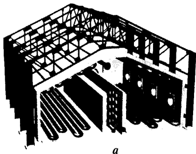
Рис. 2.86. Каркас печи
