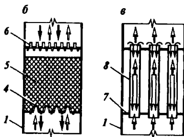
Рис. 2.5. Схемы основных типов колонных аппаратов: а – тарельчатый; б – насадочный; в – пленочный; 1 – корпус колонны; 2 – полотно тарелки; 3 – переточное устройство; 4 – опорная решетка; 5 – насадка; 6 – распределитель; 7 – трубчатая решетка; 8 – трубка
