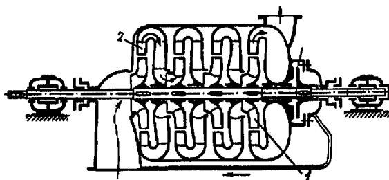
Рис. 2.187. Схема многоступенчатого секционного центробежного насоса: 1 — рабочее колесо; 2 — направляющий аппарат
