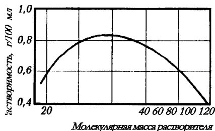
Рис. 4.12. Зависимость растворимости парафина с температурой плавления 54°C в сжиженных и жидких парафиновых углеводородах от их молекулярной массы
