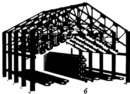
Рис. 2.86. Каркас печи
