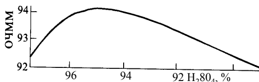
Рис. 6.10. Влияние концентрации серной кислоты на октановое число алкилбензина
