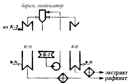
Рис. 4.11. Принципиальная схема работы отпарных колонн М-метилпирролидоновой очистки масел
