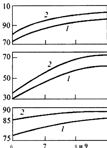
Рис. 8.1. Зависимость выхода риформата В, ароматических углеводородов А и октанового числа О 4 (по ИМ) риформата от среднего числа n атомов углерода в сырье: 1 — при 475°C; 2 — при 495°C
