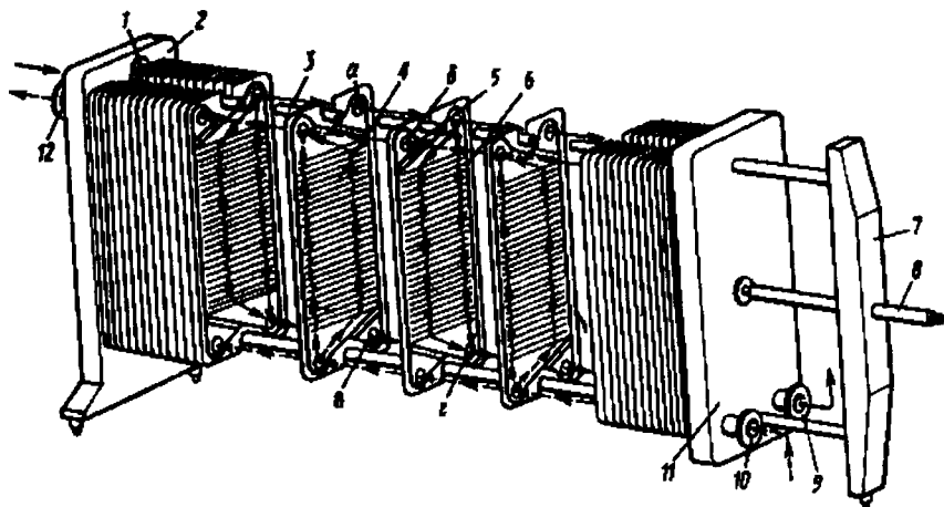
Рис. 2.54. Разборный пластинчатый теплообменник (исполнение 2):
