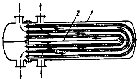
Рис. 2.27. Двухходовой теплообменник с 11-образными трубами
