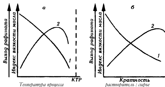
Рис. 4.9 — Зависимость качества (1) и выхода (2) рафината от: а) температуры процесса; б) кратности растворителя к сырью
