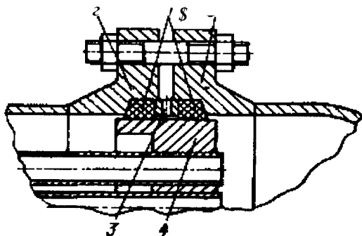
Рис. 2.37. Сальниковое кольцевое уплотнение
