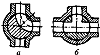
Рис. 2.176. Трехходовые краны с 1-образным (а) и с Т-образным (б) проходами в пробке
