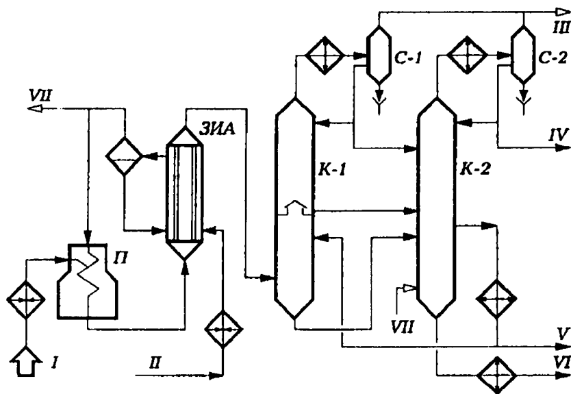
Рис. 5.10. Принципиальная схема установки пиролиза бензина: I — сырье; II — конденсат; III — газы пиролиза; IV — бензиновая фракция (н. к. — 150°С); V — легкая смола; VI — тяжелая смола; VII — водяной пар
