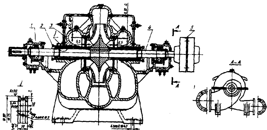
Рис. 2.200. Насос центробежный Д 2000-100 (с двусторонним вводом жидкости на колесо): 1 — подшипник; 2 — втулка сальника; 3 — корпус; 4 — вал; 5 — муфта
