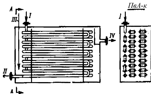
Рис. 2.51. Схема однопоточного погружного змеевикового конденсатора-холодильника:
