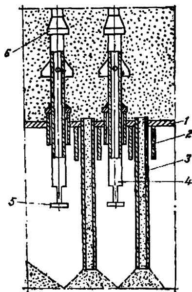
Рис. 6.16. Сепарационное устройство реактора: 1 — тарелка; 2 — ребро жесткости; 3 — труба для вывода катализатора; 4 — труба для вывода паров; 5 — отбойник; 6 — «колокольчик»
