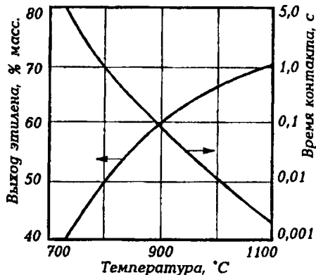
Рис. 5.8. Максимальный выход этилена при пиролизе этана в интервале 730... 1100°С
