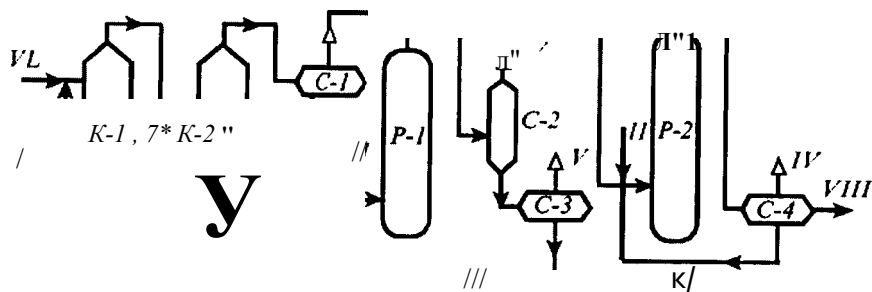
Рис. 7.4. Принципиальная технологическая схема процесса каталитической окислительной демеркаптанизации углеводородного сырья «Мерокс»: I – сырье; II – воздух; III – регенерированный раствор щелочи («Мерокс»); IV – отработанный воздух; V – дисульфиды; VI – циркулирующий раствор щелочи («Мерокс»); VII – свежая щелочь- VIII – очищенный продукт
