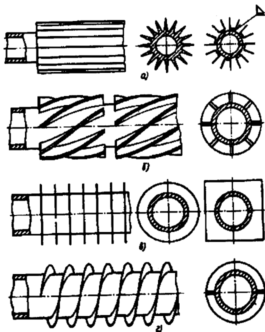
Рис. 2.43. Трубы с оребрением
