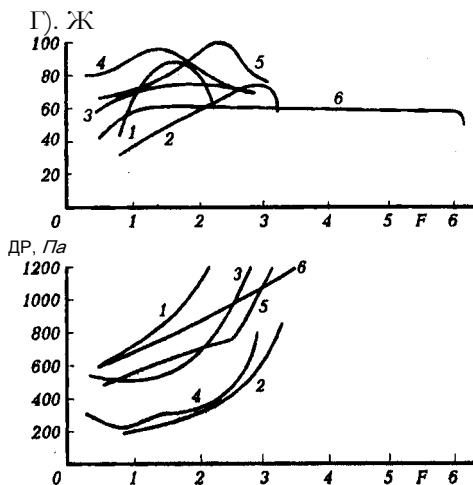
Рис. 3.11. Зависимость КПД (7) и гидравлического сопротивления ( Dp ) тарелок некоторых типов от F -фактора ( F = u \sqrt{\rho} ), где u — скорость пара, \rho — плотность пара
