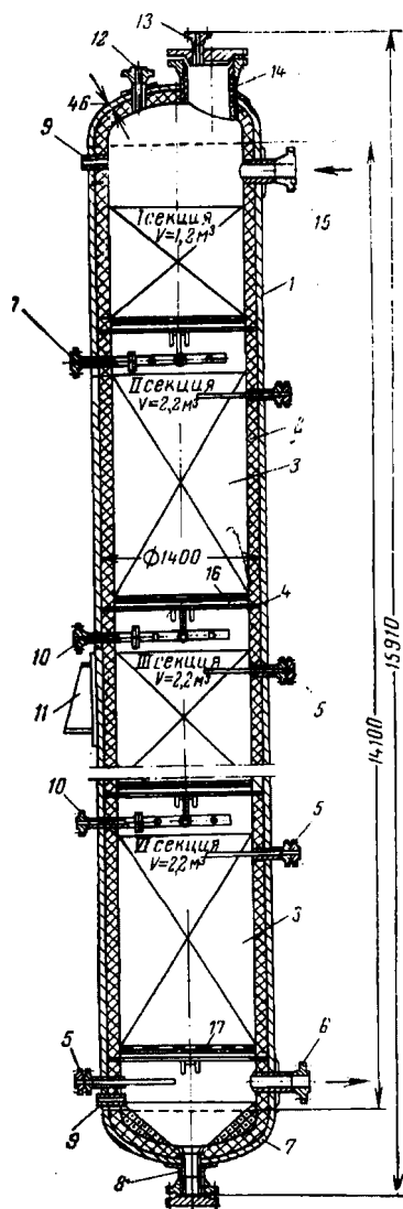
Рис.8.16. Политропический реактор установки гидроочистки дизельных топлив: 1 — корпус; 2 — футеровка; 3 — катализатор; 4 — опорное кольцо; 5 — штуцеры для термомпары; 6 — вывод газосырьевой смеси; 7 — днище; 8 — нижний штуцер; 9 — муфта для манометра; 10 — ввод охлаждающего газа; 11 — опора; 12 — штуцер для предохранительного клапана; 13 — воздушник; 14 — люк; 15 — штуцер ввода газосырьевой смеси; 16 — съемная колосниковая решетка; 17 — опорный перфорированный лист
