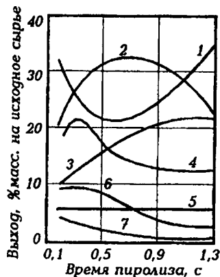
Рис. 5.7. Кинетика образования основных продуктов пиролиза фракций 85... 120°С при 810°С и атмосферном давлении:
