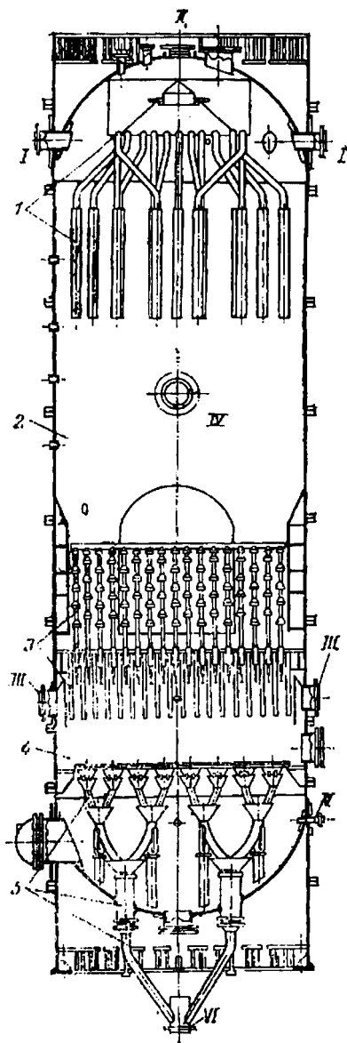
Рис. 6.14. Реактор установки крекинга с шариковым катализатором:
