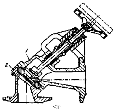
Рис. 2.165. Запорный вентиль: а — прямооточный; б — угловой; 1 — корпус; 2 — входной патрубок; 3 — седло; 4 — золотник; 5 — шпиндель; 6 — сальник; 7 — нажимная гайка; 8 — ходовая гайка
