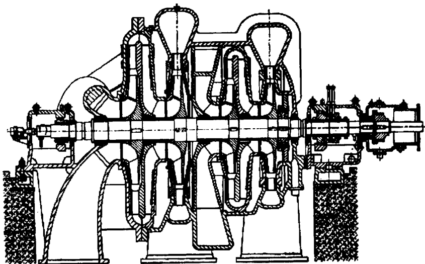
Рис. 2.220. Первый корпус двухкорпусного центробежного компрессора
