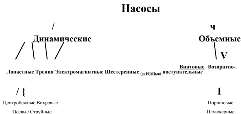
Рис. 2.183. Классификация насосов по принципу действия
