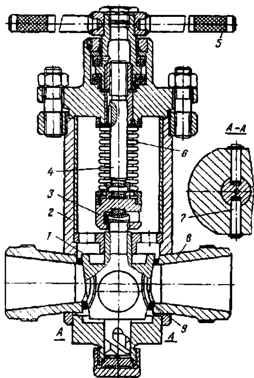
Рис. 2.178. Сильфонный кран:
