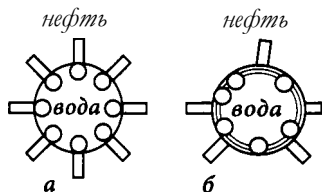
Рис. 3.2. Расположение молекул ПАВ на границе раздела фаз нефть-вода:
