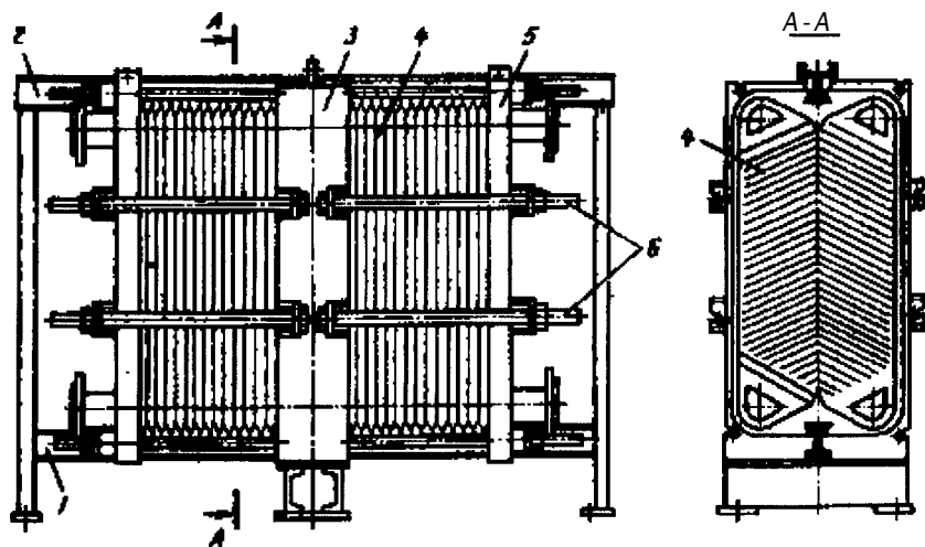
Рис. 2.55. Пластиначый теплообменник (исполнение 3):
