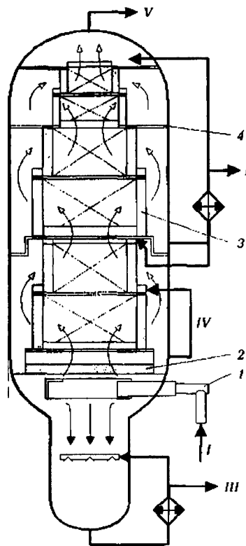
Рис. 3.20. Принципиальная конструкция вакуумной перекрестноточной насадочной колонны АВТ-4 ПО «Салаватнефтеоргсинтез»:
