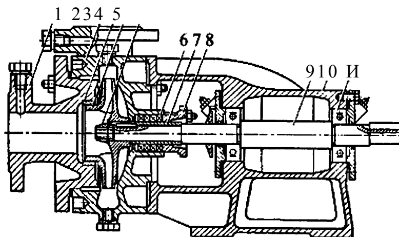
Рис. 2.185. Схема консольного насоса одностороннего всасывания типа К: 1 — крышка корпуса; 2 — корпус; 3 — сменные уплотняющие кольца; 4 — рабочее колесо; 5 — гайка крепления колеса; 6 — набивка сальника; 7 — защитная втулка; 8 — крышка сальника; 9 — вал; 10 — опорный кронштейн; 11 — шарикоподшипник
