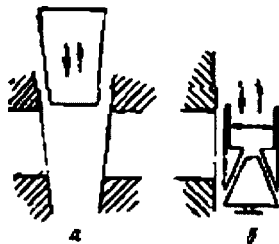
Рис. 2.150. Способы уплотнения шибер: а — клиновой; б — параллельный
