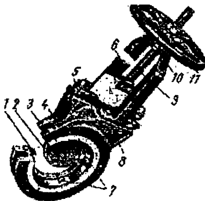
Рис. 2.158. Шиберная задвижка Рeginк: 1 — седло; 2 — шибер; 3 — футеровка; 4 — корпус; 5 — сальник; 6 — бугельная стойка; 7 — направляющая и фиксатор шиберов; 8 — ребро жесткости; 9 — шпindel; 10 — ходовая гайка; 11 — маховик
