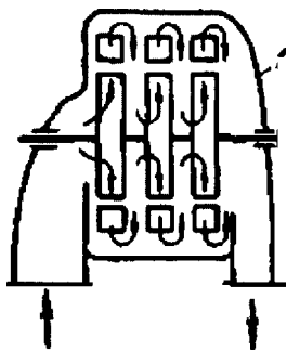
Рис. 2.216. Схема трехступенчатого центробежного нагнетателя:
