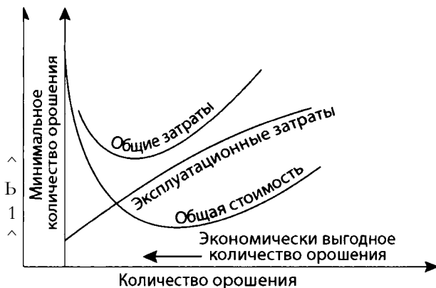
Рис. 3.7. Изменение затрат в зависимости от количества орошения в ректификационной колонне
