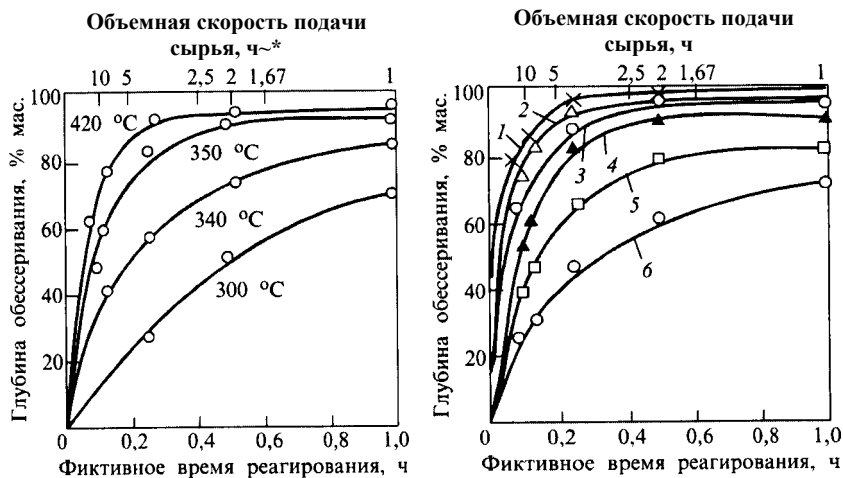
Рис. 8.10. Зависимость глубины обессеривания дизельного топлива от объемной скорости подачи сырья:
