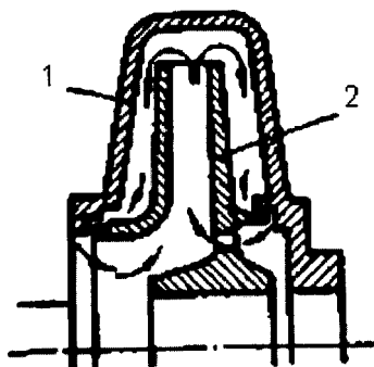
Рис. 2.210. Схема перетока жидкости в корпусе насоса:
