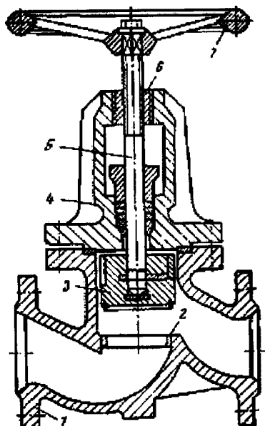
Рис. 2.162. Проходной запорный вентиль с усиленным золотником: 1 — корпус; 2 — седло; 3 — золотник; 4 — крышка со стойкой; 5 — шпindelь; 6 — ходовая гайка; 7 — маховик
