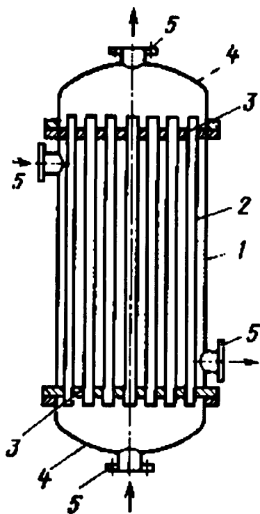
Рис. 2.20. Схема одноходового теплообменного аппарата типа ТН (вертикальное исполнение):
