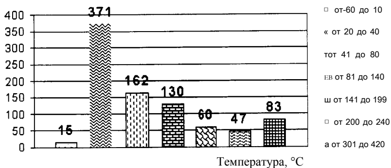
Рис. 2.193. Распределение центробежных насосов по температуре
