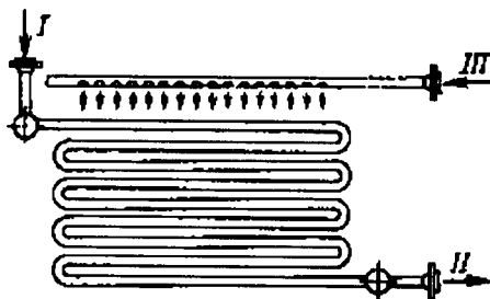
Рис. 2.53. Схема оросительного коллекторного конденсатора-холодильника:
