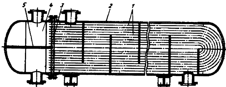
Рис. 2.26. Теплообменник с И-образными трубками
