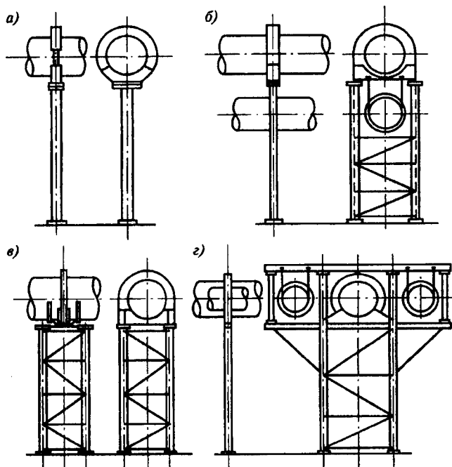
Рис. 2.146. Опоры трубопроводов:
