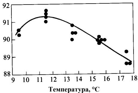
Рис. 6.9. Влияние температуры на октановое число алкилата
