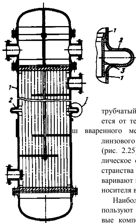
Рис. 2.24. Вертикальный кожухотрубчатый теплообменник типа ТК
