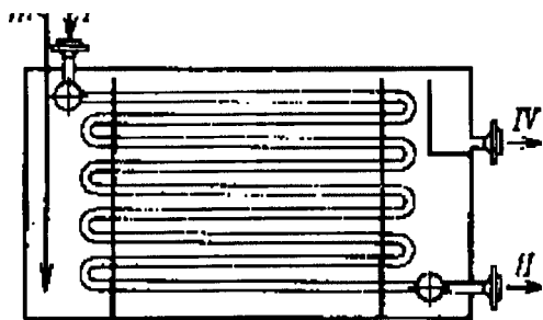
Рис. 2.52. Схема коллекторного погружного конденсатора-холодильника:
