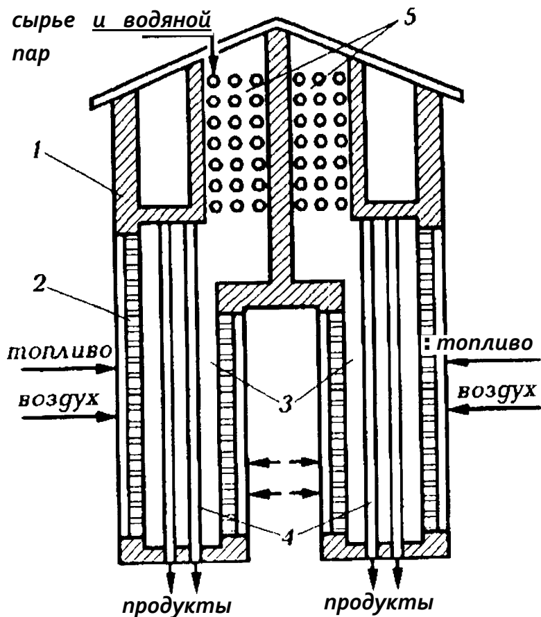
Рис. 5.9. Схема печи пиролиза:
