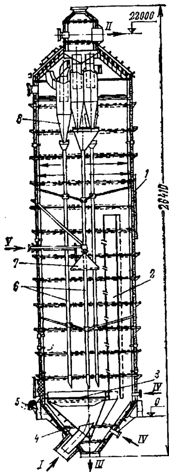
Рис. 6.21. Реактор установки крекинга с пылевидным катализатором:
