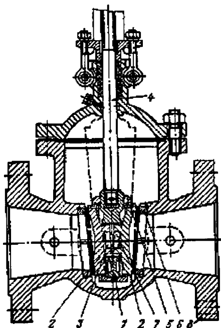
Рис. 2.156. Задвижка с составным клином и выдвижным шпинделем:
