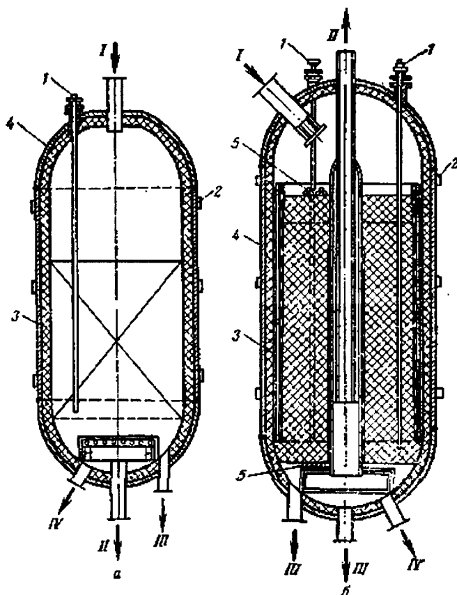
Рис. 8.18. Схема реакторов установки с аксиальным вводом сырья:
