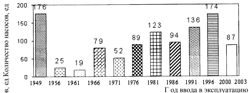
Рис. 2.194. Распределение центробежных насосов по дате ввода в эксплуатацию
