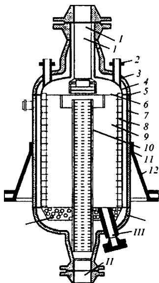
Рис. 8.7. Реактор риформинга: 1 — распределитель; 2 — штуцер для термомпары; 3 — днище верхнее; 4 — кожух; 5 — корпус; 6 — тарелка; 7 — футеровка; 8 — желоб; 9 — катализатор; 10 — труба центральная; II — пояс опорный; 12 — опора; 13 — днище нижнее; 14 — шары фарфоровые; I — ввод сырья; II — вывод продукта; II — вывод катализатора
