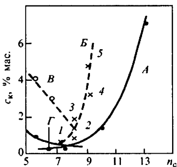
Рис. 8.2. Влияние числа углеродных атомов n_c и группового состава индивидуальных углеводородов на содержание кокса C_k при риформинге на алюмоплатиновом катализаторе: катализатор — 0,37% Р А , 0,9% С 12 ; T = 515^\circ\text{C} ; p = 1 МПа (пунктирная), p = 0,1 МПа (сплошная линия); H_2/CH = 4 ; массовая скорость подачи сырья — 6 ч -1 ; продолжительность — 20 ч: А — н-парафины; Б — ароматические; 1 — м-ксилол; 2 — этилбензол; 3 — о-ксилол; 4 — изопропилбензол; 5 — н-пропилбензол; В — нафтеновые с пятью атомами углерода в кольце; Г — те же с шестью атомами
