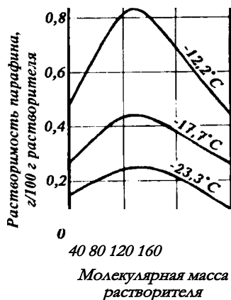
Рис. 4.3. Изменение растворимости парафинов = 50°C) в углеводородных растворителях различной молекулярной массы
