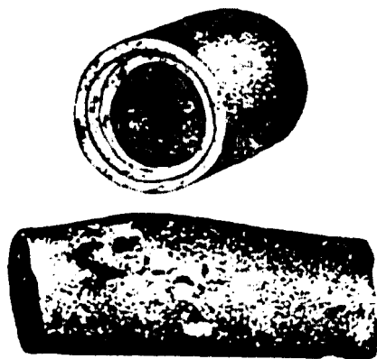
Рис. 2.78. Отдулины на печной трубе
