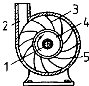
Рис. 2.209. Схема центробежного насоса 1 — вал; 2 — нагнетательный патрубок; 3 — лопасть; 4 — рабочее колесо;
