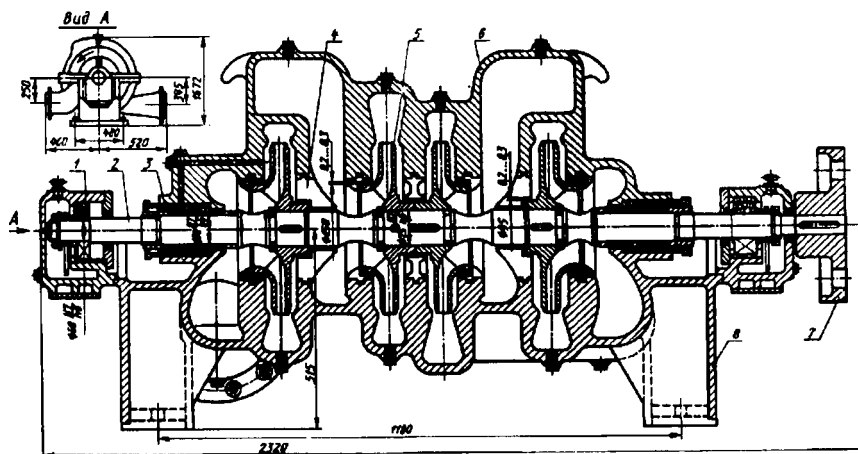
Рис. 2.198. Насос многоступенчатый ЦН 400-210:
