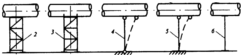
Рис. 2.140. Типы опор трубопроводов:
