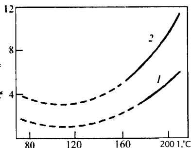
Рис. 8.3. Влияние средних температур кипения гидроочищенных узких бензиновых фракций на закоксовывание катализатора с в процессе их риформинга:
