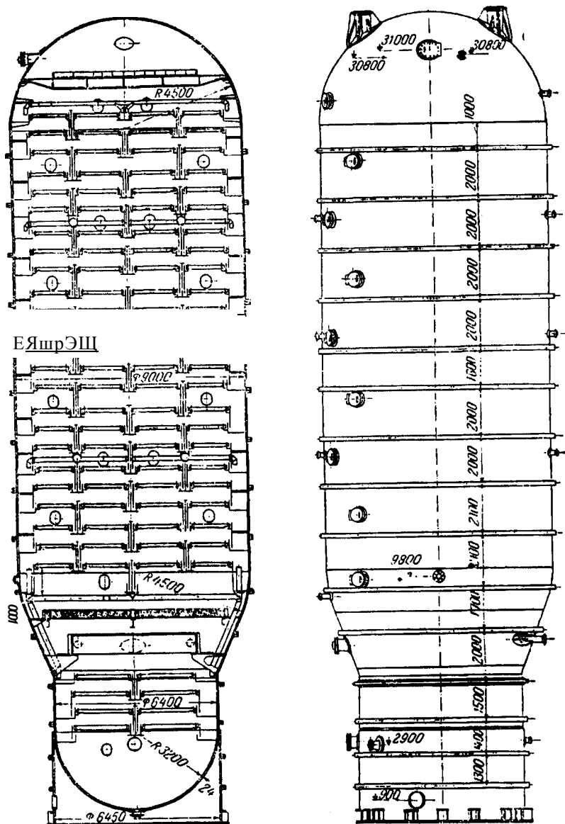
Рис. 2.4. Вакуумная колонна
