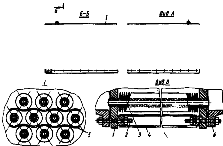
Рис. 2.48. Теплообменная секция АВО
