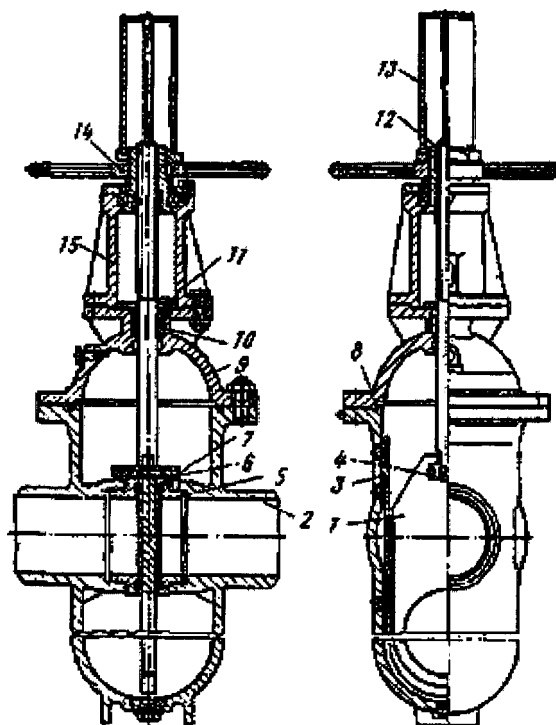
Рис. 2.157. Параллельная однодисковая задвижка:
