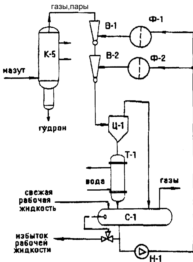
Рис. 3.31. Принципиальная схема двухступенчатой гидроэжекторной системы «Технотон»
