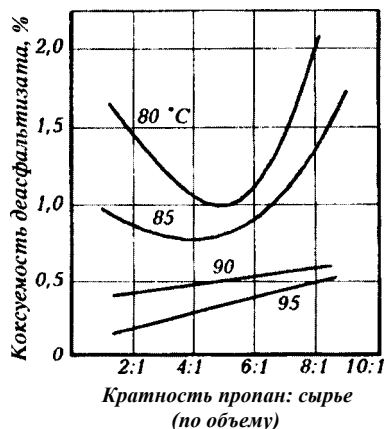
Рис. 4.5. Влияние кратности пропан:сырье на качество деасфальтизатов, получаемых из гудрона западно-сибирских нефтей при различных температурах деасфальтизации (данные В. М. Школьников)
