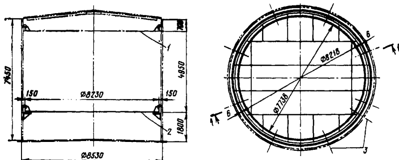
Рис. 2.129. Резервуар с понтоном объемом 400 м 3 : 1 — высшее положение понтона; 2 — положение понтона на кронштейнах; 3 — оси кронштейна
