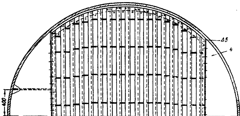
Рис. 2.17. Тарелка с Б-образными элементами:
