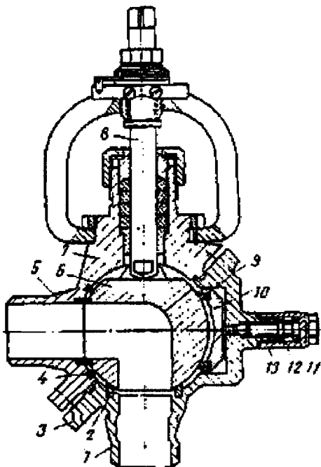
Рис. 2.179. Угловой запорно-регулирующий шаровой кран:
