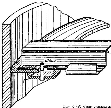
Рис. 2.16. Узел крепления Б-образного элемента к корпусу аппарата
