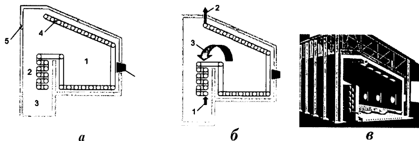
Рис. 2.112. Конструкция однокамерной печи с наклонным сводом:
