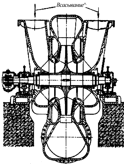
Рис. 2.218. Одноступенчатый нагнетатель с двусторонним колесом
