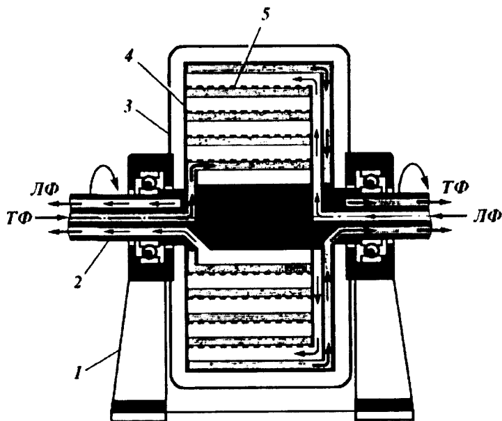
Рис. 4.24. Схема центробежного экстрактора Подбельняка:
