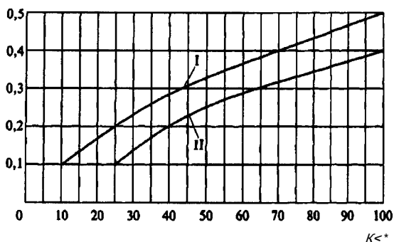
Рис. 2.229. Определение коэффициента B для нахождения остаточного ресурса
