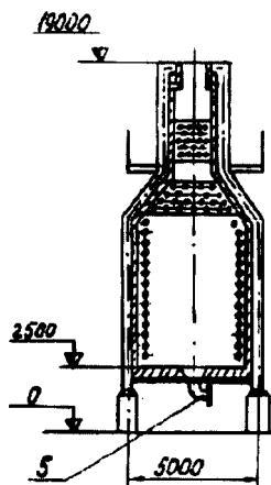
Рис. 2.118. Печь типа ПС: — лестничная площадка; 2 — корпус; 3 — змеевик; 4 — футеровка; 5 — горелка
