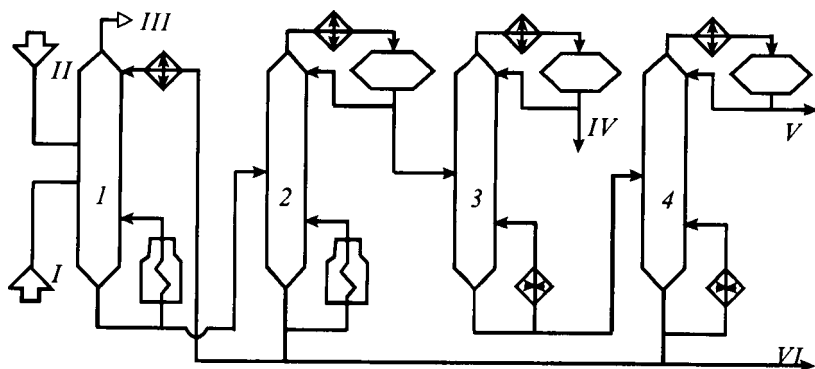
Рис. 3.23. Принципиальная схема абсорбционно-газофункционирующей установки (АГФУ): 1 — фракционирующий абсорбер; 2 — стабилизационная колонна; 3 — пропановая колонна; 4 — бутановая колонна; I — очищенный жирный газ; II — нестабильный бензин; III — сухой газ; IV — пропанпропиленовая фракция; V — бутан-бутиленовая фракция; VI — стабильный бензин
