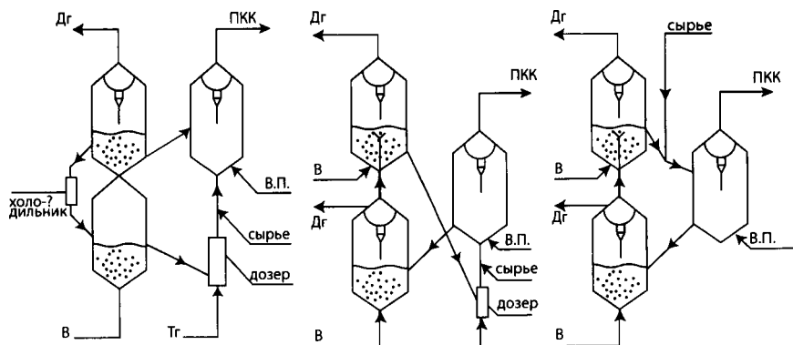
Рис. 6.8. Принципиальная схема реакторного блока установок каталитического крекинга с двухступенчатым регенератором: а - РСС; б — Я-2-Р; в — ККМС
