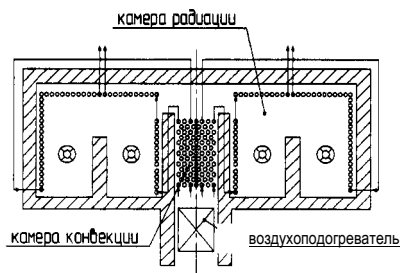
Рис. 2.119. Коробчатые печи с горизонтальным расположением змеевиков
