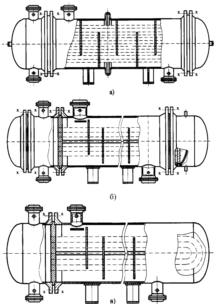
Рисунок 2.19. Основные типы кожухотрубчатых теплообменных аппаратов: а) - с неподвижными решетками (ТН) или с компенсатором на кожухе (ТК); б) - с плавающей головкой; в) - с и-образными трубами
