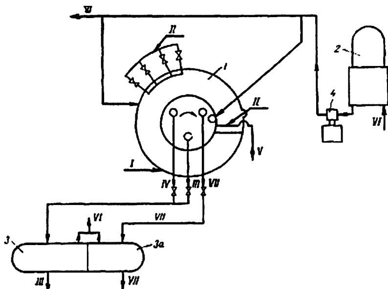
Рис. 4.19. Схема вакуумного фильтра непрерывного действия:
