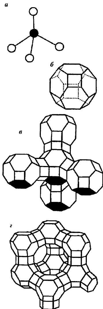
Рис. 6.2. Строение цеолитов типа фожазита:
