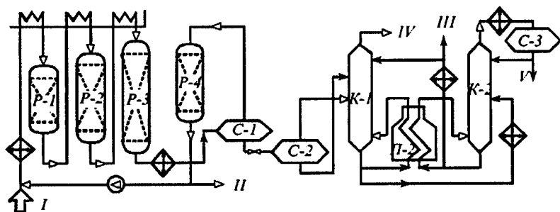
Рис. 8.6. Принципиальная технологическая схема установки каталитического риформинга со стационарным слоем катализатора: I — гидроочищенное сырье; II — ВСГ; III — стабильный катализат; IV — сухой газ; V — головная фракция
