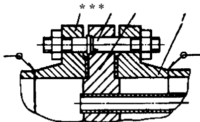
Рис. 2.29. Способ крепления распределительной камеры к кожуху теплообменника
