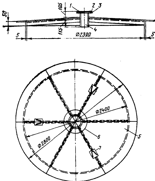
Рис. 2.128. Центральный щит покрытия:
