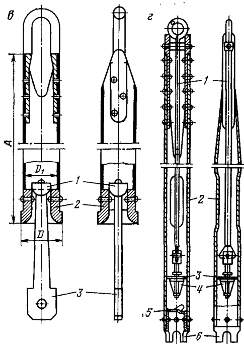
Рис. I.10. Желонки:
