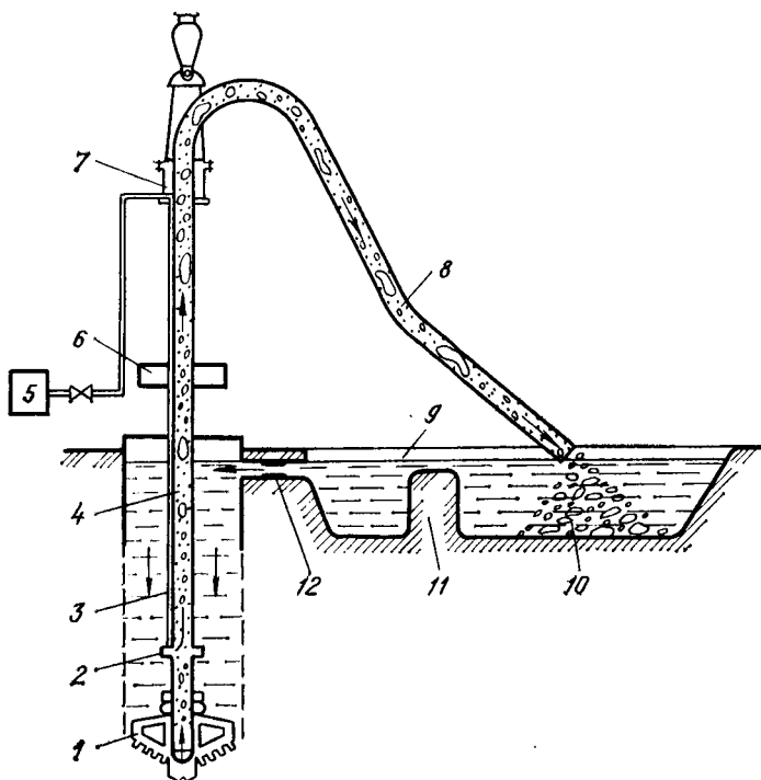
Рис. П.2. Схема бурения с обратной промывкой при использовании для создания циркуляции эрлифта:
