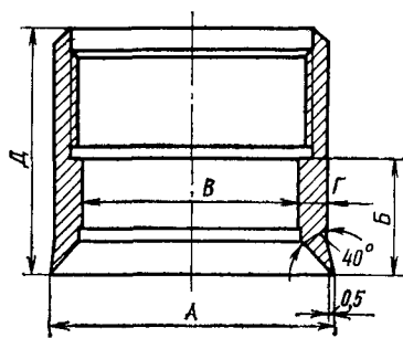
Рис. I.16. Трубный башмак
