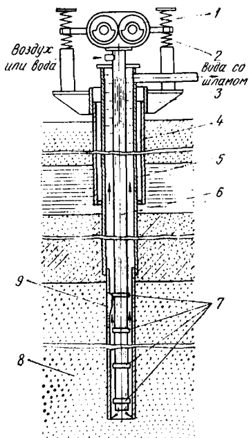
Рис. VI.8. Схема виброустановки:
