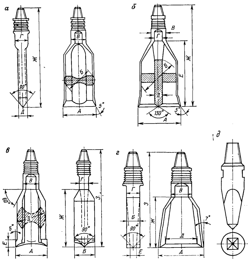
Рис. 1.8. Долота:
