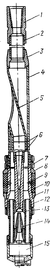
Рис. V.6. Струйный аппарат (эжекторный насос) типа НЭ-8-12:
