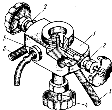
Рис. III.12. Переводник для извлечения пробы из пробоотборников
