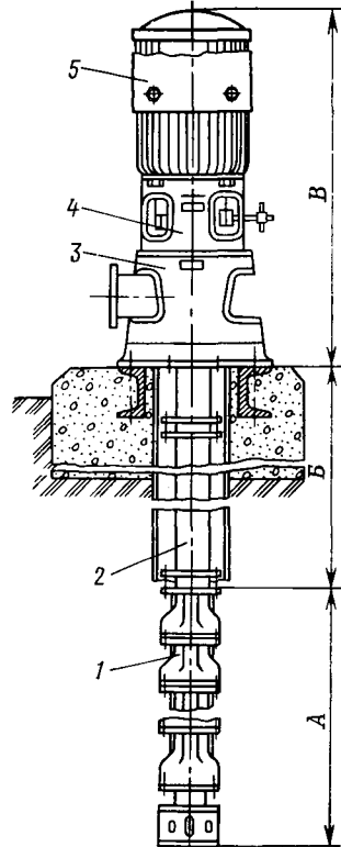
Рис. V.15. Насосная установка типа АТН:
