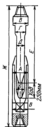
Рис. I.13. Раздвижная штанга
