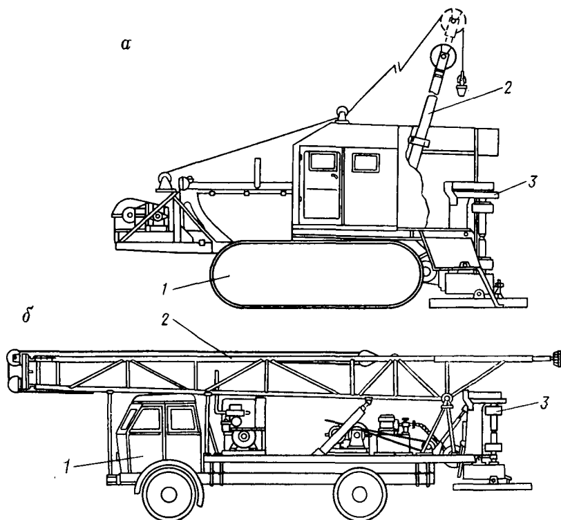
Рис. 1.39. Самоходная трубоподъемная установка на базе трактора Т-100М (а) и автомашины МАЗ-500 (б): 1 — транспортная база; 2 — мачта; 3 — гидравлический домкрат
