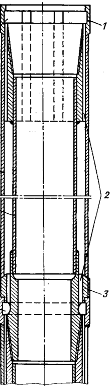
Рис. II.13. Соединения бурильных труб:
