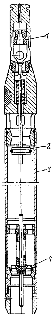
Рис. III.10. Герметичный пробоотборник
