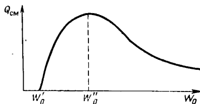
Рис. V.4. Зависимость производительности эрлифта от удельного расхода воздуха
