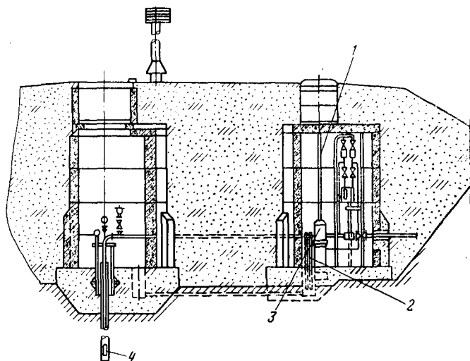
Рис. V.11. Типовая подземная насосная станция с насосами ЭЦВ:
