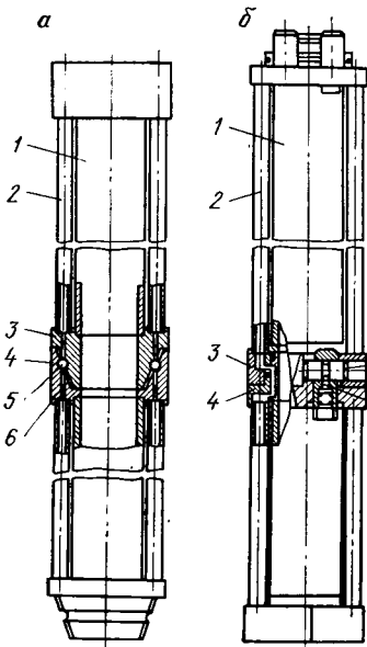
Рис. II.13. Соединения бурильных труб:
