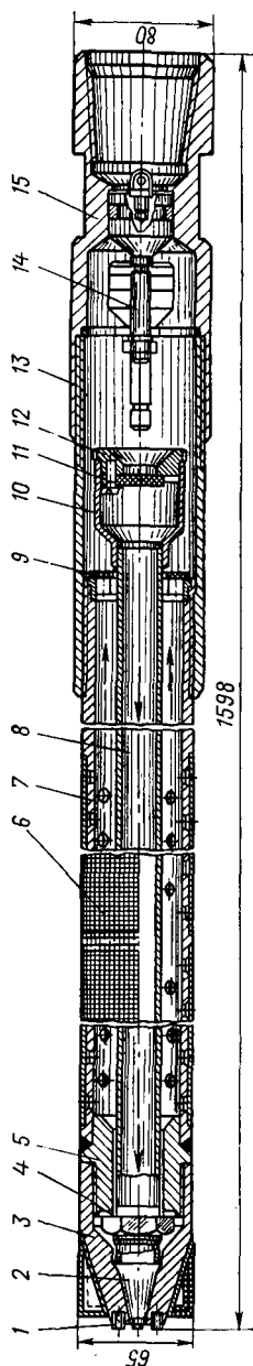
III.1 Фильтр-опробователь
