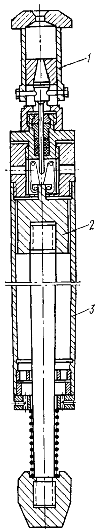
Рис. III.9. Поршневой бесклапанный пробоотборник
