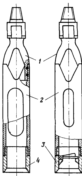
Рис. I.9. Забивные стаканы:
