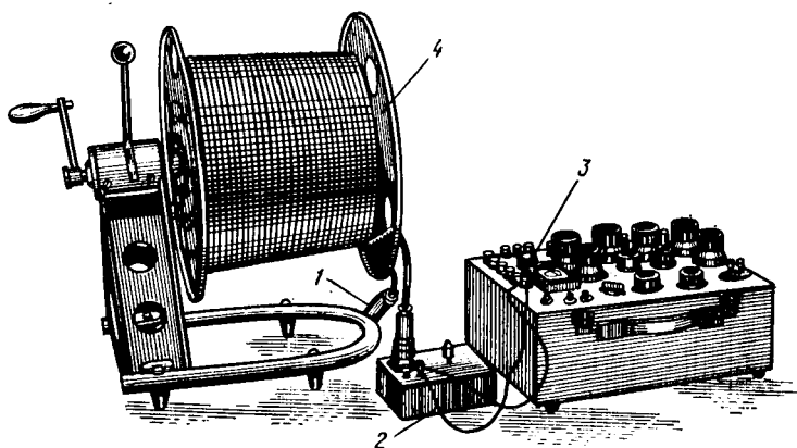
Рис. IV.5. Измеритель температуры ИТ:
