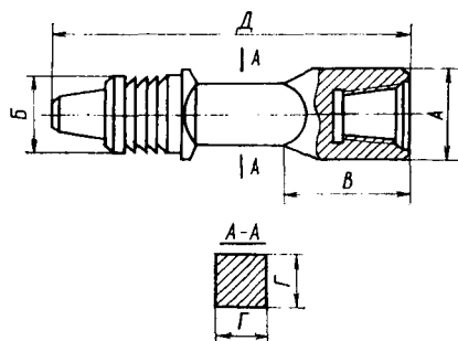
Рис. I.15. Резьбовой переводник
