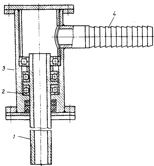
Рис. II.14. Специальный вертлюг: 1 — ствол; 2 — подшипники; 3 — корпус; 4 — штуцер
