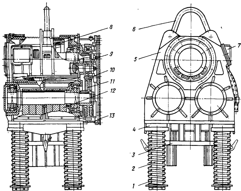
Рис. 1.28. Вибромолот ВВС-1:
