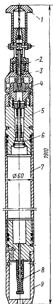
Рис. III.11. Вакуумный пробоотборник
