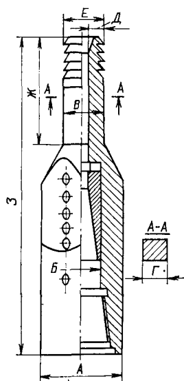
Рис. I.13. Раздвижная штанга
