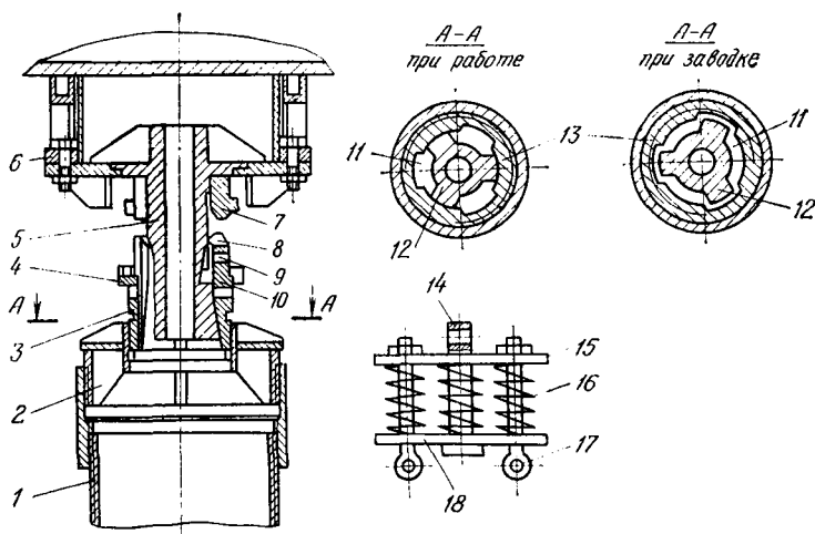
Рис. I.30. Самозаклинивающийся захват и амортизатор:
