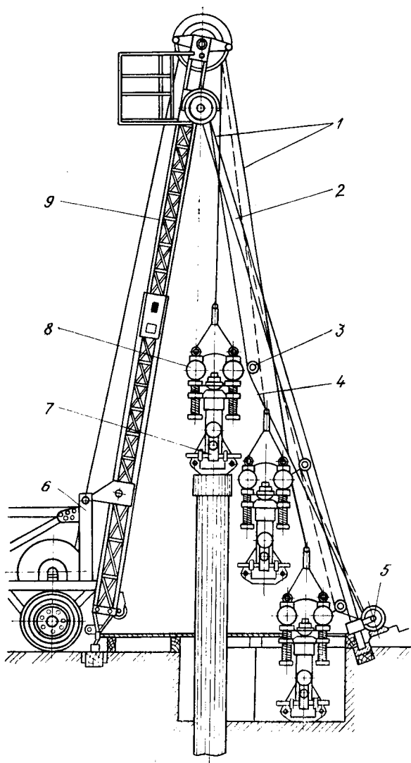
Рис. I.38. Схема установки и снятия вибромолота с колонны обсадных труб устройством УСВ-1:
