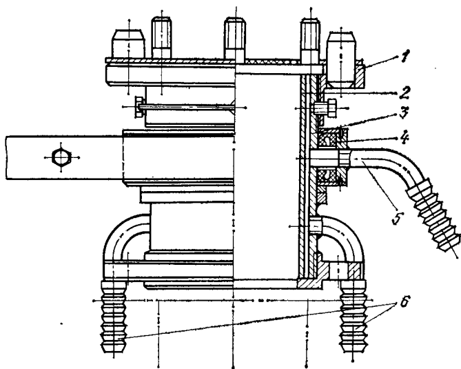
Рис. II.10. Переходный вертлюг-воздухораспределитель:
