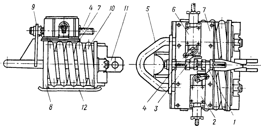
Рис. I.29. Ограничитель натяжения троса:
