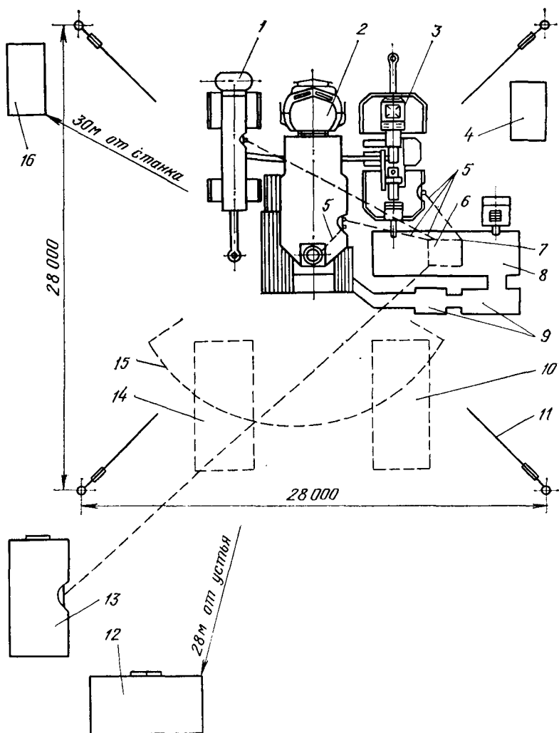
Рис. VI.18. Типовая схема защитного заземления установки вращательного бурения:
