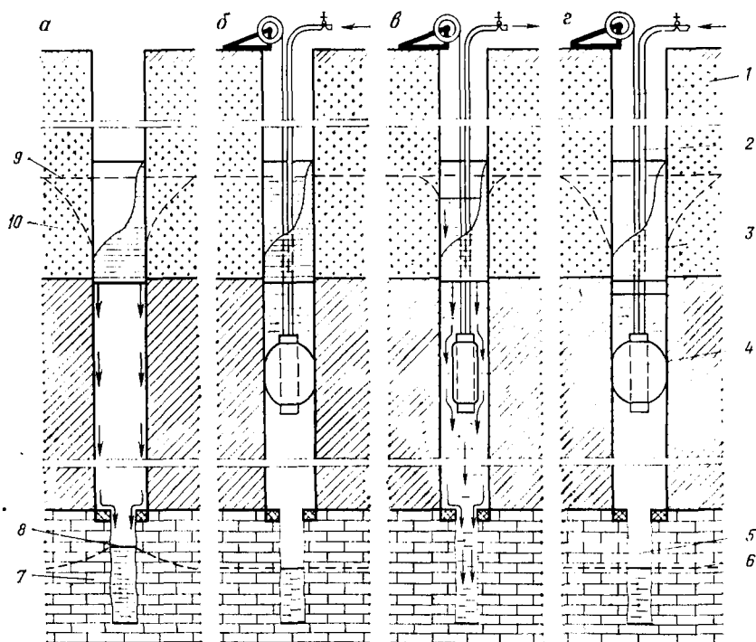
Рис. VI.7. Схема имплозионной обработки поглощающей скважины:
