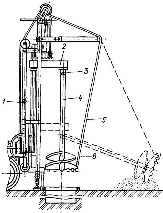
Рис. II.20. Схема сброса породы с рейсового шнека при бурении установкой УШБМ-16:
