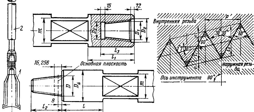
Рис. 1.7. Резьбовое конусное соединение
