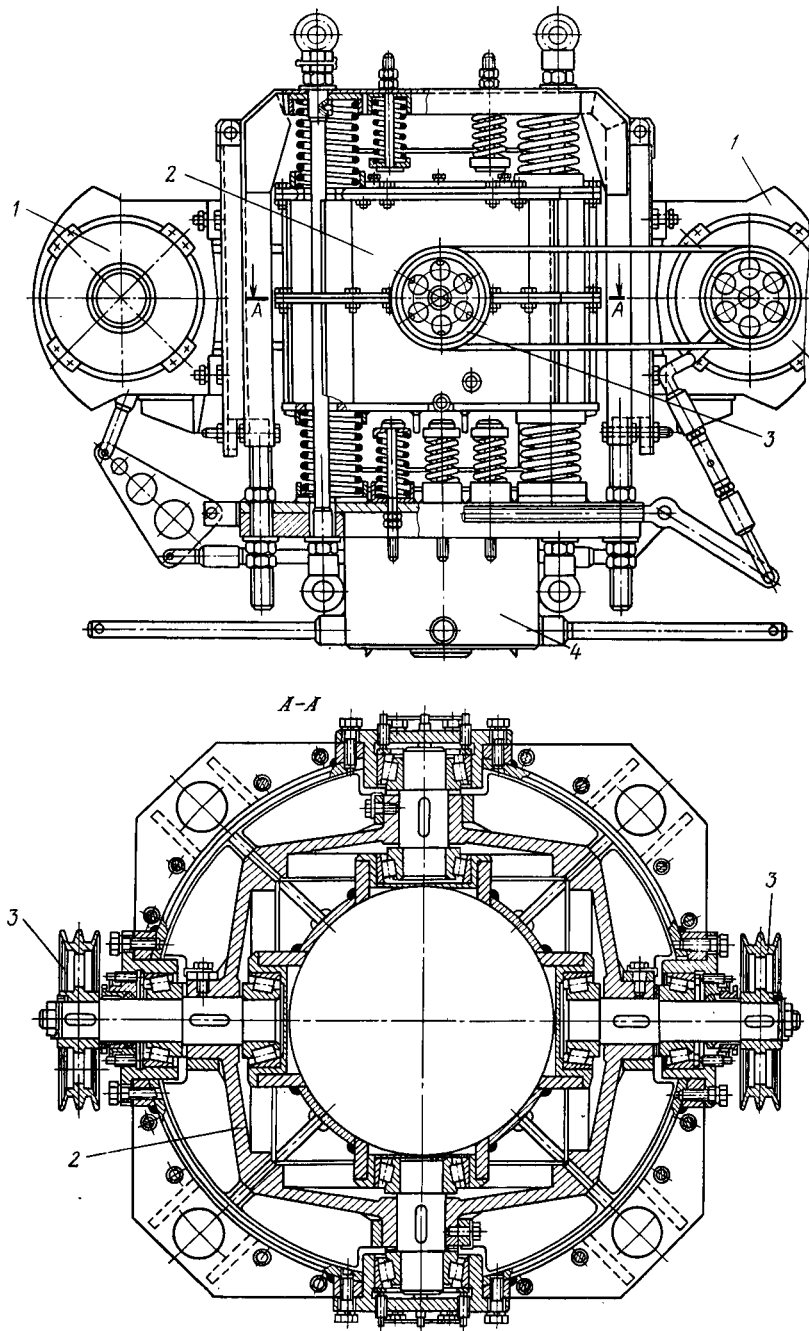
Рис. 1.27. Вибратор ВО-10:
