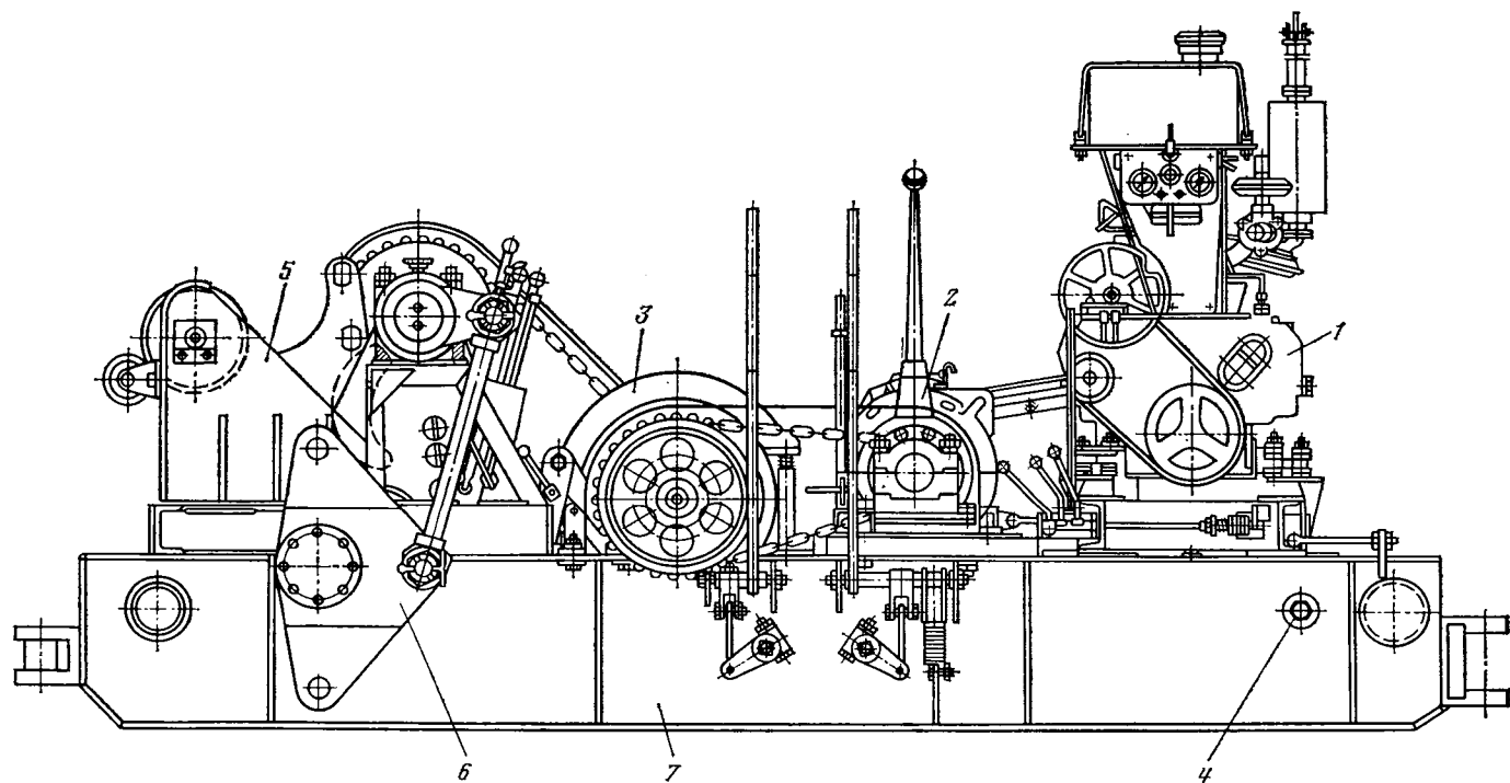
Рис. 1.5. Буровой станок БУГ-100М:
