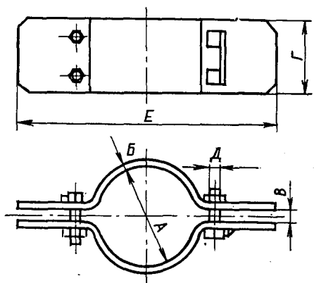
Рис. I.19. Хомут
