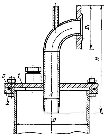
Рис. V.14. Оголовка устья скважины комбинированной конструкции треста «Промбурвод»:
