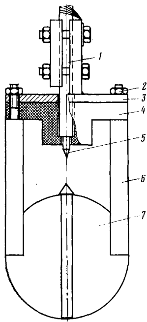
Рис. VI.4. Жидкостный разрядник с отрицательным электродом в виде пересекающихся дисков
