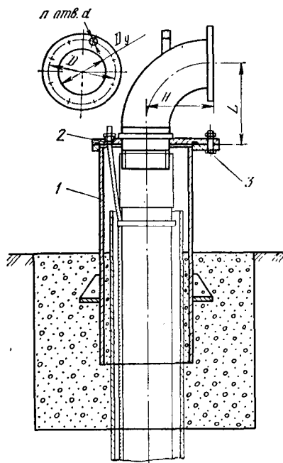
Рис. V.13. Оголовка устья скважины конструкции СКТБН:
