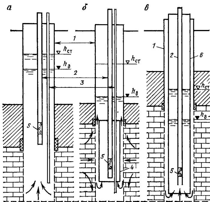
Рис. V.1. Схемы эрлифта:
