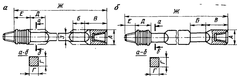
Рис. 1.11. Ударные штанги:
