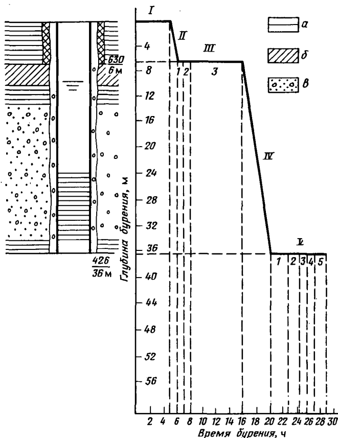
Рис. II.24. Конструкция скважины и график затрат времени на ее сооружение:
