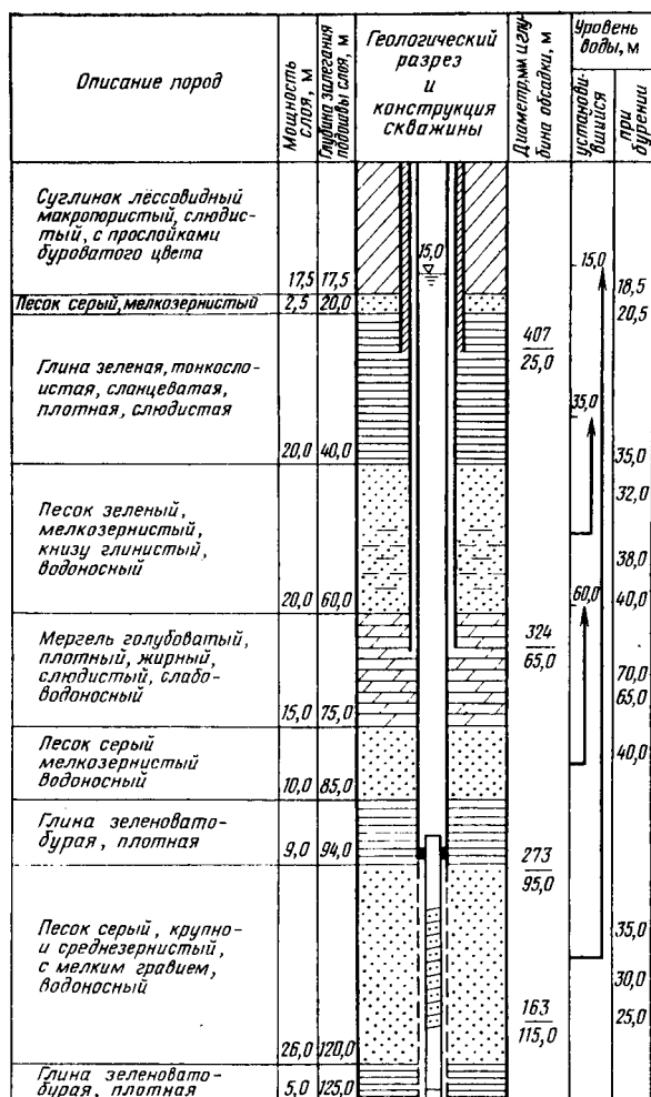
Рис. I.25. Конструкция скважины при каптаже воды из рыхлых пород:
