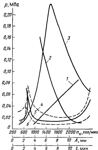
Рис. VI.9. Зависимость амплитуды колебания гидродинамического давления p от технологических параметров:
