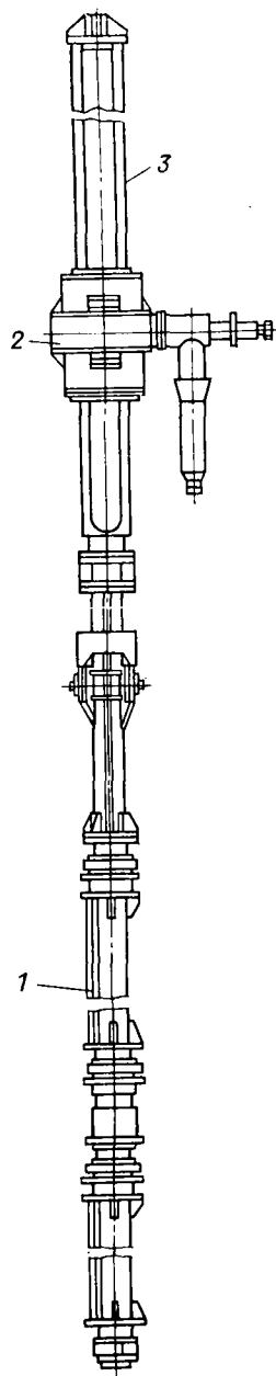
Рис. II.15. Буровой инструмент конструкции ППО «Востокбурвод»
