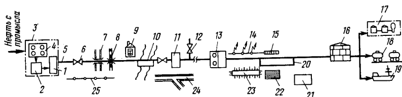
Рис. 19. Схема магистрального нефтепровода
