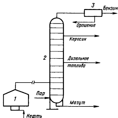
Рис. 17. Схема разделения нефти в ректификационной колонне
