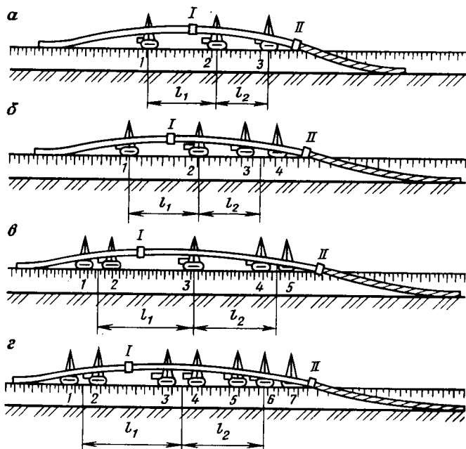
Рис. 35. Схема проведения изоляционно-укладочных работ совмещенным способом при диаметрах трубопровода (в мм) 529 — 820 ( a ), 1020 ( б ), 1220 ( в ) и 1420 ( г ):
