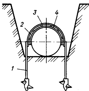
Рис. 37. Схема закрепления трубопровода винтовым анкером:
