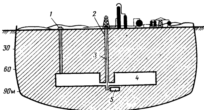
Рис. 29. Шахтное хранилище:
