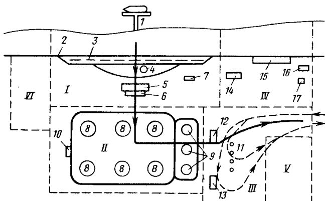
Рис. 21. План нефтебазы с разбивкой по зонам I—V/:
