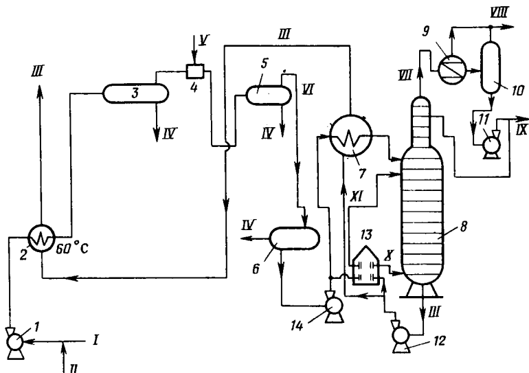
Рис. 14. Технологическая схема УКПН
