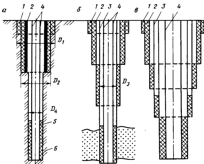
Рис. 8. Конструкция скважин
