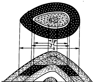
Рис. 5. Сводовая газонефтяная залежь:
