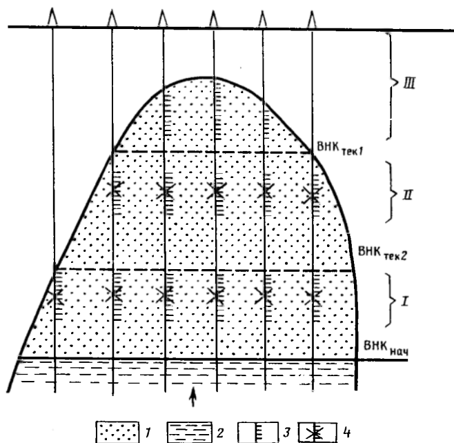
Рис. 138. Последовательный перенос интервалов перфорации при разработке массивной залежи.
