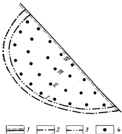
Рис. 84. Незамкнутые ряды добывающих скважин.
