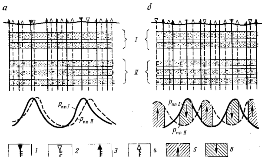
Рис. 74. Профили пластового давления p_{пл} эксплуатационных объектов I и II при разном размещении нагнетательных и добывающих скважин.
