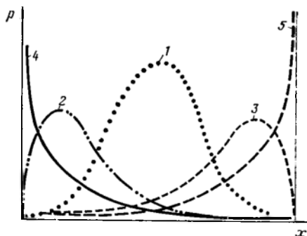
Рис. 12. Основные типы кривых распределения значений геологических признаков.
