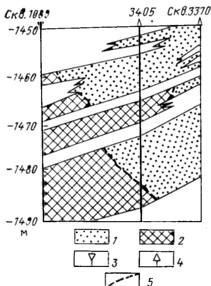
Рис. 124. Схематический геологический профиль по горизонту D 1 Абдрахмановской площади.
