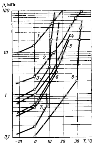
Рис. 48. Диаграмма гетерогенного состояния газов (по Ю. Ф. Мажогуну).
