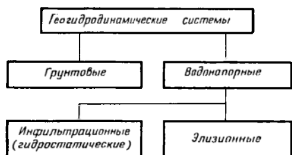
Рис. 54. Классификация геогидродинамических систем
