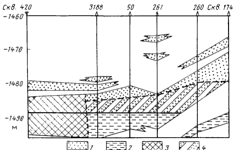
Рис. 124. Схематический геологический профиль по горизонту D 1 Абдрахмановской площади.
