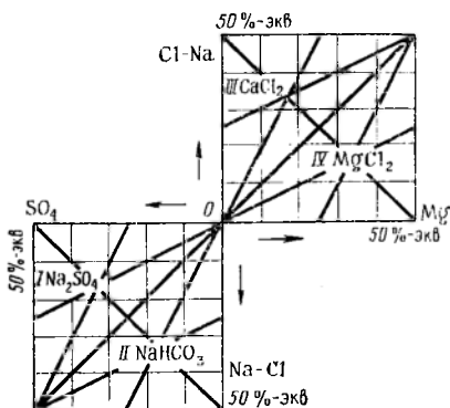
Рис. 51. Классификация подземных вод по В. А. Сулину.
