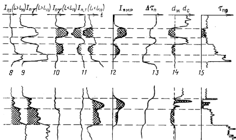
Рис. 5. Характеристика коллекторов по данным различных геофизических методов исследования скважин (по В. Н. Дахнову).
