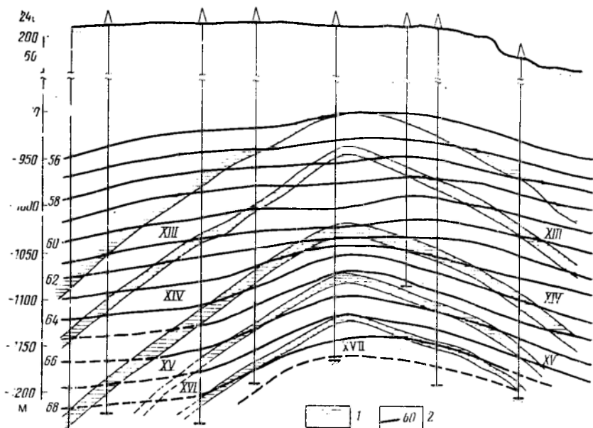
Рис. 60. Схематический геолого-геотермический профиль месторождения Узень (по В. А. Луткову).
