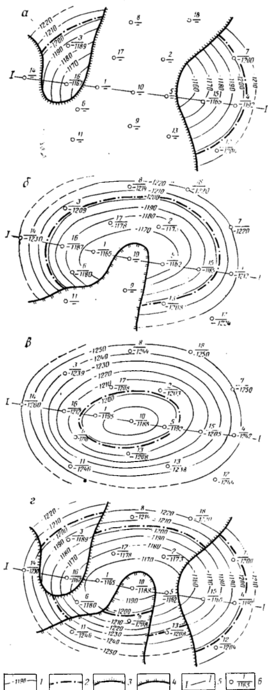
Рис. 44. Пример определения в многопластовом объекте разработки положения внешнего контура нефтеносности.
