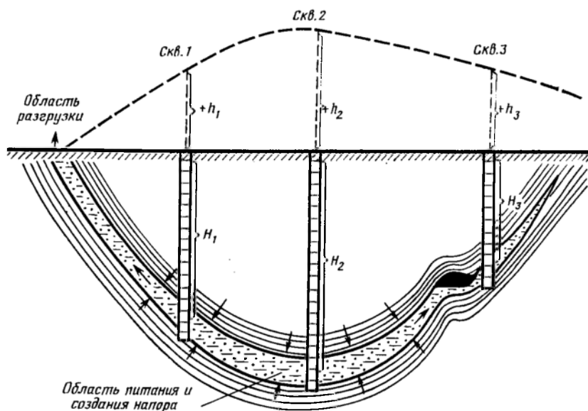
Рис. 55. Схема элизионной водонапорной системы.
