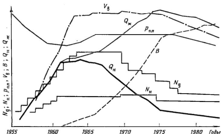
Рис. 92. График разработки нефтяного эксплуатационного объекта.
