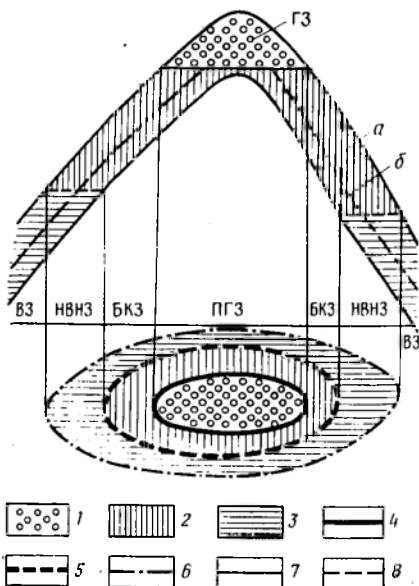
Рис. 18. Схематическое отображение метаструктуры и метанеоднородности залежи нефти и газа на геологическом профильном разрезе и в плане (по В. С. Керим-Заде).
