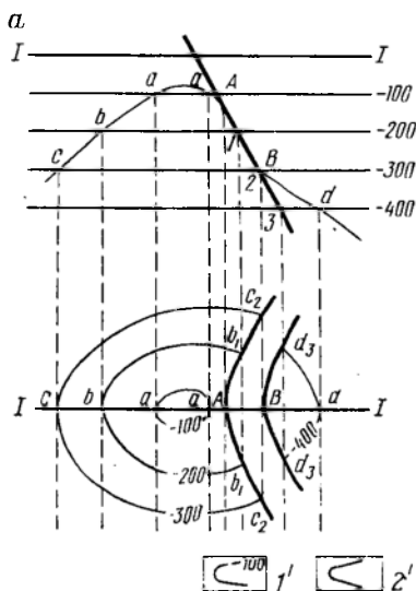
Рис. 34. Принципиальная схема изображения поднятий, осложненных сбросом (а) и взбросом (б). 1' — изогипсы пласта, м; 2' — горизонтальные проекции следов пересечения кровли пласта с поверхностью нарушения; 3' — сброс и взброс; 4' — профили; а—г, 1—4, А, В — проекции точек, необходимых для построения карты
