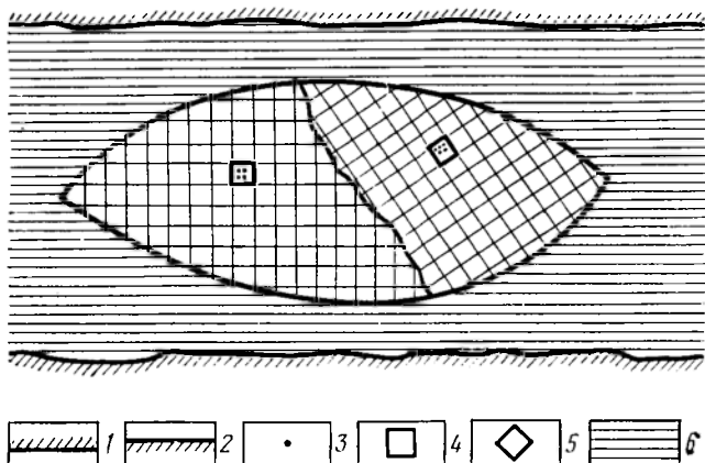
Рис. 1. Линза терригенного коллектора как система.
