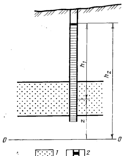
Рис. 52. Пьезометрическая высота и напор в скважине.
