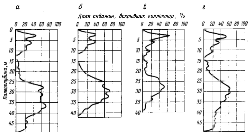
Рис. 21. Групповые геолого-статистические разрезы продуктивных отложений яснополянского надгоризонта Арланского месторождения.
