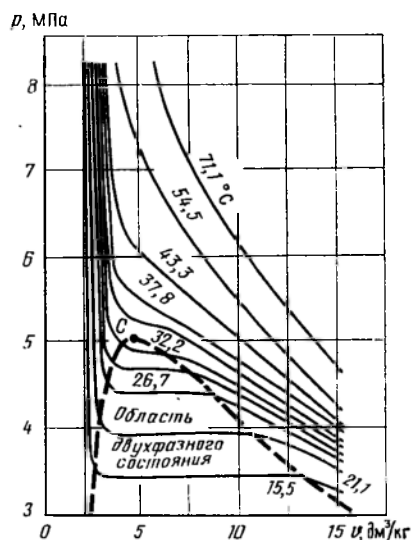
Рис. 46. Диаграмма фазового состояния чистого этана (по Ш. К. Гиматудинову).
