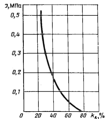
Рис. 7. Усредненная кривая капиллярное давление p — водонасыщенность k_B для образцов со средней проницаемостью 0,15 мкм 2 (по Ш. К. Гиматудинову)
