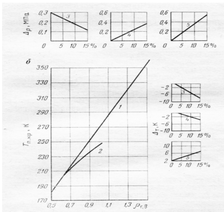
2.4-рasm. Ҳаво бўйича \rho_{г.хаво} углеводород газларининг зичликларига псевдокритик босим P_{п.кр.} (а) ва температура T_{п.кр.} (б) нинг боғлиқлик графиги (Ю.П.Гаттенбергер бўйича).
