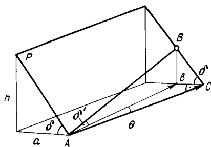
РИС. 5.4. К определению зависимости между направлением штрека и линией простирания пласта
