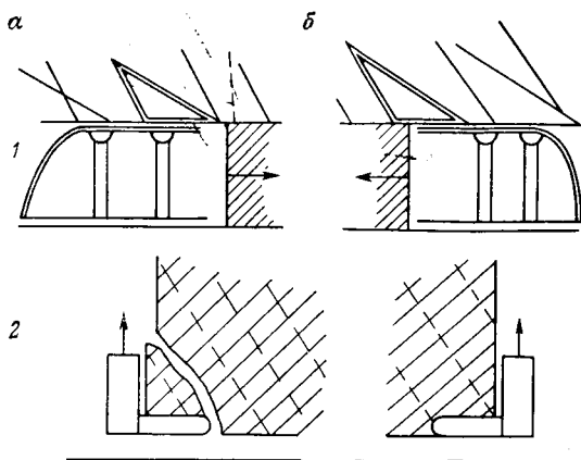
РИС. 11.9. Схема влияния ориентировки трещин на крепление (1) и работу комбайна в очистном забое (2):
