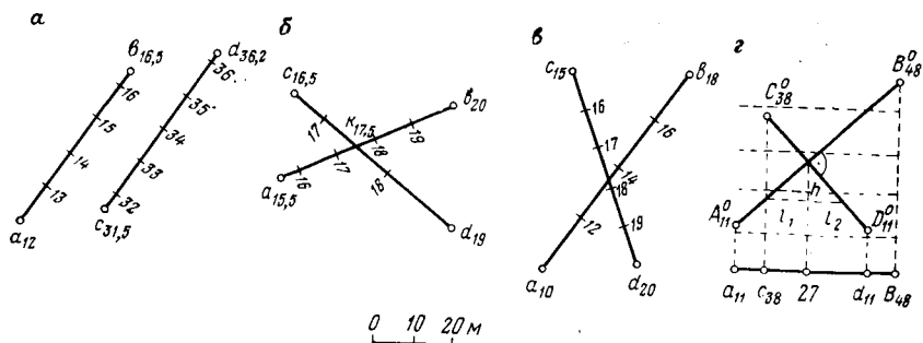
РИС. 2.4. Взаимное положение прямых
