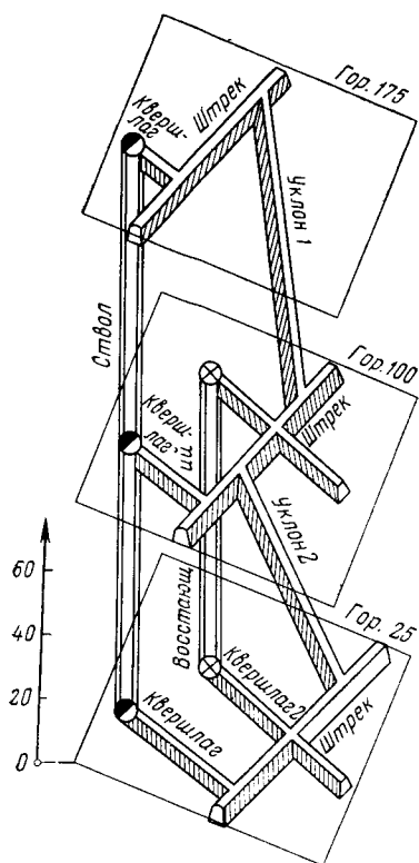
РИС. 2.32. Векторная проекция горных выработок
