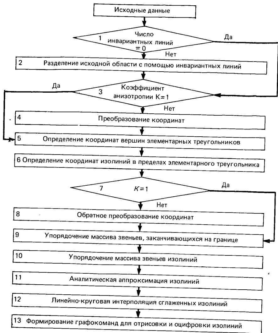
РИС. 2.17. Блок-схема алгоритма построения плана изолиний по методу многогранника
