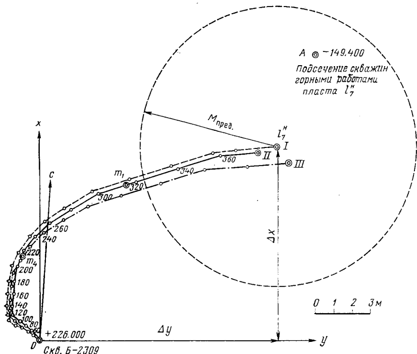
РИС. 5.16. Инклинограмма оси скважины и предельная погрешность определения забоя
