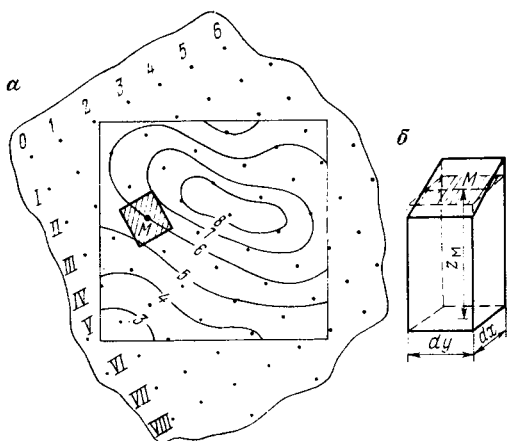
РИС. 18.4. К определению объема тела, ограниченного топографической поверхностью и горизонтальной плоскостью, палеткой П. К. Соболевского: а — изо мощности залежи; б — вертикальные призматические столбики, на которые мысленно делится объем тела наложением палетки
