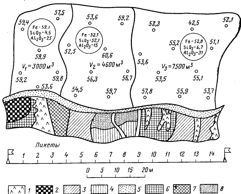
РИС. 16.5. План-карта забоя гор. +75 м Лебединского карьера:
