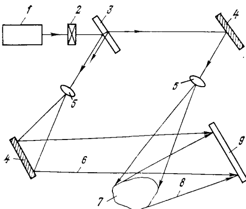
РИС. 2.43. Схема восстановления объемного изображения предмета по голограмме:
