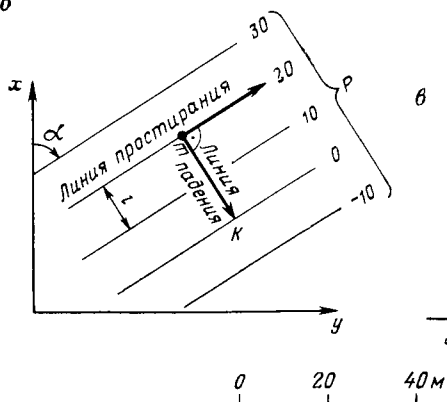
РИС. 2.5. Изображение плоскости в проекциях с числовыми отметками
