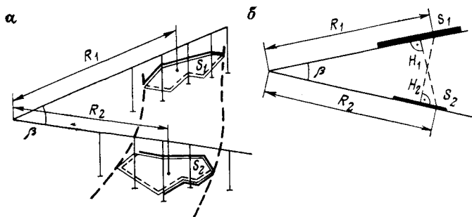
РИС. 18.7. К подсчету запасов при непараллельных разрезах при значительных (а) и малых (б) углах между сечениями
