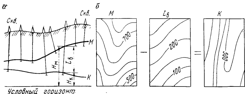
РИС. 8.2. Схема построения гипсометрического плана малоразведанного пласта K :
