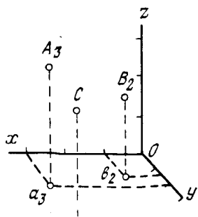
РИС. 2.34. Аксонометрические проекции точек
