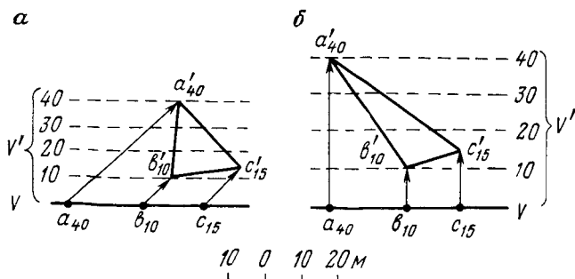
РИС. 2.29. План ( V ) и векторная проекция ( V' ) вертикальной плоскости при косом ( a ) и нормальном ( b ) направлении векторов
