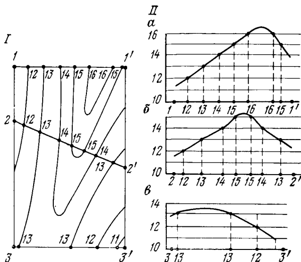
РИС. 2.14. К построению изолиний поверхности I методом профилей II по линиям a — I-I' ; b — 2-2' ; c — 3-3'
