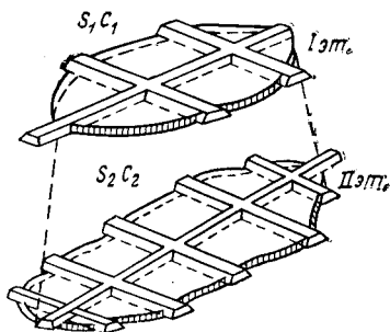
РИС. 17.8. Схема блока между двумя горизонтами горноразведочных работ
