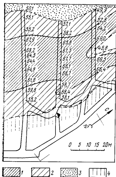
РИС. 12.2. Часть плана опробования железорудной залежи:
