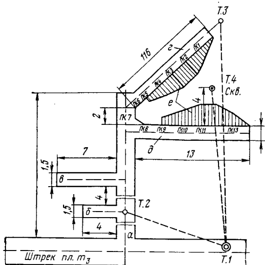
РИС. 5.17. Схема поиска скважины из горных выработок .
