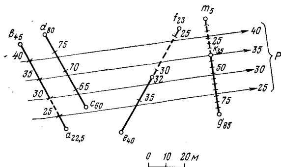
РИС. 2.6. Взаимное положение точек и прямых с плоскостью
