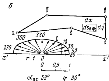
РИС. 2.26. Построение масштабного полуэллипса для непосредственного измерения углов и длин по аффинной проекции горизонтального плана
