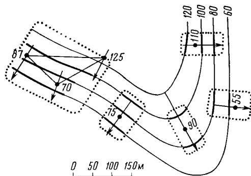
РИС. 2.13. Схема построения изолиний поверхности методом многогранника
