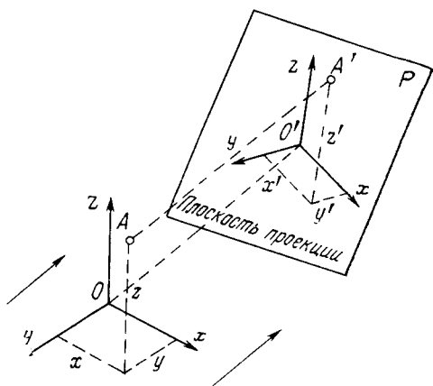
РИС. 2.33. Схема аксонометрического проектирования
