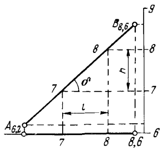
РИС. 2.3. Градуирование прямой с помощью трафарета
