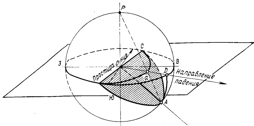
РИС. 2.39. Изображение прямой и плоскости на стереографической сетке
