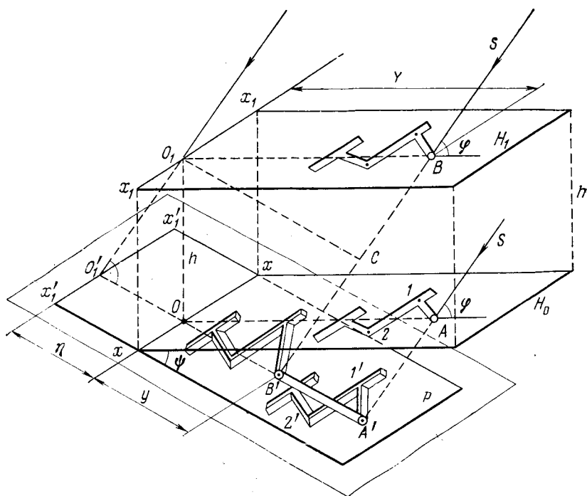
РИС. 2.21. Схема аффинного проектирования
