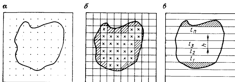
РИС. 17.5. Палетки для определения площади:
