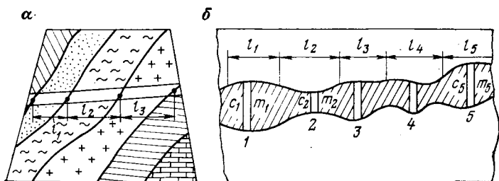
РИС. 17.7. Схема секционного опробования забоя (а) и стенки (б) штрека
