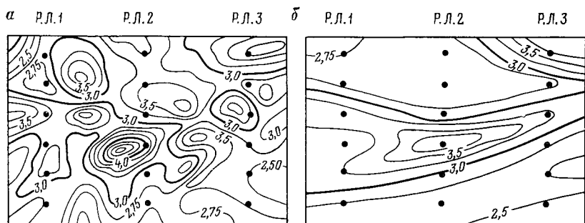
РИС. 2.15. К построению изолиний поверхности по профилям:
