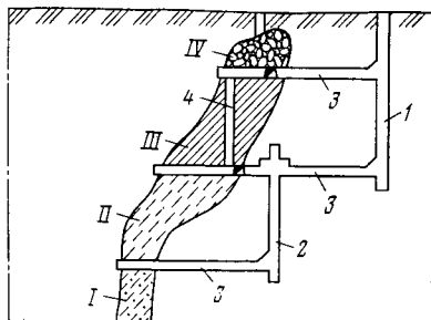
РИС. 20.1. Схема расположения балансовых запасов при подземной разработке:
