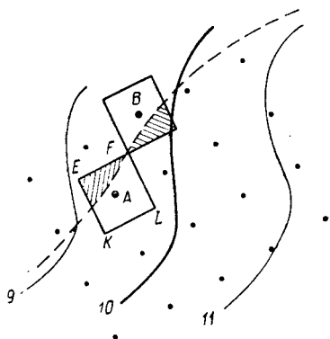
РИС. 18.5. Участок плана с изомощностями залежи, контуром подсчета и наложенной точечной палеткой
