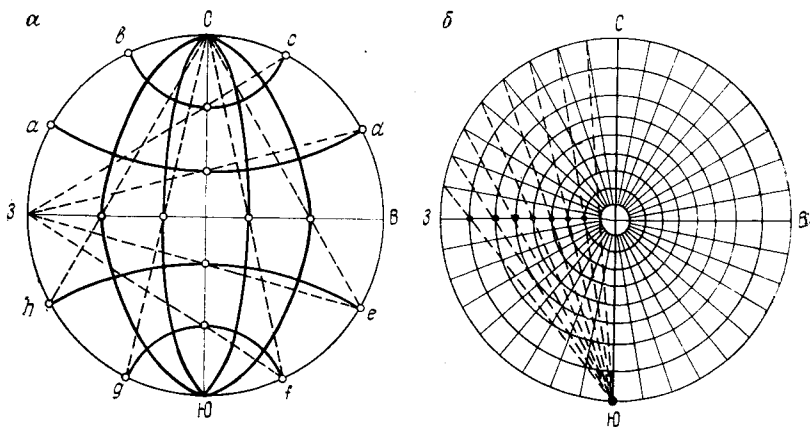
РИС. 2.38. Построение меридиональной (а) и полярной (б) сеток
