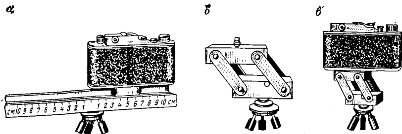
РИС. 5.8. Линейка (а) и шарнирное устройство (б, в) для стереофото съемки забоев
