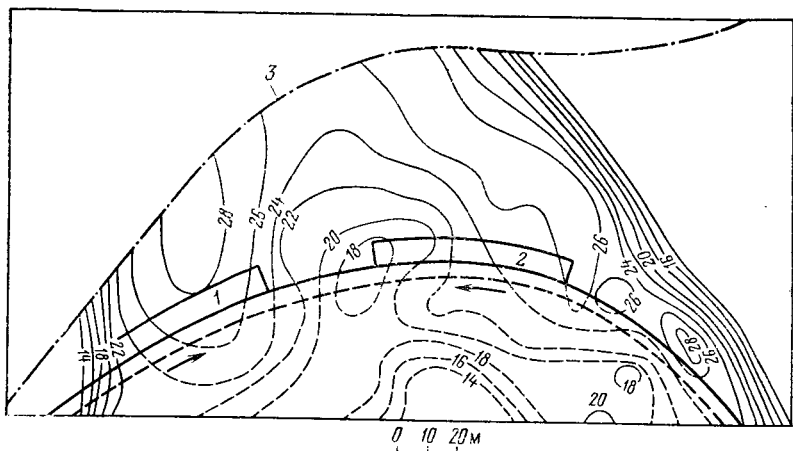
РИС. 16.2. План размещения технологических типов руд по уступу Ново-Криворожского месторождения:
