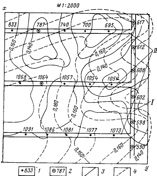
РИС. 15.5. План в изолиниях содержания фосфора в руде по участку шахты № 8 Марганецкого ГОКа:
