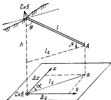
РИС. 5.14. Графическое определение координат точек оси скважины:
