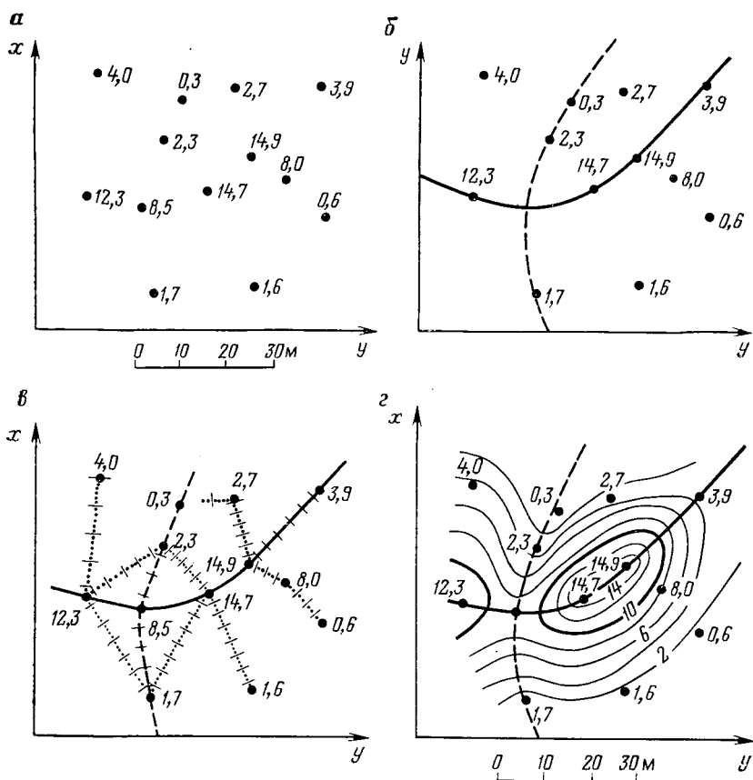
РИС. 2.12. Последовательность построения на плане изолиний топографической поверхности методом инвариантных линий
