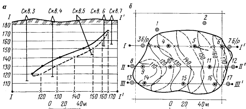
РИС. 8.1. Построение профиля и гипсометрического плана залежи: а — разрез по линии I—I'; б — план поверхности кровли и почвы залежи
