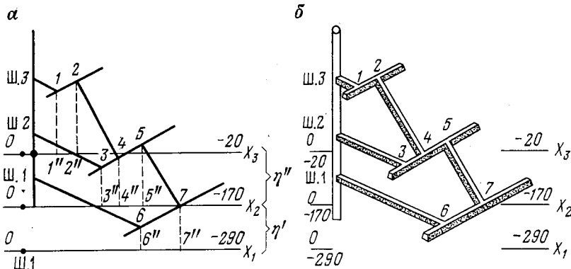
РИС. 2.23. Последовательность построения изображения горных выработок в аффинной проекции
