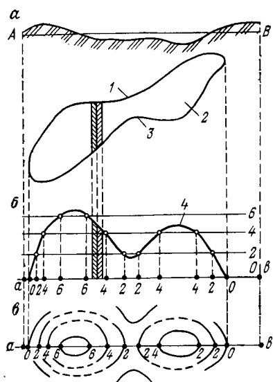
РИС. 8.4. Схема построения изомощностей залежи:
