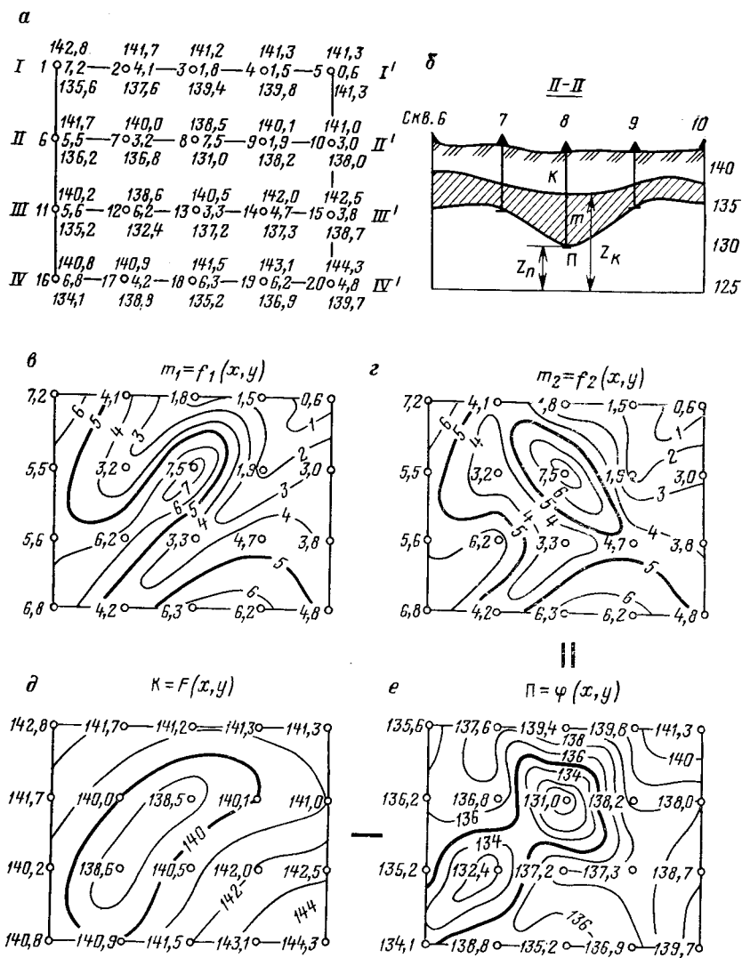
РИС. 8.5. Схема построения изоощностей по комплексу данных разведки: а — план; б — разрез по II—II; в, г — возможные планы изоощностей; д — план поверхности кровли; е — план поверхности почвы залежи
