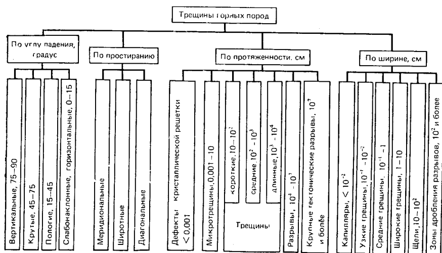
РИС. 11.1. Геометрическая классификация трещин
