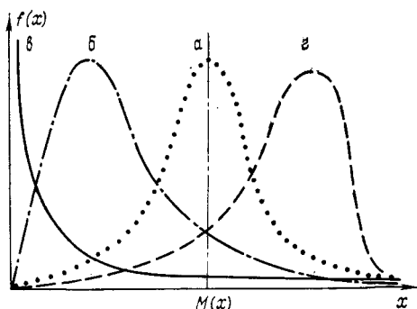
РИС. 3.1. Типы кривых распределения плотности вероятности:
