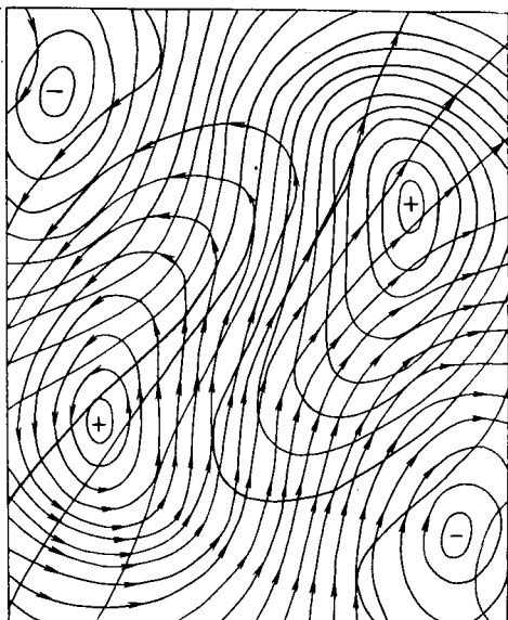
РИС. 13.2. Изображение комплексной топографической поверхности при несовпадении изолиний потенциальной и вихревой поверхности: +источник, —сток
