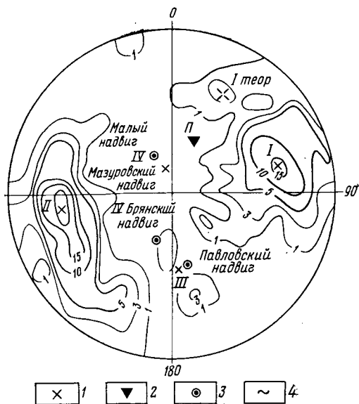
РИС. 11.8. Структурная диаграмма пласта l_5 в восточной лаве на гор. — 70 м:
