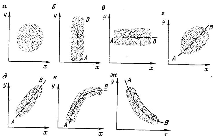
РИС. 3.2. Поле корреляции случайных величин X и Y :
