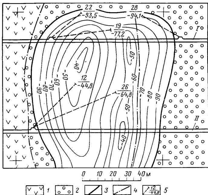
РИС. 14.3. План поверхности в изогипсах кровли рудного тела железорудного месторождения Северного Урала:
