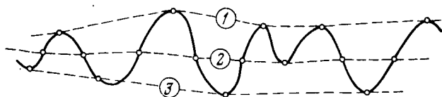
РИС. 3.6. Функция размещения показателя и ее 1, 2, 3 неэргодические реализации
