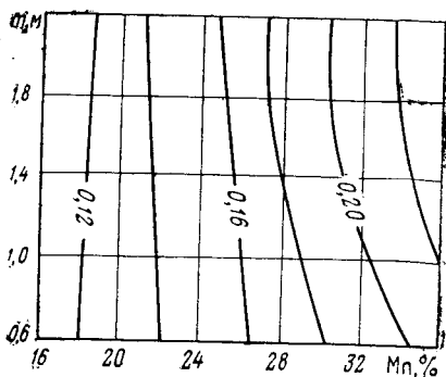
РИС. 15.6. Вид уравнения (15.16) для определения содержания фосфора в руде в зависимости от мощности пласта m (м) и содержания марганца Mn (%)
