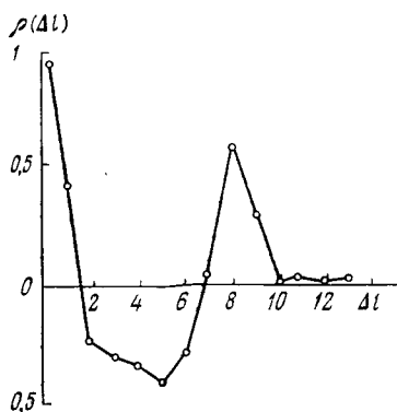
РИС. 3.7. Корреляционная функция по реализации 3, представленной на рис. 3.5
