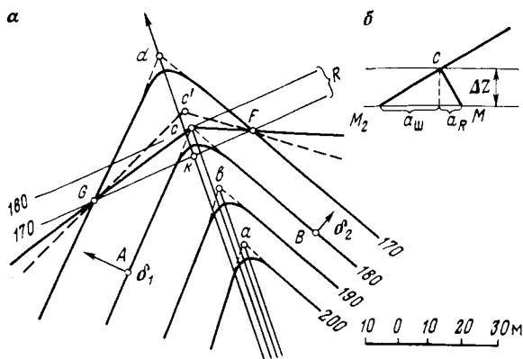
РИС. 9.8. К определению геометрических элементов складки
