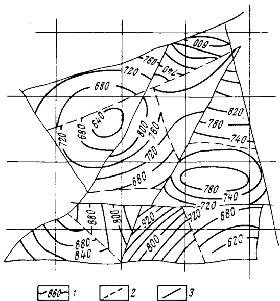
РИС. 13.4. Контуры блоков и тренды поверхности в горизонталях: 1 — горизонталь поверхности тренда блоков; 2 — линии рельефообразующих разломов; 3 — границы блоков по разности гипсометрических уровней
