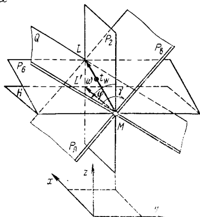
РИС. 10.8. Геометрические элементы скрещения:
