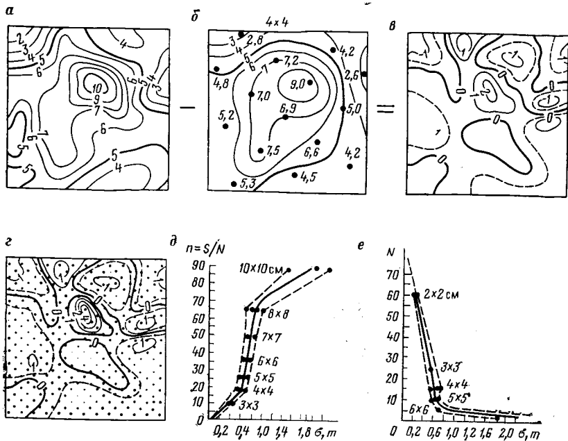
РИС. 7.1. Оценка реализаций топографической функции
