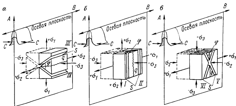
РИС. 9.3. Схема расположения осей пластических деформаций и напряжений при образовании складки, трещин скола и отрыва
