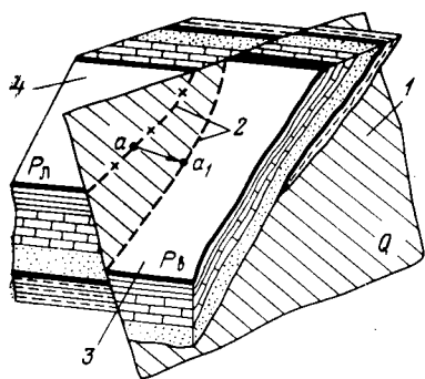
РИС. 10.1. Элементы разрывного нарушения:
