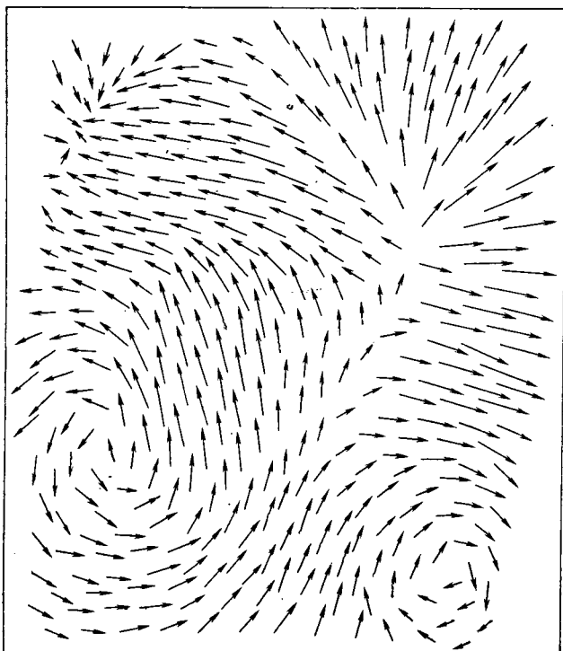
РИС. 13.3. Векторная форма изображения комплексной поверхности, представленной на рис. 13.2
