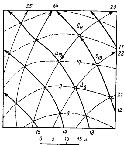
РИС. 4.1. Вычитание двух топографических поверхностей при взаимно пересекающихся изоглиниях
