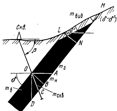
РИС. 5.5. Виды мощности залежи
