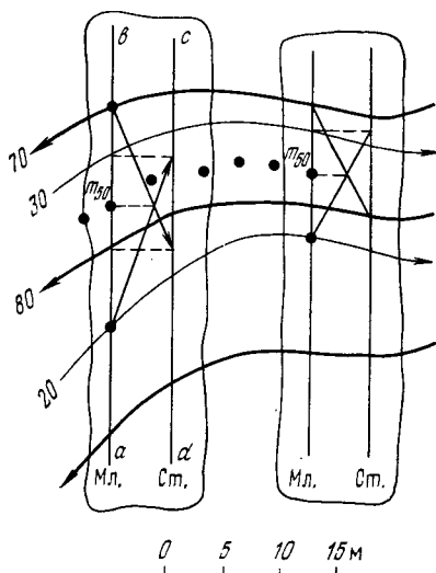
РИС. 4.2. Вычитание топографических поверхностей при непересекающихся изоглиниях
