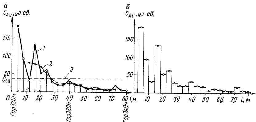
РИС. 12.3. Полигональная (а) и ступенчатая (б) кривые изменения содержания компонента по выработке:
