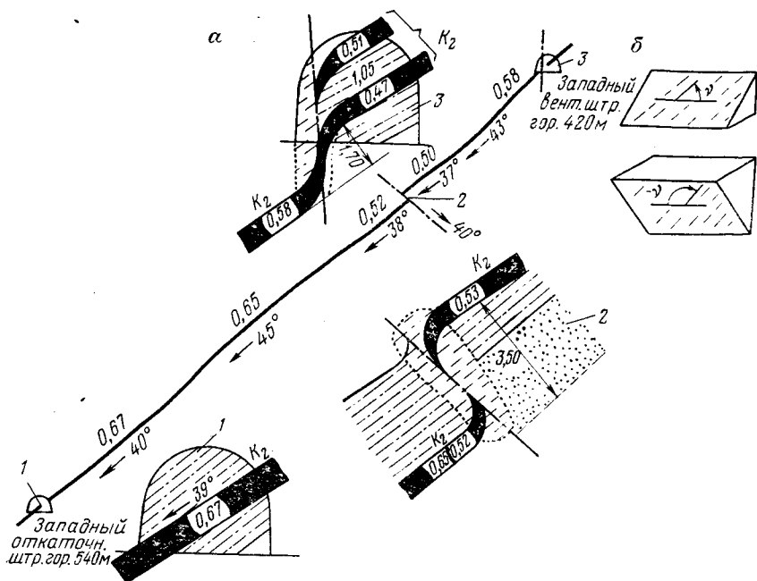
РИС. 10.15. Схема профиля лавы (а), документация нарушений 1, 2, 3, встреченных горными выработками, и измерение направления v перемещения (б)
