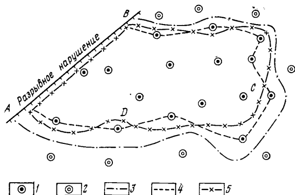
РИС. 17.3. Оконтуривание залежи и балансовых запасов на плане:
