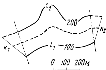
РИС. 17.6. К определению площади поверхности, изображенной в изогипсах
