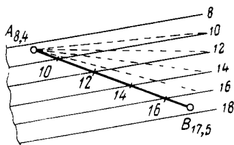
РИС. 2.3. Градуирование прямой с помощью трафарета
