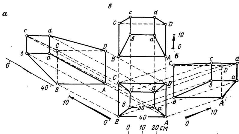
РИС. 2.31. План и векторные проекции усеченной пирамиды
