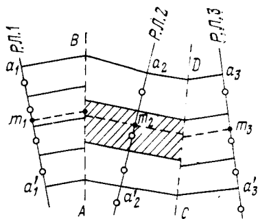
РИС. 18.9. Построение ближайшего района по разведочным линиям россыпного месторождения
