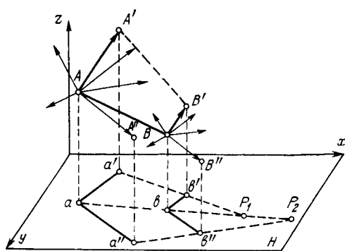
РИС. 2.27. Параллельные векторы точек A и B прямой в пространстве и на плане H
