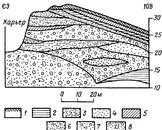
РИС. 14.9. Литологический разрез Тучковского песчано-гравийного месторождения:
