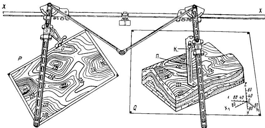
РИС. 2.24. Универсальный аффинограф УА-3
