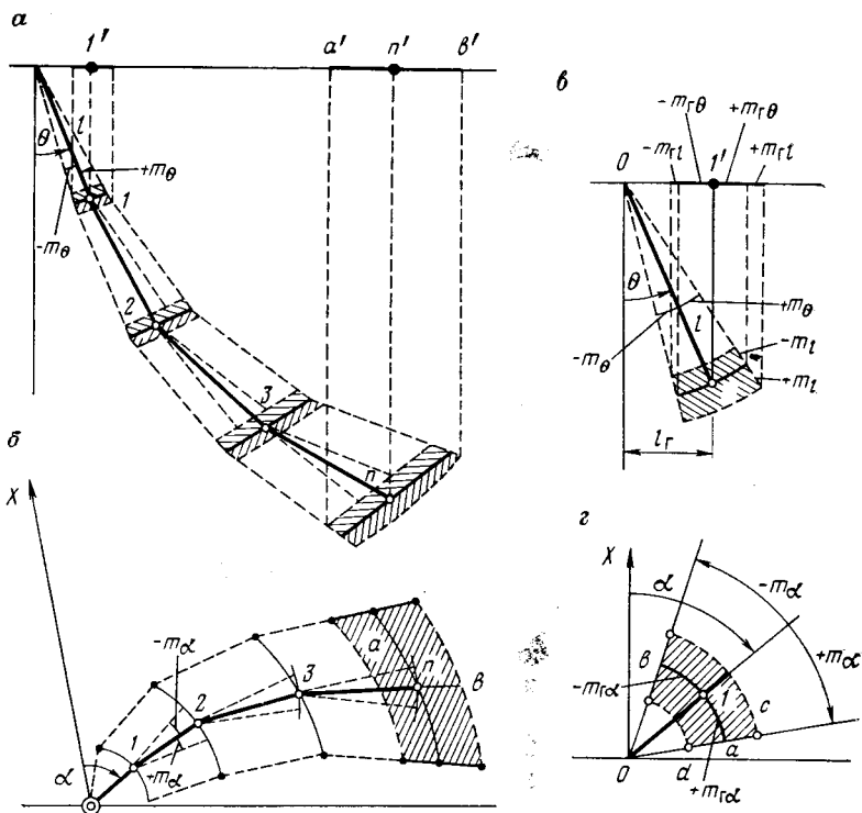
РИС. 5.15. Положения точек оси скважины с учетом погрешности измерений: а и в — в профиле; б и г — в плане
