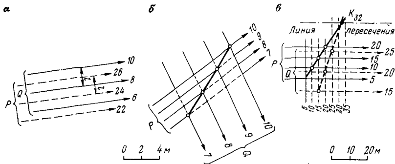
РИС. 2.7. Взаимное положение плоскостей
