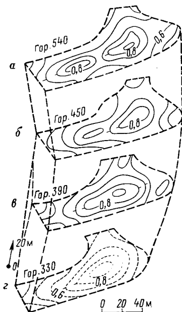
РИС. 14.4. Изолинии содержания компонента по горизонтам штокового месторождения цветных металлов (векторная проекция):
