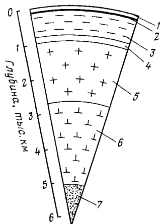
РИС. 9.1. Схема внутреннего строения Земли
