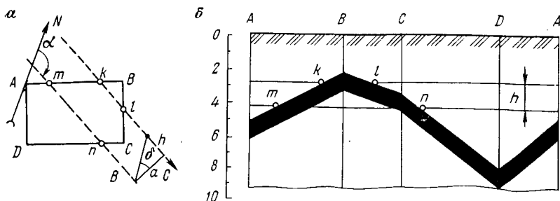
РИС. 5.3. К определению простирания и падения пласта по плану (а) и развертке (б) стенок шурфа
