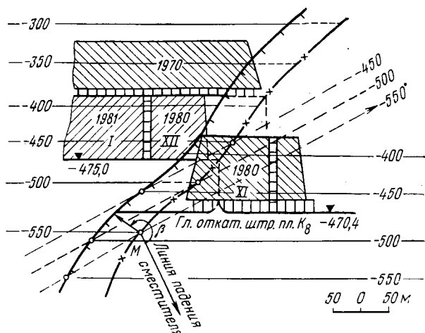
РИС. 10.13. Наименование разрыва по плану горных работ (взброс-пересдвиг с перекрытием)
