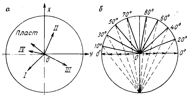
РИС. 11.7. Векторная диаграмма систем трещин (а), масштаб векторов (б)
