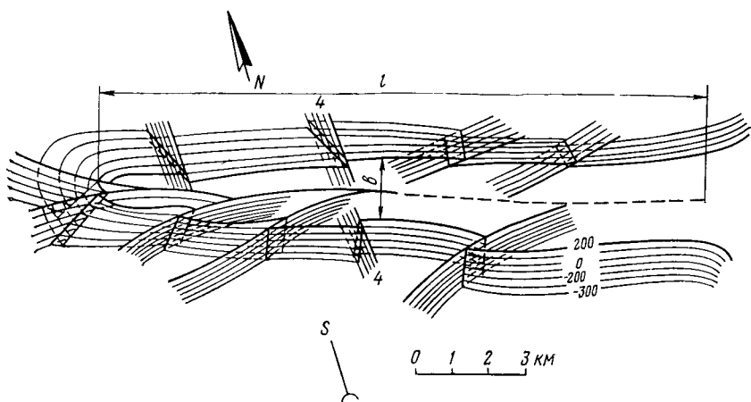
РИС. 9.4. Гипсометрическая карта складки и разрывов
