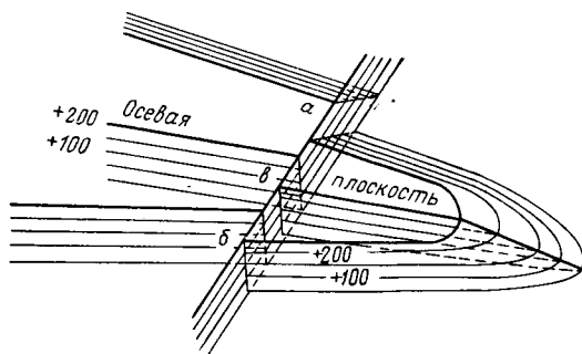
РИС. 10.13. Наименование разрыва по плану горных работ (взброс-пересдвиг с перекрытием)
