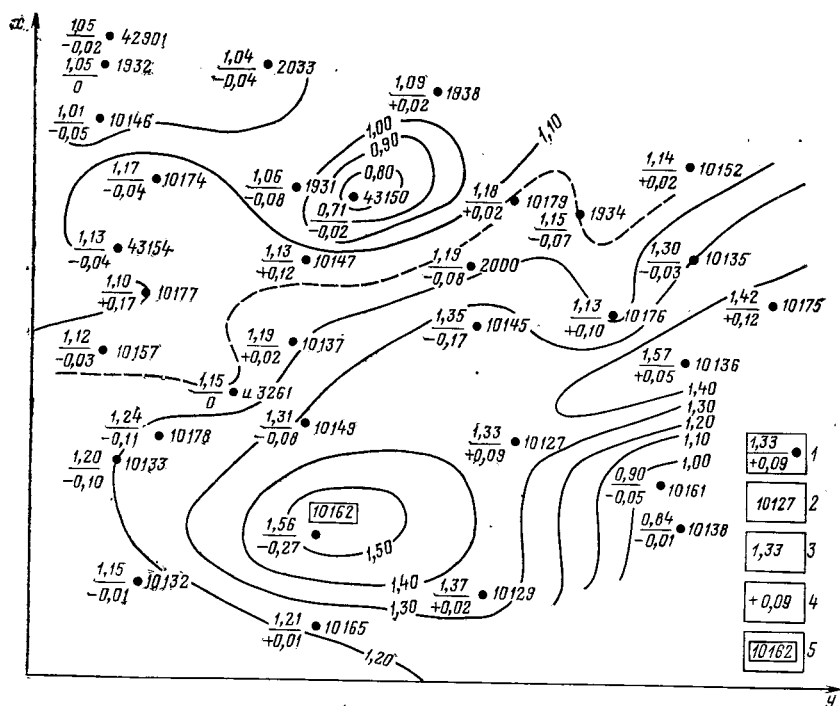
РИС. 15.2. Карта прогноза общей мощности пласта k_6 (шахта Гуковская, Донбасс):
