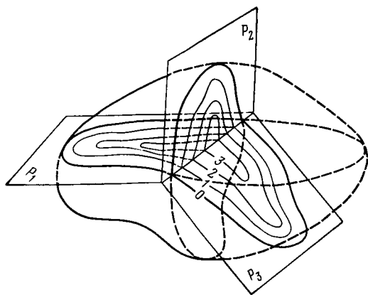
РИС. 1.1. Модель геохимического поля
