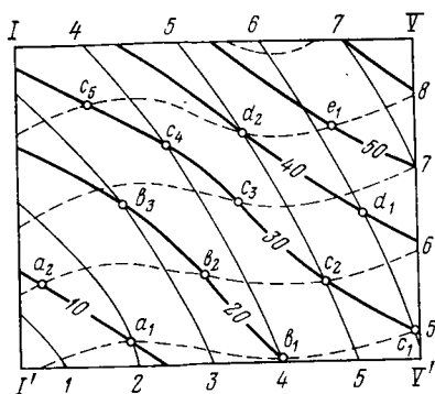
РИС. 4.5. Умножение двух поверхностей
