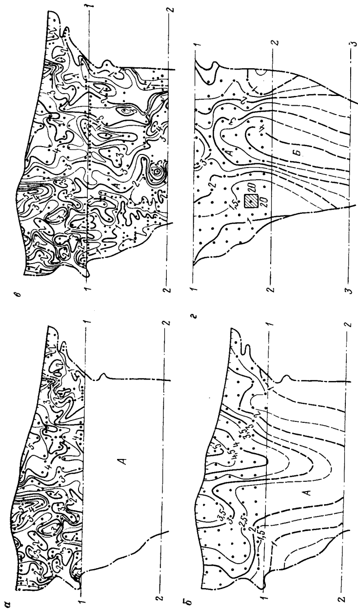
РИС. 15.3. Прогнозирование функции размещения компонента в рудной залежи: а — изолинии по частным пробам; б — сглаженная топофункция и прогноз на участок А; в — изолинии на участке А по частным пробам; г — сглаженная топографическая функция и прогноз на участок В: 1, 2, 3 — горизонты
