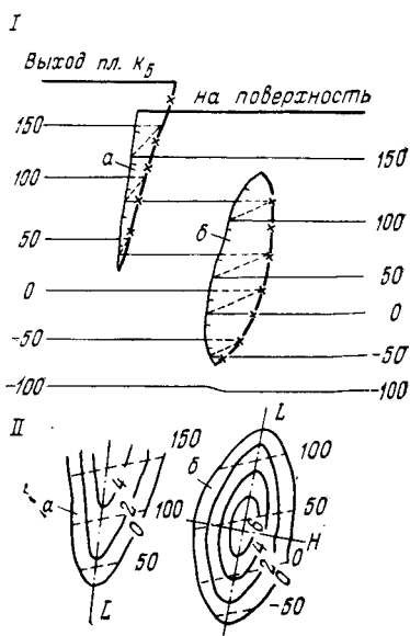
РИС. 10.7. Гипсометрический план пласта k_5 с нарушениями (I) и эпюры сместителей (II)
