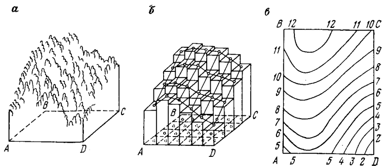
РИС. 1.3. Геометрическая интерпретация размещения оруденения
