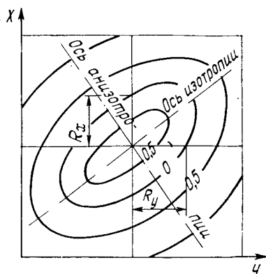
РИС. 12.6. Изокорреляционные коэффициенты автокорреляции
