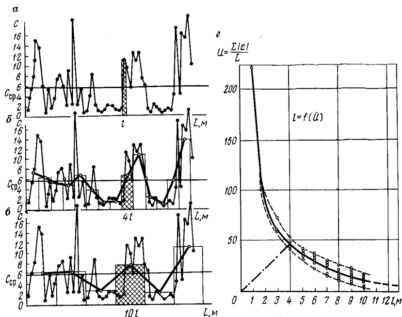
РИС. 3.8. К определению окна сглаживания:
