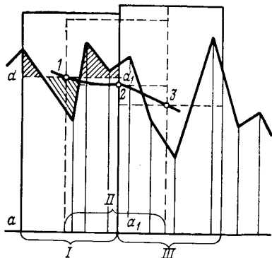
РИС. 12.4. Сглаживание полигональной кривой с помощью статистического «окна»
