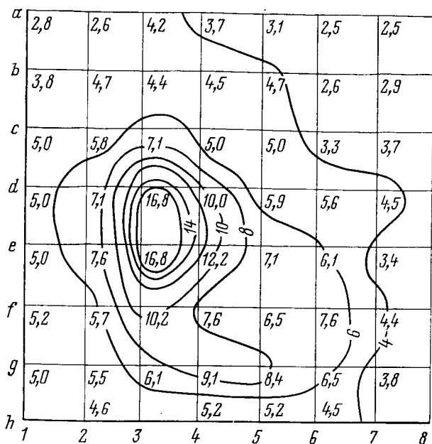
РИС. 4.9. План изогradientов поверхности, представленной на рис. 4.7
