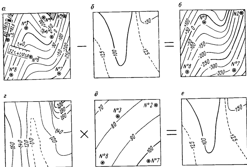
РИС. 9.14. Построение гипсометрического плана малоразведанного пласта k : a — детально разведанная поверхность верхнего пласта l ; б — изолинии вертикальной мощности пород между пластами; в — искомая поверхность пласта k ; г — изосекансы поверхности пласта l ; д — изолинии нормальной мощности пород между пластами; е — изолинии вертикальной мощности пород между пластами l и k
