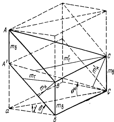
РИС. 9.11. Вертикальные разрезы наклонного пласта:
