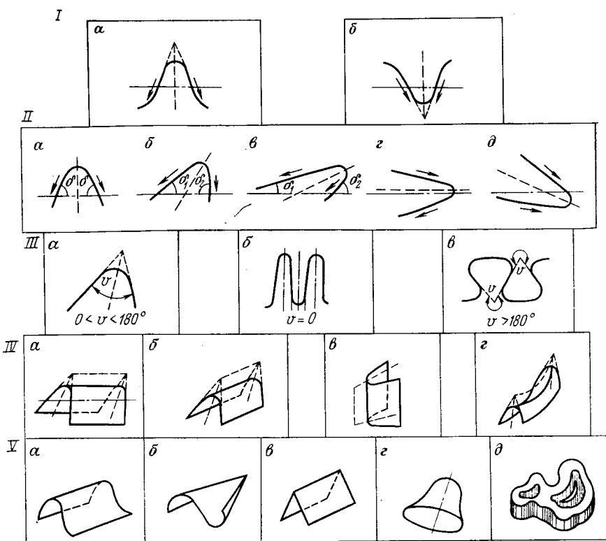
РИС. 9.7. Геометрическая классификация основных форм складок
