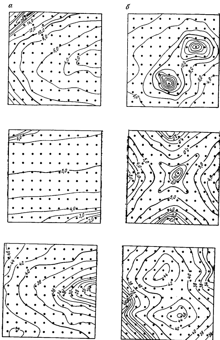
РИС. 6.1. Различные виды размещения показателей (а, б, в) при одинаковых законах распределения: правоасимметричном (I 2 ), нормальном (II 2 ), левоасимметричном (II 2 )
