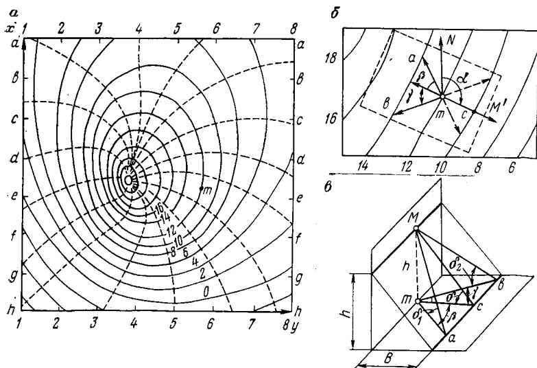
РИС. 4.7. Схема дифференцирования топографической поверхности
