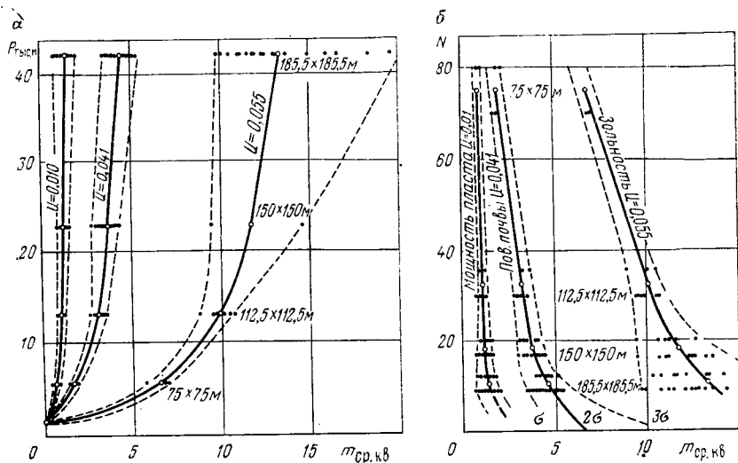
РИС. 7.2. Зависимость между плотностью разведочной сети и точностью реализации при различной изменчивости исходной топографической функции
