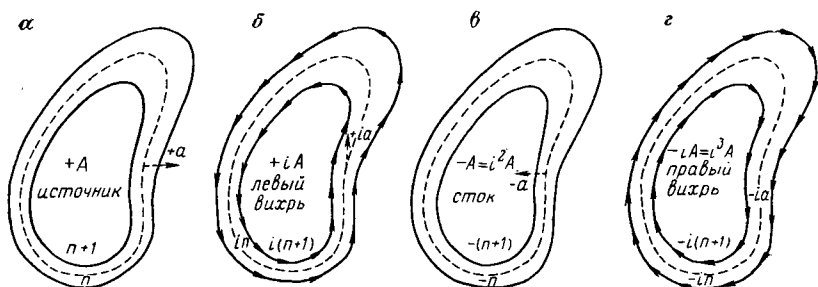
РИС. 13.1. Изображение сечения потока изолиниями
