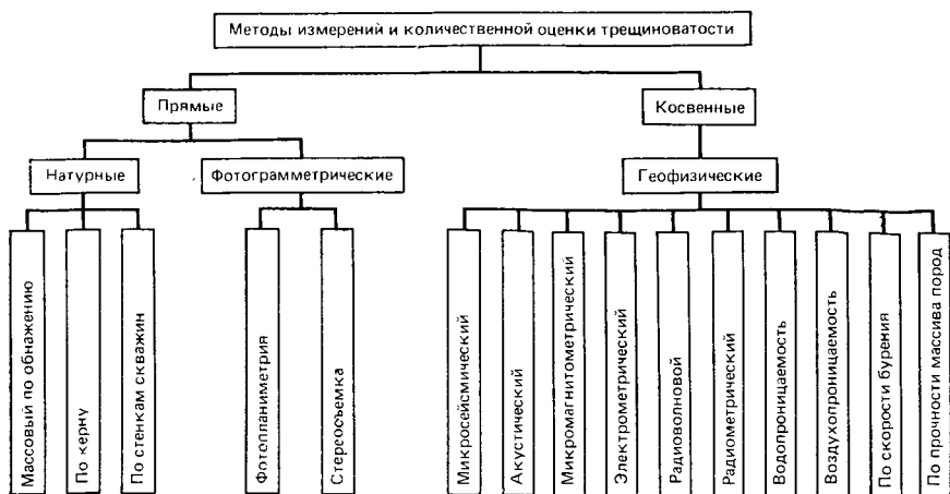
РИС. 11.5. Классификация методов измерения и количественной оценки трещиноватости
