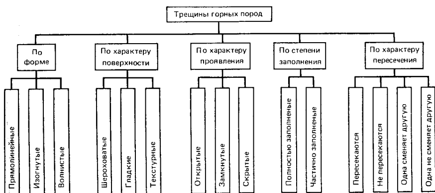
РИС. 11.3. Морфологическая классификация трещин
