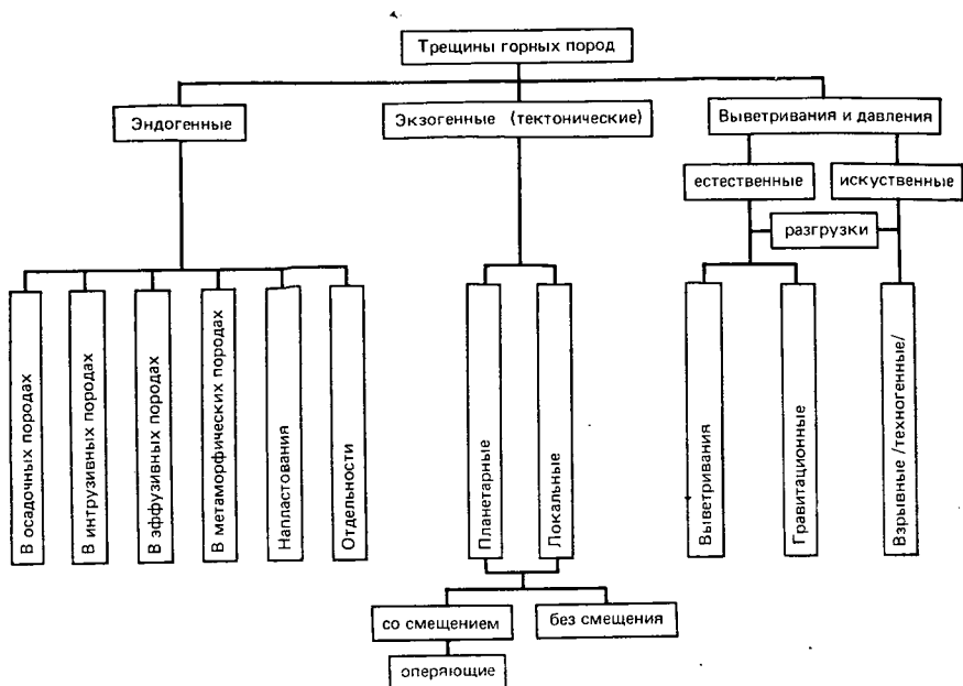
РИС. 11.2. Генетическая классификация трещин
