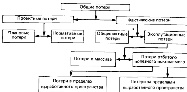
РИС. 20.4. Классификация потерь полезных ископаемых
