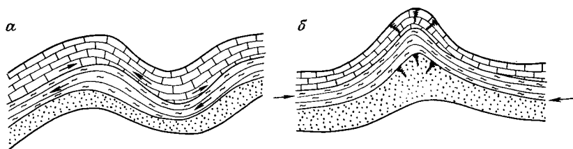
РИС. 9.5. Схема образования складок
