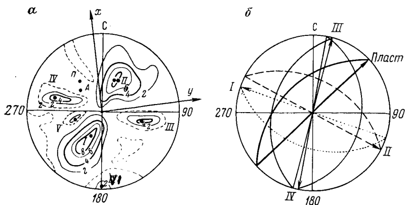
РИС. 11.6. Круговые диаграммы трещиноватости:
