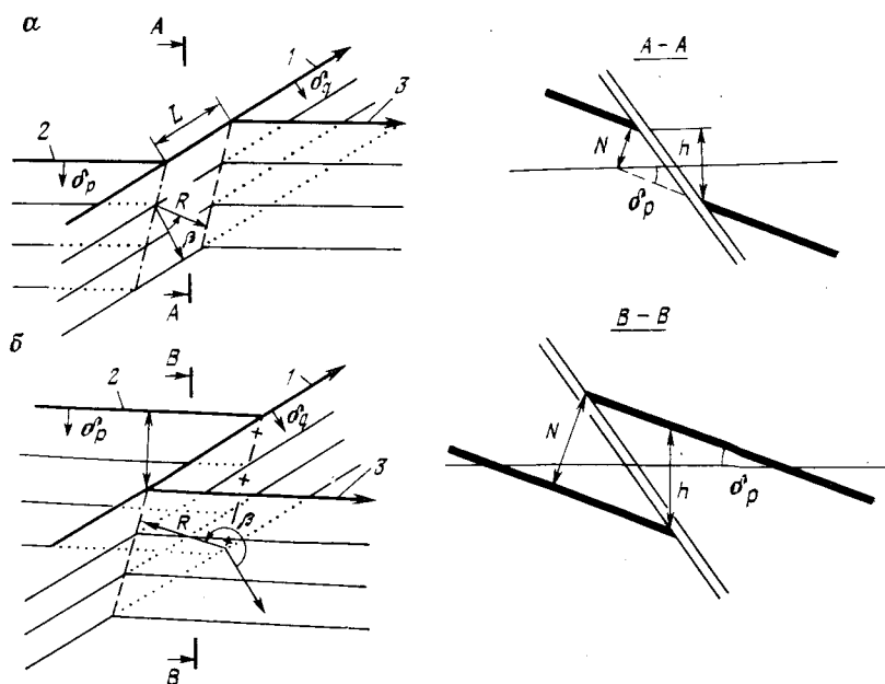
РИС. 10.6. Виды амплитуд смещения: а — с зиянием; б — с перекрытием крыльев
