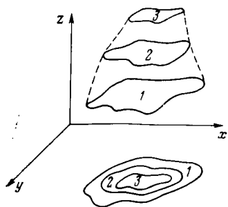
РИС. 1.5. Графическая и аналитическая модель параметра залежи:
