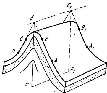
РИС. 9.6. Геометрические элементы складки
