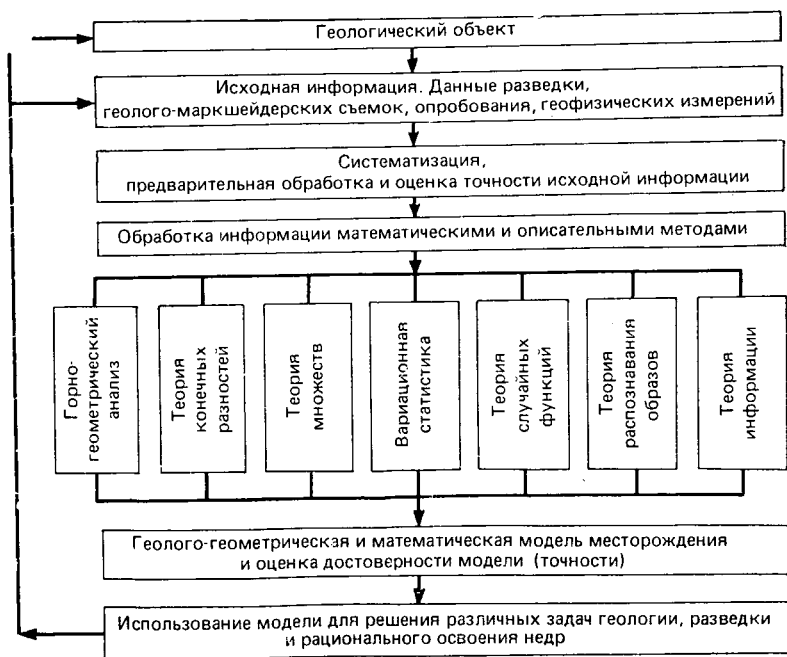
РИС. 1.4. Общая схема геометризации
