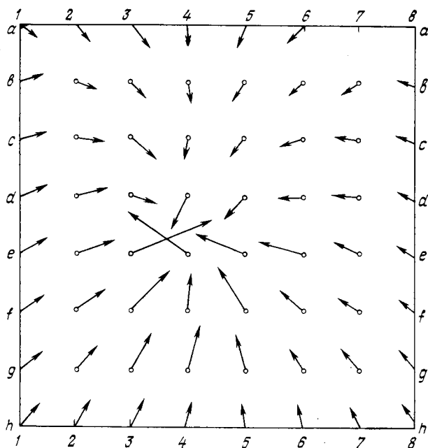
РИС. 4.8. План векторно-градиентного поля поверхности, изображенной на рис. 4.7
