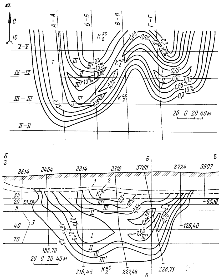
РИС. 16.1. Распределение типов руд (показано в разрезе): а — план; б — разрез
