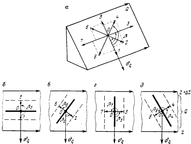
РИС. 10.9. Типовые смещения по П. К. Соболевскому
