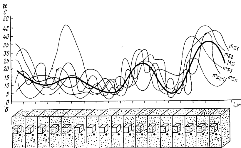
РИС. 3.4. Геометрическое выражение размещения минерализации на участке залежи:
