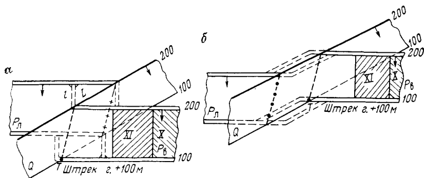
РИС. 10.18. Возможные положения и задание выработок на смещенное крыло P_d при перекрытии (а) и зиянии (б) крыльев
