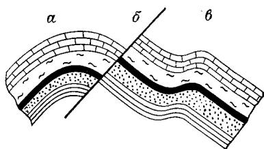
РИС. 9.2. Нарушения в залегании свиты пластов
