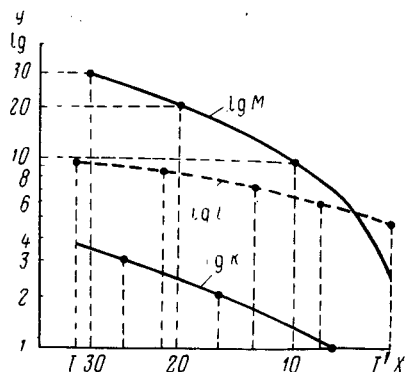
РИС. 4.6. Построение логарифмических кривых по линии I—I' (рис. 4.5)
