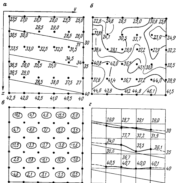
РИС. 12.5. Сглаживание по площади:
