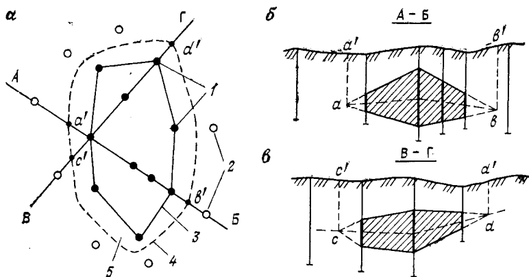
РИС. 17.1. Построение внешнего контура на плане ( \alpha ) и разрезах ( \delta, \nu ) с учетом морфологии залежи:
