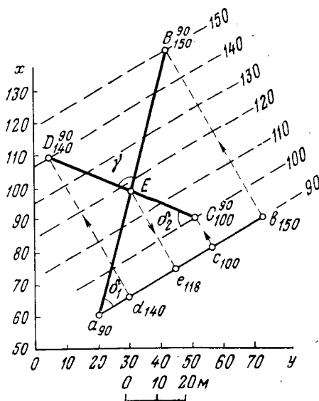
РИС. 2.9. Схема перемены плоскости проекции
