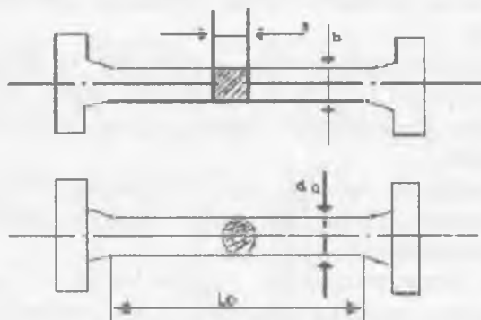
6.7-rasm. Tajriba uchun ishlatiladigan namunalarning sxematik tuzilishi
