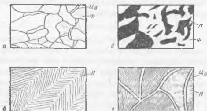
8.8-rasm. Po‘lat mikrostrukturasi (tarkibdagi uglerodning protsent miqdori a=0. 01, b=0. 4, v=0. 8, g=1.3).
