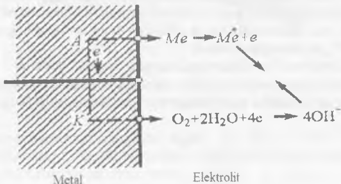
11.2-rasm. Korroziyon element sxemasi
