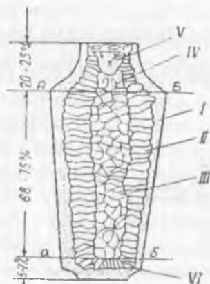
4. 9 –rasm. Po'lat quymaning tuzilish sxemasi.
