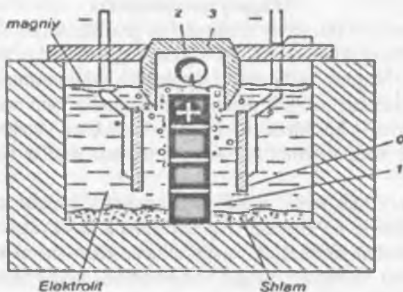
13.5-rasm. Mayniy xloridni elektroliz qilish vannasi sektsiyasining sxemasi. 1-anod; 2-katod plastinkasi; 3-to‘siq; 4-xlorni chiqarish trubasi.
