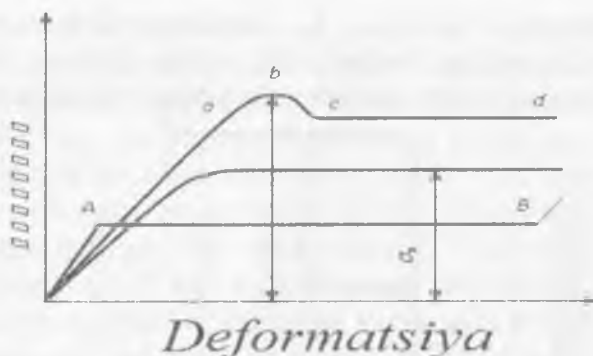
16. 3-rasm. Shishasimon (yuqori va pastdagi) hamda kristall strukturali (oʻrtadagi) polimerlarning “deformatsiya- kuchlanish” grafigi.
