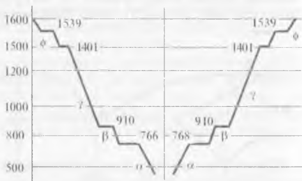
5. 7-rasm Temirning sovish va erish grafigi.
