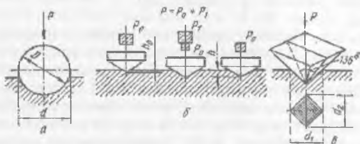
6. 10-rasm. Qattqlikni o'lchash: a) Brinel usuli b) Rokvell usuli v) Vikkers usuli
