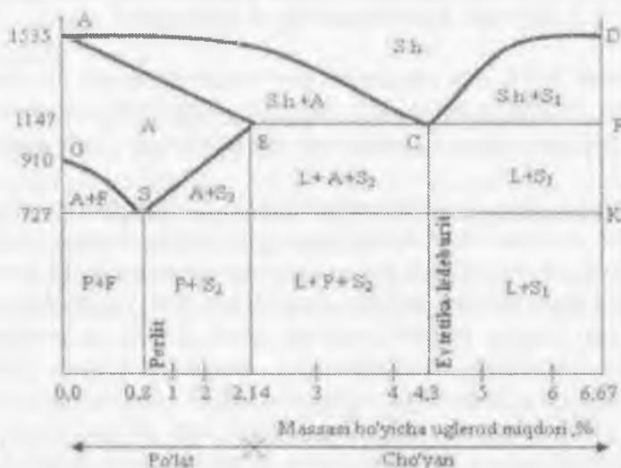
Temir-uglerod qotishmalarining holat diagrammasi
