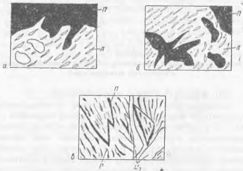
8.10-rasm. a-evtektigacha: b-evtektik: v-evtektikadan keying cho'yan strukturalari.
