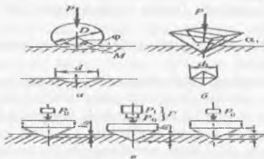
7.4-rasm. Qattiqlikni sinash usullari sxemalari. a-Brinell usuli, b-Vickers usuli, v-Rokvell usuli.
