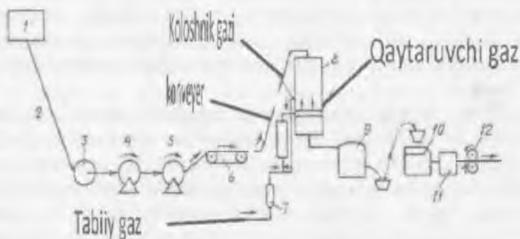
Temir rudalaridan po'latlarni do'imiy olish usulining texnologik shemasi
