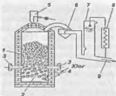
13.6-rasm. Rutii briketlariga xlor bilan ishlov berish qurilmasining sxemasi. 1-rutil briketlari; 2-qarshilik elementlari; 3-elektrodlar; 4-trubka; 5-bunker; 6-chang yutgich; 7-kondensat; 8-sovutgich(chapda).
