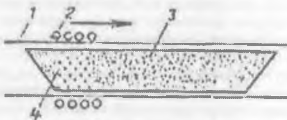
13.2-rasm. Zonalik qayta kristall sxemasi; 1-kvars tuba; 2-qizdirgichlar; 3- grafit yoki kvardsdan yasalgan qayiqcha(idish); 4-erish zonasi.
