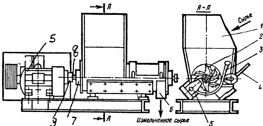
6.7-rasm. MGKM – markali muzlagan go'sht mahsulotlarini kesuvchi uskuna.
