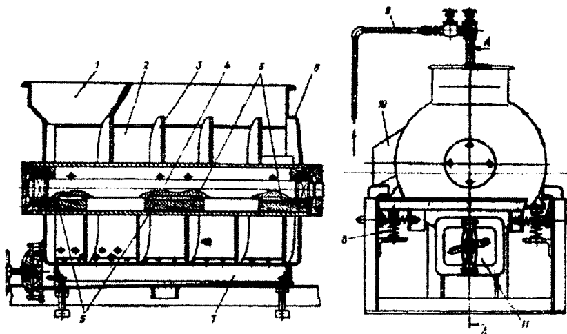
2.1-rasm. Tebranma harakat qiladigan YUMB-2000 markali sabzovot mahsulotlarini yuvuvchi jihoz.
