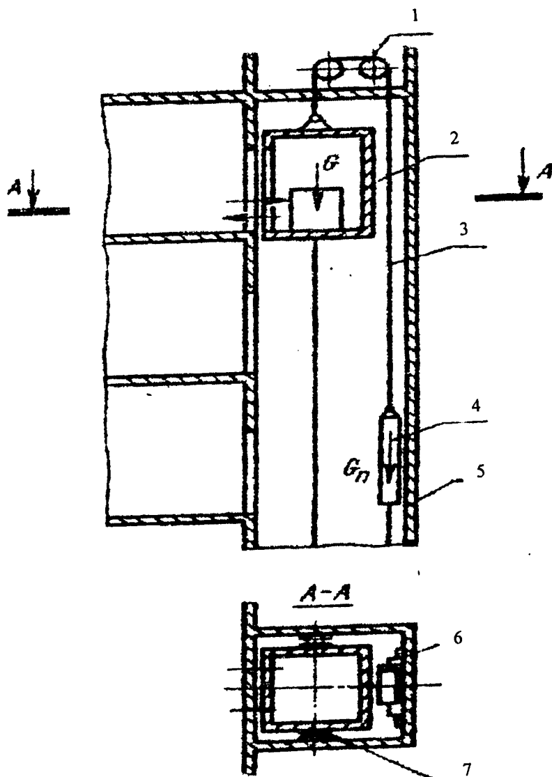
11.22-rasm. Liftning printsipl chizmasi.
