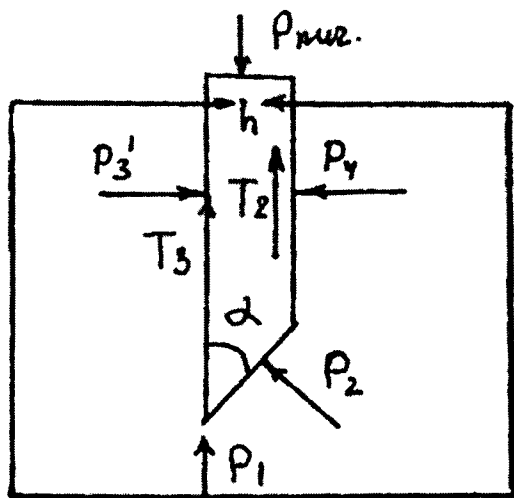
5.6-rasm. Mahsulotlarni egmasdan kesayotgan paytidagi pichoqlarga ta'sir qiluvchi kuchlar chizmasi.
