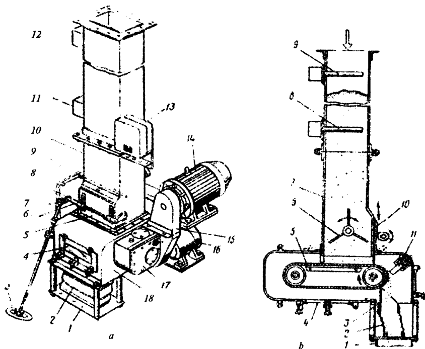
8.7-rasm. Tasmali o'lchagich uzluksiz ishlangan: a) umumiy ko'rinishi; b) ishlash chizmasi.
