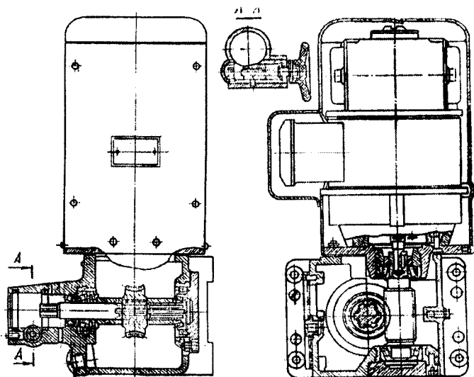
1.5-rasm. XUM-o'zg va XUM-o'xgr. markali harakat uzatuvchi moslama.
