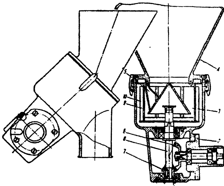
4.1-rasm. MEM-XB-1 markali mahsulotlarni elovchi jihoz.
