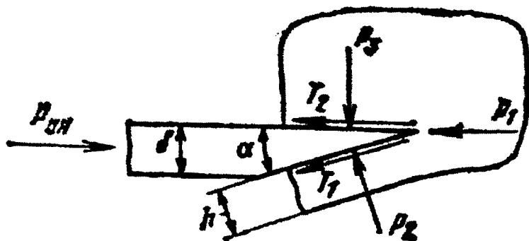
5.5-rasm. Pichoq kesiladigan mahsulotning ichiga kirib boraverishda unga qarshiliklar chizmasi.
