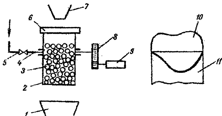
3.3-rasm. VNIITORMASHning sabzovotlarni tozalovchi agregati 1-oluvchi bunker; 2-aylanuvchi ish kamerasi; 3-mahsulot; 4-bug' berish sistemi; 5-ochiluvchi moslama; 8-tishli g'ildirak; 9-xarakat beruvchi moslama; 10-tozalash; 11-kamera.
