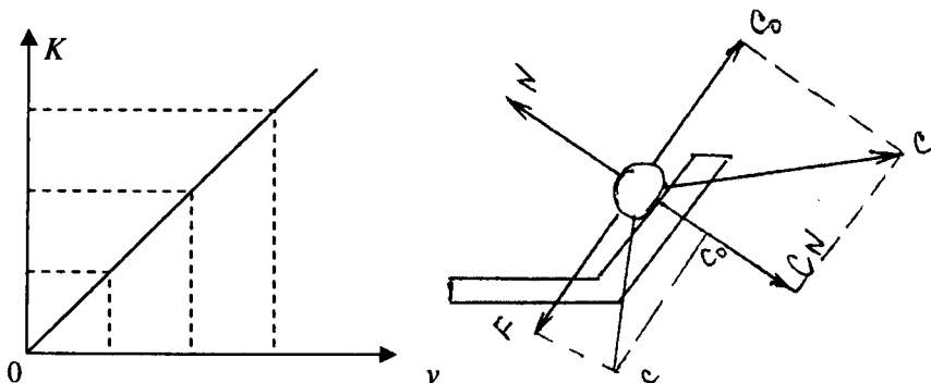
3.12-rasm. Tozalash uskunalar tezligining o'zgarishi bilan ishqalanish koeffitsientining o'zgarishini ko'rsatuvchi chizma.
