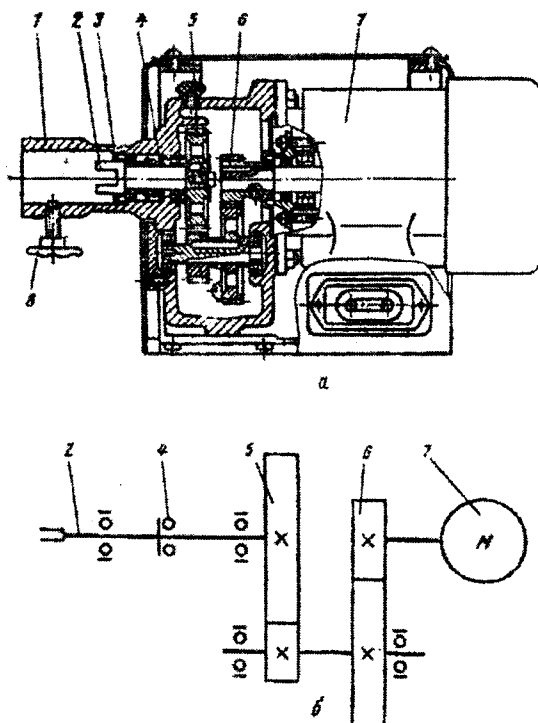
1.3-rasm. XUM - 0,6 1.1. Markali harakat yzatuvtchi moslama.
