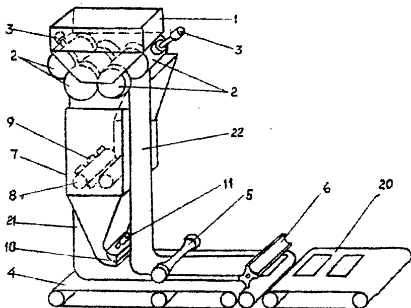
9.9-rasm. Ichida masallig'i bor mahsulotlarga shakl beruvchi jihoz.
