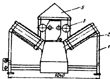
4.9-rasm. O'lchamiga qarab ajratuvchi mashina:
