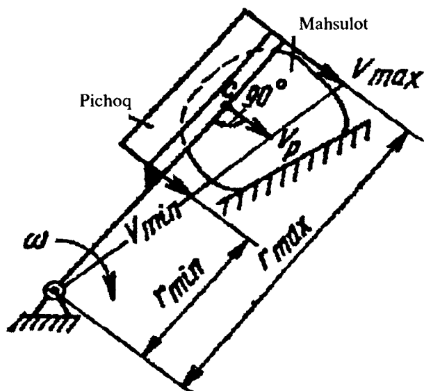
5.8-rasm. Pichoqlarni mahsulotlarning chopish jarayonlarida ularga nisbatan harakat chizmasi.
