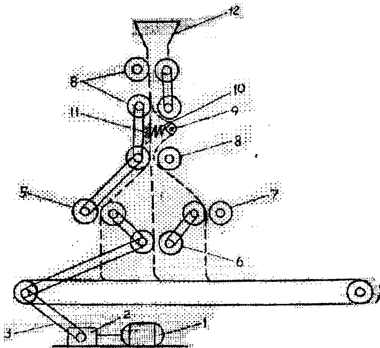
9.7-rasm. Ko'p g'o'lachali xamir mahsulotlariga shakl beruvchi jihozning chizmasi:
