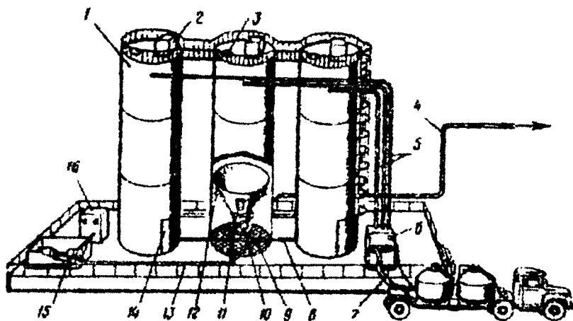
7.2-rasm. Ochiq yuzada unni saqlash va tashishning texnologik liniyasi.
