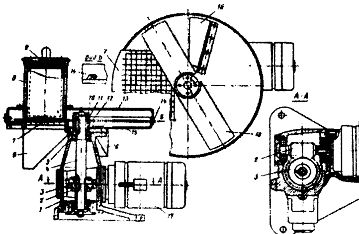
5.16-rasm. CKM-160 markali pishgan sabzavot mahsulotlarini kesuvchi jihoz.
