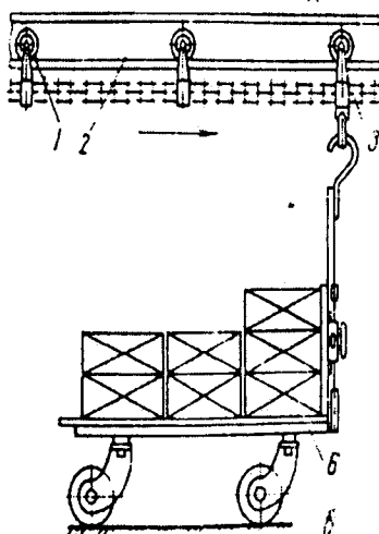
11.29-rasm. Osma konveyerning chizmasi.
