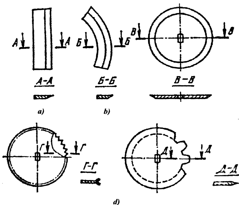
5.1-rasm. Pichoqlarni turlari:
