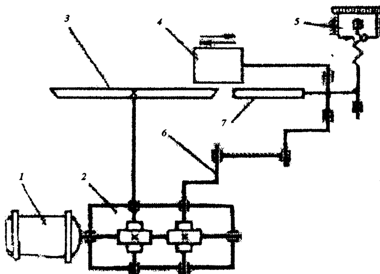
6.10-rasm. GMKM-300A markali uskunani harakat yo'lini ko'rsatuvchi chizmasi.
