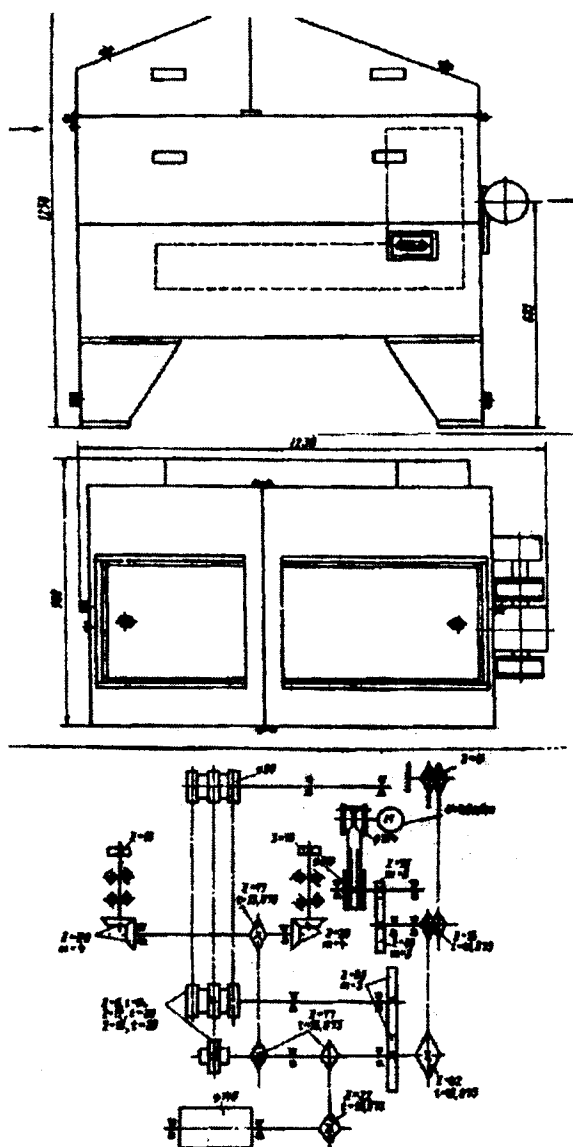
7.22-rasm. Karamel qoliplovchi mashinaning umumiy ko'rinishi va kinematik chizmasi.
