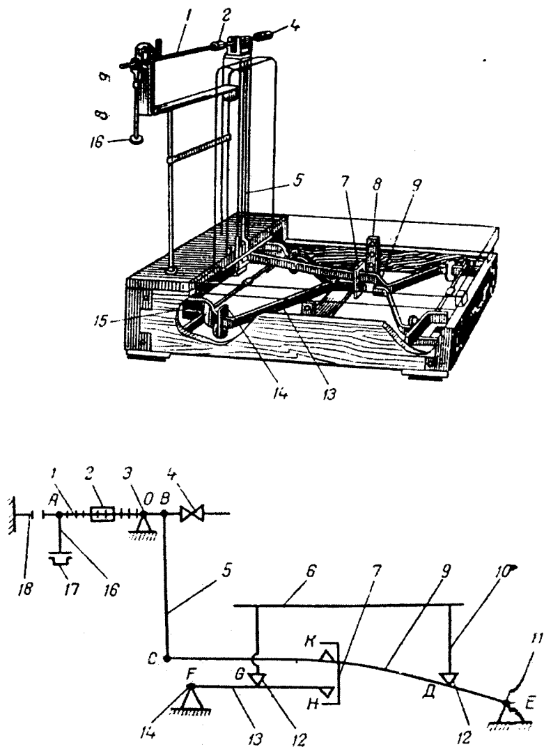
10. 10-rasm. Platformasi siljiydigan tarozining umumiy ko'rinishi va kinematik chizmasi.
