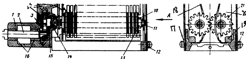
6.4-rasm. GBM-15 markali go'sht mahsulotlarini bo'shatuvchi jihaz.
