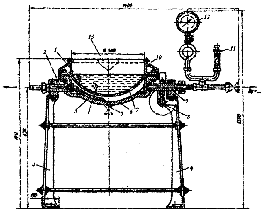
7.19-rasm. Qaynatish qozonining umumiy ko'rinishi.
