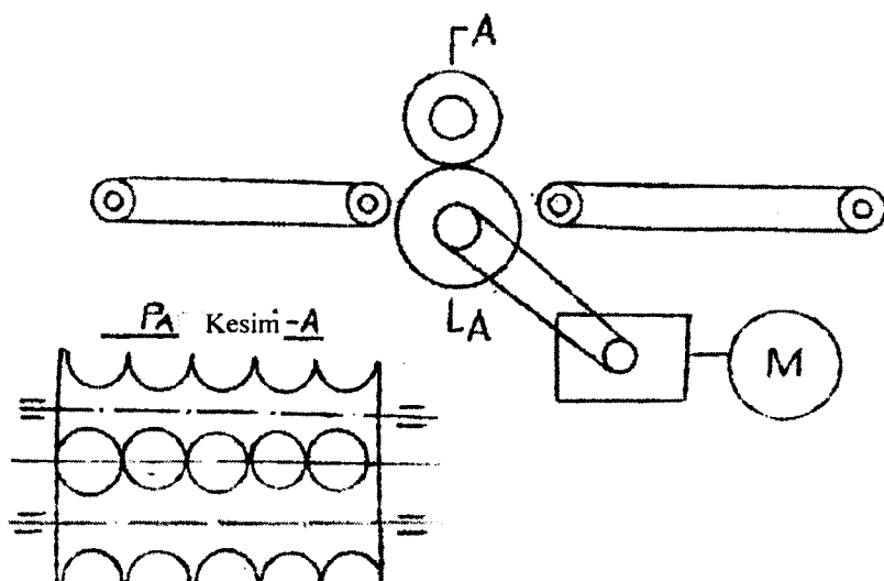
9.11-rasm. Qandolat tayoqchalariga shakl beruvchi jihoz.
