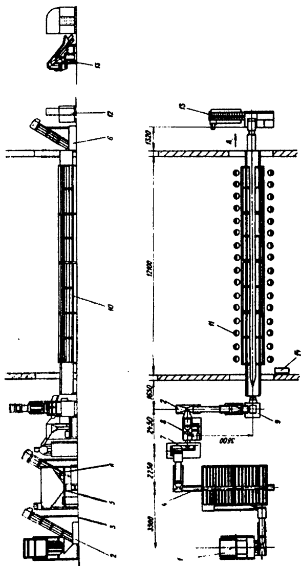
4.10-rasm. Texnologik liniyaning umumiy ko'rinishi: 1—konteyner to'rtaruvchi; 2—qabul qiluvchi; 3—taqsimlovchi; 4—tasmali qabul qiluvchi; 5—mahsulot soluvchi moslama; 6—qiya ortuvchi; 7—yuvish mashinasi; 8—tosh ushlovchi; 9—tozalovchi mashina; 10—qayta tozalaydigan konveyer; 11— boshqaruvchi stol; 12—sulfitlevchi mashina; 13—avtomat tarozi; 14-boshqaruv pulti.
