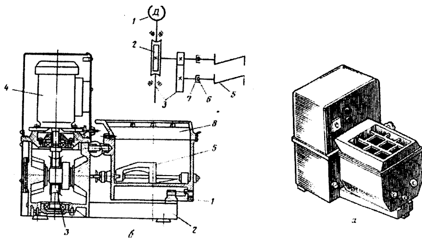
7.11-rasm. XQM-15 markali xamir qoruvchi uskuna.
