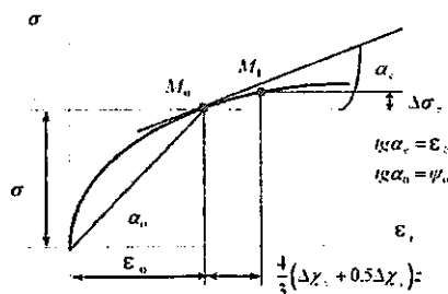
5.2-chizma. Urinma va kesuvchi modulni aniqlash diagrammasi.
