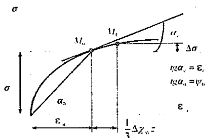
5.4-chizma. Urinma va kesirvchi modullarni aniqlash diagrammasi.
