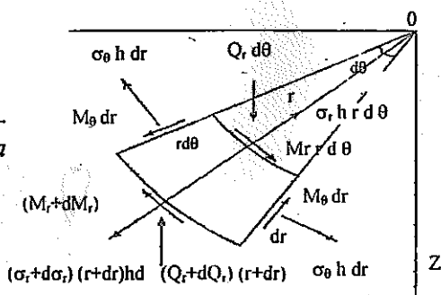
4.4-chizma. Plastinka deformatsiyalangan elementiga qo'yilgan zo'riqlar.
