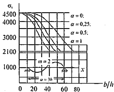
5.18-uzama. a/h = 3 ; m = 2 miqdorlarda deformatsiya intensivligi bilan nisbiy qalinlik orasidagi bog'lanish grafiklari
