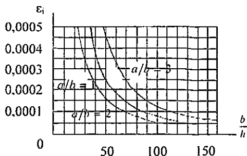
5.6-chizma. Deformatsiya intensivligining nisbiy qalinlikka nisbatan o'zgarish grafigi.
