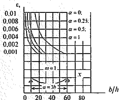
5.17-chizma. a/h = 3 ; m = 1 miqdorlarda deformatsiya intensivligi bilan, nisbiy qalinlik orasidagi bog'lanish grafigi
