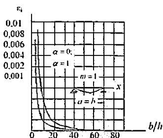
5.23-chizma. Materiali chiziqli puxatlanishga bo'ysimuvchi kvadrat plastinka uchun \varepsilon , bilan nisbiy qalinlik orasidagi bog'lanish grafiqi ( \alpha = 0, \alpha = 1 )
