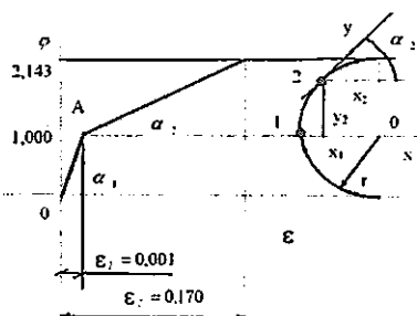
3.12-chizma. Qiya to'g'ri chiziqning silliq o'tish grafifi.
