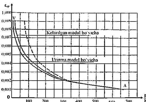
6.6-chizma. Ikki yo'nalish bo'yicha to'liqlarning hosil bo'lishida kritik deformatsiyaning qobiq nisbiy qalinligiga bog'liqlik grafigi.
