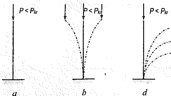
1.2-chizma. Sterjenning muvozanat holatlari.
