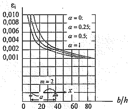
5.11-chizma. a/b=1 ; m=2 miqdorlarda deformatsiya intensivligi bilan, nisbiy qalinlik orasidagi bog'lanish grafigi.
