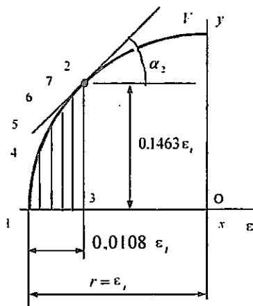
3.13-chizma. O'tish yoyi.
