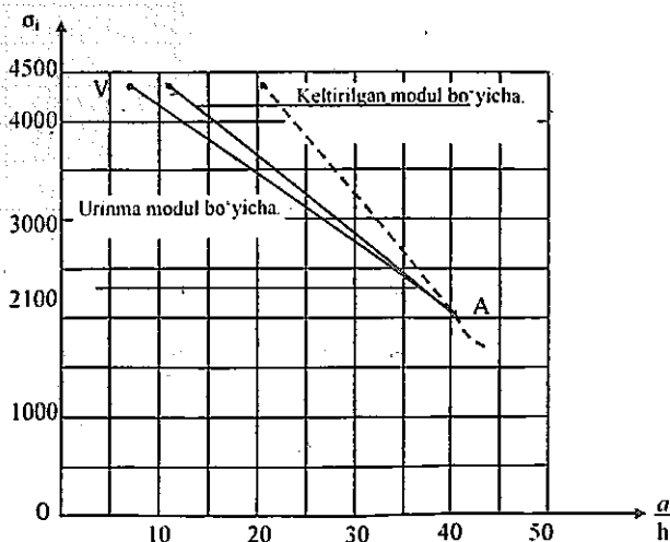
4.6-chizma. Qistirib mahkamlangan plastinka radiusining qalinligiga nisbatidan kritik kuchlanishning o'zgarish grafigi.
