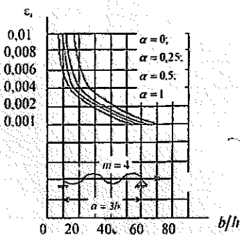
5.21-чизма. a/h=3 ; m=4 miqdorlarda deformatsiya intensivligi bilan, nisbiy qalinlik orasidagi bog'lanish grafiklari
