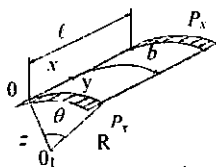
6.7-chizma. Bo'ylama siqilgan silindrik panel.
