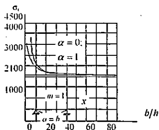
5.22-chizma. Materiali chiziqli puxatlanishga bo'ysimuvchi kvadrat plastinka uchun \sigma , bilan nisbiy qalinlik orasidagi bog'lanish grafiqi ( \alpha = 0, \alpha = 1 )
