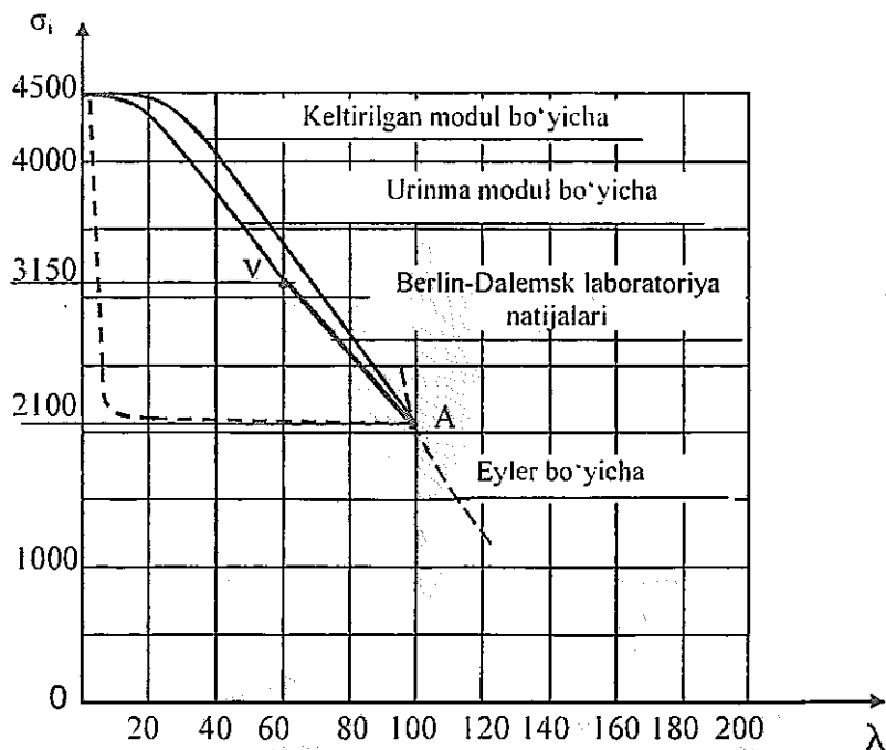
3.16-chizma. Qurilish po'lati uchun kritik kuchlanishning egiluvchanlikka bog'liqlik grafigi.
