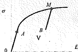
3.1-chizma. Materialning siqilish diagrammasi.
