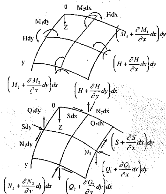
6.1-chizma. Qobiqning o'rtasiga ta'sir etuvchi zo'rliqlar.
