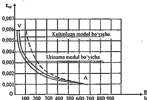
6.5- chizma. O'qqa simmetrik to'lqin hosil bo'lganda kritik deformatsiyaning qobiq nisbiy qalinligiga bog'liqlik grafigi.
