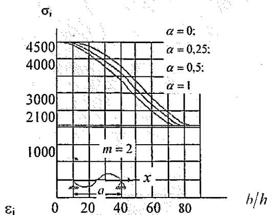
5.10-chizma. a/b=1 ; m=2 miqdorlarda kuchlanish intensivligi bilan, nisbiy qalinlik orasidagi bog'lanish grafigi.
