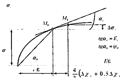
5.3-chizma. Urinma va kesuvchi modulni aniqlash diagrammasi.
