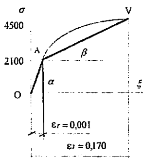
3.10-chizma. Qurilish po'lati materialining cho'zilish - siqilish diagrammasi.
