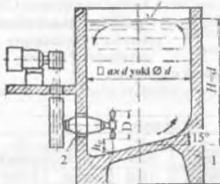
3.8-rasm. Vertikal mashina havzasi: 1 – havza; 2 – parrakli aralashtiruvchi qurilma
