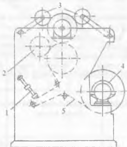
10.13-rasm. Babinaga o'ralgan polotnnoni qirqish dastgohining sxemasi.
