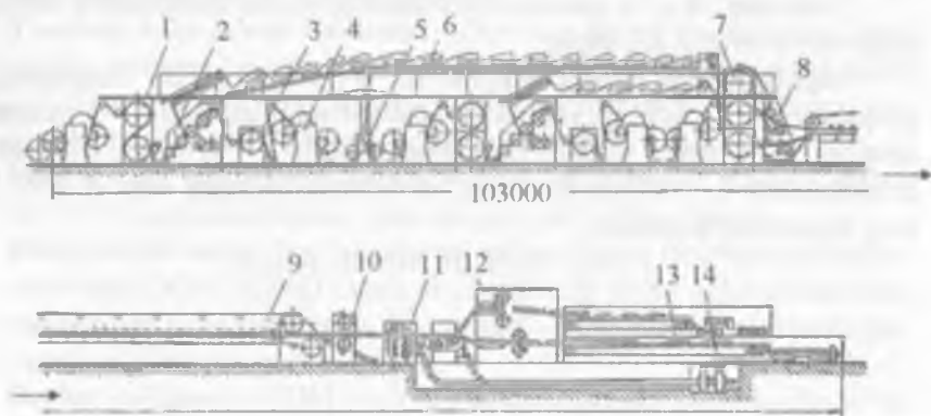
11.1-rasm. АФП2с-3Б rusumli gofrlash agregatining sxemasi:
