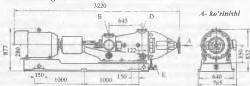
2.16-rasm. MKЛ-01М rusumli konussimon tegirmon va uning gabarit o'lchamlari.
