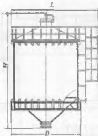
3.3-rasm. Suyultirilgan kimyoviy critmalar saqlaydigan bak.
