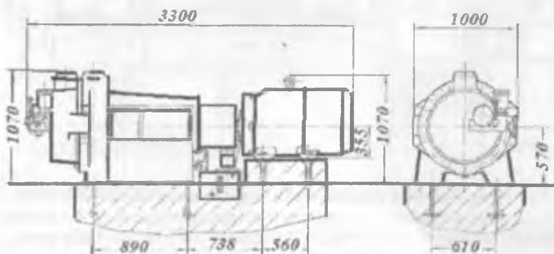
2.12-rasm. M/D-14-1 rusumli diskli tegirmonning umumiy ko'rinishi va o'lchamlari chizmasi.
