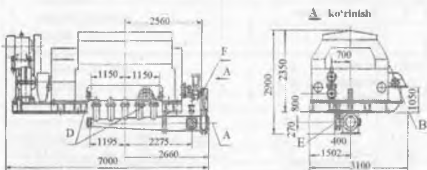
5.5-rasm. C2B-16 ikki barabanli quyultirgichning gabarit chizmasi.
