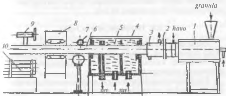
9-rasm. Polietilen quvurlar olish texnologik jarayoni:
