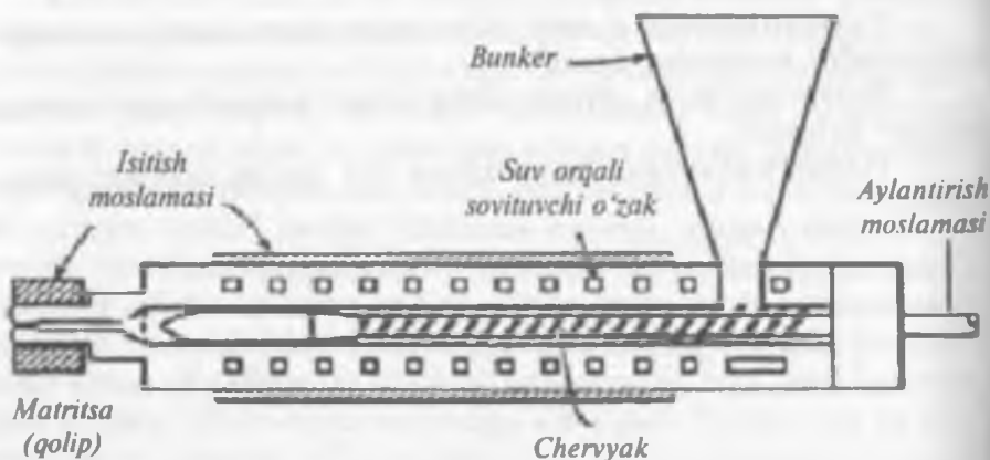
3-rasm. Ekstruder sxemasi.
