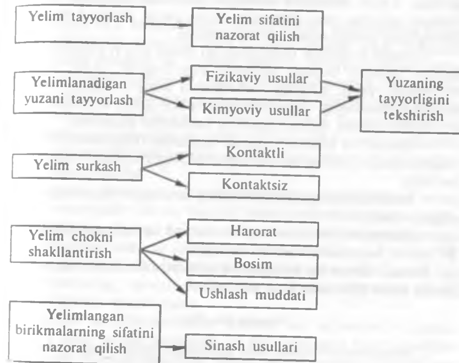
Yelimlash namunaviy texnologik sxemasi
