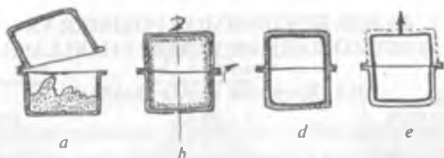
19-rasm. Rotatsion shakllash operatsiyalari:
