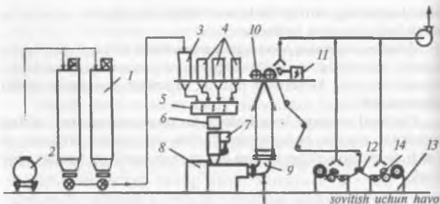
8-rasm. Polietilen plyonka ishlab chiqarish texnologik sxemasi:
