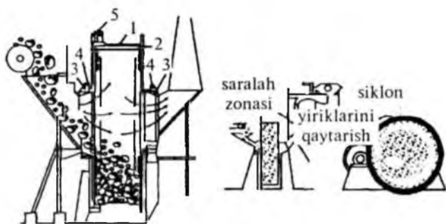
19-rasm. Maydalovchi jinslarsiz «Aerofol» barabanli tegirmon: 1 – baraban; 2 – baraban tubi; 3 – sapfalar; 4 – podshipniklar; 5 – gardishli shesterna.
