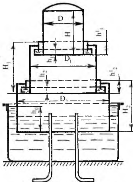
13-rasm. Ho'l tipdagi gazgolder.
