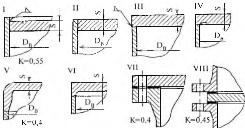
4-rasm. Obechaykalar yassi (tekis) tublarni birlashtirish varianti va tub konstruksiyasi koeffitsienti K ning ahamiyati.
