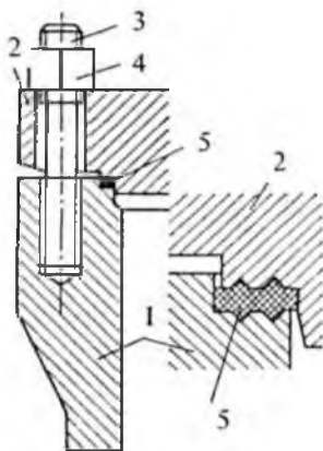
5-rasm. Plastik tekis obtyurator bilan majburiy zichlovchl boltli zatvor:
