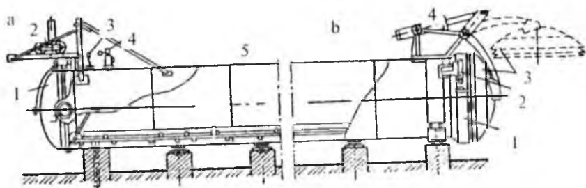
16-rasm. Diametri 2 va uzunligi 19 m o'lchamli o'tkazuvchi avtoklav:
