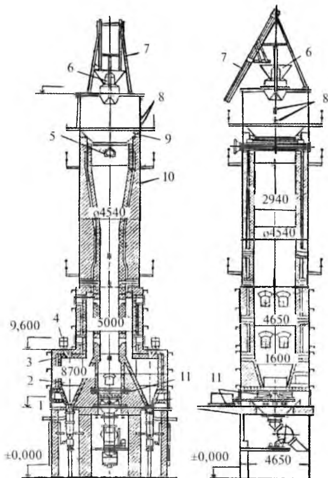
2-rasm. Aerofontan o'txonalı ohak kuydirish shaxta pechi:
