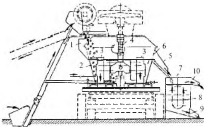
14-rasm. Uzlüksiz ishlovchi «IO3» markali ohak so'ndirish mashinasi:
