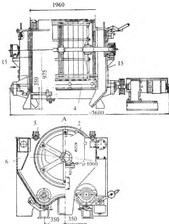
7-rasm. To'rtli silindr va vanna.
