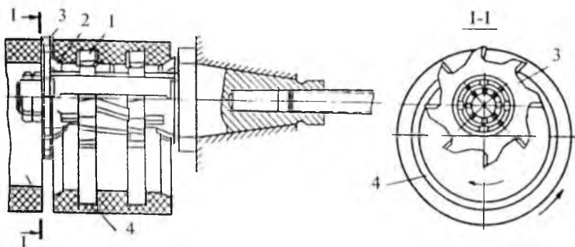
9-rasm. SAM turidagi muftalarni charxlash va qirqish uchun freza:
