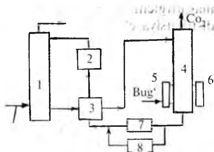
2-rasm. Monoetanolamin eritmasi bilan konvertirlangan gazdan \text{CO}_2 ni tozalashning prinsipial sxemasi.
