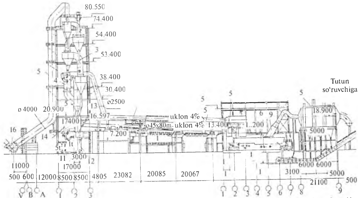
20-rasm. O'lchami Ø 4,5x80 m, siklonli issiqlik almashtirgichli, RSP dekarbonizatorli, sovitgich va uskunalar majmuasidan iborat aylanma pechli kuydirish sexi kesimi:
