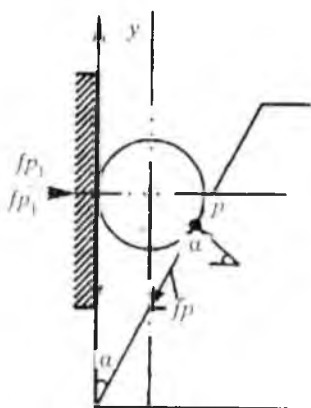
3-rasm. Jag'li maydalagichning optimal qamrov burchagmi aniqlash sxemasi:
