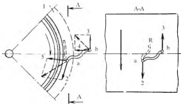
6-rasm. To'rli silindrda to'planuvchi tolalarning orientirlanish jarayoning sxemasi.
