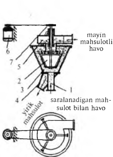
27-rasm. Urib-sovurib ishlovchi o'tish separatori:
