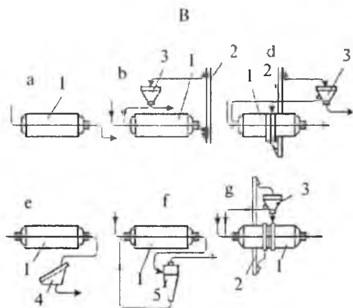
14-rasm. Zoldirli tegirmonlar va ularning ishlashi sxemasi:
