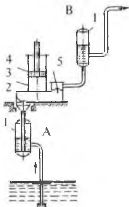
10-rasm. Bir marta harakatlanuvchi suruvchi (A) va haydovchi (V) liniyalarda havo qalpoqlari bor porshenli nasos:
