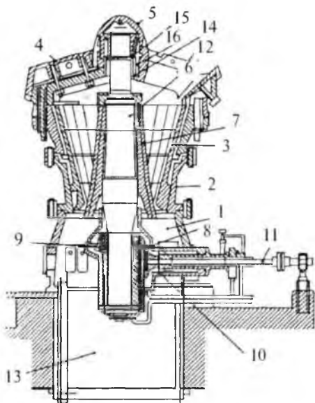
2-rasm. O'rnatma o'qli konusli maydalagich:
