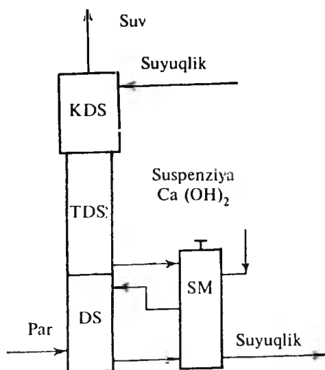
1-rasm. Soda ishlab chiqarishdagi distillatsiya elementining prinsipial sxemasi.
