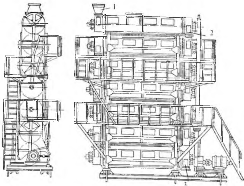
11-rasm. Uzlüksiz ishlovchl ko'p barabanli-kurakli gidrator: 1 – yuqori barabanning yuklash voronkasi; 2 – to'kuvchi patrubok; 3 – bo'shatish lyuki.
