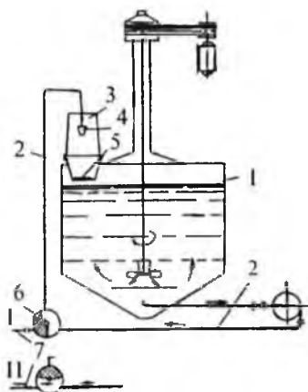
8-rasm. Asbest gidro'tg'itgichining ishlash sxemasi:
