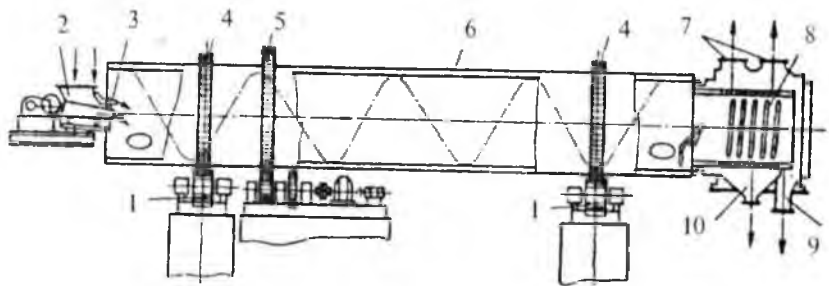
13-rasm. Uzlüksiz ishlovchi soʻndirish barabani:
