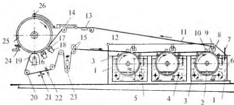
5-rasm. Yumaloq to'rtli varaq qoliqlash mashinasining sxemasi.
