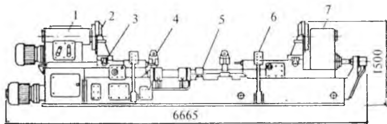
3-rasm. IS48N turidagi yarim avtomatlashgan quvur charxlovchi stanok 1 – old babka; 2 – konusli gribok; 3 – support; 4 – qabul qilgich; 5 – s'xina; 6 – knopkali boshqarish stansiyasi; 7 – orqa babka.
