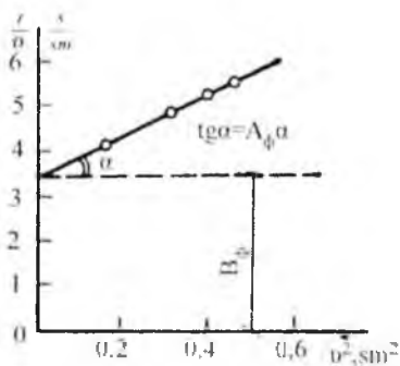
3-rasm. Filtratsiya tenglamasining filtratsiya grafigi bo'yicha doimiyligini aniqlash.
