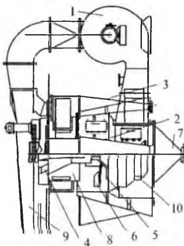
30-rasm. Tashqi ventilatorli va cho'ktirish zonasi tashqariga chiqarilgan sirkultatsion separator:
