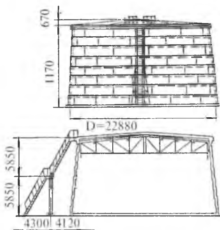
7-rasm. Vertikal rezervuar
