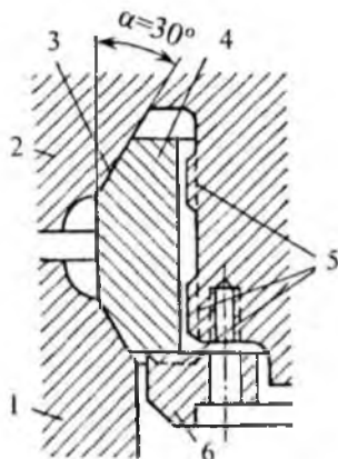
6-rasm. Plastik obtyurator bilan radial o'zi zichlovchi ikki konusli bolt:
