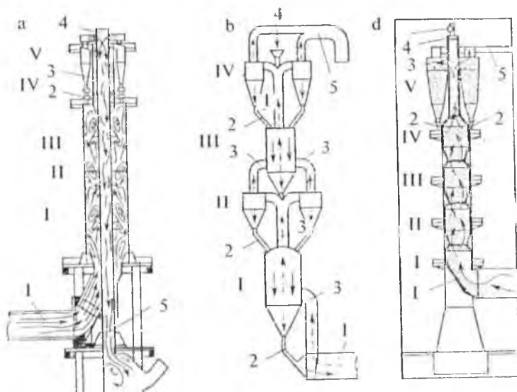
10-rasm. Shaxta siklonli va pech orqasida joylashgan sbaxtali issiqlik almash-tirgichlar sxemalari konstruksiyalari Giprotsement (a), Dopol (b), Sementalagenbau va Krupp (v): issiqlik almashtirgichning I, II, III va IV bosqichlari:
