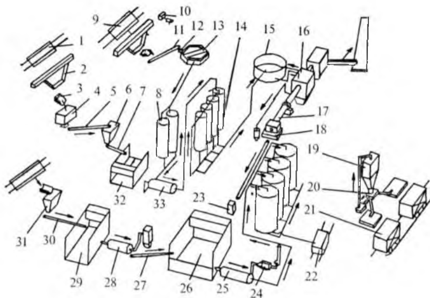
1-rasm. Sement zavodida ho'l usulda ishlovchi uskunalarning joylashish sxemasi.
