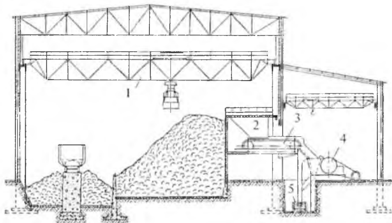
2-rasm. Yirik maydalash uchun qurilmasi bor greyferli ombor: 1 – greyferli kran; 2 – qabul qiluvchi bunker; 3 – plastinkali ta'minlagich; 4 – jag'li maydalagich; 5 – tasmali tranportyor.
