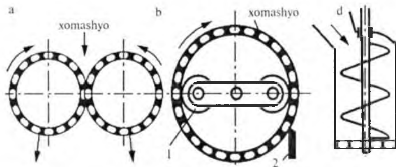
41-rasm. Ekstruzion tipdagi donalagichlar:
