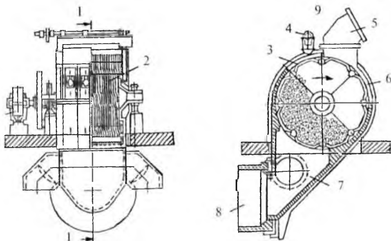
4-rasm. Shlam konsentratori.
