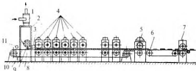
4-rasm. Quruq usulda taxtalangan varaqlar qoliqlash qurilmasi.
