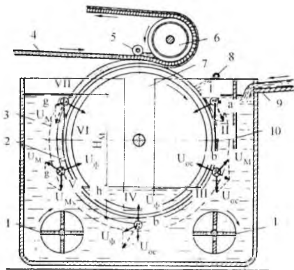
4-rasm. Asbestsement varag'i qoliqlash mashinasining to'rtli silindri va vannasining sxemasi.
