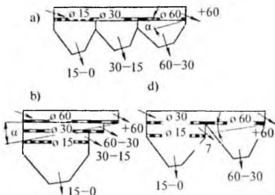
1-rasm. Sim g'alvirlarda elash sxemasi.
