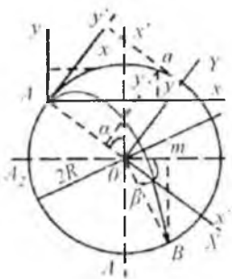
13-rasm. Zoldirlarning baraban ichida harakatlanish yo'lini aniqlash sxemasi.
