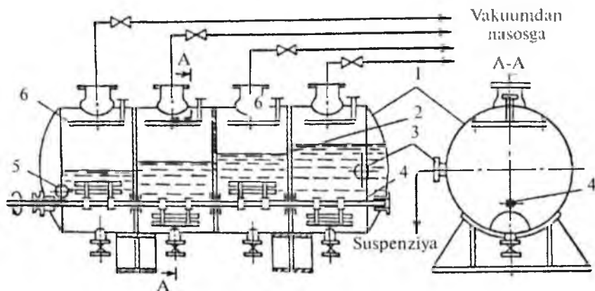
1-rasm. Ko'p bosqichli gorizantal vakuum-kristallizator:
