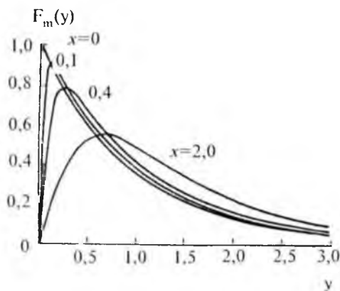
5-rasm. Yakka reaktorda bo'lib turish vaqti bo'yicha noideal aralashtirishning zarrachalarni taqsimlanishiga ta'siri.
