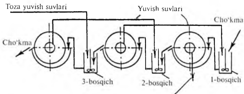
6-rasm. Cho'kmani uch bosqichli qarama-qarshi oqimda yuvish sxemasi: 1 – 3 – repulporlar.
