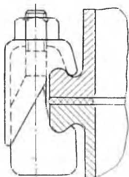
11-rasm. Skobalar bilan tortiladigan flanetsli birikma.
