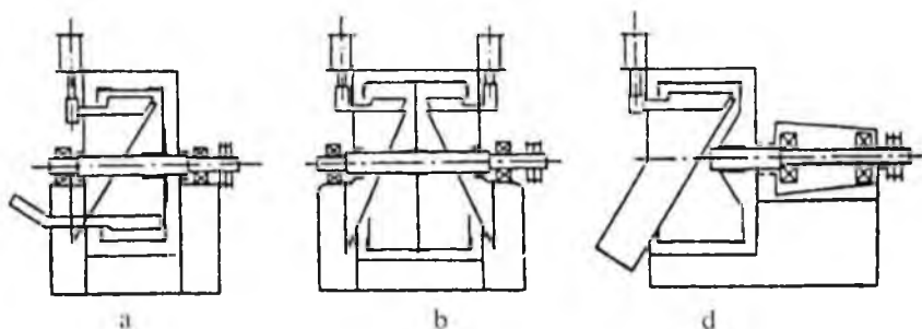
4-rasm. FGN tipidagi sentrifugalarda rotorning joylashish sxemasi:
