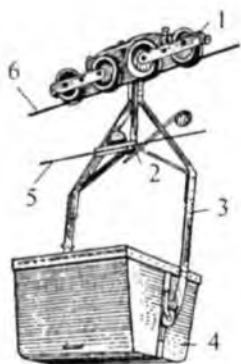
2-rasm. Osma arqonli yo'l vagonetkasi: 1 – suriluvchi qism; 2 – tortuvchi arqonli tirkash moslamasi; 3 – ilgak; 4 – kuzov; 5 – tortuvchi arqon; 6 – tutib turuvchi arqon.
