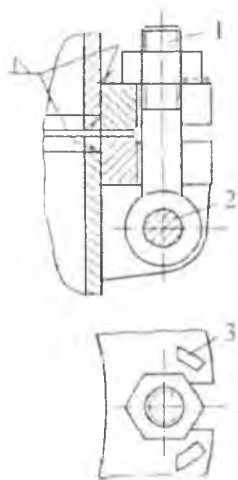
13-rasm. Qaytarma boltli flanesli birikma.
