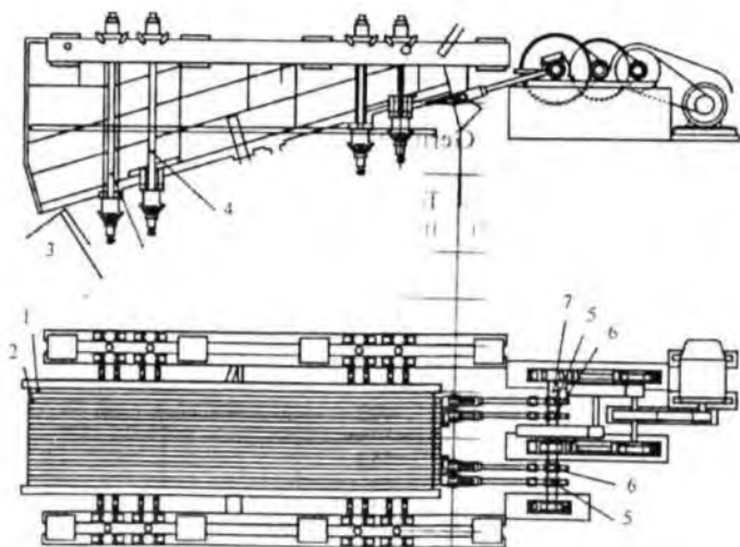
3-rasm. Harakatlanuvchi kolosnikli-g'alvirli ta'minlagich.
