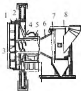
10-rasm. Harakat chetdan uzatiladigan va tuyilgan mahsulot barabanning o'rta qismidan bo'shatib olinadigan tegirmonning bo'shatish qismi:
