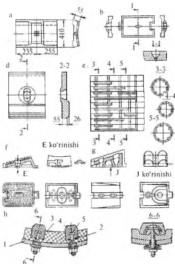
4-rasm. Tegirmondagi zirh taxtlar va ularning joylashish sxemasi:
