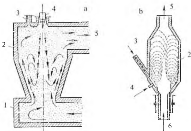
12-rasm. Xomashyo kukunini to'liq dekarbonizatsiyalash va yoqilg'ini yoqish (kalsinator) kameralari sxemasi:
