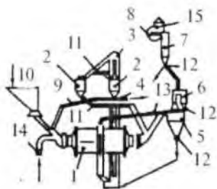
17-rasm. Markazdan qochma separatorli quritish-maydalash sxemasi:
