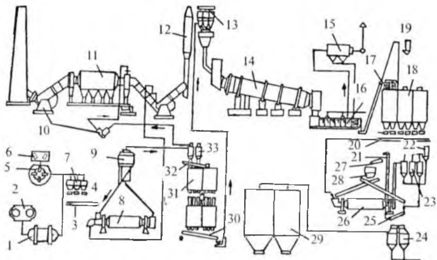
2-rasm. Quruq usulda sement ishlab chiqaruvchi uskunalarining joylashish sxemasi.
