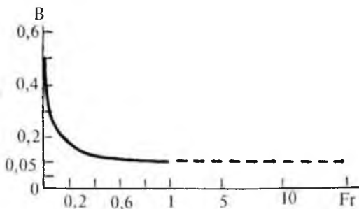
1-rasm. Propellerli aralashtirgichlar uchun B=f(Fr) funksiyasining grafigi.
