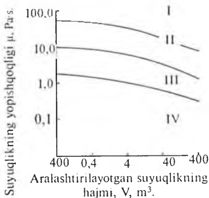
3-rasm. Turli xil aralashtirgichlarning qo'llanish oralig'i (diapazoni):
