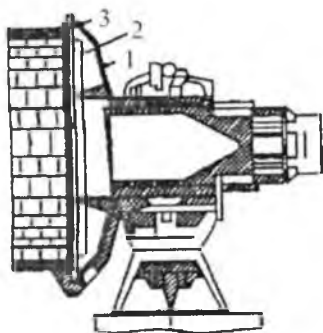
8-rasm. Markaziy uzatma va materialni chetda bo'shatadigan tegirmonning bo'shatish qismi:
