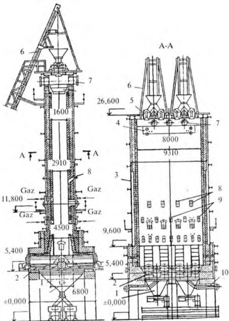
3-rasm. Gazsimon yoqllg'ida ishlovchi, unumdorligi sutkasiga 150 t bo'lgan ohak kuydirish shaxta pechi:
