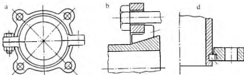
10-rasm. Flanetslarni ajraladigan turlari:
