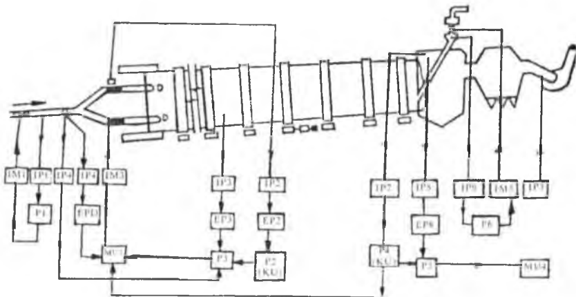
22-rasm. Rekuperatorli sovitgichlari bo'lgan 3,6x150 m o'lchamli aylanma pechlar uchun kuydirish jarayonlarini avtomatik boshqarishning blok sxeması:
