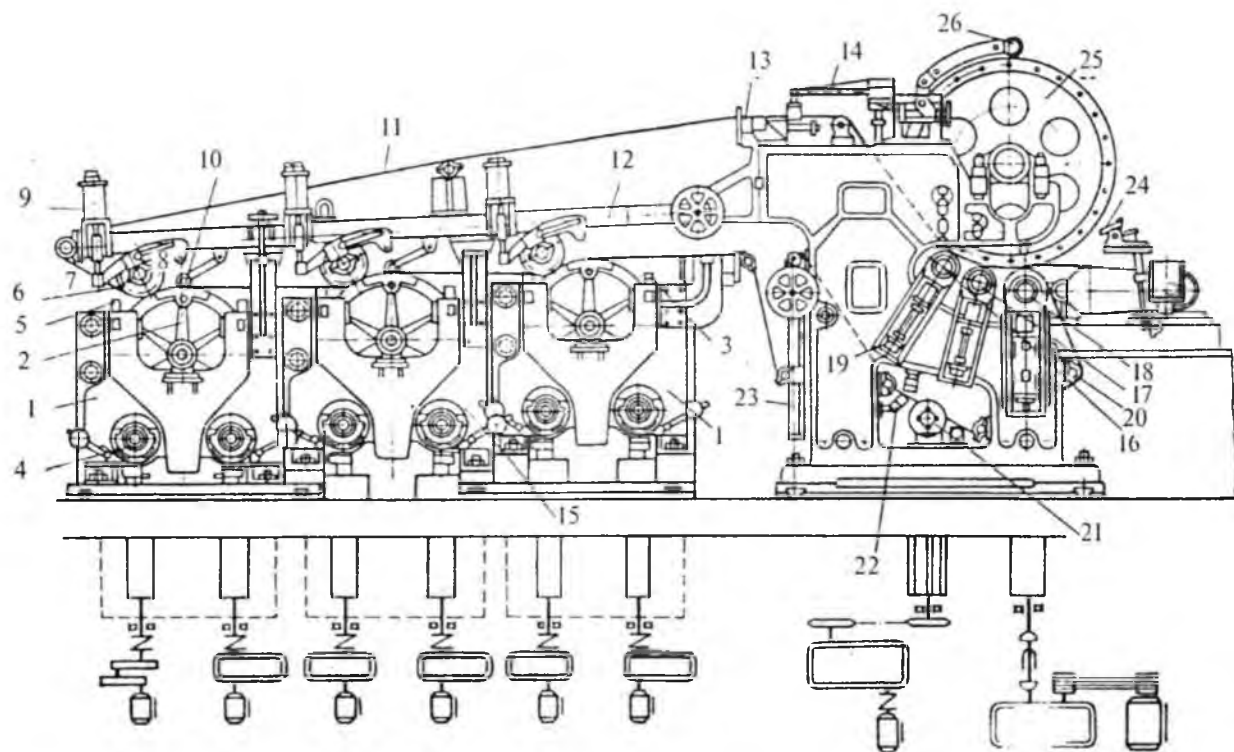
6-rasm. SM-942 (SM-943) varaq qoliplash mashinalari asosiy uzellarining tuzilishi.
