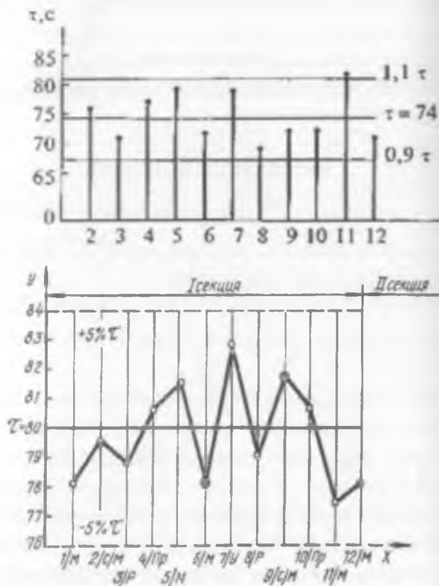
22 - rasm. Moslik (sinxron) grafiglar
