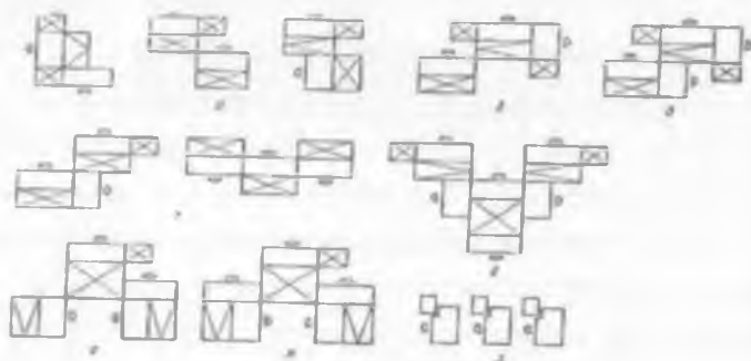
29 - rasm. Ish o'rinlarini joylashtirish variantlari
