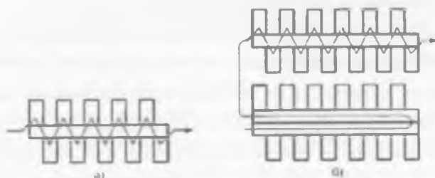
15 - rasm. Bir guruhli konveyerli oqimlar.
