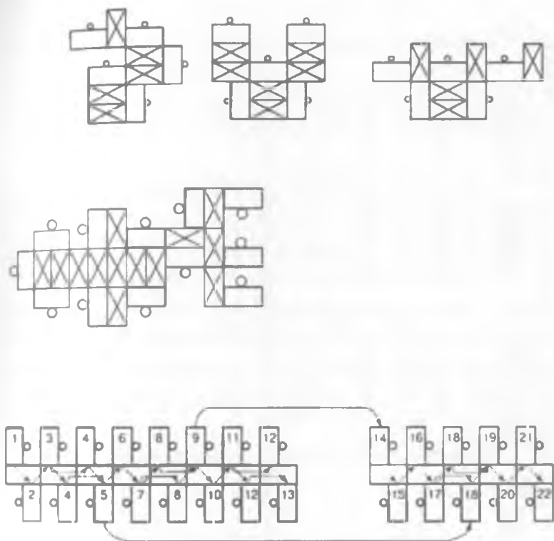
33 - rasm. Oqimda ish o'rinlarini joylashtirish namunalari
