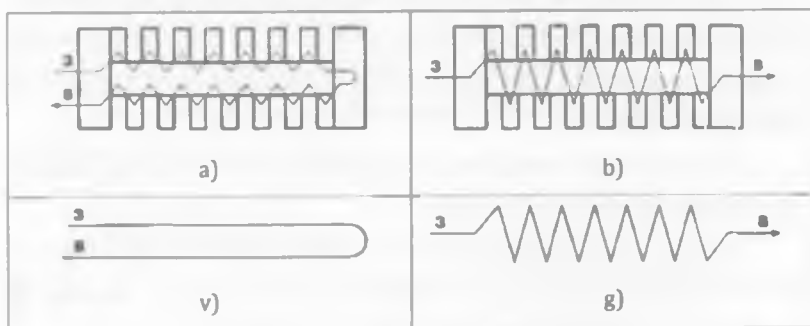
16 - rasm. Yarimfabrikatlarning oqimdagi harakati.
