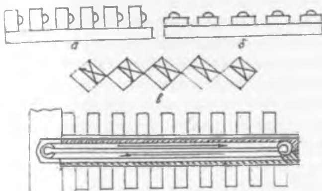
27 - rasm. Ish o'rinlarini joylashtirish
