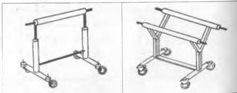
44 - rasm. Detallar pachkasini fiksatsiyalab uzatish qurilmasi.
