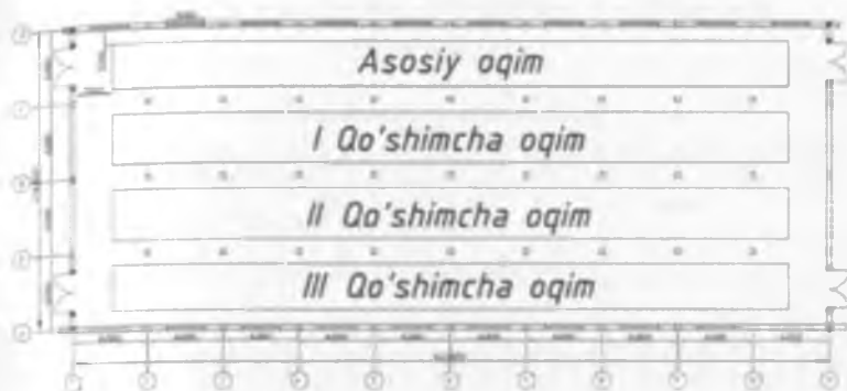
25 - rasm. Texnologik jarayondagi qo'shimcha oqimlarni loyihalash
