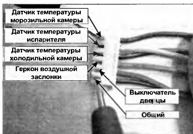
Рис. 6.7. Проверка датчиков на соединителе
