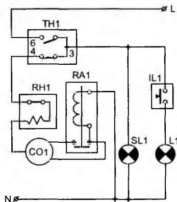
Рис. П2.12. Электрическая принципиальная схема электрооборудования холодильника «СТИНОЛ-242»:
