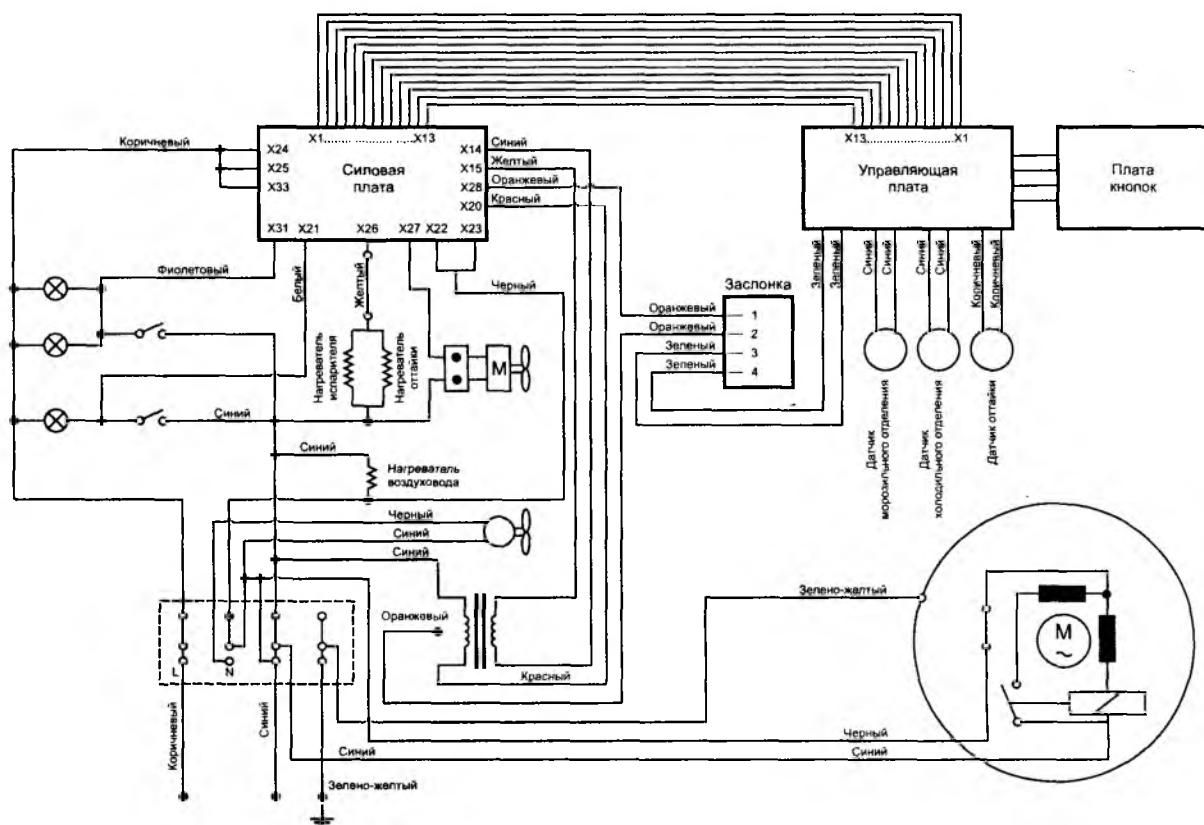
Рис. 9.8. Электрическая схема соединений узлое и плат холодильника
