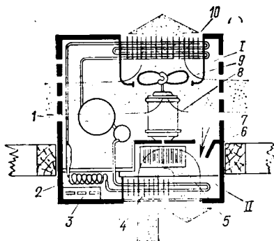
Рис. V.14. Автономный кондиционер оконного типа
