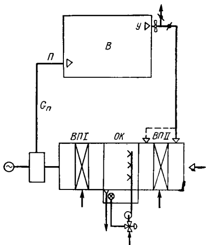
Рис. IV.15. Схема СКВ с применением первой рециркуляции
