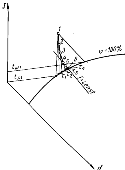
Рис. II.19. Изменение во времени состояния воздуха в точке 1 при его контакте с водой, имеющей начальную температуру t_{p1} < \tau_1 < t_{M1} (при параллельном токе)
