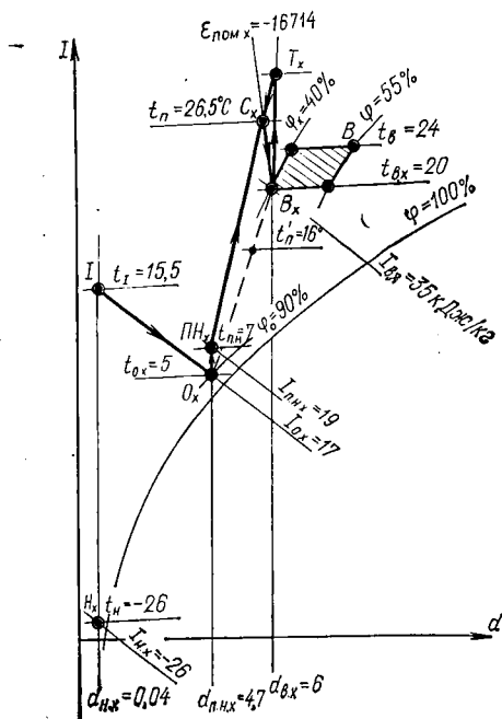
Рис. VI.18. I-d -диаграмма к примеру расчета режимов обработки воздуха в эжекционной СКВ в холодный период
