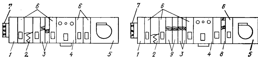
Рис. VI.3. Базовая схема 1 (Сх. 1) и ее модификация (Сх. 1.8)
