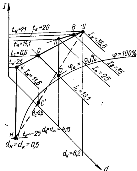
Рис. IV.21. I-d -диаграмма изменения состояния воздуха в СКВ с первой рециркуляцией для режима холодного периода при подмешивании рециркуляционного воздуха после воздухоподогревателя I ступени
