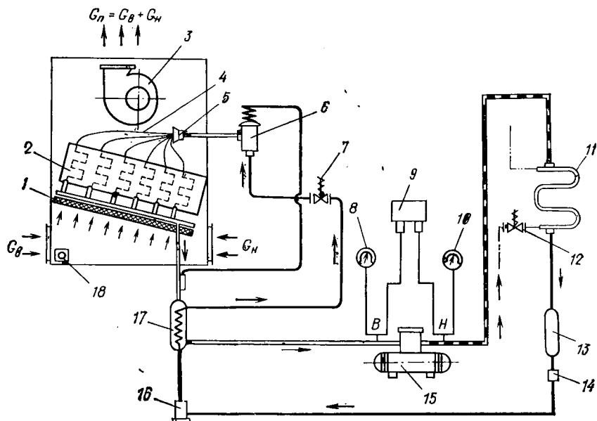
Рис. VII.7. Автономный кондиционер КТА 1 с водяным конденсатором
