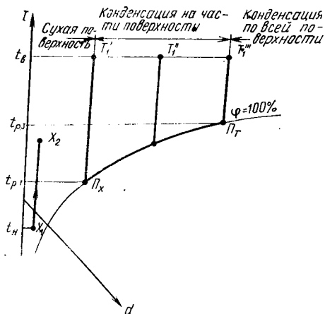
Рис. X.3. Области сухого теплообмена и теплообмена с конденсацией в воздухо-воздушных рекуператорах
