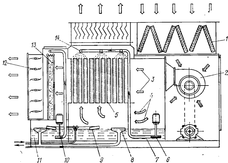
Рис. VII.5. Местный кондиционер двухступенчатого испарительного охлаждения
