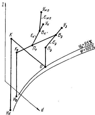
Рис. IV.33. I-d -диаграмма с режимами кондиционирования воздуха и вентиляции помещений с различным характером выделения вредных веществ для режима холодного периода
