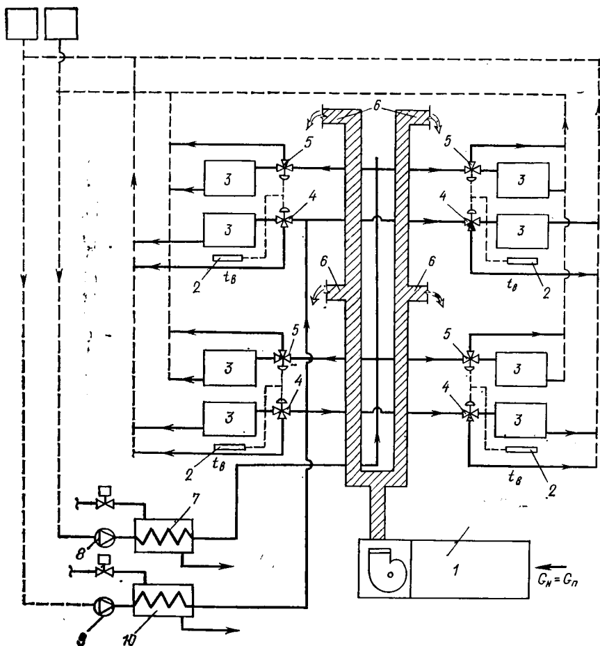
Рис. IX.12. Четырехтрубная система холодо- и теплоснабжения местных неавтономных кондиционеров с регулированием по воде
