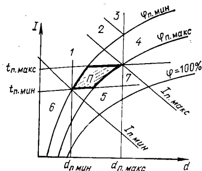
Рис. IV.35. К выбору способа обработки воздуха
