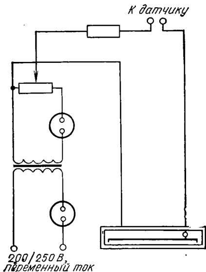
Рис. 11.5. Принципиальная схема устройства для измерения влажности воздуха с отрицательной температурой психрометрическим методом
