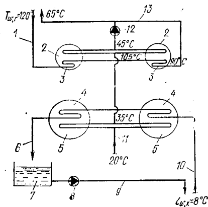
Рис. VIII.12. Принципиальная схема применения двух абсорбционных холодильных машин для одновременной выработки холода и воды, подаваемой на нужды горячего водоснабжения
