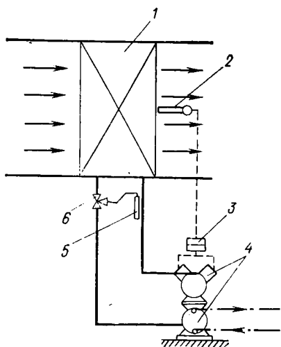
Рис. VIII.11. Принципиальная схема местной системы холодоснабжения от холодильной машины
