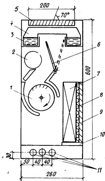
Рис. VII.3. Местный неавтономный кондиционер-доводчик (ВКД)
