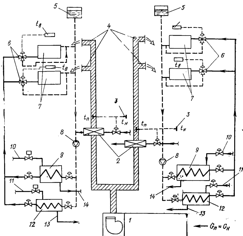
Рис. IX.7. Двухтрубная система тепло- и холодоснабжения местных неавтономных кондиционеров
