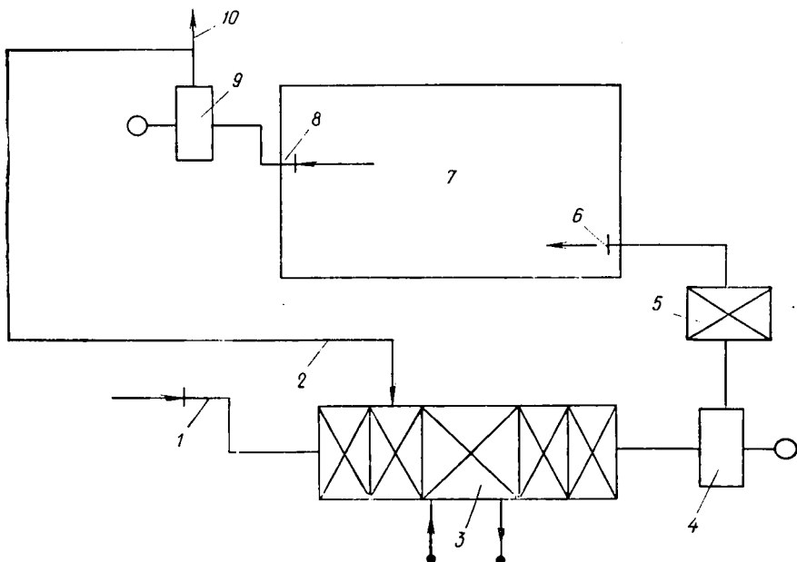
Рис. 1.3. Принципиальная схема системы кондиционирования воздуха
