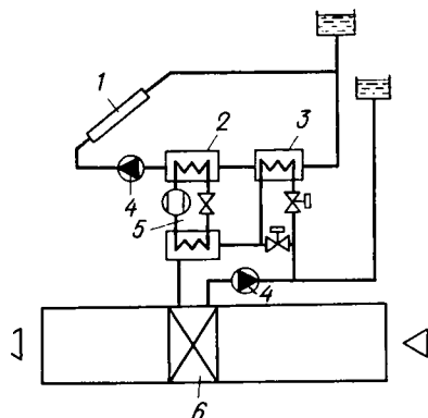
Рис. X.16. Непосредственное включение гелиоприемника в СКВ
