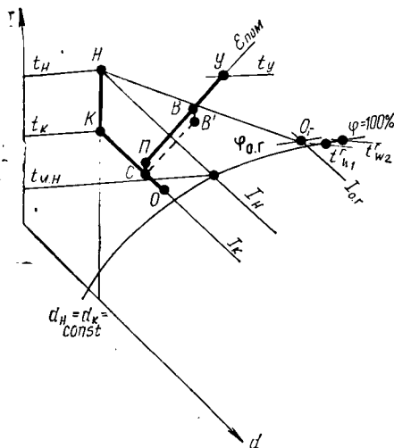
Рис. IV.9. I-d диаграмма с режимом двухступенчатого испарительного охлаждения
