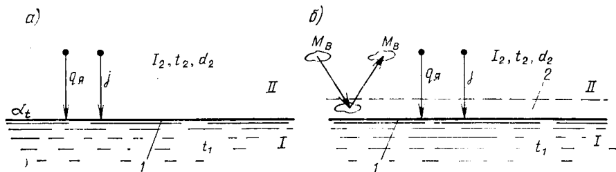
Рис. III.1. Трактовки обменных процессов между водой I и воздухом II на основе закона Ньютона (а) и аналогии Рейнольдса (б) 1 — поверхность воды; 2 — слой воздуха, непосредственно прилегающий к поверхности
