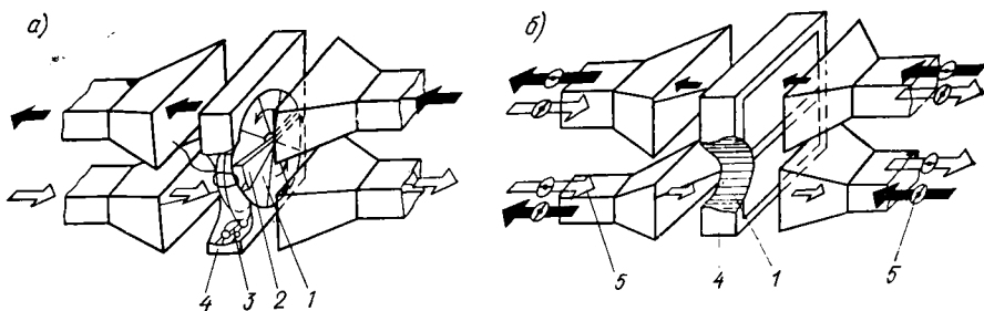
Рис. X.8. Схемы устройства воздушно-воздушных регенеративных утилизаторов
