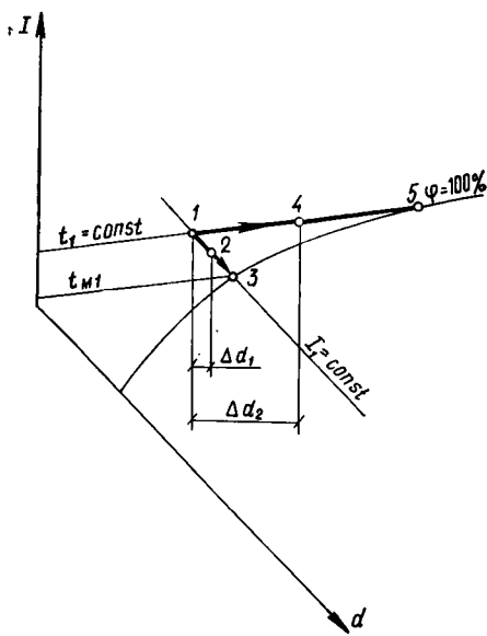
Рис. II.12. I-d -диаграмма с режимами изохентального и изотермического увлажнения воздуха
