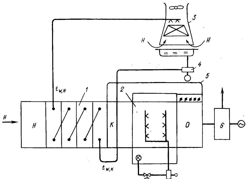
Рис. IV.8. Схема СКВ двухступенчатого испарительного охлаждения
