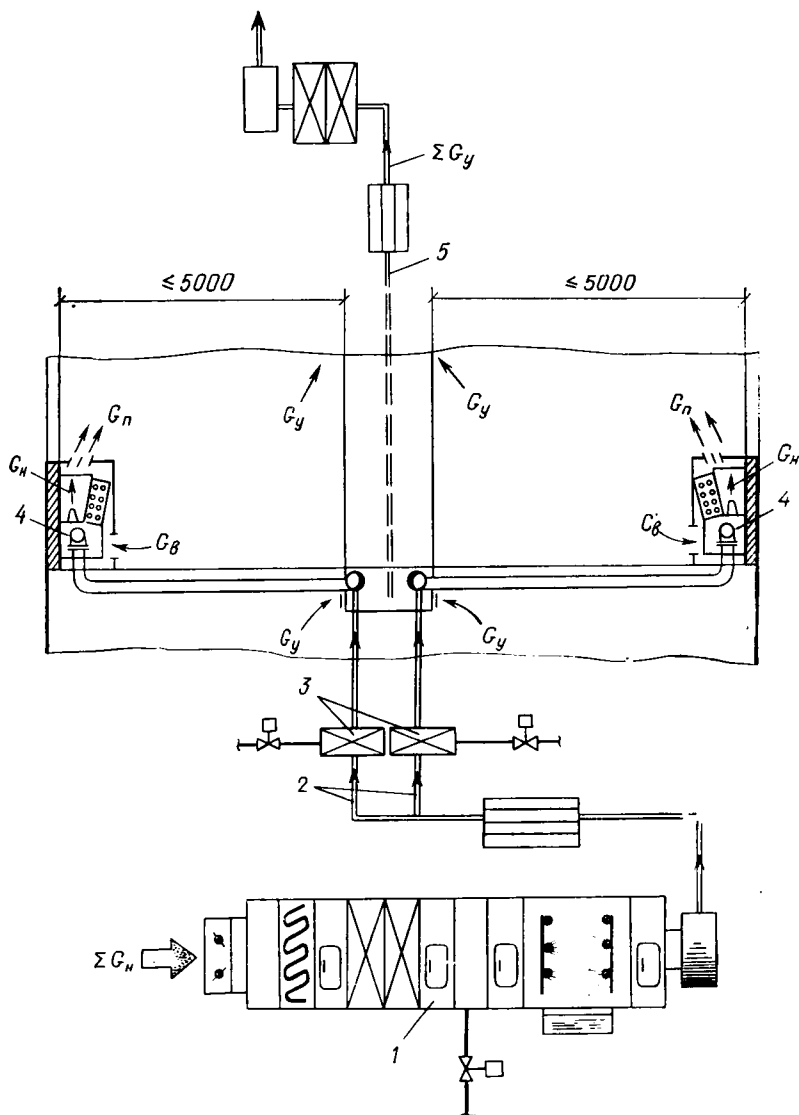
Рис. V.9. Местно-центральная СКВ с ЭКД
