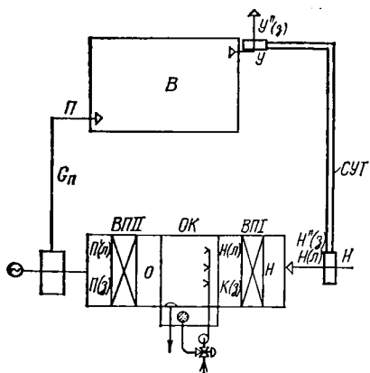
Рис. IV.12. Схема проточной СКВ с использованием воды от внешних источников холодоснабжения
