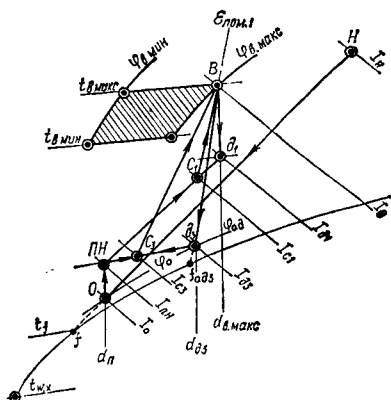
Рис. V.6. Выкопировка из I-d -диаграммы режимов обработки воздуха в центральной УКВ и местных агрегатах-доводчиках в теплый период года в многозональной местно-центральной СКВ
