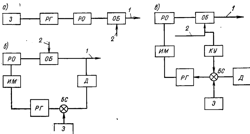
Рис. XI.8. Структурные схемы САР
