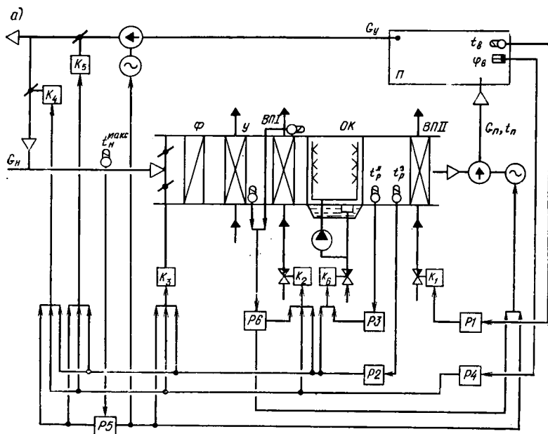
Рис. XI.5. Принципиальная схема с контурами регулирования (а), процесс тепловлажностной обработки воздуха (б), график регулирования параметров воздуха в помещении (в), графики регулирования работы теплообменных и смешивающих аппаратов (г) СКВ
