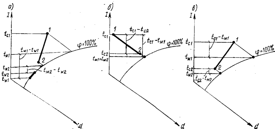
Рис. III.8. К определению коэффициентов эффективности (по методу НИИСТ) а — коэффициента эффективности полного теплообмена; б — коэффициента эффективности адиабатного (изотальпийного) процесса; в — универсального коэффициента эффективности
