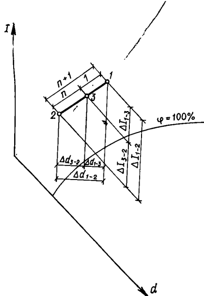
Рис. 11.13. I-d -диаграмма с режимом смещения двух масс воздуха различного состояния
