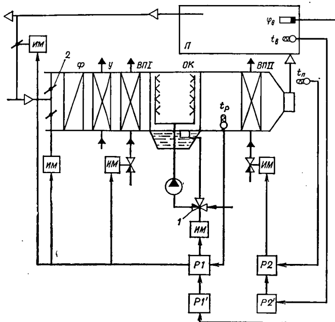
Рис. XI.16. Функциональная схема каскадной системы управления СКВ
