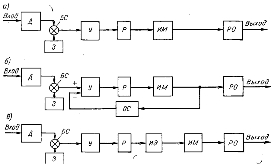
Рис. XI.7. Блок-схемы автоматических регуляторов, применяемых в СКВ
