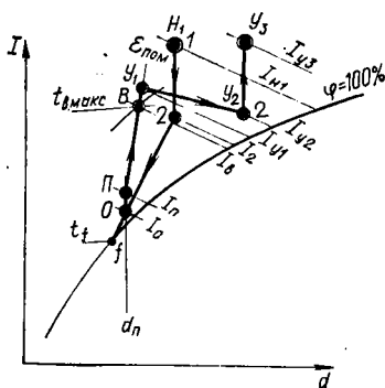
Рис. VIII.16. I-d -диаграмма режимов работы СКВ с использованием комбинированной схемы охлаждения приточного воздуха
