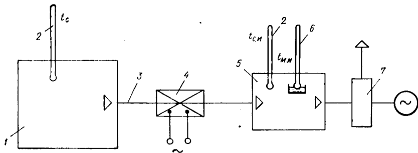
Рис. 11.5. Принципиальная схема устройства для измерения влажности воздуха с отрицательной температурой психрометрическим методом
