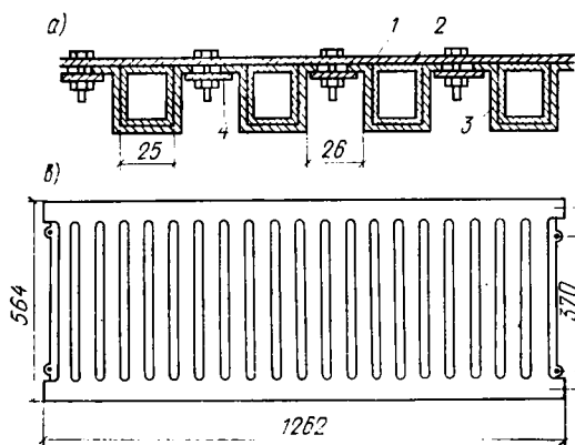
Рис. X.15. Типы абсорбционных гелиоприемников
