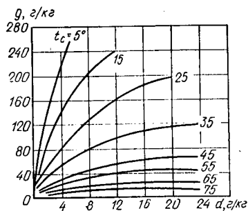
Рис. 11.26. Зависимость равновесного влагосодержания силикагеля от температуры и влагосодержания воздуха
