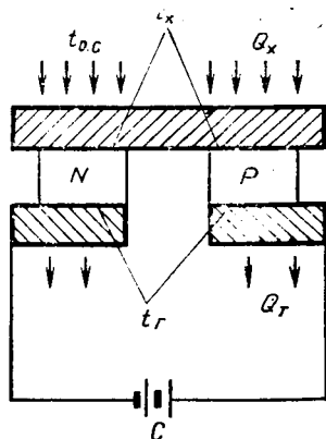
Рис. VIII. 5. Принципиальная схема термоэлектрического метода получения холода и тепла
