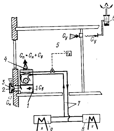
Рис. V.12. Местная СКВ на базе вентиляторных кондиционеров-доводчиков (ВКД) 1 — ВКД; 2 — клапан регулирования забора наружного воздуха; 3 — отверстия в стене; 4 — приточная решетка; 5 — датчик контроля температуры внутреннего воздуха; 6 — вытяжной вентилятор; 7 — трубопроводы циркуляции горячей и холодной воды; 8 — центральный теплообменник нагрева воды; 9 — то же, охлаждения воды
