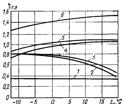
Рис. X.24. Термозкономический показатель по затратам первичного топлива различных систем
