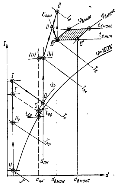
Рис. V.11. I-d -диаграмма с режимами обработки воздуха в центральной УКВ с ЭКД в холодный период
