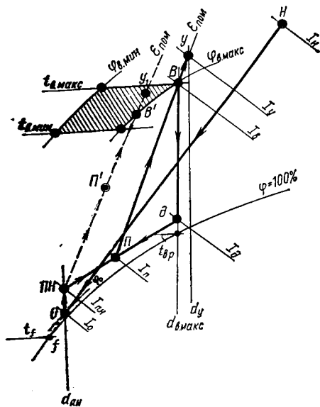
Рис. V.10. Выкопировка из I-d -диаграммы режимов обработки воздуха в центральной УКВ с ЭКД в теплый период
