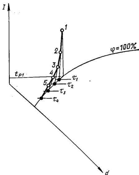
Рис. II.21. Изменение во времени состояния воздуха в точке 1 при его контакте с водой, имеющей начальную температуру \tau_1 < t_{p1} (при противотоке)
