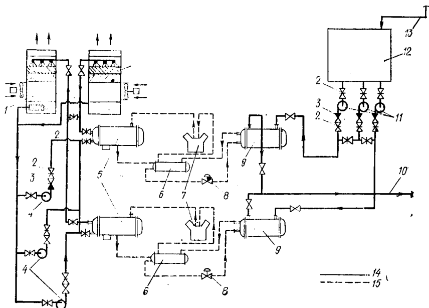
Рис. IX.1. Принципиальная схема центральной холодильной станции из двух агрегируемых машин 2МКТ 110
