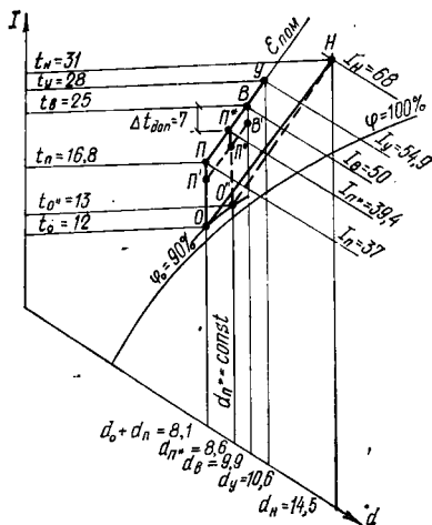
Рис. IV.13. I-d -диаграмма изменения состояния воздуха в проточной СКВ при минимальном расходе приточного воздуха
