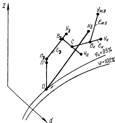
Рис. IV.32. I-d -диаграмма с режимами кондиционирования воздуха и вентиляции помещений с различным характером выделения вредностей для режима теплого периода
