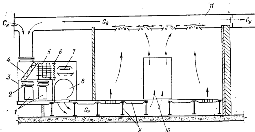
Рис. V.16. СКВ для обслуживания помещения с ЭВМ
