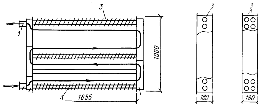
Рис. VI.9. Одномерный базовый теплообменник для кондиционеров КТЦ2
