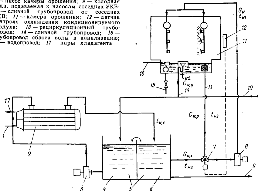
Рис. IX.2. Схема снабжения холодной водой небольшой группы камер орошения, расположенных вблизи холодильной станции
