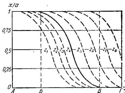
Рис. 11.27. Изменение влажности силикагеля
