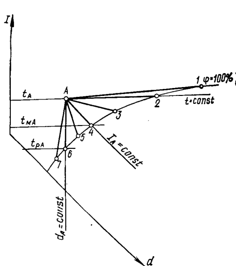
Рис. II.17. I-d -диаграмма характерных процессов тепло- и влагообмена воздуха с водой при различных ее температурах
