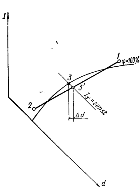
Рис. П.14. I-d -диаграмма с режимом смещения воздуха при расположении точки смеси ниже линии \varphi=100\%
