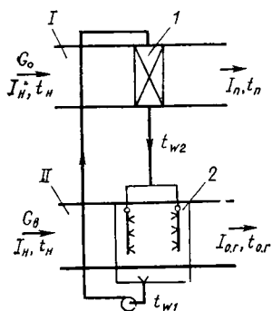
Рис. IV.5. Схема косвенного испарительного охлаждения 1 — теплообменник-воздухоохладитель; 2 — контактный аппарат
