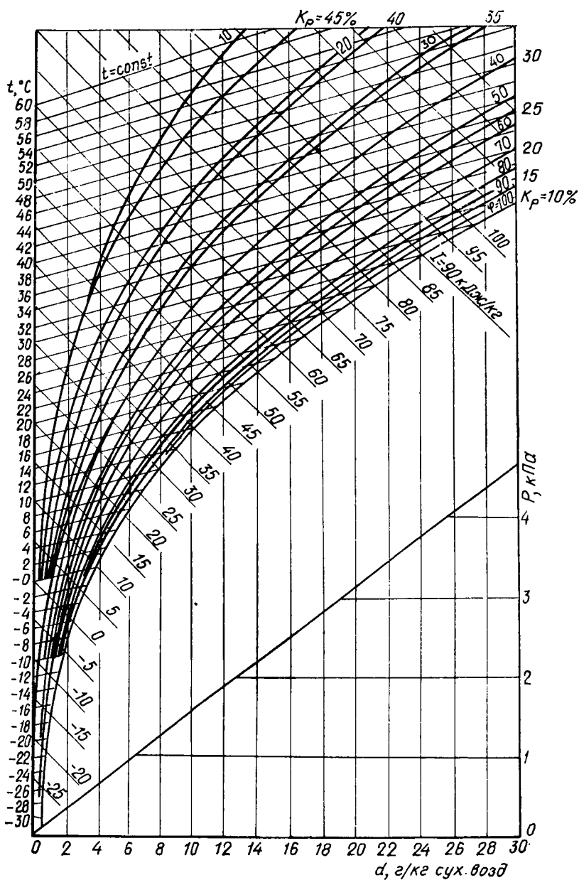
Рис. II.25. t-d -диаграмма равновесного состояния водяного пара над поверхностью раствора хлористого лития
