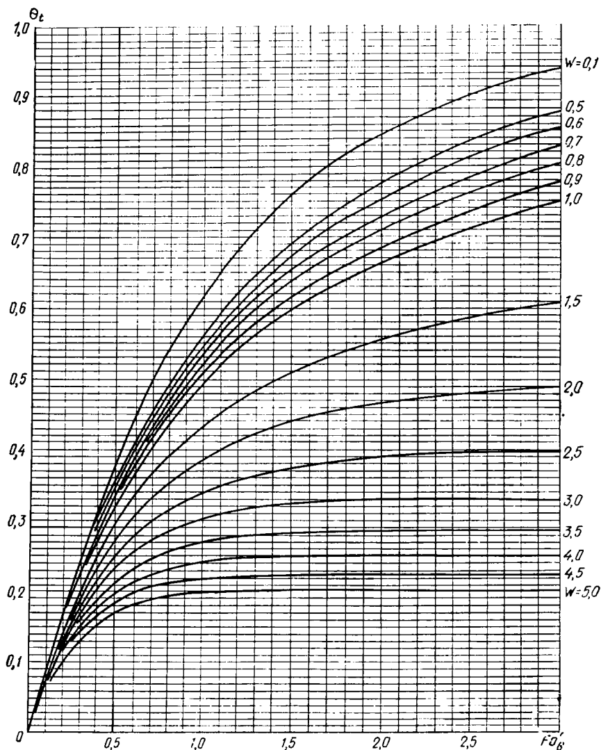
Рис. VI.10. Графическая зависимость \theta_t от критерия Fo'_B в противоточном теплообменнике
