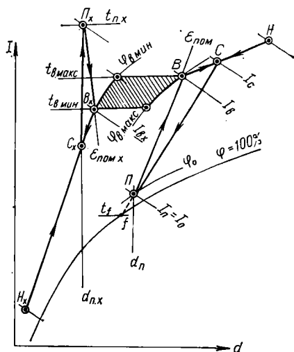
Рис. V.13. I-d -диаграмма с режимами круглогодичной обработки воздуха в вентиляторном кондиционере-доводчике
