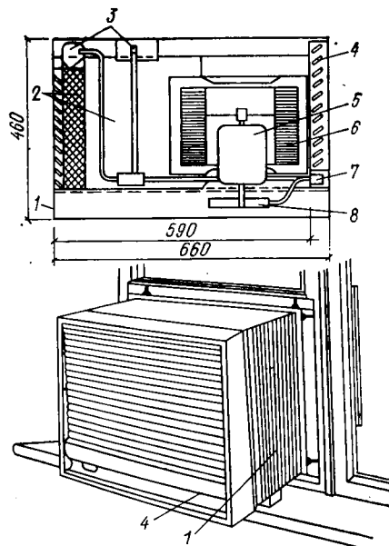
Рис. V.15. Кондиционер испарительного охлаждения
