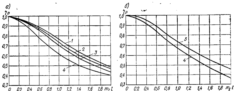
Рис. 111.3. Эффективность плоского (а) и круглого (б) ребер различной геометрической конфигурации, имеющих разную форму сечения 1 — вогнутая парабола; 2 — выпукнутая парабола; 3 — треугольник; 4 — прямоугольник
