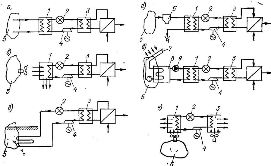
Рис. X.11. Способы использования теплового насоса для утилизации тепла различных источников
