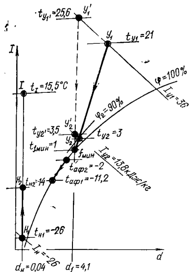
Рис. VI.19. I-d -диаграмма к примеру расчета системы утилизации тепла вытяжного воздуха
