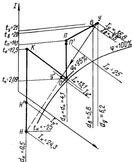
Рис. IV.19. I-d -диаграмма изменения состояния воздуха в приточной СКВ для режима холодного периода
