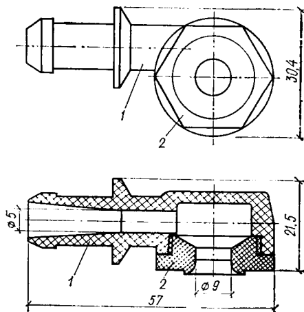
Рис. VI.5. Широкофакельная форсунка ШФ 9/5
