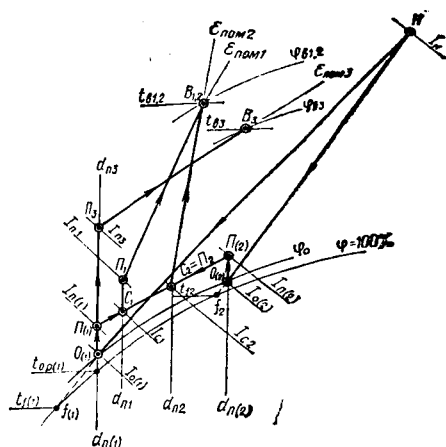
Рис. V.8. Выкопировка из I — d-диаграммы режимов обработки воздуха в теплый период в многозональной СКВ с двумя параллельными УКВ и зональными ДС и ВК
