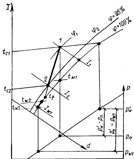
Рис. III.10. К расчету процесса охлаждения и осушки воздуха в камере орошения (к методу О. Я Кокорина) ( t_f — условная средняя температура поверхности контакта)
