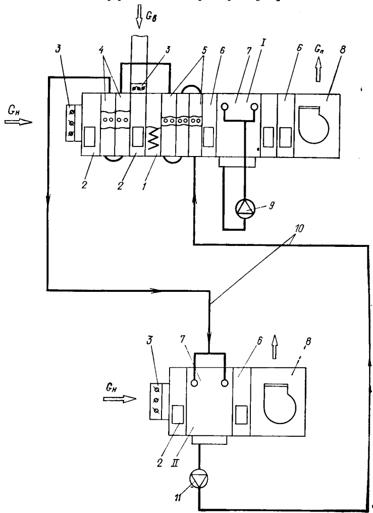
Рис. VIII.14. Принципиальная схема СКВ с двухступенчатым испарительным охлаждением воздуха
