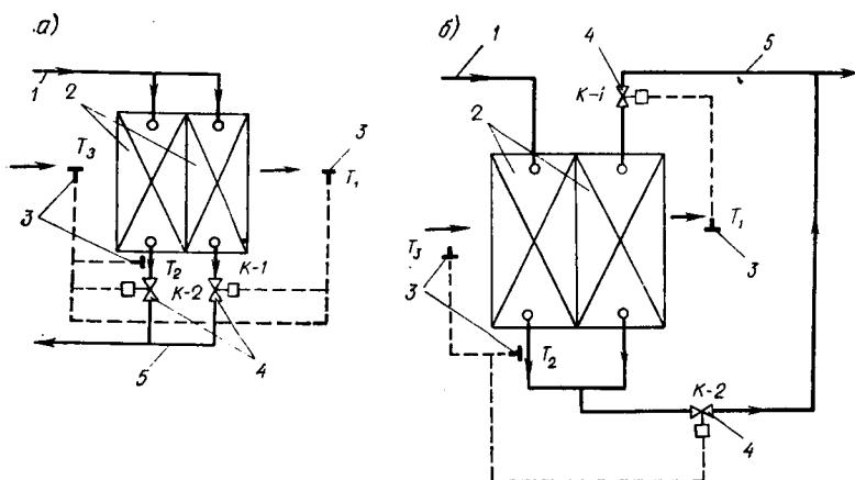
Рис. IX.4. Схема снабжения горячей водой воздухонагревателей I подогрева с защитой от замерзания
