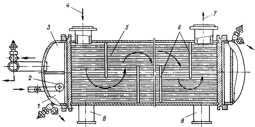
Рис. VIII.10. Кожухотрубный испаритель
