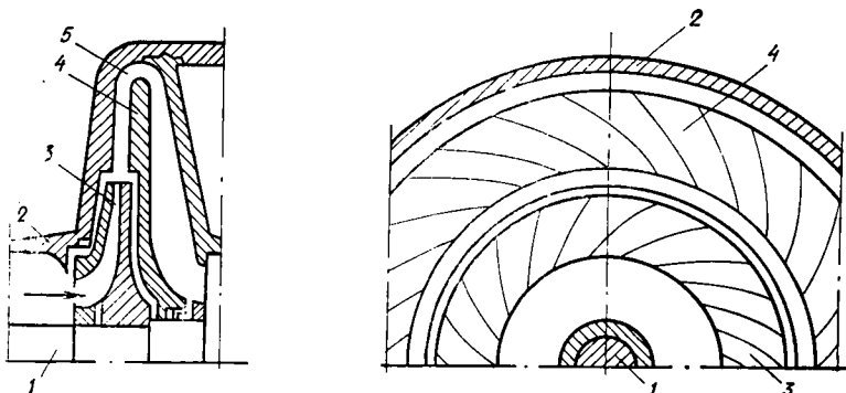
Рис. VIII.8. Ступень сжатия холодильного агента в турбокомпрессоре 1 — вал, соединенный с приводом; 2 — неподвижный корпус; 3 — лопатки рабочего колеса; 4 — диффузор; 5 — направляющий канал
