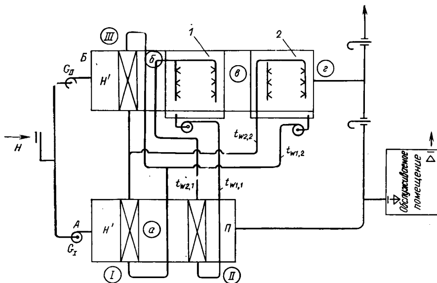
Рис. IV.10. Схема бескомпрессорной системы кондиционирования воздуха (БСКВ)
