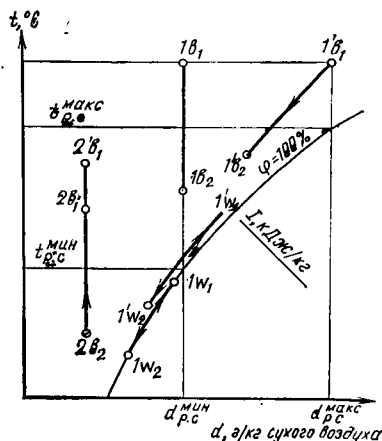
Рис. X.7. Процессы изменения состояния воздуха на t-d -диаграмме в системе утилизации тепла с рекуперативными теплообменниками и промежуточным теплоносителем
