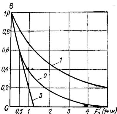
Рис. III.7. Зависимость \theta=f[Fo'(1+W)] 1 — среднеинтегральные по Fo'(1+W) значения \theta ; 2 — локальные значения \theta ; 3 — то же, на начальном участке до Fo'(1+W) < 0,5
