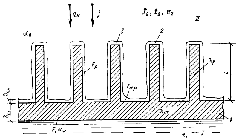
Рис. III.2. Передача полного тепла через оребренную поверхность при совместно протекающем процессе тепло- и массообмена
