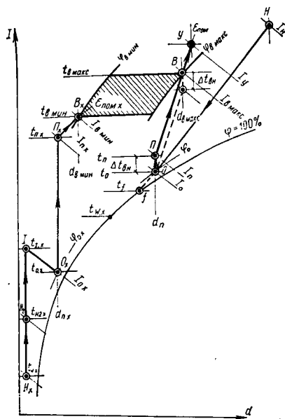
Рис. V.2. I-d -диаграмма с режимом обработки приточного воздуха в однозональной приточной СКВ в расчетных условиях теплого и холодного периодов года
