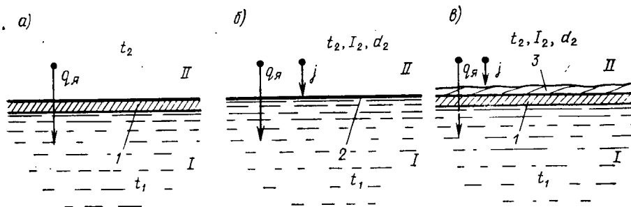
Рис. III.4. Модели тепло- и массопереноса в аппаратах СКВ
