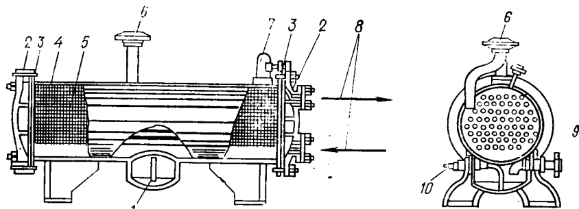
Рис. VIII.9. Горизонтальный кожухотрубный конденсатор 1 — ресивер; 2 — крышки; 3 — трубные решетки; 4 — кожух; 5 — оребренные теплообменные трубы; 6 — патрубок для подачи паров хладагента; 7 — предохранительный клапан; 8 — охлаждающая обратная вода; 9 — патрубок для выхода жидкого хладагента; 10 — спускной клапан
