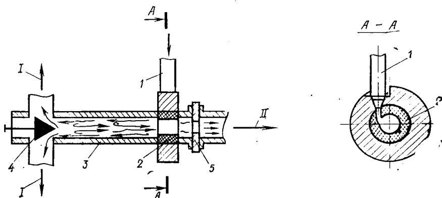
Рис. VIII.4. Вихревая труба
