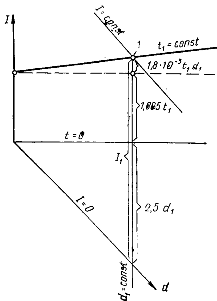
Рис. 11.2. Графическое изображение энтальпии, соответствующей точке I_1 , лежащей на линии t_1 = \text{const}
