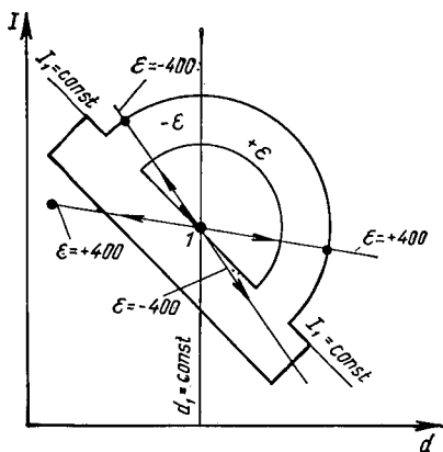
Рис. 11.9. Применение транспорта углового масштаба для нанесения на I-d -диаграмму линий изменения состояния влажного воздуха
