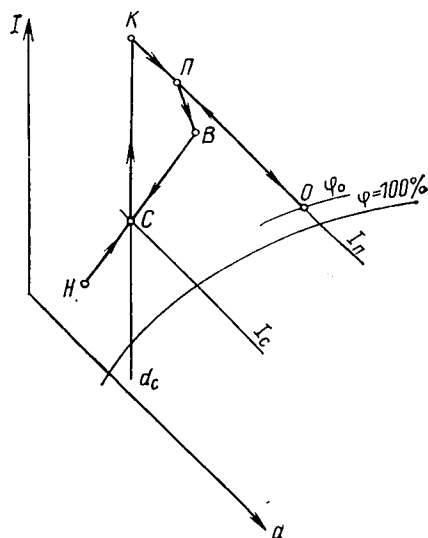
Рис. IV.24. I-d диаграмма с режимом кондиционирования воздуха для холодного периода с использованием кондиционера двухступенчатого испарительного охлаждения
