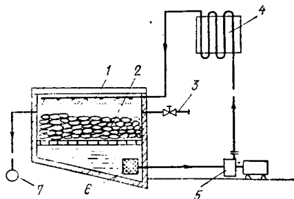
Рис. VIII.1. Принципиальная схема использования заготовленного зимой льда для охлаждения кондиционируемого воздуха
