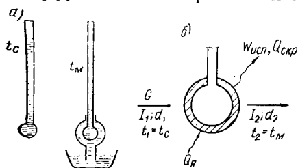
Рис. II.4. Психрометр
