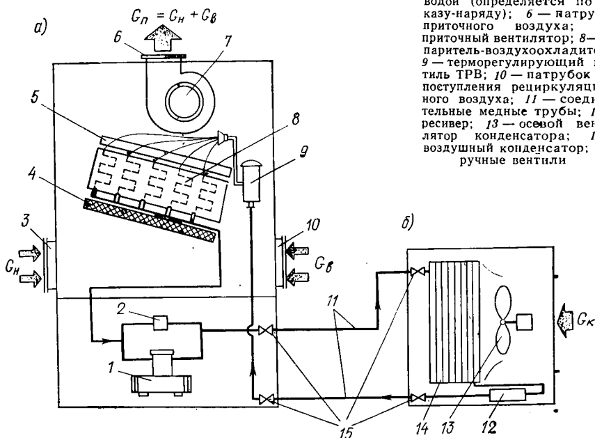
Рис. VII.8. Автономный кондиционер КТА2 с воздушным конденсатором
