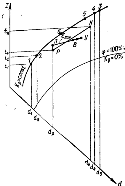
Рис. IV.27. I-d -диаграмма изменения состояния воздуха в СКВ с применением раствора хлористого лития для помещений с большими влаговыведениями для режима теплого периода
