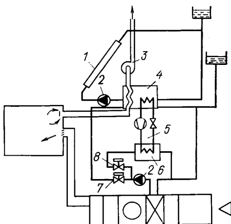
Рис. X.17. Подключение гелиоприемника к СКВ через постоянно работающий тепловой насос
