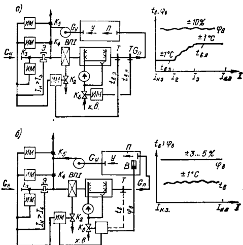
Рис. XI.9. Возможные схемы контура регулирования t_B в однозональной КВ
