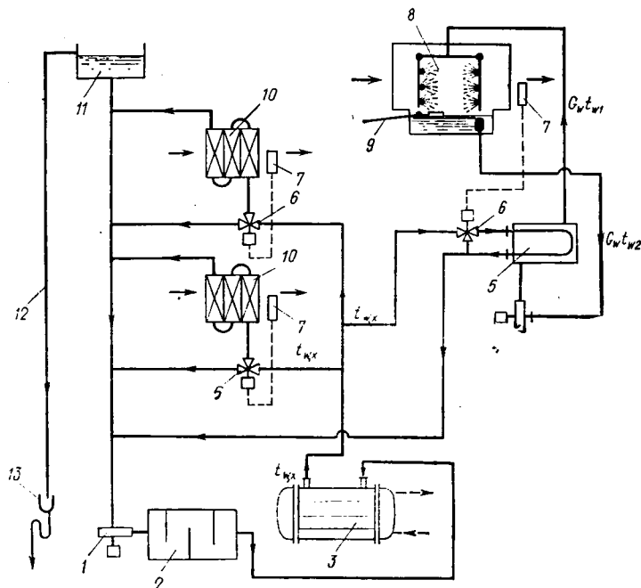
Рис. IX.3. Закрытая схема снабжения холодной водой камер орошения и поверхностных теплообменников в УКВ
