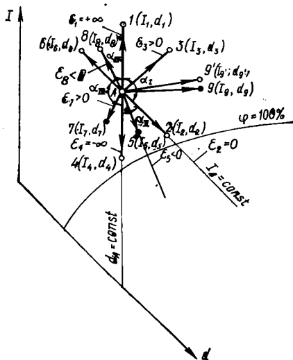
Рис. 11.8. Транспорт углового масштаба
