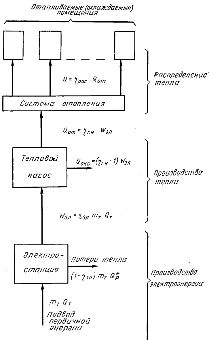
Рис. X.23. Структура термозкономического показателя по затратам первичного тепла в геотермальной установке с компрессионным тепловым насосом и электрическим приводом
