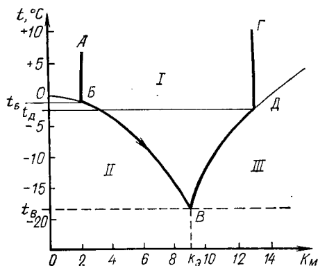
Рис. II.24. Диаграмма фазового состояния раствора
