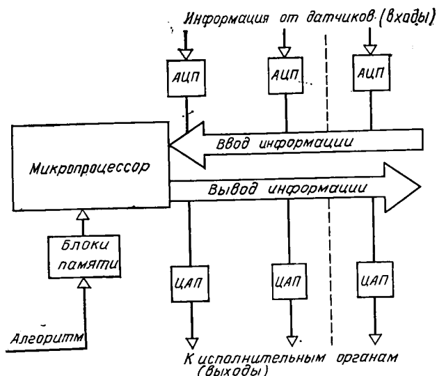
Рис. XI.17. Схема управления СКВ с помощью микропроцессора ЦАП — цифроаналоговые преобразователи; АЦП — аналого-цифровые преобразователи
