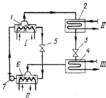
Рис. VIII.3. Абсорбционная холодильная машина
