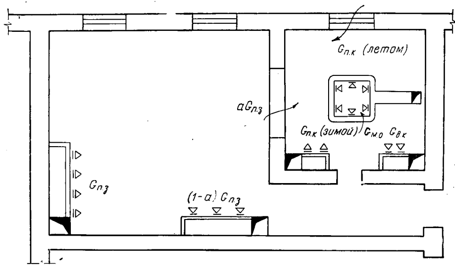
Рис. IV.31. Принципиальная схема организации воздухообмена в помещениях с различным характером выделения вредностей
