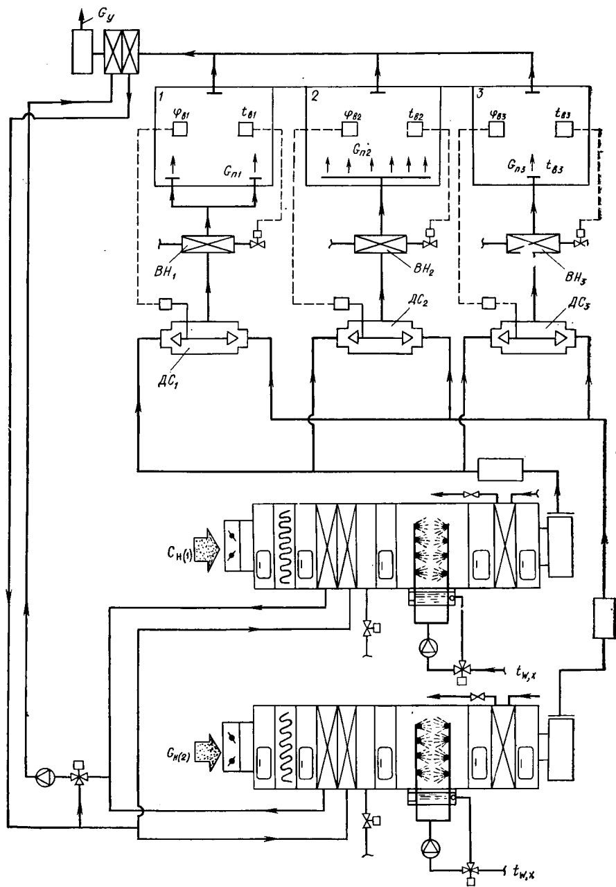
Рис. V.7. Многозональная СКВ с двумя параллельными центральными УКВ и последовательно установленными двухканальными смесителями ДС и воздухонагревателями ВН в каждой зоне
