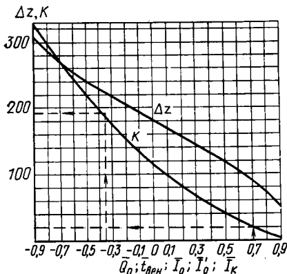
Рис. XI.13. Зависимость продолжительности периода потребления тепла или холода \Delta z и величины K от безразмерных величин \bar{Q}_n, t_{вн}, \bar{t}_o, \bar{t}_k
