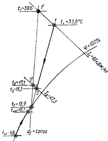
Рис. VI.13. I-d -диаграмма к расчету режима охлаждения и осушения воздуха в воздухоохладителях
