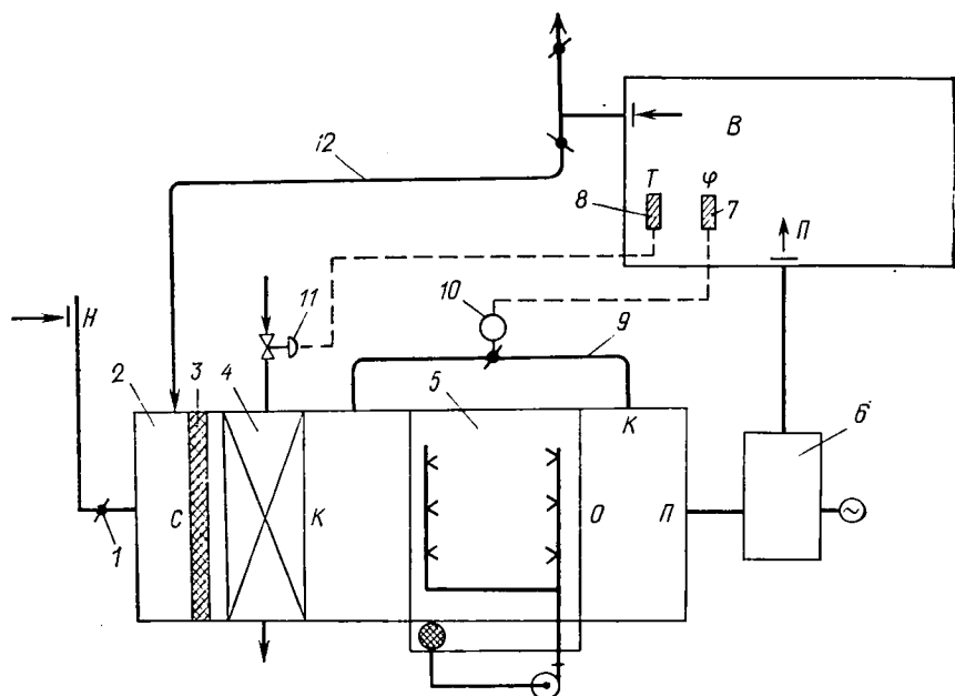
Рис. IV.23. Схема СКВ с использованием кондиционера системы двухступенчатого испарительного охлаждения для режима холодного периода 1, 10 и 11 — клапаны; 2 — смешительная камера; 3 — фильтр; 4 — теплообменник; 5 — камера орошения; 6 — вентилятор; 7 и 8 — датчики; 9 и 12 — каналы
