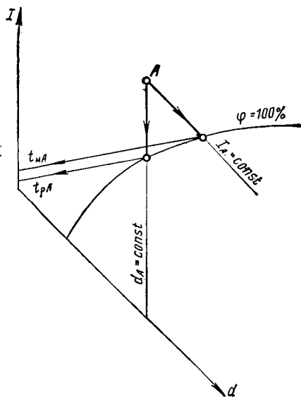
Рис. 11.3. К определению на I-d -диаграмме температур мокрого термометра t_{ма} и точки росы t_{ра} , соответствующих состоянию точки A
