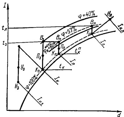
Рис. XI.12. I - d -диаграмма процессов обработки воздуха в СКВ
