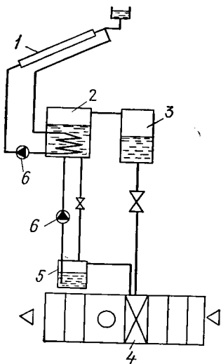
Рис. X.20. Схема солнечного абсорбционного охлаждения
