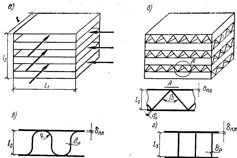
Рис. X.2. Схема устройства воздухо-воздушного рекуператора а — с гладкими пластинами; б — с треугольными пластинами; в — с U-образными пластинами; г — с П-образными пластинами
