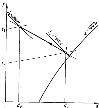
Рис. II.28. I - d -диаграмма с режимом адсорбции
