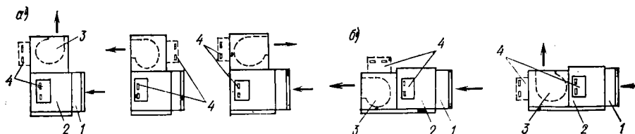
Рис. VII.1. Схемы неавтономных УКВ из стандартных блоков а — вертикальная; б — горизонтальная; 1 — фильтр; 2 — блок поверхностных теплообменников; 3 — вентиляторный блок; 4 — дверцы для осмотра и обслуживания
