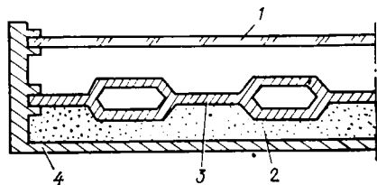
Рис. X.13. Конструкция солнечного коллектора ЭНИН им. Г. М. Кржижановского 1 — остекление; 2 — теплоизоляционный материал; 3 — абсорбционная пластина из стали; 4 — алюминиевый корпус
