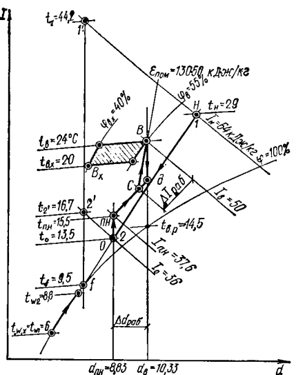
Рис. VI.17.1 — d -диаграмма к примеру расчета режимов обработки воздуха в эжекционной СКВ в теплый период
