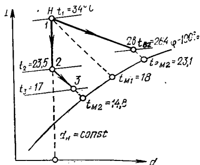
Рис. VII.6. l - d -диаграмма с режимом обработки воздуха в местном кондиционере двухступенчатого испарительного охлаждения
