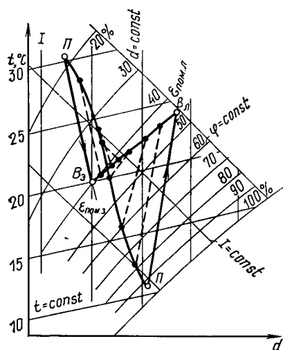
Рис. XI.6. Построение на I-d -диаграмме области возможных изменений положения луча процесса в помещении в течение года
