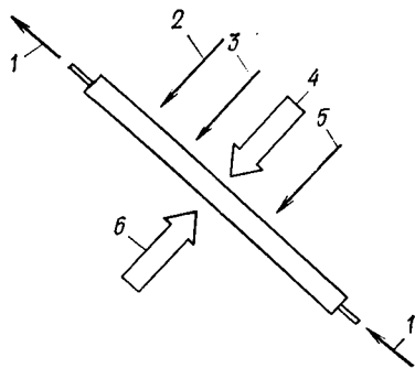
Рис. X.14. Составляющие теплового баланса абсорбционного гелиоприемника
