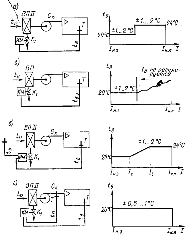
Рис. XI.9. Возможные схемы контура регулирования t_B в однозональной КВ
