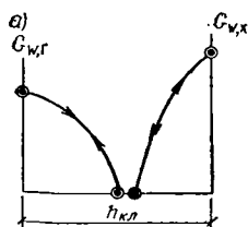
Рис. IX.11. Круглогодичное изменение расходов горячей и холодной воды (а) через трехпроходной автоматический клапан (б) 1 — термобаллон, воспринимающий температуру t_{в} ; 2 — настроенный сильфон; 3 — настроечная рукоятка; 4 — сильфон в установочной крышке, закрепленной на головке клапана; 5 — разделительный сильфон клапана; 6 — седло клапана изменения расхода холодной воды; 7 — шток клапана; 8 — трубопровод к теплообменнику ЭКД; 9 — седло клапана изменения расхода горячей воды; 10 — возвратная пружина штока; 11 — подающий трубопровод холодной воды; 12 — то же, горячей воды
