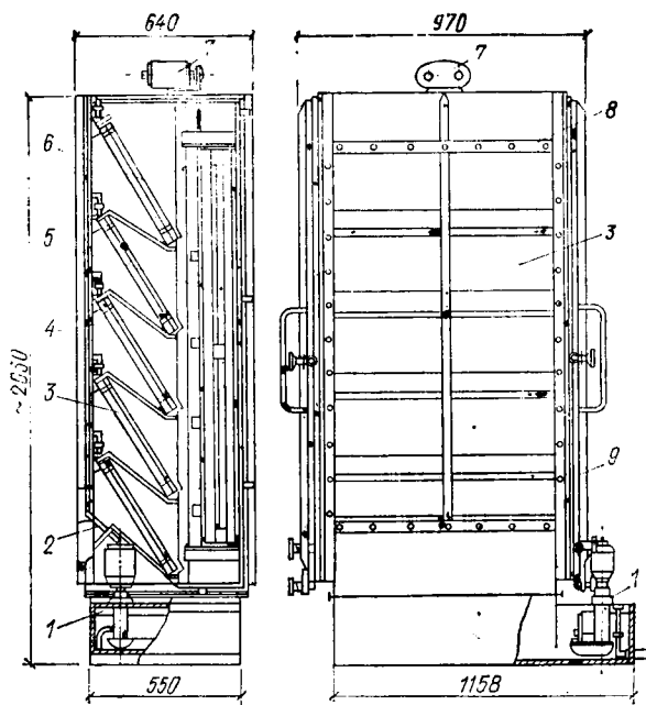
Рис. VIII.13. Секция аппарата адиабатного увлажнения в орошаемых кассетах
