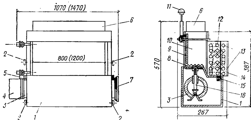
Рис. VI.16. Эжекционный кондиционер-доводчик КНЭ-У
