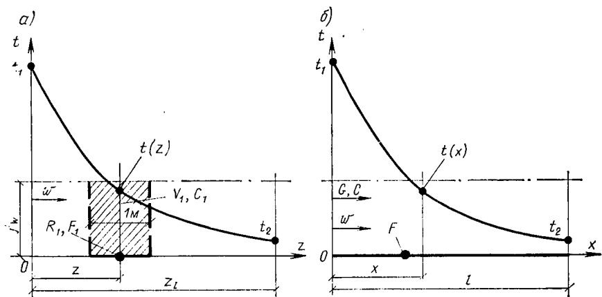
Рис. III.6. К определению обобщенной пространственной временной характеристики — модифицированного критерия Фурье ( Fo' ) а — в постановке Лагранжа; б — в постановке Эйлера
