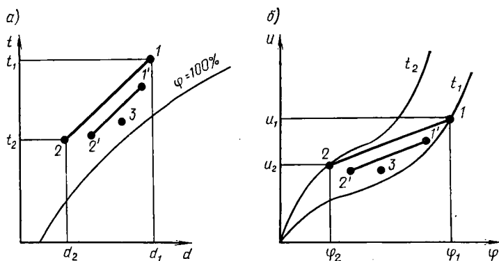
Рис. X.10. Процесс изменения тепловлажного состояния насадки регенератора а — изображение на t-d диаграмме; б — изображение на диаграмме изотермы сорбции
