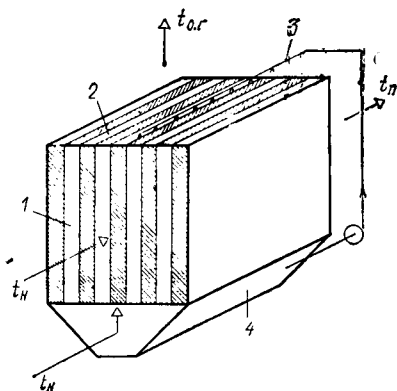
Рис. IV.7. Схема устройства совмещенного аппарата косвенного испарительного охлаждения 1, 2 — группы каналов; 3 — водораспределительное устройство; 4 — поддон
