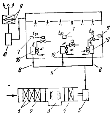
Рис. V.5. Местно-центральная СКВ 1-9 — см. рис. V.1; 10 — местный агрегат-доводчик для тепловой обработки внутреннего рециркуляционного воздуха
