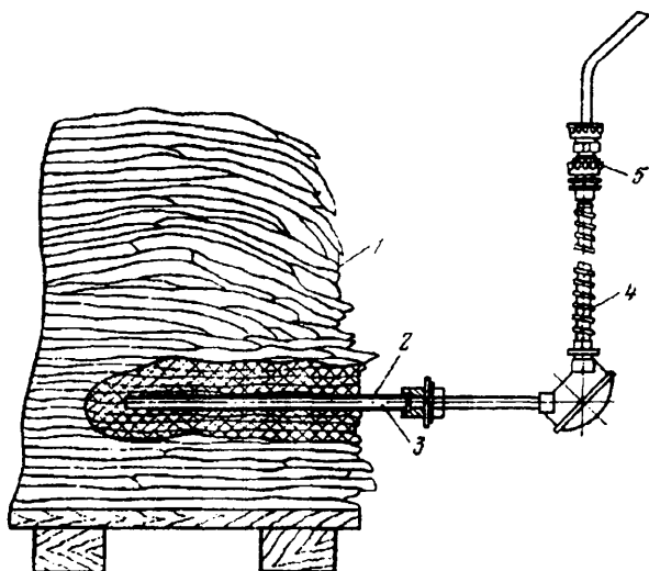
67-rasm. Qarshilik termometrini taxlovda joylashtirish tasviri: 1-taxlov; 2-himoyalovchi gilza; 3-qarshilik termometri; 4-shlangli chiqish yo'li; 5-shtepselli ajratma.
