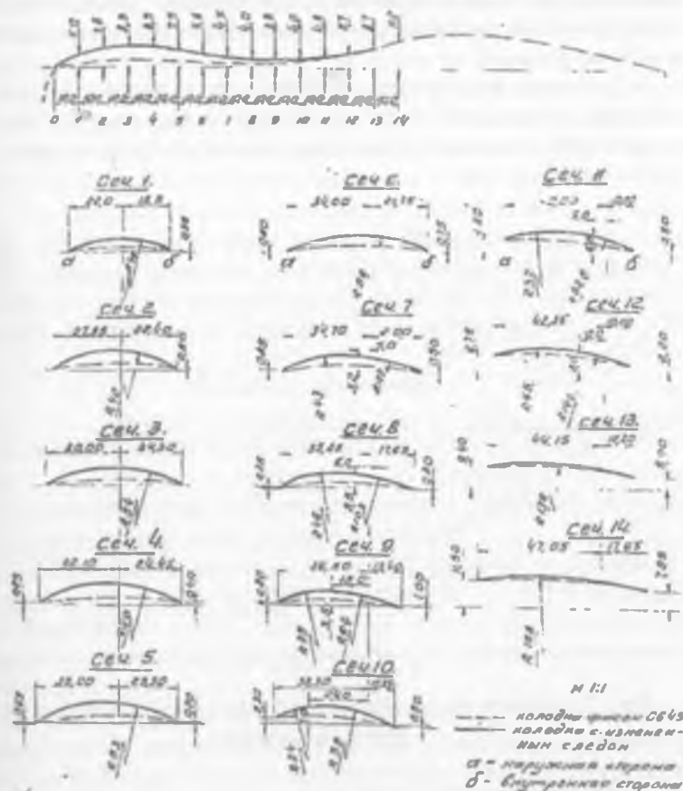
Рис. 1.4. Изменение формы следа калодки с высотой каблука 20 мм
