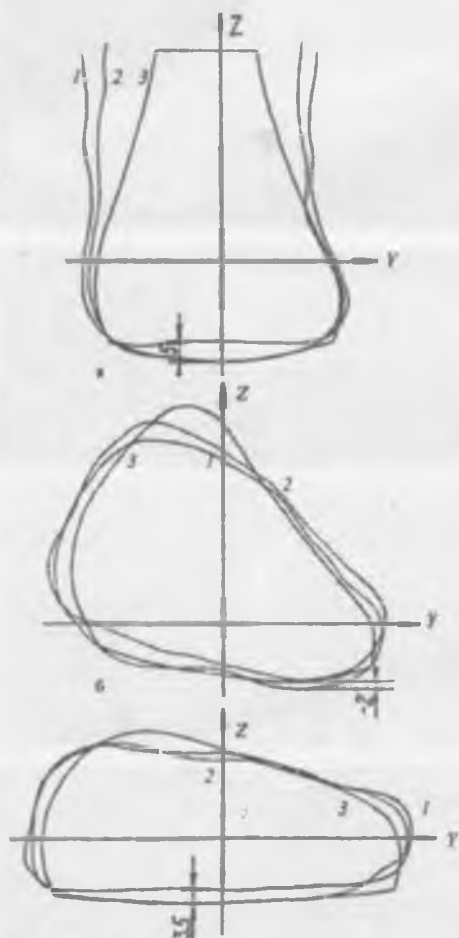
Рис.4.2. Построение контуров поперечно-вертикальных сечений калодки (Д-250) для женской обуви повышенной комфортности (а – сеч.0,18Д; б- сеч.0,5Д; в- сеч.0,73Д; 1-контур стопы в положении плоской опоры с плиткой, приподнятой на каблук; 2-контур стопы в положении опоры на мягкое основание; 3-контур калодки)
