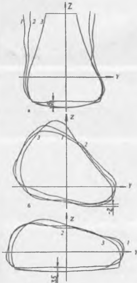
Рис.4.2. Построение контуров поперечно-вертикальных сечений калодки (Д-250) для женской обуви повышенной комфортности (а – сеч.0,18Д; б- сеч.0,5Д; в- сеч.0,73Д; 1-контур стопы в положении плоской опоры с пяткой, приподнятой на каблук; 2-контур стопы в положении опоры на мягкое основание; 3-контур калодки)
