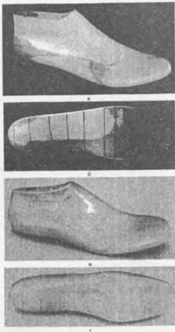
Рис. 4.3. Разработанные эталоны колодок для женской (а,б) и мужской (в,г) обуви повышенной комфортности (а,в-вид с наружной стороны; б,г-вид со стороны следа)
