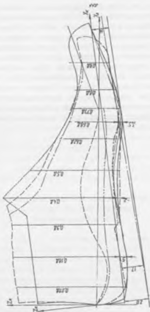
Рис.4.1. Построение продольно-осевого сечения калодки (Т-250) для женской обуви повышенной комфортности (—стопа в положении опоры на плоское основание с припнятой пяткой; —стопа в положении опоры на мягкое основание; ---калодка)
