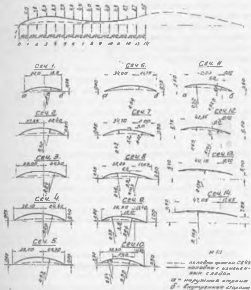
Рис. 1.4. Изменение формы следа колодки с высотой каблука 20 мм
