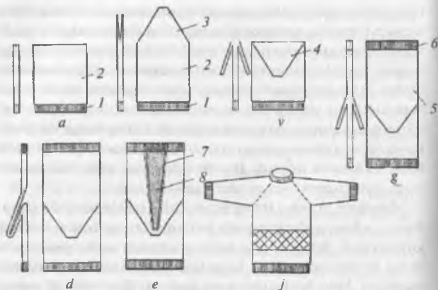
7.2-rasm. «Kometa FCM» mashinasida sviter to'qish sxemasi.
