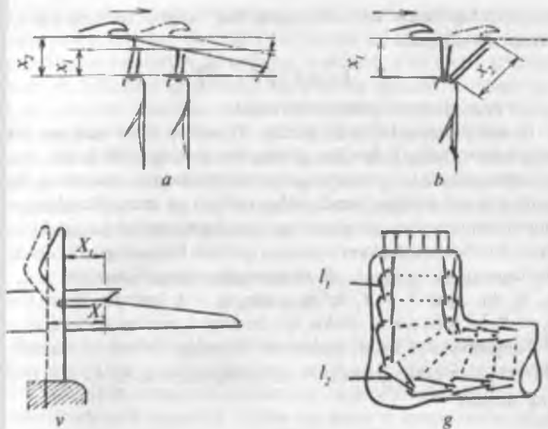
4.1-rasm. Ipning egilish chuqurligini o'zgarish jarayoni sxemasi.
