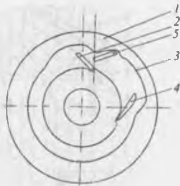
2.14-rasm. Ripshaybaning takomillashtirilgan qurilmasi.
