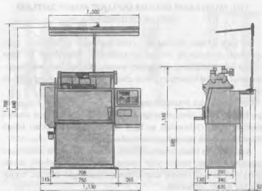
8.1-rasm. Qo'lqop to'quv avtomatining umumiy ko'rinishi.
