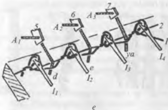
7.12-rasm (davomi): e — to'quv ignalarda 2-halqa qatorini hosil qilish jarayoni.
