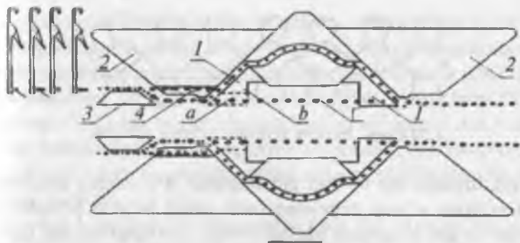
4.33-rasm. Halqa hosil qilish jarayonida kalta tovonchali ignalar harakat trayektoriyasi.
