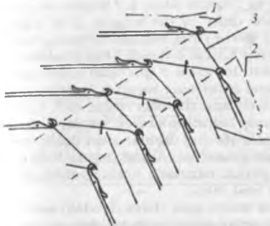
2.26-rasm. Dastlabki qatorni ribana o'rinishda ikkala ignadon ignalarida hosil etish usuli.
