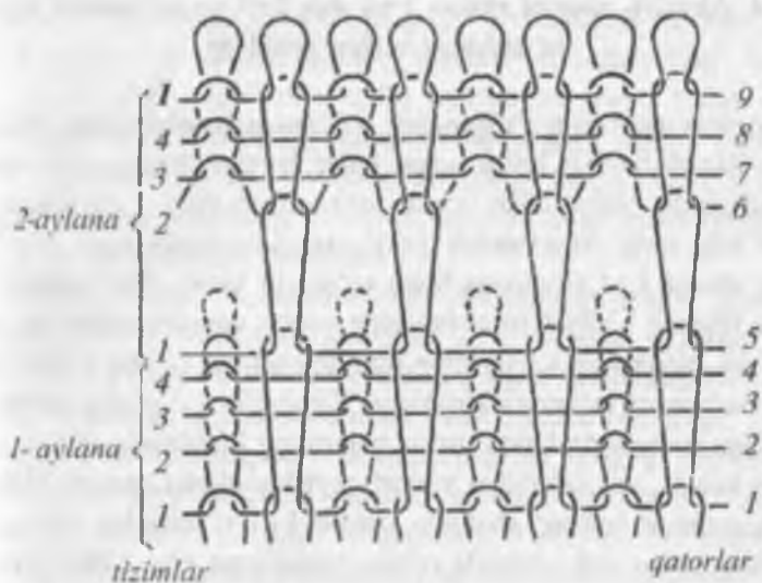
3.5-rasm. To'rt to'quv tizimli mashinada hosil qilingan ajratish qismning tuzilishi.
