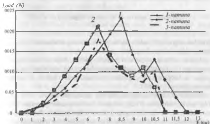
4.28-rasm. Bitta ipdan shakllantirilgan arqoqli trikotajdagi arqoq ipining so'tilishidagi birikish mustahkamligi ipning chiziqli zichligiga bog'liqlik grafigi.
