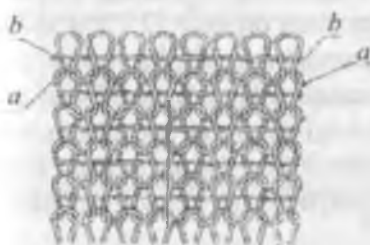
4.26-rasm. Arqoqli trikotaj mato: «a-a» — halqalarni tashkil etuvchi asos ipi; «b-b» — arqoq ipi.
