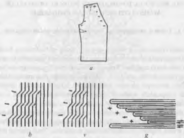
7.1-rasm. Jaketning old qismida (polochka) zaxirali chok hosil qilish sxemasi.
