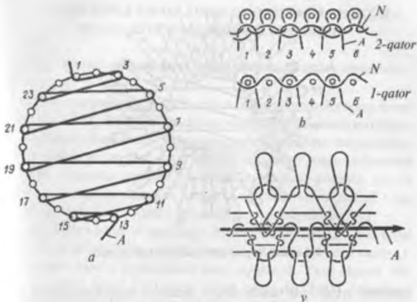
6.3-rasm. Paypoqning yopiq uch qismini birlashtiruvchi ip bilan hosil qilish sxemasi.
