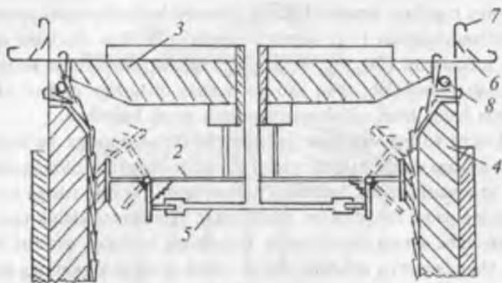
3.13-rasm. Aylana ignadonli to'quv mashinasida mahsulot qismlarini ajratuvchi qatorsiz to'qish sxemasi.
