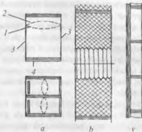
9.2-rasm. Tanda o'rilishli, donali maishiy trikotajlar tuzilish sxemalari.
