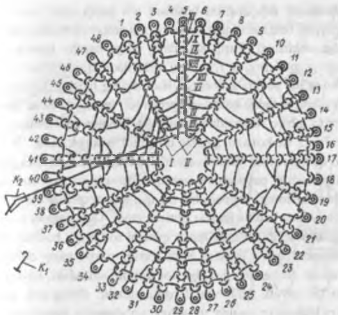
6.2-rasm. Ignalar sonini o'zgartirib to'qiladigan yopiq uch qismining tuzilishi.
