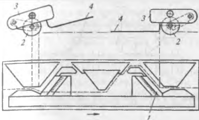
2.27-rasm. Halqa qatorlarini ignadon oralig'iga yo'naltiruvchi (tortuvchi) chiviqli qurilma tuzilishi.
