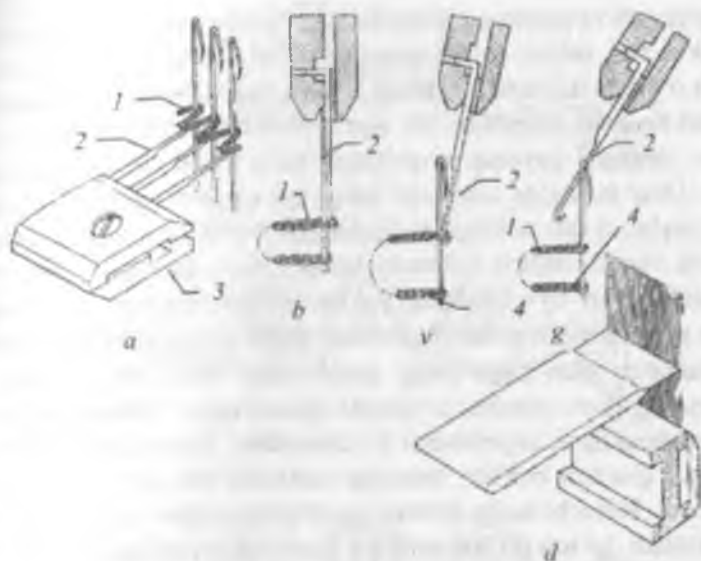
2.4-rasm. Koton mashinasida mahsulotning quyi bort qismining boshlang'ich qatorini hosil qilish sxemasi.
