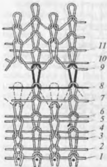
3.3-rasm Ikki qatorli suprem o'rinishli to'qima bilan mustahkamlangan ajratish qismining tuzilishi.
