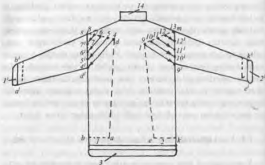
7.8-rasm. Yassi fang avtomatida jempelni bir yo'la to'qish sxemasi.
