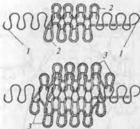
2.33-rasm. Yassi ignadonli qo'lqop to'quv avtomatda boshlang'ich halqa qatorlarini to'qish sxemasi.
