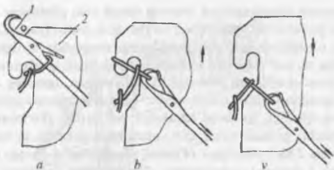
2.32-rasm. Yassi ignadonli fang qo'lqop to'qiydigan avtomatlarda boshlang'ich halqa qatorlarini platinalar bilan hosil qilish sxemasi.
