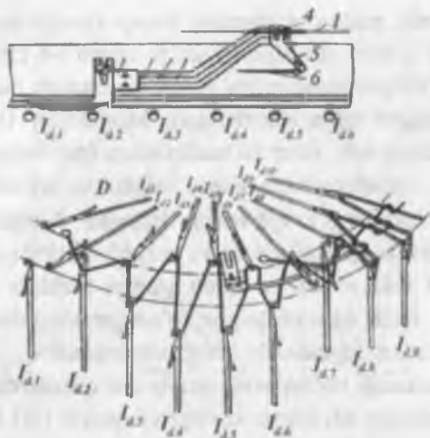
3.12-rasm. Kuponning dastlabki qatorini ribana 1+1 o'rilishida avtomatik hosil qilish.
