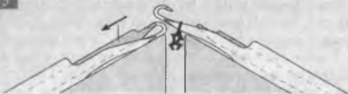
4.23-v-rasm. Tarnovsimon o'yiqli igna bilan jihozlangan fang mashinasida halqa ko'chirish jarayoni ketma-ketligi.
