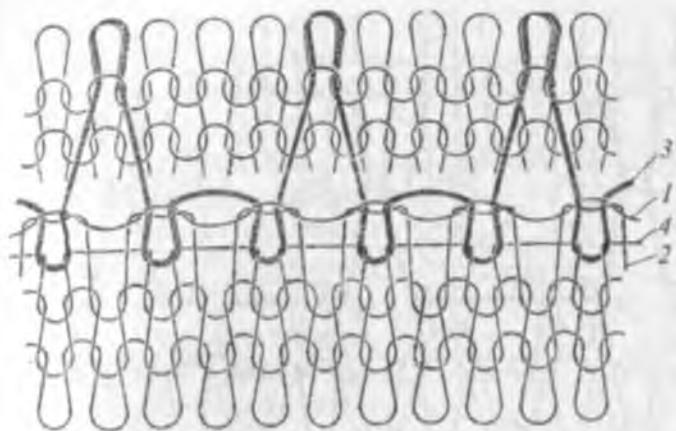
2.18-rasm. Aylana ignadonli paypoq to'quv avtomatida to'qilgan paypoq bortini birlashtiruvchi chokining yangi tuzilishi, paypoq bortini yopchiqli halqalar bilan birlashtirib to'qilgan tuzilishi.
