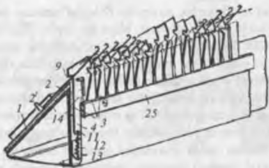
2.31-rasm. Platinalar bilan jihozlangan yassi ignadonli fang avtomatining ignadon tuzilishi.
