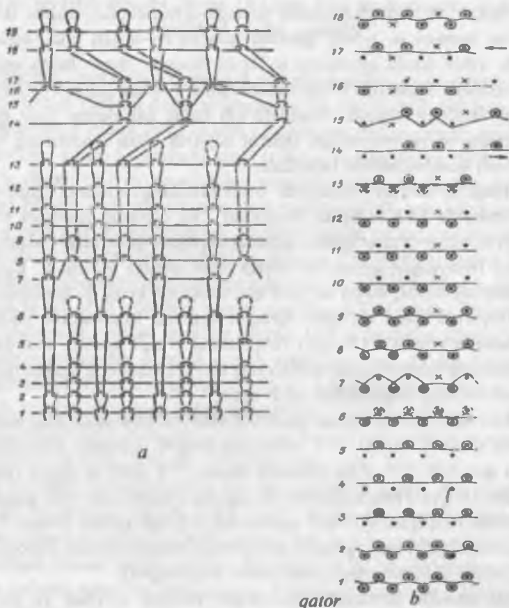
3.6-rasm. Ikki ignadonli mashinalarda dastlabki qatomi ribana 2+2 asosida ishlay boshlashda qo'llaniladigan ajratuvchi qator tuzilishi va grafik yozuvi.
