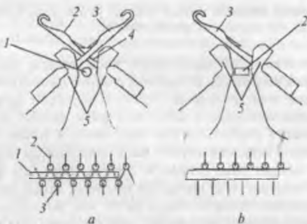
2.29-rasm. Chiviqni halqalarga ta'sir etish sxemasi.
