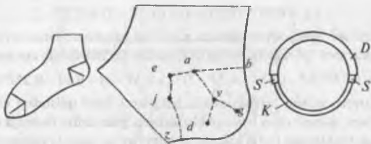
5.7-rasm. Paypoqning murakkab shaklli tovonining kichraytirilgan qismi va uni to'qiydigan ignalarning joylashuvi.
