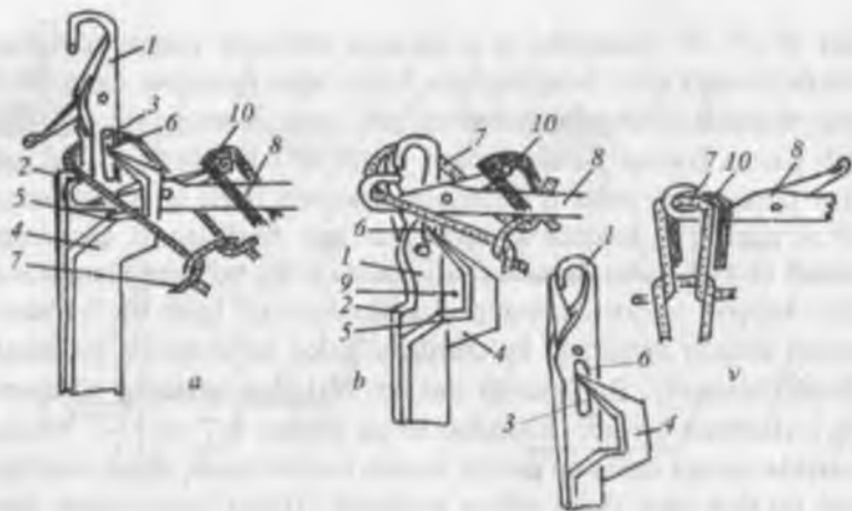
4.21a,b,v-rasm. Kengaytiruvchisi bo'lgan tilchali ignalarda halqa ko'chirish jarayoni.
