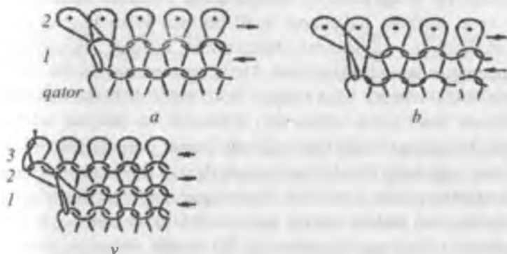
4.10-rasm. Halqalarni qo'shish va qo'shilgan ignalarga halqaning yarim yoyini kiygizish usuli bilan hosil qilingan gardish tuzilishi.
