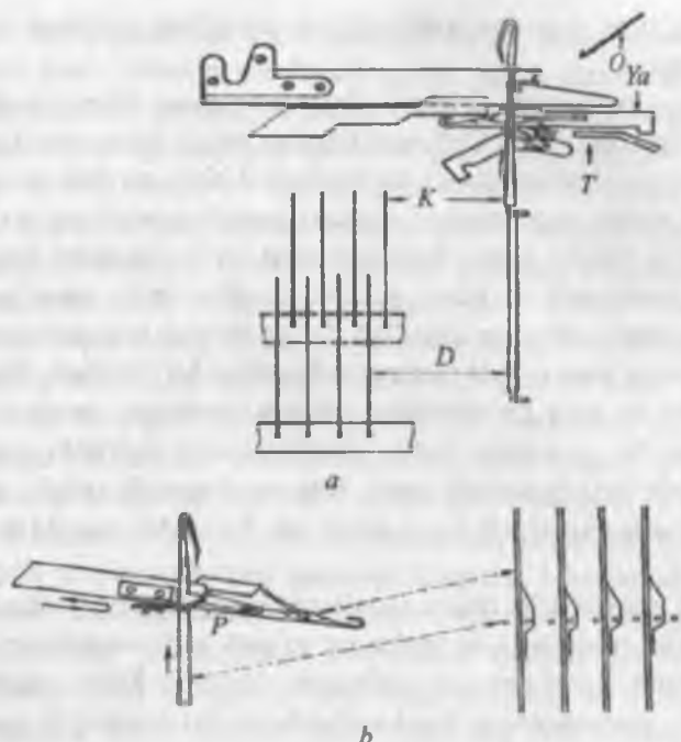
2.37-rasm. Koton mashinalarida tilchali ignalardan ilgakli ignalarga halqalarni ko'chirish va mahsulot ishlay boshlash qismini avtomatik hosil qilish sxemasi.
