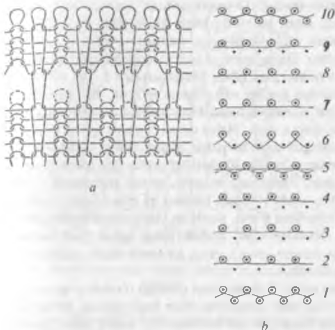
3.1-rasm. Ajratish qismining tuzilishi va grafik yozuvi.
