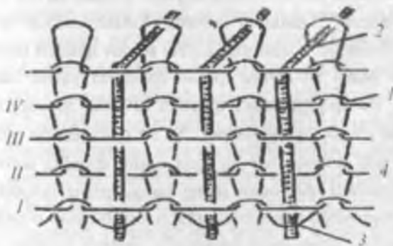
7.11-rasm. Arqoqli o'rigan to'qima tuzilishi.
