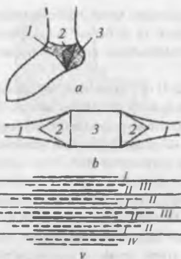
5.11-rasm Ignadonning bir tomonlama aylanishida to'liqmas halqa qatorlarini to'qib hosil etilgan tovon qismi.
