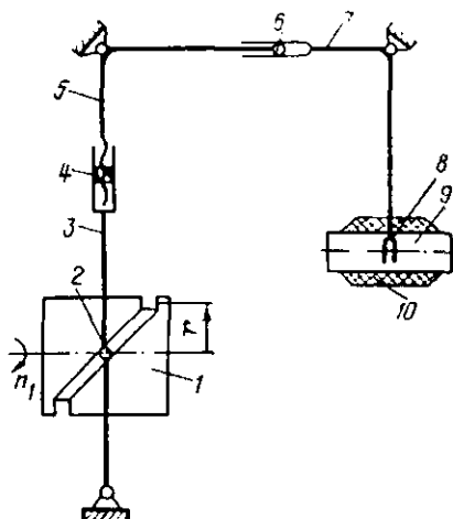
2.8- rasm. Ipkashlik bobinalash mashinasi yotqizish mexanizmi:
