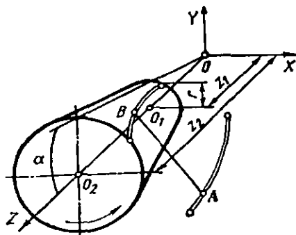
4.6-rasm. Kesik konusga o'rashdagi umumiy hol sxemasi.
