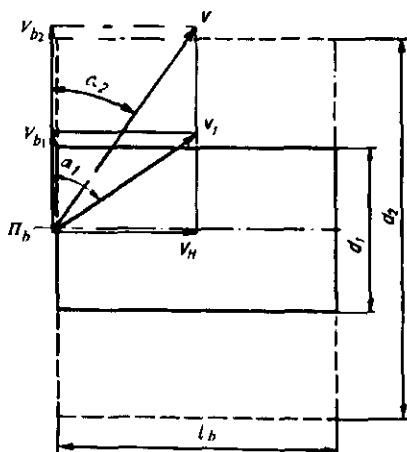
10.4-rasm. Joylama o'qi orqali yuritilgandagi kinematik ko'rsatkichlar sxemasi:
