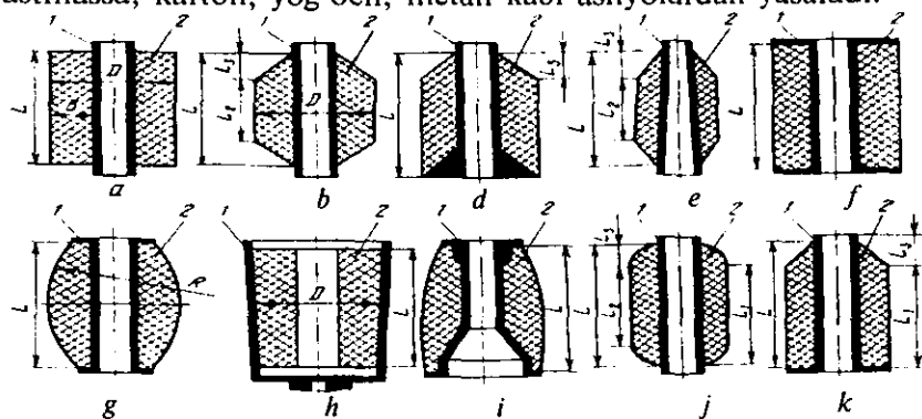
2.1 rasm. Ipbardorlar va joylamalar shakllari.
