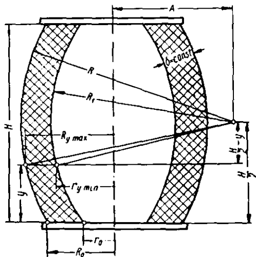
3.11- rasm. Sferik jismga nimqavat qalinligi o'zgaras o'rash sxemasi.
