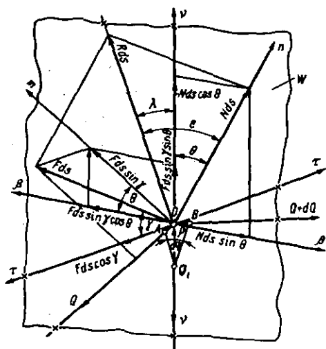
7.1- rasm. O'ralayotgan ipning muvozanatvor joylashuv shartlarini chiqarishga doir sxema.
