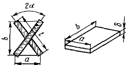
8.5-rasm. Qiya kesishuvli oʻralish elementi.
