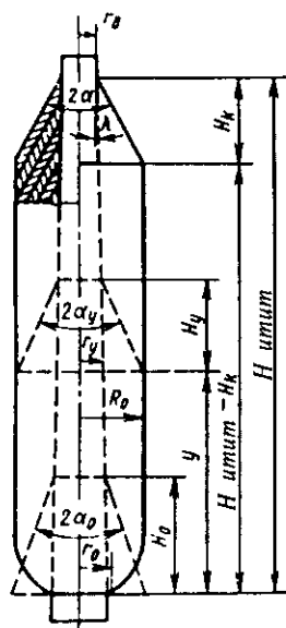
16.9- rasm. So'ta o'ralishini hisoblash sxemasi.
