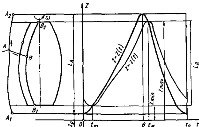
5.1-rasm. Ipyotqizish va o'rash nuqtalarining harakat qonuniyatlari tahliliy ko'rinishi sxemasi.
