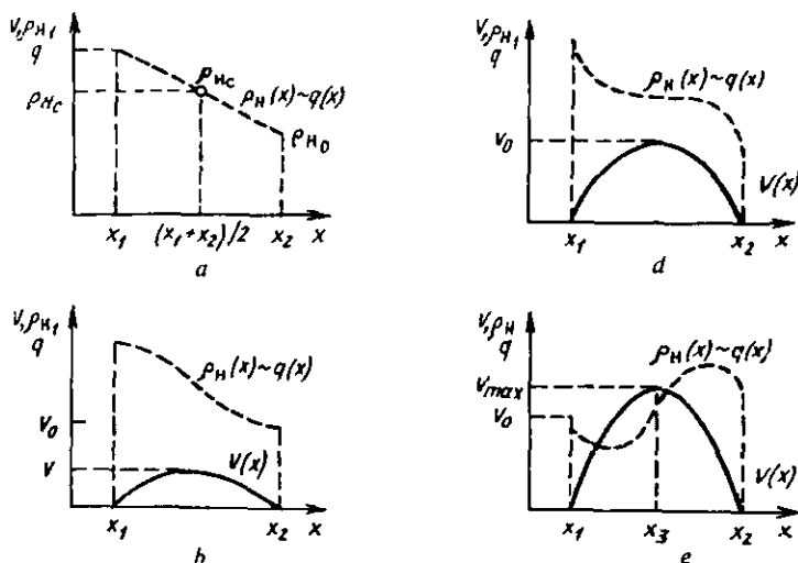
8.9- rasm. Tayyor joylamada zichlik egrilanmalari.
