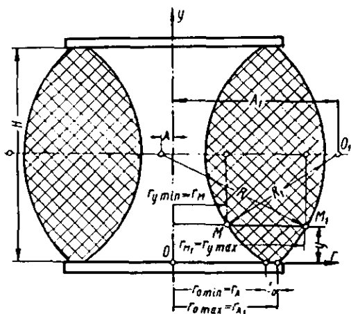
3.10- rasm. Egarsimon g'altakka o'rash sxemasi.
