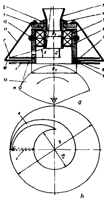
2.11- rasmda. Doiraviy harakatli ipyetaklagichli inersiyasiz yotqizish mexanizmi.
