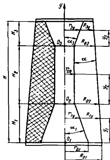
5.4-rasm. O'rash nuqtasining boshlang'ich tezligini aniqlashga doir sxema.
