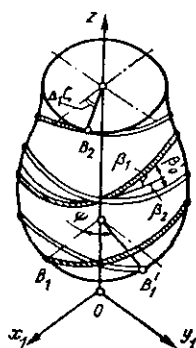
6.3- rasm. O'ramlarning kesishuv \beta_0 va siljish \psi burchaklari sxemasi.
