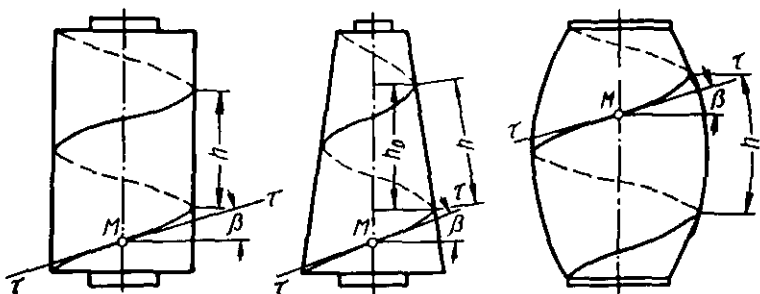
3.3- rasm. O'ramlarning qadami va ko'tarilish burchagi.
