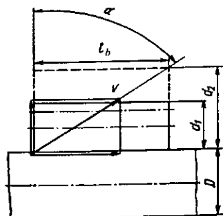
10.1-rasm. Joylamani urinmaviy aylantirish grafigi.
