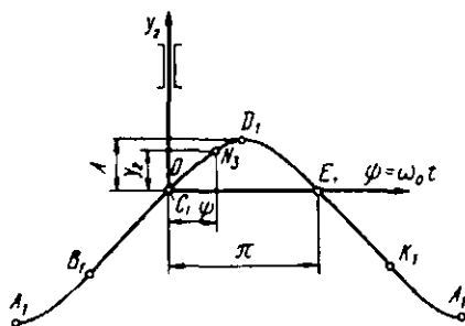
14.7- rasm. Ariqchasining vintli chiziqlari sinusoidal tutashgan silindrik mushtchanning markazlar chizig'ining yoyilmasi.
