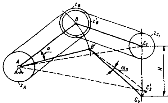
17.5-rasm. Differensialdan g'altaklarga zanjirli uzatma chizilmasi.
