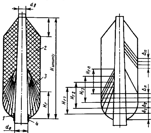
16.1-rasm. So'taning tuzilish sxemasi.
