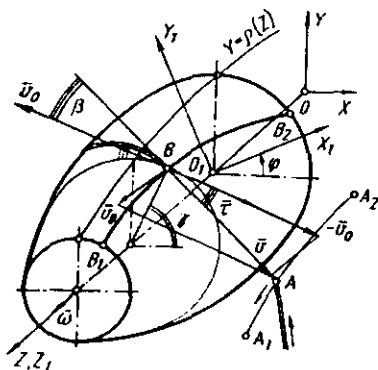
4.1-rasm. Ipni joylamaga o'rash jarayoni.
