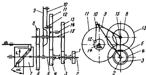
18.2- rasm. Differensial uzatmali krivoship-shatunli tarqoqlantirish qurilmasi sxemasi.
