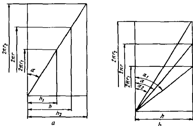
8.6- rasm. Turli qavatlardagi o'ramlar yoyilmalari grafiklari:
