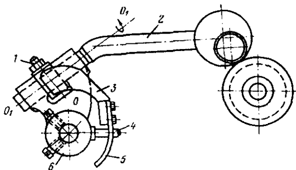
12.8- rasm. Yumaloqlashtirgichning tuzilishi.
