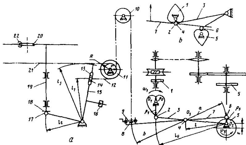
2.7- rasm. Ikki mushtchali ipyotqizish mexanizmlari:
