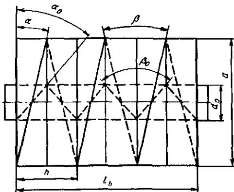
10.5-rasm. Kesishuvli pretsizion o'ralish sxemasi:
