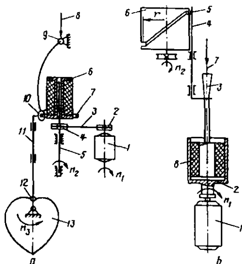
2.5 rasm. O'rash va yotqizish mexanizmlari:
