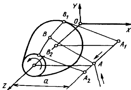
4.2-rasm. Yotqizish nuqtasining joylama o'qiga parallel to'g'ri chiziq bo'ylab harakati sxemasi.
