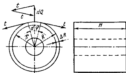
8.1- rasm. Joylamada bosim hosil bo'lish sxemasi.
