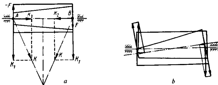
12.4- rasm. Bobina va yurgizuvchi barabanchaning nisbiy joylashuv sxemalari.
