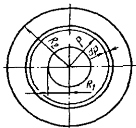
8.2- rasm. Joylamaning elementar halqaviy qatlamli kesim sxemasi.
