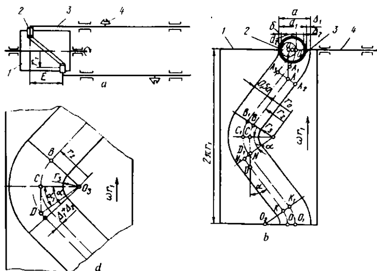
14.8-rasm. Silindrik mushtakli yotqizish mexanizmi sxemasi:
