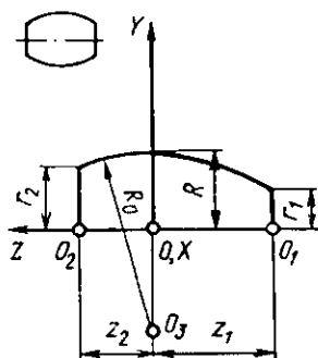
4.10-rasm. Sferoid shaklli joylama sxemasi.
