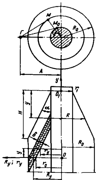
5.3-rasm. O'rash nuqtasining burchak siljishini aniqlash sxemasi.
