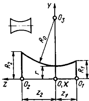
4.11-rasm. Egarsimon shaklli joylama sxemasi.
