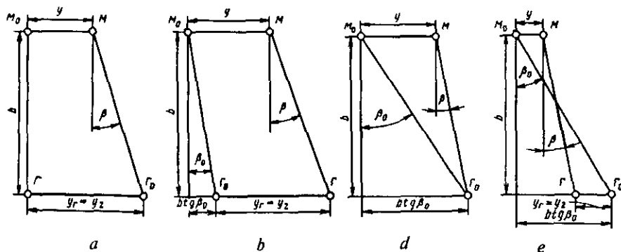
5.5-rasm. O'rash nuqtasi ko'rsatkichlarini aniqlash chizilmasi:
