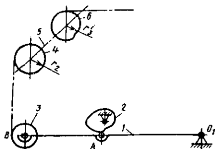
16.11- rasm. Shakldor g'altakcha o'lamini hisoblash sxemasi:
