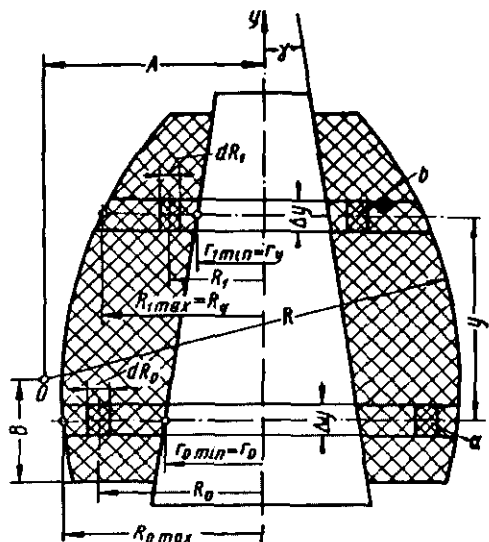
3.6- rasm. O'rash jismi shakli murakkab bo'lganda o'rashning tenglamasini chiqarishga oid sxema.
