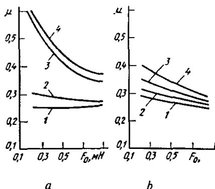
9.2-rasm. Ishqalanish yuzasidan oldindagi ip tarangligi F_0 va ishqalanish ko'effitsiyenti \mu orasidagi bog'lanish grafiklari.
