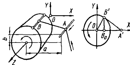
4.4-rasm. Yotqizish chizig'i joylama aylanish o'qiga parallel bo'lganida silindrik o'rash sxemasi.
