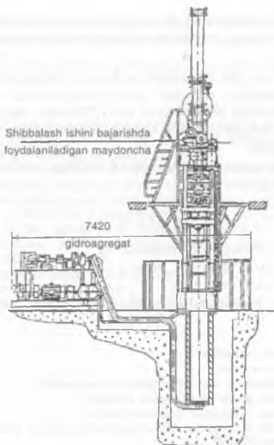
1.27-rasm. Paxta tolasi va lintni toyash uchun mo'ljallangan gidravlik bosgichning tuzilishi.
