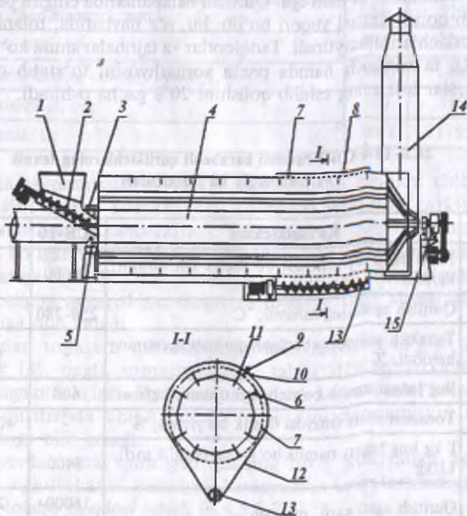
7.2- rasm. CBO rusumli barabanli quritkich sxemasi.
