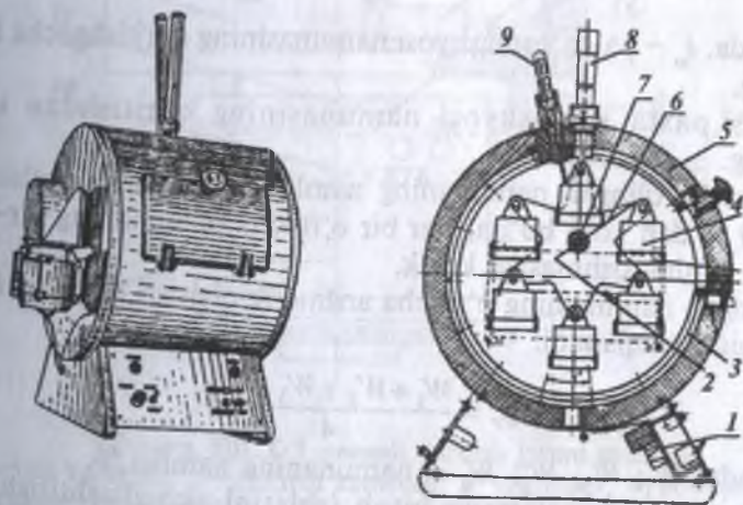
9.1-rasm. Y3-7M rusumli quritish shkafi: 1-boshqarish pulti; 2-termoelement; 3-o'rmatgich; 4-byuksa; 5-korpus; 6-yulduzcha; 7-val; 8-kontakt termometri; 9-nazorat termometri.
