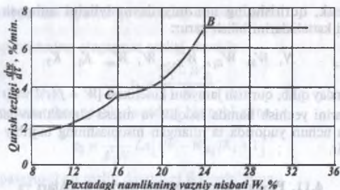
4.8- rasm. v_A = 1 m/s va t = 120^\circ\text{C} da paxta xomashyosining quritish tezligi egri chizig'i.
