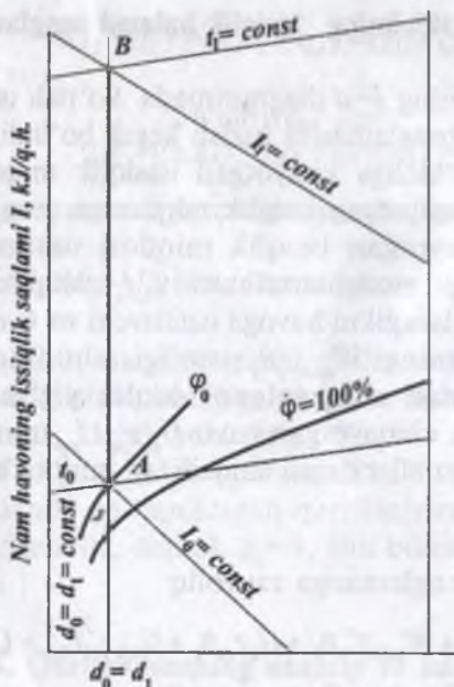
5.3-rasm. Issiqlik o'txonasida havoni qizish jarayonining I - d diagrammadagi tasviri.
