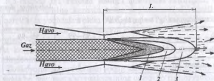
8.7-rasm. Gazli yoqilg'ilarning alanga olishi: L —yonish uzunligi; 1—aralashtirish zonasi; 2—qizdirish va bug'lanish zonasi; 3—alanganish zonasi.
