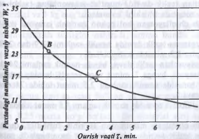
4.7-rasm. \vartheta_h = 1 m/s va t = 120^\circ\text{C} da paxta xomashyosining quritish egri chizig'i.
