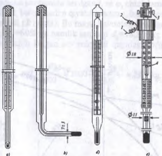
2.8-rasm. Termometrlar.
