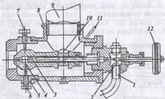
8.8-rasm. Past bosimli forsunka sxemasi: 1—yoqilg'io'tkazgich; 2—mazut uzatkichning tartibga soluvchi igna; 3—mazut soplosining qo'zg'almas trubkasi; 4—qo'zg'aluvchan soplo; 5—uchlik; 6,7—markazlashtirilgan bintlar; 8—korpus; 9—havo o'tkazgich; 10—mazut soplosining eksentrigi; 11—eksentrik dastasi; 12—mazut uzatkichning sozlash maxovigi.
