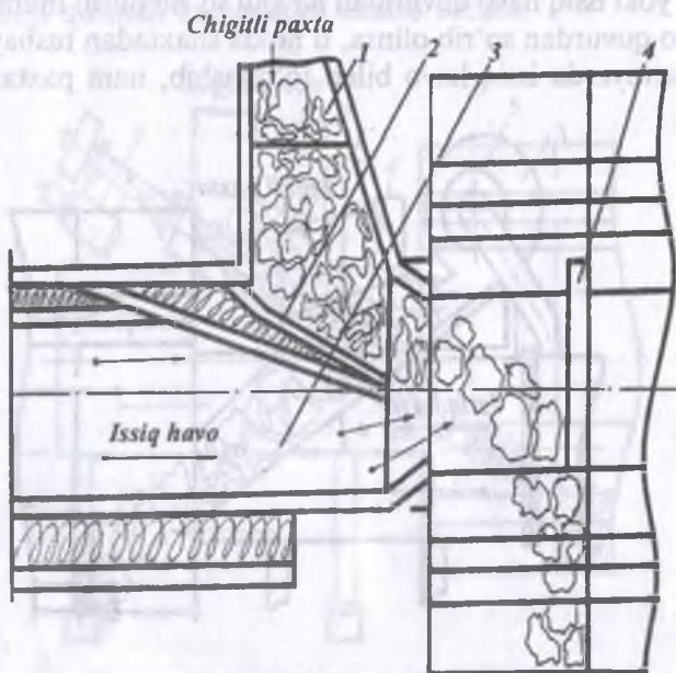
7.5-rasm. Lotokli ta'minlagich sxemasi:
