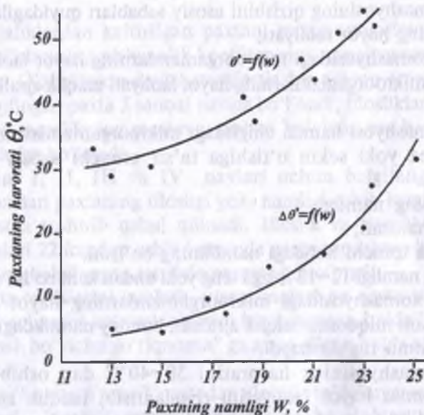
6.5-rasm. Paxta yuzasidagi haroratning ko'tarilishini namligiga bog'liqligi.
