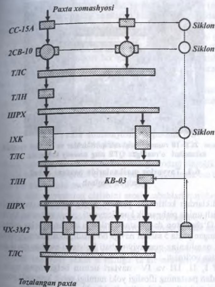
6.3- rasm. 2CB-10, IXK va CHX-3M2 rusumli uskunalari o'rnatilgan QTБning texnologik jarayon sxemasi.
