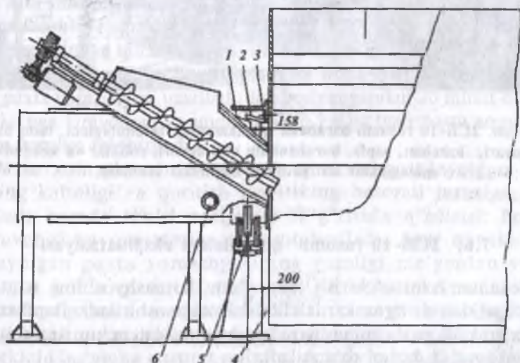
7.8-rasm. 2СБ-10 rusumli quritkichning ta'minlagichi sxemasi:
