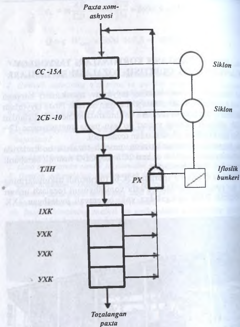
6.2- rasm. 2CB-10, IXK va YKK rusumli uskunalar o'rnatilgan QTBning texnologik jarayon sxemasi.
