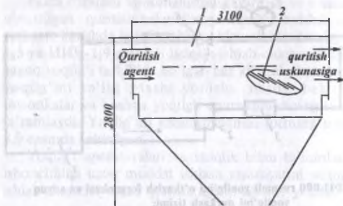
8.11-rasm. Quritish agenti bilan qo'shilib kelayotgan yong'in chiqaruvchi uchqunlarni ushlab qoluvchi ППХ 05.150 rusumli qurilma: 1-ishchi kamera; 2-pog'onasimon jalyuzali qobirg'alar.
