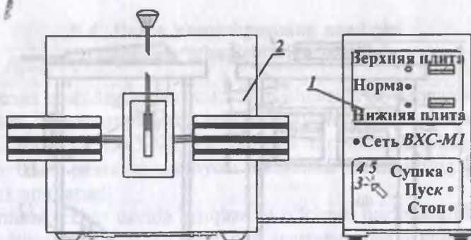
9.4-rasm. BXC-1M rusumli termonamo'lgachichning chizmasi: 1—boshqaruv pulti; 2—quritish kamerasi.
