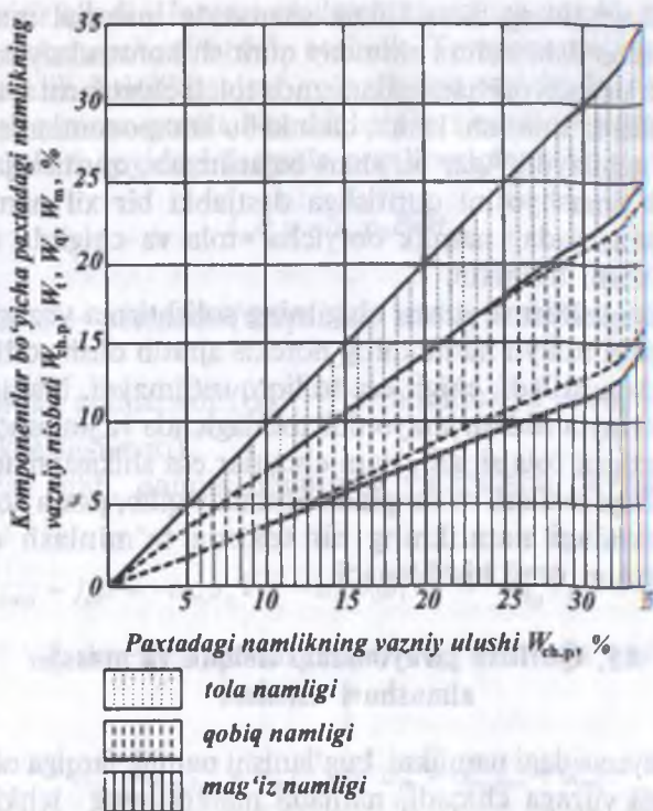
4.5-rasm. Namlikning paxta xomashyosi komponentlari bo'yicha taqsimlanishi.
