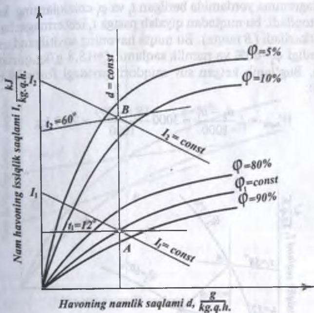
2.5-rasm. Havoning I - d diagrammasi bo'yicha qizdirilgandagi parametri.
