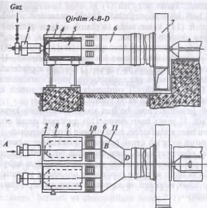
8.1-rasm. TT-1.5 rusumli issiqlik ishlab chiqargich sxemasi:
