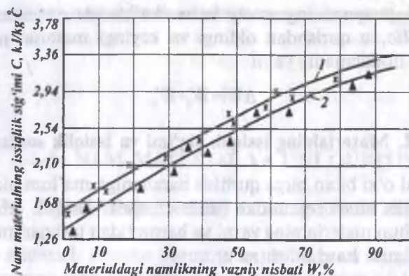
3.1-rasm. Paxtaning issiqlik sig'imini namlikga bog'liqlik grafigi.
