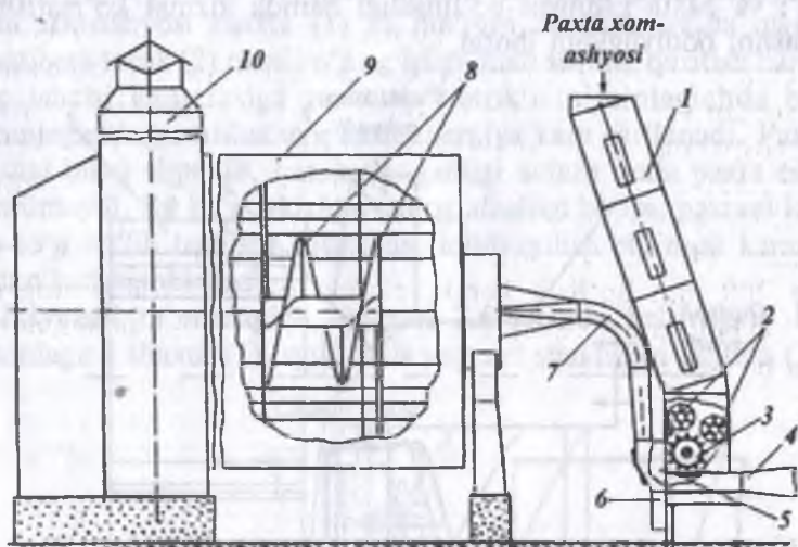
7.7-rasm. Tituvchi qismli va to'plovchi sig'imli PPC rusumli quritkich ta'minlagichi:
