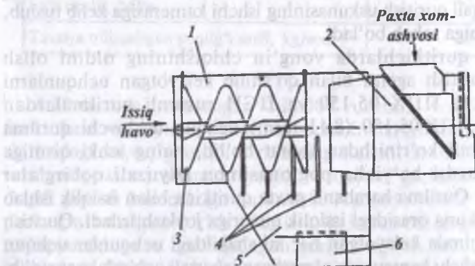
8.12-rasm. ПСИ rusumli uchqun ushlagich - ta'minlagich: 1-uchqun ushlagich; 2-ta'minlagich qismi; 3-shnekli aylantirgich; 4-panjarali qobirg'alar; 5-qattiq jisimlarni yig'uvchi shaxta; 6-qopqoq.
