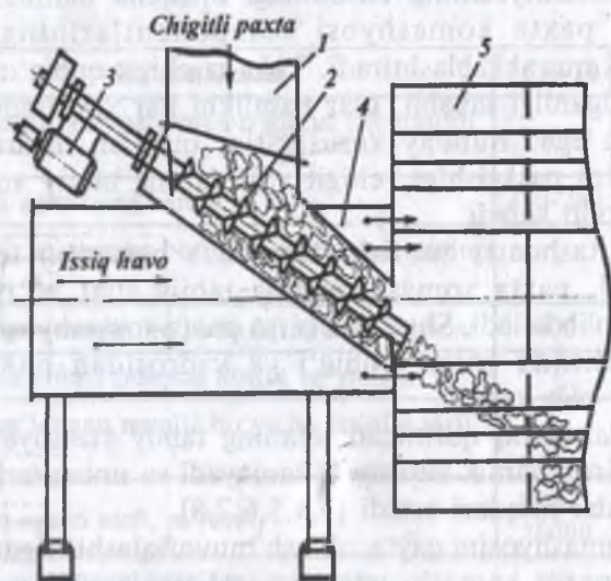
7.3-rasm. Shnekli ta'minlagich sxemasi:
