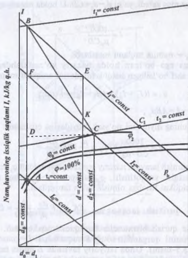
5.5- rasm. Haqiqiy quritish jarayonining I-d diagrammadagi tasviri.
