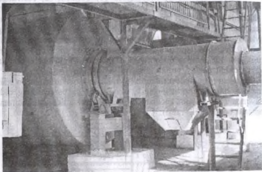
7.9-rasm. 2CB-10 rusumli barabanli quritkichning ta'minlagichi, issiq havo quvuri, baraban, sapfa, barabanning oldi devori, roliklar va uchqun ushlagichlar ko'rsatilgan majmuasi sxemasi.
