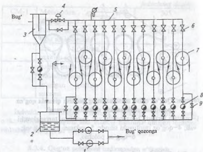
45-rasm. Qog'oz qilish mashinasi quritish qismini parallel usulda par bilan ta'minlash va kondensatini chiqarish sxemasi:
