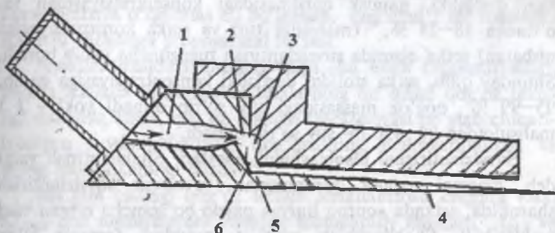
22-rasm. Yuqori konsentratsiyali massa uchun napusk qurilmasining sxemasi:
