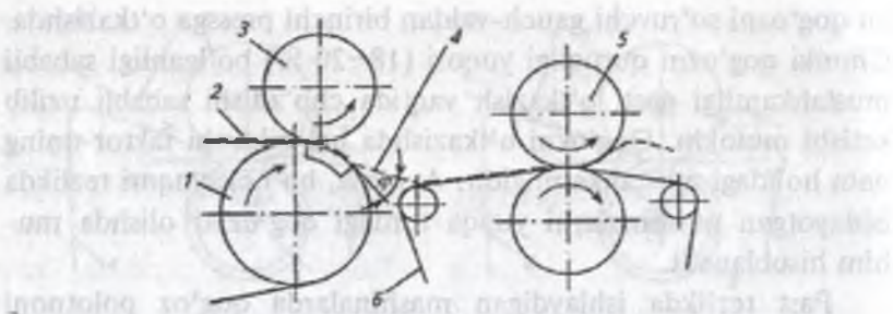
35-rasm. Qog'oz polotnini presslash qismiga uzatishning odatdagi usuli:
