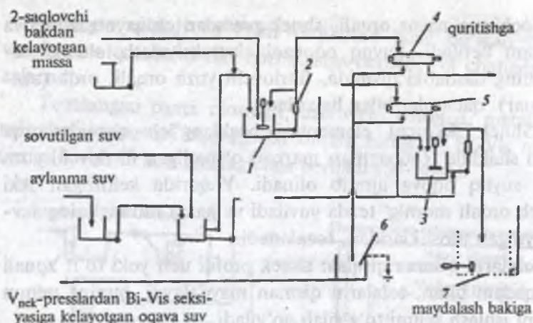
51-rasm. Massani shnek — pressdan keyin suyultirish seksiyasi:
