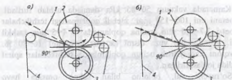
34-rasm. Jelobli pressga qog'oz polotnoni uzatish sxemasi:
