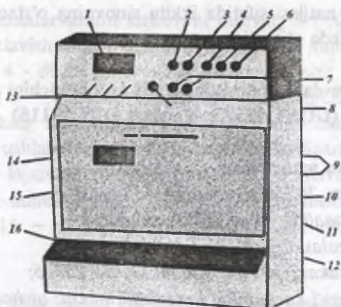
74-rasm. Qog'ozning g'ovakligini va silliqqligini aniqlovchi Bentdsen pribori:
