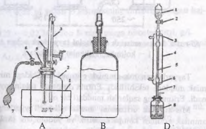
64-rasm. A. Avtomat byuretkali qurilma:
