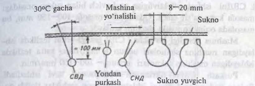
38-rasm. Presslovchi suknoni konditsionirlash elementlarining joylashish sistemalari.
