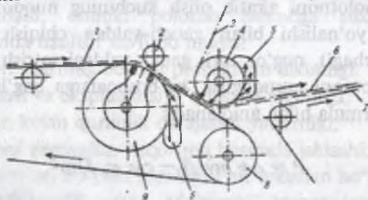
36-rasm. Vakuu orqali so'rib oluvchi qurilmada setkani burish vali:
