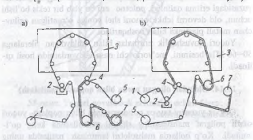
59-rasm. Laminlash sxemasi: a - quruq; b - ho'l:
