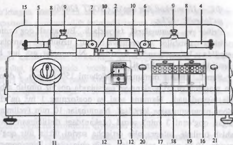
72-rasm. Qog'ozning ikki tomonga bukilishga chidamliligini aniqlaydigan pribor:
