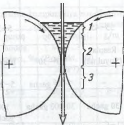
54-rasm. Qog'oz polotnining yelimlovchi press ishchi vallari orasidan o'tish sxemasi:
