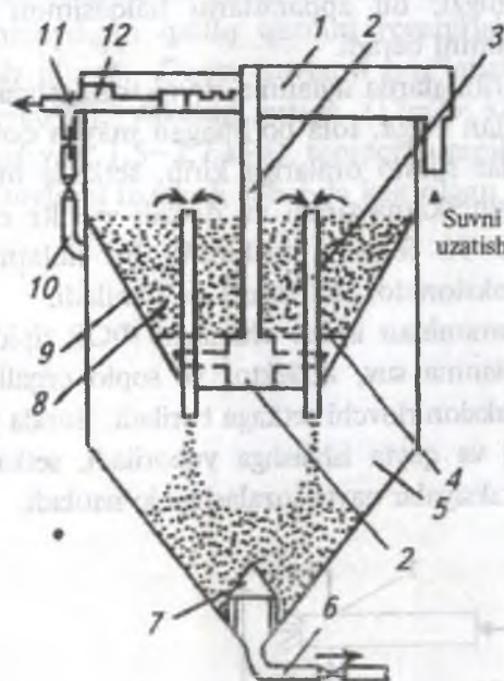
1—havoajratgich; 2—boʻluvchi qurilma; 3—shlam ajratib yoʻnaltiruvchi truba; 4—koʻp teshikli tag (dno); 5—korpus; 6—choʻkma chiqargich; 7—konusli shitcha; 8—choʻkmaning osma qismi; 9—chashkasimon germetik tag; 10—suvni chiqaruvchi trubalar sistemasi; 11—tindirilgan suvni chiqargich; 12—yigʻuvchi jeloba.
