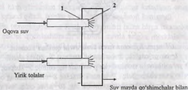
62-rasm. Struyali fraksionatorning ishlash sxemasi:
