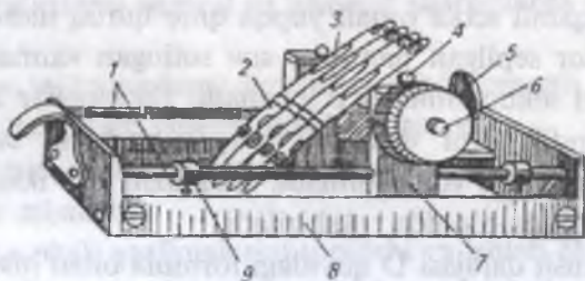
10-rasm. Qog'ozning yelimlash darajasini aniqlashda qo'llaniladigan ИПБ pribori:
