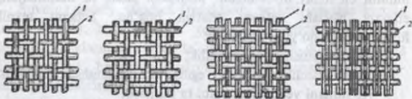
25-rasm. To'qilgan setkalar turi: a – bittalik setka (Inyanli to'qilma); b – bittalik setka ( yarimsarjlik to'qilma); d – ikkitalik setka; e – uchtalik setka:
