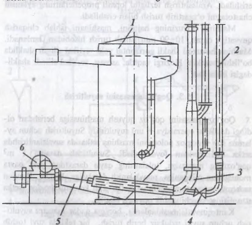
13-rasm. Qog'oz massasini suyultiruvchi qurilma:
