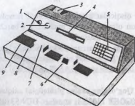
71-rasm. Qog'ozning pishiqligini aniqlaydigan pribor:
