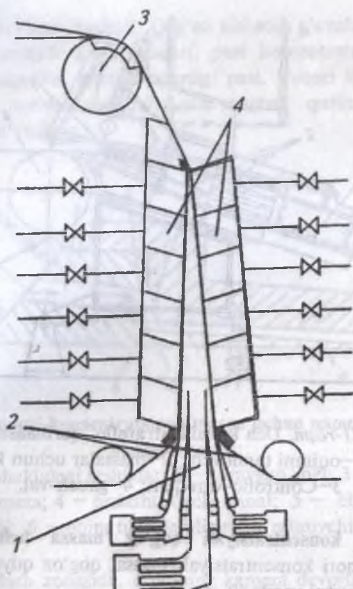
20-rasm. Controflo-Foemer shakllantiruvchi qurilmasining sxemasi:
