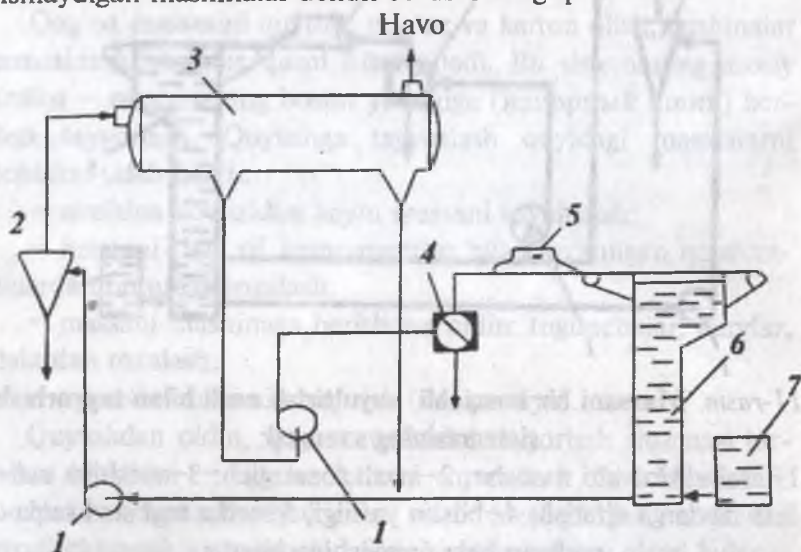
12-rasm. Massani tayyorlashda deaeratsiyalash sxemasi:
