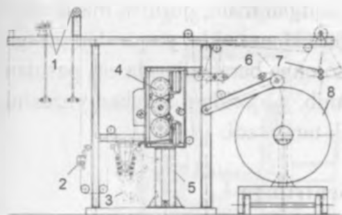
153- rasm. "Goller" firmasi siqish mashinasining texnologik sxemasi:
