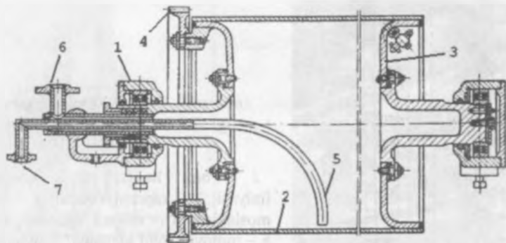
65- rasm. Quritish mashinasi silindring konstruksiyasi:
