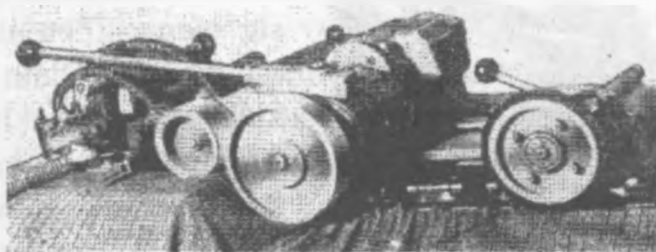
186- rasm. Mato chetini ignalarga chanchish mexanizmining koʻrinishi
