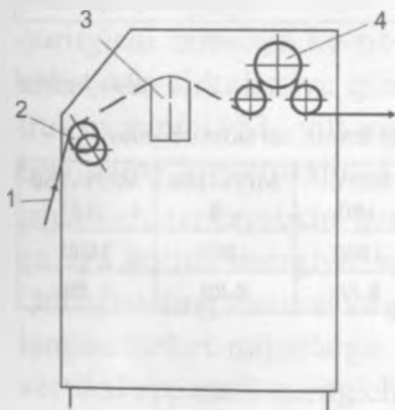
158- rasm. MOV – 180 mashinasining texnologik sxemasi:
