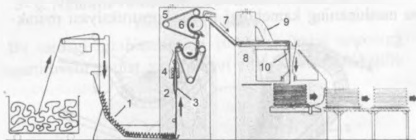
228- rasm. Ikkita kirishtirish mexanizmlari mashina sxemasi:
