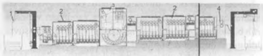
78- rasm. Tarkibida LU turidagi relaksatsiya kamerasi bor yuvish agregati: 1 – mato; 2 – yuvish vannasi; 3 – LU turidagi relaksatsiya kamerasi; 4 – siqish vallari.
