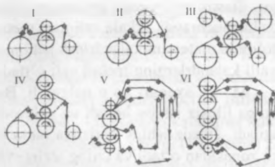
231- rasmi Kalandrlarga matoni zapravka qilish sxemalari
