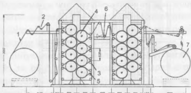
163- ras. "Goller" firmasi quritish mashinasining sxemi:
