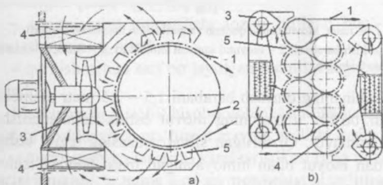
169- rasm. Quritish barabanida matoni ko'p saploli moslama yordamida puflash sxemasi;
