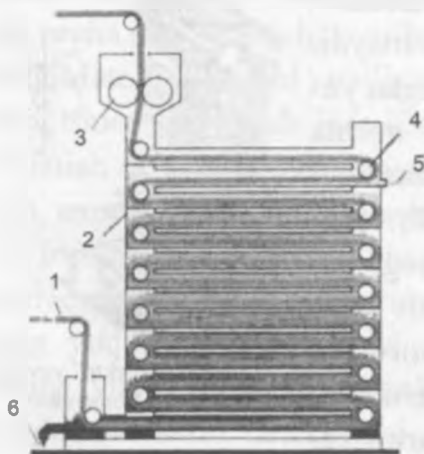
68- rasm. "Menzel" firmasining mato jgutini yuvish mashinasi.
