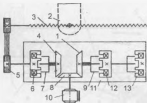
182- rusm. Mato chetining holatini moslovchi mexanizm sxemasi:
