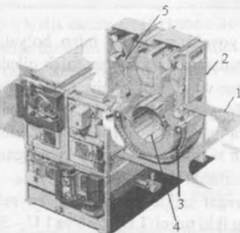
79- rasm. LU – 250 turidagi relaksatsiya kamerasi.
