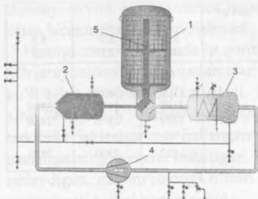
159- rasm. "Tiss" firmasi quritgichining sxemasi:
