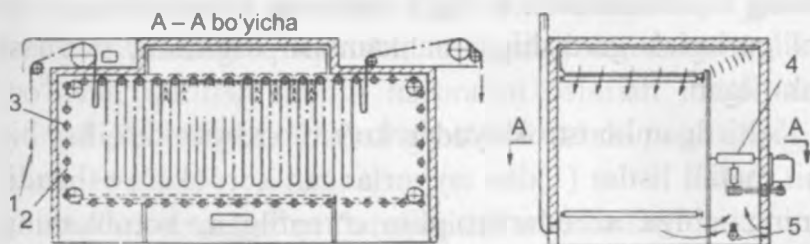
172- rasm. Mato sirtmog'ini osilgan holda quritish mashinasi sxemasi.
