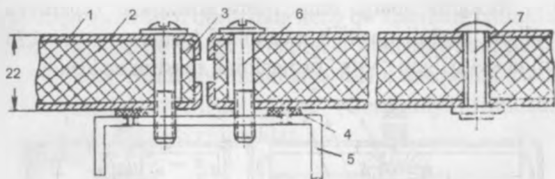
173- rasm. Barabanli quritgichning teploizolatsion to'sig'i konstruksiyasi:
