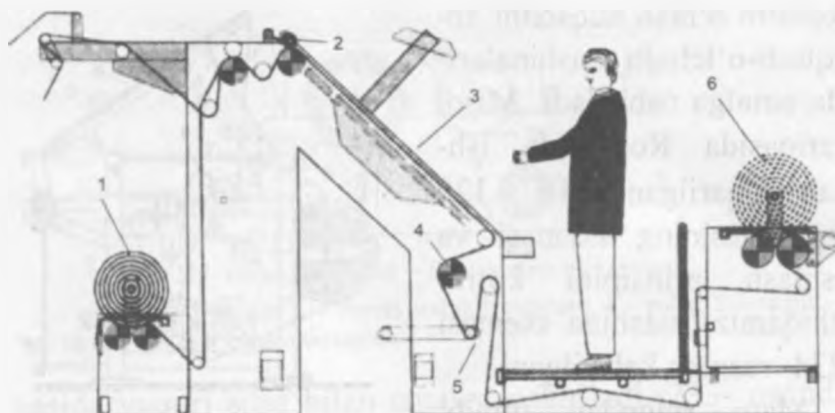
235- rasm. RB/T – 05 sifat nazorat mashinasining sxemasi:
