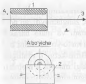
3- rasm. Mato jgutini yoʻnaltiruvchi halqa: 1 – halqa; 2 – rolik; 3 – mato.
