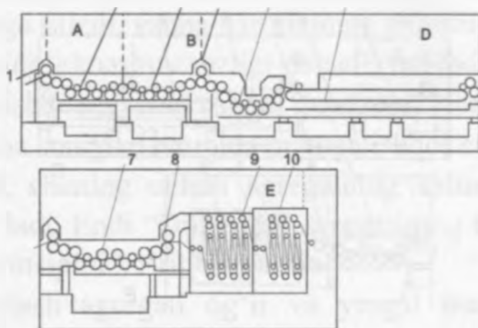
90- rasm. Og'ir matolarni merserlash agregatining texnologik sxemasi:
