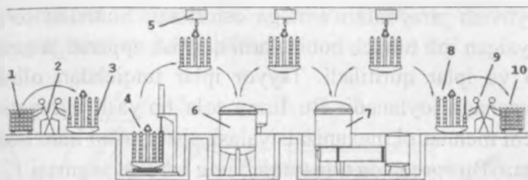
122- rasm. Bo'yash va quritish apparatlaridan iborat agregatda yarim mahsulotlarni transportirlash:
