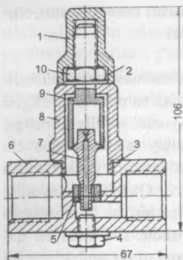
167- rasm. Kichik o'lchamli kondensat chiqaruvchi:
