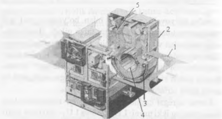
79- rasm. LU – 250 turidagi relaksatsiya kamerasi. 1 – mato; 2 – kamera korpusi; 3 – konveyer; 4 – markaziy baraban; 5 – taxlagich.
