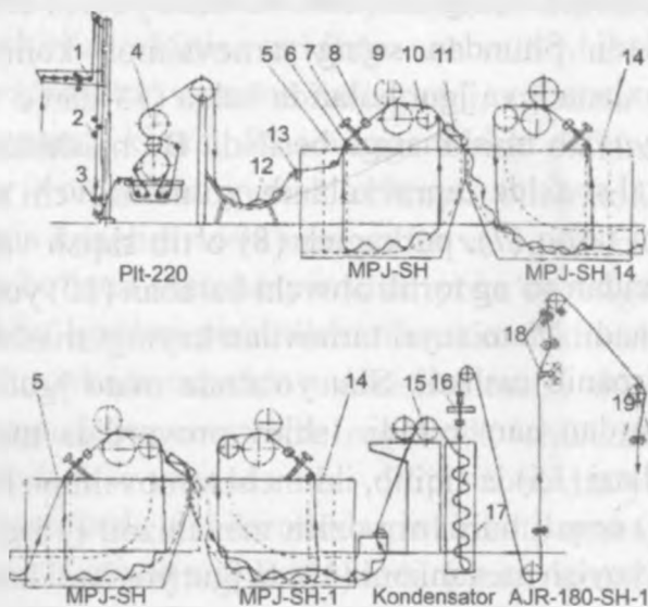
94- rasmda LPJ – 1 – Sh agregatining texnologik sxemasi:
