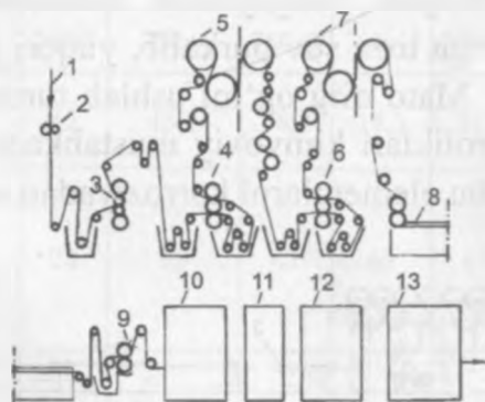
85- ras. Zanjirli merserlash agregatining texnologik sxemasi:
