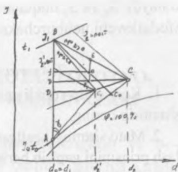
194- rasm. Quritish grafisini ifodalash
