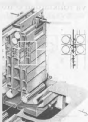
66- rasm. "Injekta" yuvish mashinasi konstruktiv elementlari
