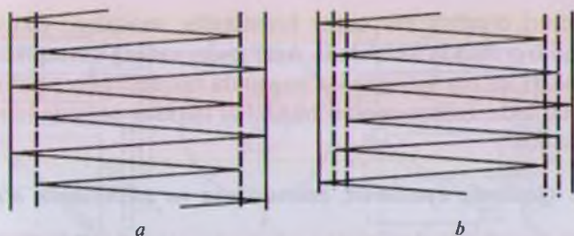
11.7- rasm. Ipyotqizgichning „nafas“ mexanizmi (a) va tarqoqlantirish mexanizmi (b) qoʻllagandagi harakat qonuniyatlari sxemalari.
