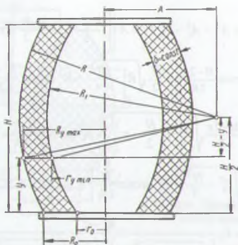
3.11- rasm. Sferik jismga nimqavat qalinligi o'zgaras o'rash sxemasi.
