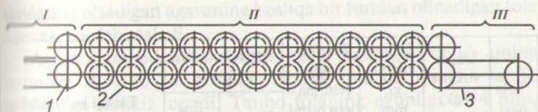
3.16-rasm. MM-2 ezish mashinasining sxemasi: I—,3—tashigichlar; 2—valiklar.
