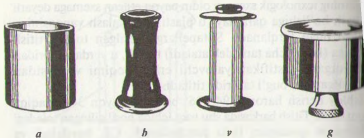
6.15-rasm. TOM dan chiqayotgan iplarni qabul qiluvchi moslamalar: a—bobina; b—shpulya; v—g'altak; g—markazdan qochirma krujka (sentrifugalovchi krujka).
