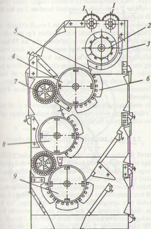
78-рasm. «Мехнат» (CHX-3M2) русумли чигитли пaxтани тозалagич mashinaning sxemasi:
