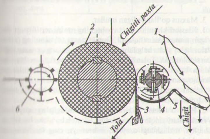
2.10-rasm. XDV rsumli valikli jin mashinasining sxemasi: 1—ignali baraban; 2—ishchi valik; 3—qo'zg'almas pichoq; 4—tola ajratgich valik; 5—to'rli sirt; 6—cho'tkali valik.
