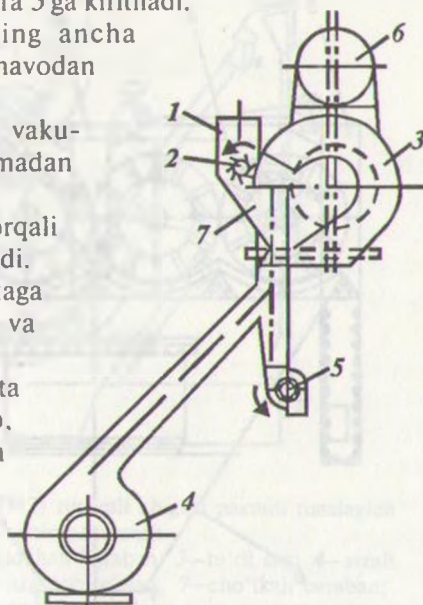
2.6-rasm. YTP-1,5 toshutgich:
