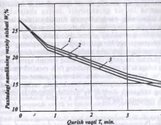
4.10- rasm. Paxtaning quritish egri chizig'iga havo harakati tezligining ta'siri: 1- \vartheta , da=1 m/s; 2- \vartheta , da=1,5 m/s; 3- \vartheta , da=2 m/s.
