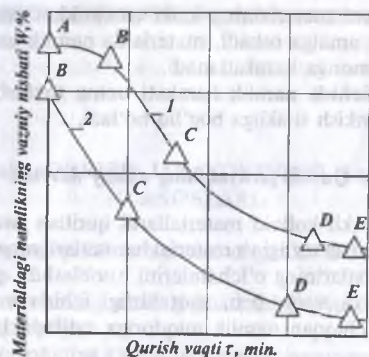
4.1-rasm. Materiallar uchun quritish egri chizig'i: 1—qalin; 2—yupqa.
