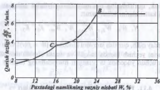
4.8- rasm. \vartheta_A = 1 m/s va t = 120^\circ\text{C} da paxta xomashyosining quritish tezligi egri chizig'i.
