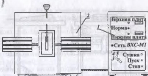
9.4-rasm. BXC-1M rusumli termonamo'lgagichning chizmasi: 1—boshqaruv pult; 2—quritish kamerasi.
