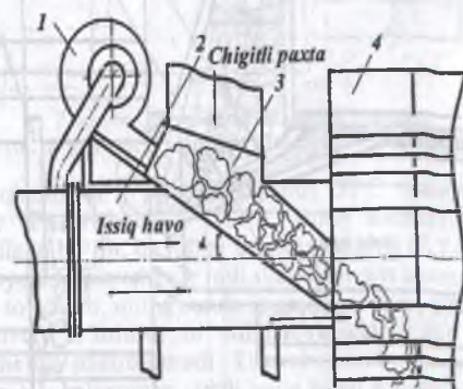
7.3-rasm. Pnevмота'minlagich sxemasi: 1—ventilator; 2—issiq havo quvuri; 3—chigildi paxta shaxtasi; 4—quritish barabani.
