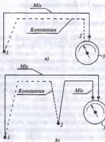
2.9-rasm. Termojuftni galvanometrqa ulash sxemasi.
