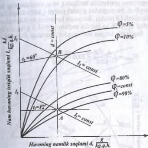
2.5-rasm. Havoning I-d diagrammasi bo'yicha qizdirilgandagi parametri.
