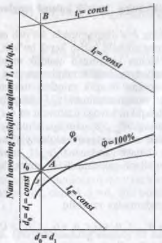
Havoning namlik saqlami d , g/kg q.h.
