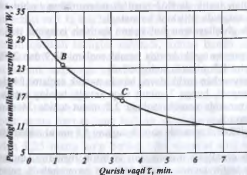
4.7-rasm. v_d = 1 m/s va t = 120^\circ\text{C} da paxta xomashyosining quritish egri chizig'i.
