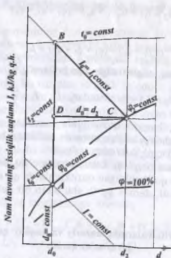
5.4-rasm. Nazariy quritish jarayonining I-d diagrammasidagi tasviri.
