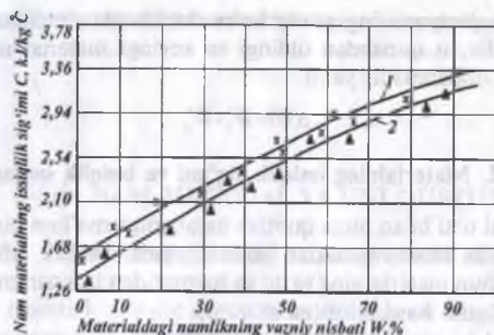
3.1-rasm. Paxtaning issiqlik sig'imini namlikga bog'liqlik grafigi.
