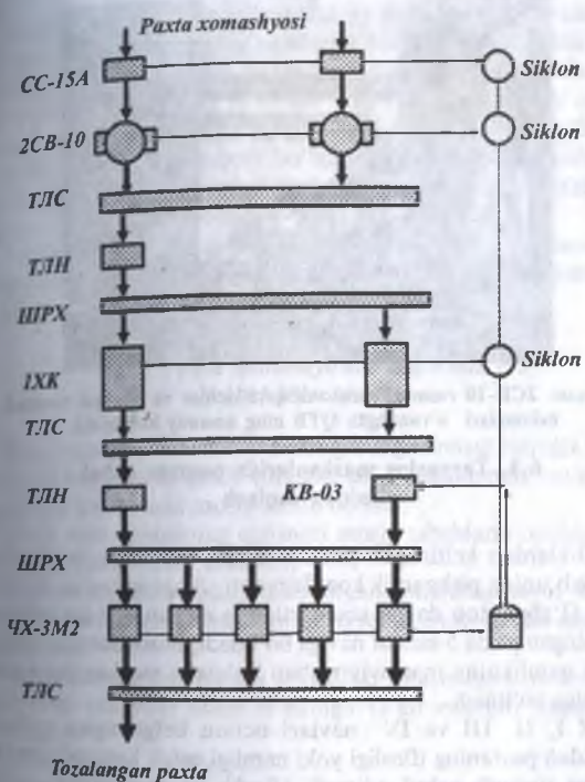
6.3- rasm. 2CB-10, IXK va ЧХ-3М2 rusumli uskunalari o'rnatilgan QTBning texnologik jarayon sxemasi.
