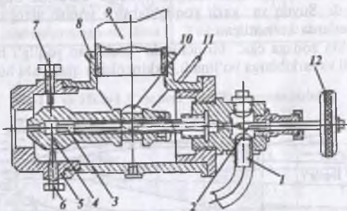
8.8-rasm. Past bosimli forsunka sxemasi:
