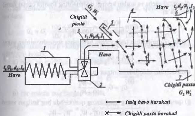
5.1-rasm. Quritish uskunasi hisob sxemasi:
