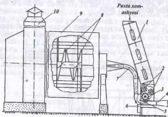
7.7-rasm. Tituvchi qismli va to'plovchi sig'imli PPC rusumli quritkich ta'minlagichi:
