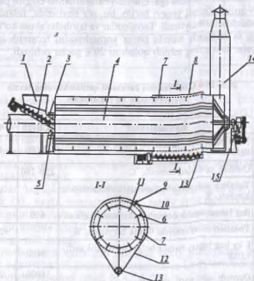
7.2- rasm. CBO rusumli barabanli quritkich sxemasi.
