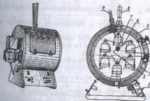
9.1-rasm. Y3-7M rusumli quritish shkafi: 1—boshqarish pult; 2—termoelement; 3—o'rnatgich; 4—byuksa; 5—korpus; 6—yulduzcha; 7—val; 8—kontakt termometri; 9—nazorat termometri.
