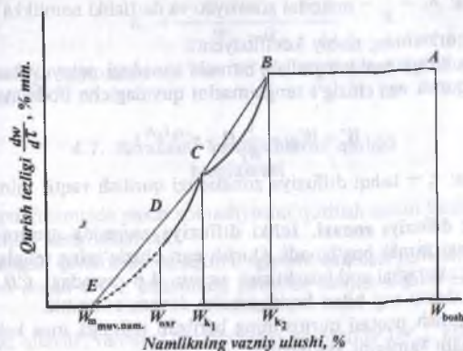
4.6-rasm. Quritish tezligini hisoblash sxemasi.
