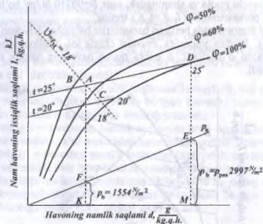
2.4-rasm. I-d diagrammasi bo'yicha havoning nisbiy namligi.
