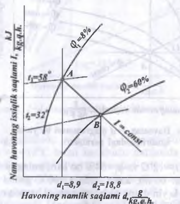
2.6-rasm. Suvning adiabatik bug'lanishida (havoning sovishi) I - d diagrammasi bo'yicha havo ko'rsatkichlarini aniqlanishi.
