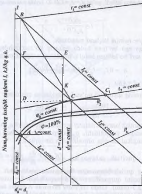
5.5- rasm. Haqiqiy quritish jarayonining I-d diagrammadagi tasviri.
