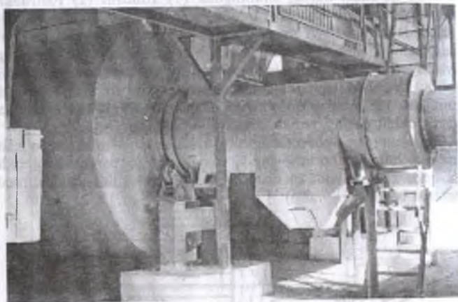
7.9-rasm. 2CB-10 rusumli barabanli quritkichning ta'minlagichi, issiq havo quvuri, baraban, sapfa, barabanning oldi devori, rolıklar va uchqun ushlagichlar ko'rsatilgan majmuasi sxemasi.
