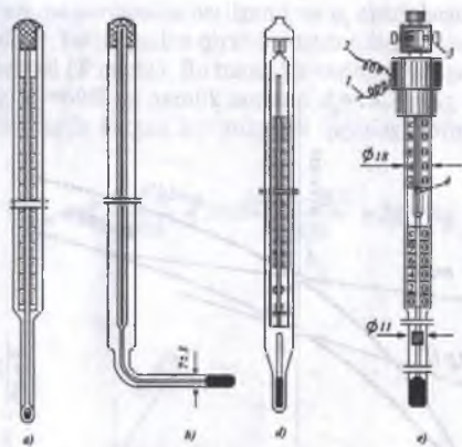
2.8-rasm. Termometrlar.
