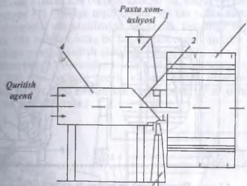
7.6-rasm. Jalyuzali ta'minlagich sxemasi: 1-shaxta; 2-jalyuza; 3-quritish kamerasi; 4-issiq havo quvuri.
