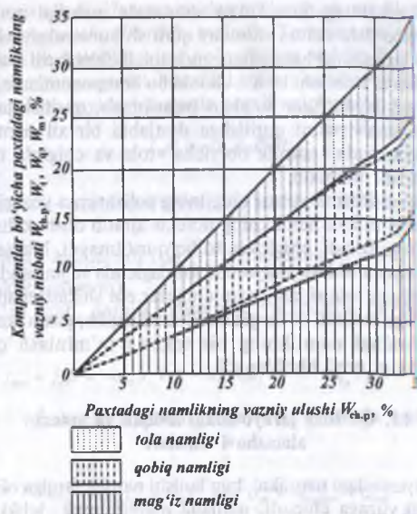
4.5-rasm. Namlikning paxta xomashyosi komponentlari bo'yicha taqsimlanishi.
