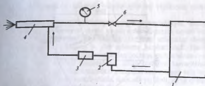
8.10-rasm. ФП.000 rusumli yonilg'ini o'tkazish forsunkasi va suyuq yoqilg'ini purkash tizimi:
