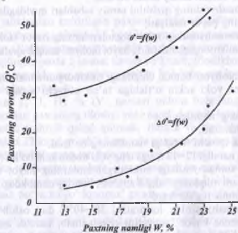
6.5-rasm. Paxta yuzasidagi haroratning ko'tarilishini namligiga bog'liqligi.
