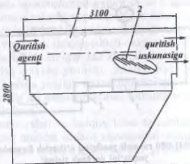
8.11-rasm. Quritish agenti bilan qo'shilib kelayotgan yong'in chiqaruvchi uchqunlarni ushlab qoluvchi ППХ 05.150 rusumli qurilma: 1—ishchi kamera; 2—pog'onasimon jalyuzali qobirg'alar.
