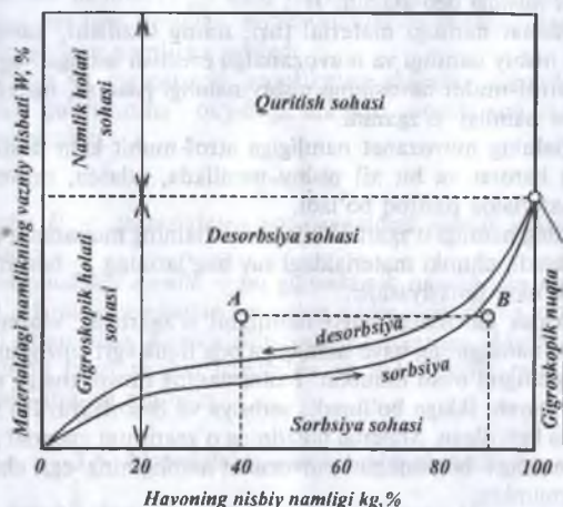
3.2-rasm. Sorbsiya va desorbsiya izotermasi.
