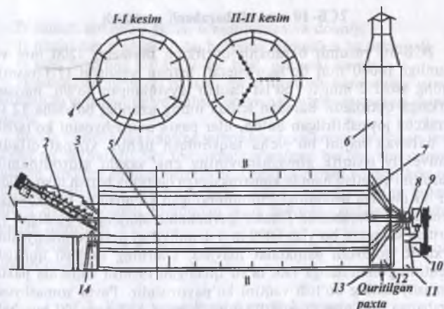
7.1- rasm. 2CB-10 rusumli barabanli quritkich sxemasi.
