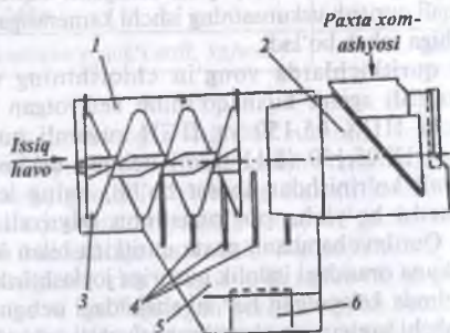
8.12-rasm. ПЦИ rusumli uchqun ushlagich - ta'minlagich: 1—uchqun ushlagich; 2—ta'minlagich qismi; 3—shnekli aylantirgich; 4—panjarali qobirg'alar; 5—qattiq jisimlarni yig'uvchi shaxta; 6—qopqoq.
