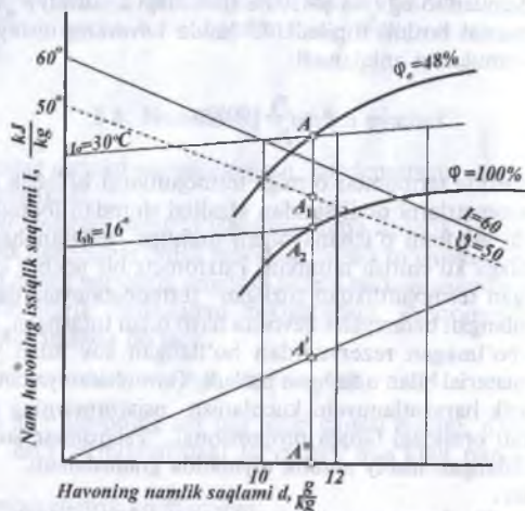
2.11-rasm. I-d diagrammada havoning asosiy ko'rsatkichlarini aniqlash.
