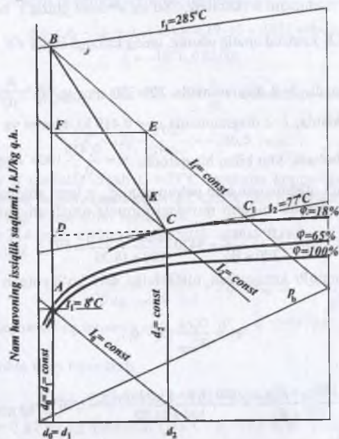
5.6-rasm. I-d diagrammada qurish jarayoni.
