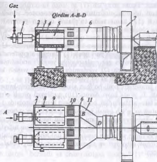
8.1-rasm. TT-1.5 rusumli issiqlik ishlab chiqargich sxemasi:
