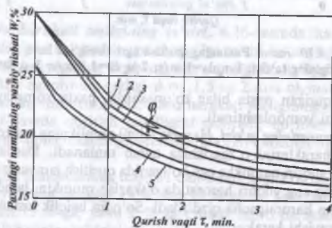
4.11-rasm. Quritish harorati rejimlarini paxta xomashyosining qurish egri chizig'iga ta'siri: 1- t da = 120°C; 2- t da = 160°C; 3- t da = 190°C; 4- t da = 120°C; 5- t da = 160°C.
