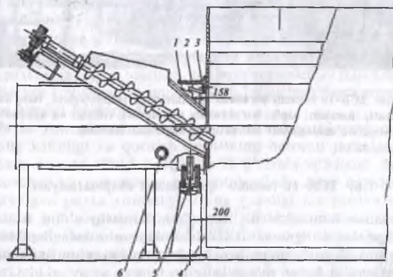
7.8-rasm. 2CB-10 rusumli quritkichning ta'minlagichi sxemasi:
