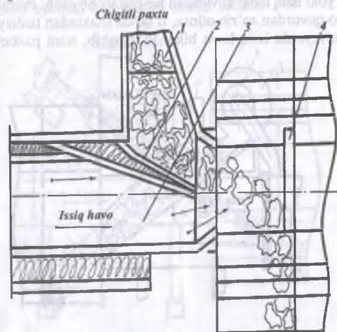
7.5-rasm. Lotokli ta'minlagich sxemasi: 1-shaxta; 2-lotok; 3-issiq havo quvuri; 4-quritish kamerasi
