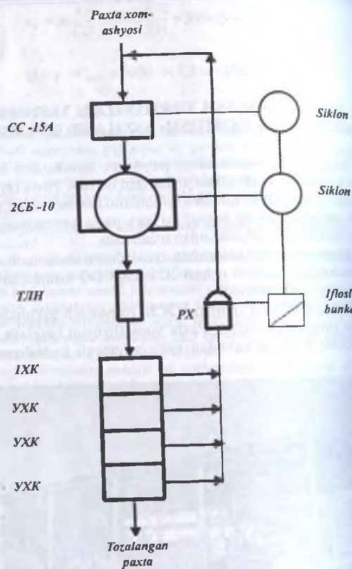
6.2- rasm. 2CB-10, IXK va YXK rusumli uskunalari o'rnatilgan QTBning texnologik jarayon sxemasi.
