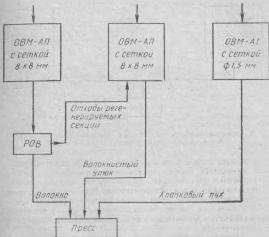
19. Схема технологического процесса переработки утилизируемых волокнистых отходов на хлопкозаводах пильного джинирования.
