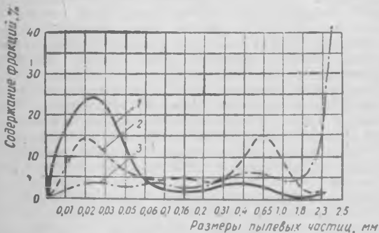
3. Дисперсный состав пыли.
