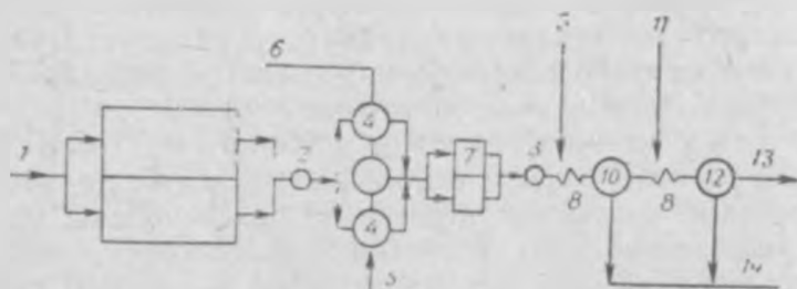
39. Схема установки для очистки сточных вод от сернистой меди и хромпика:
