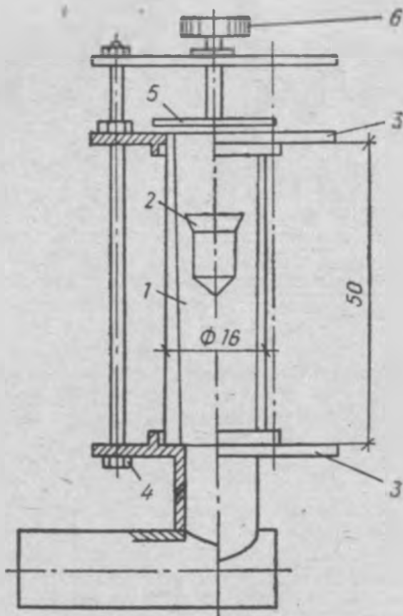
22. Ротаметр.
