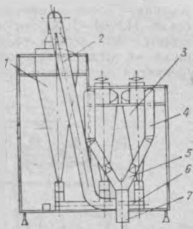
8. Схема двухступенчатой трехциклонной установки.
