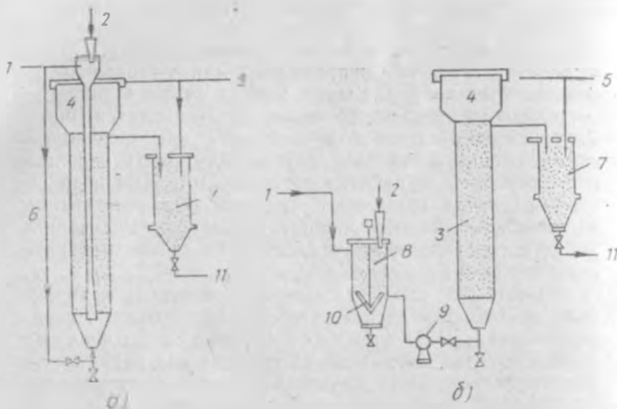
38. Схема адсорберов для очистки сточных вод:
