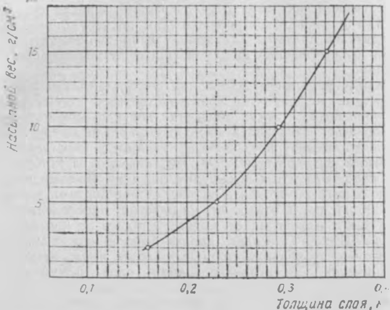
27. Зависимость насыпного веса пыли от толщины осевшего на горизонтальную поверхность слоя.
