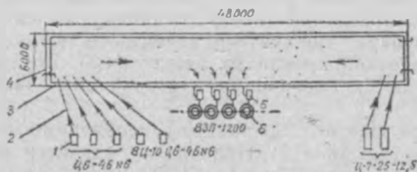
18. Система очистки воздуха ПК-ВЗП.
