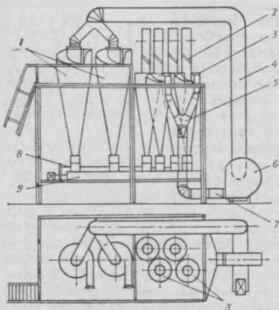
9. Схема двухступенчатой шестициклонной установки.
