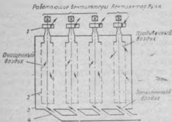
16. Принципиальная схема фильтра ФХК-6.
