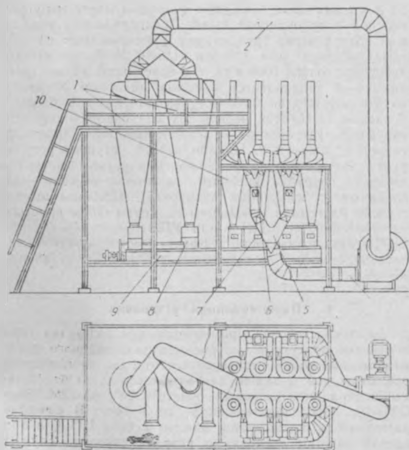
10. Схема двухступенчатой десятициклонной установки.
