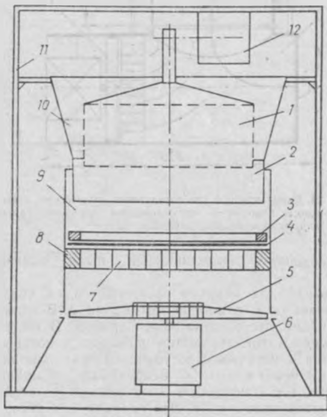
26. Схема прибора для определения количества глыб в массе коконов с использованием ткани ПФП-15 для осаждения выделившейся пыли.
