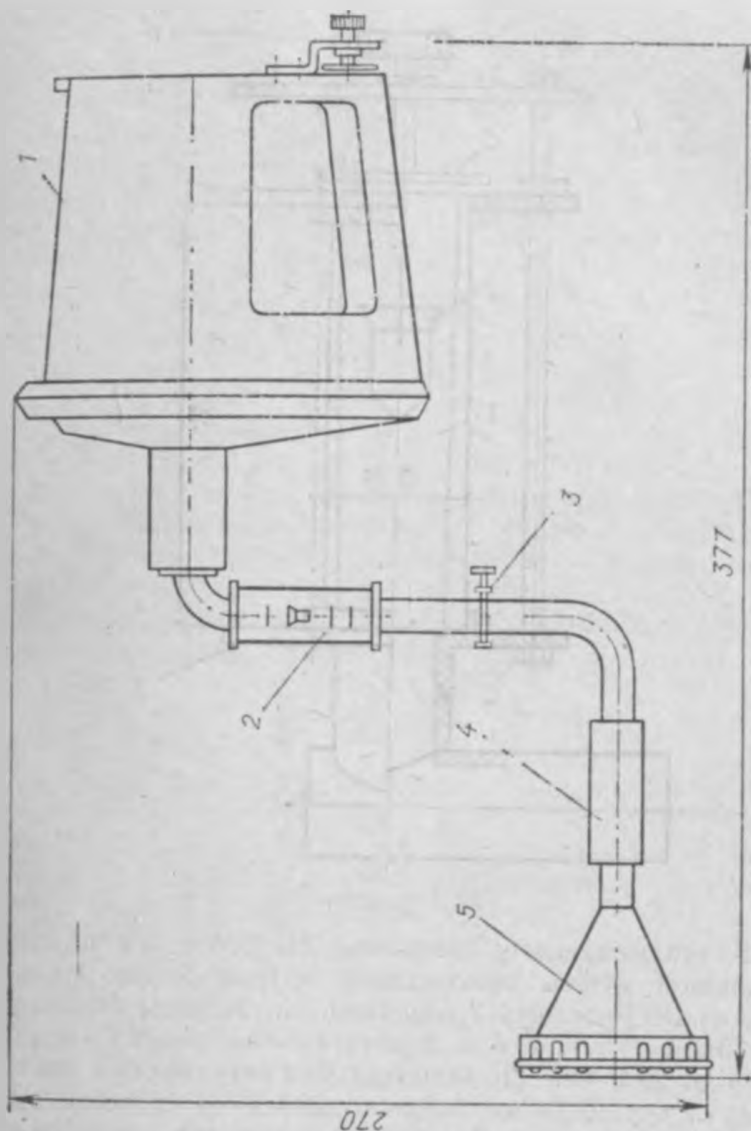
21. Универсальный портативный пылемер.
