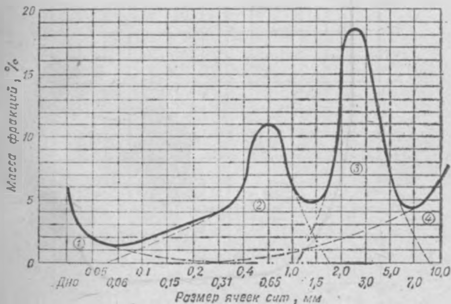
29. Дисперсный состав пылевых отходов, выделяющихся в сдиро-сдиральной машине.
