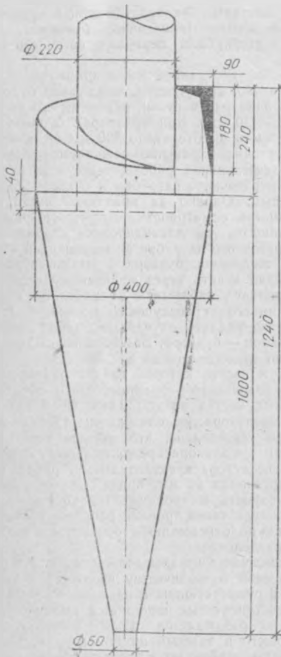
35. Габаритные размеры циклона 2-й ступени очистки воздуха.
