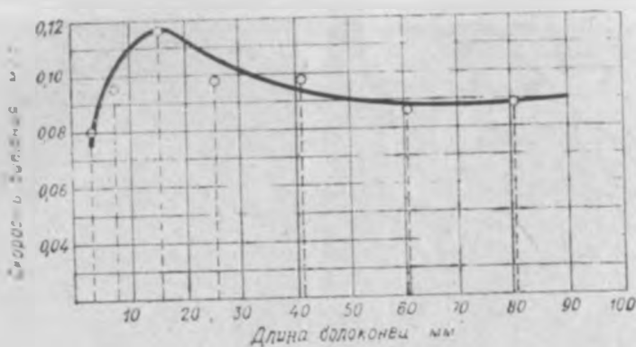
32. Зависимость скорости витания пропыленных шелковых волоконцев от их длины.
