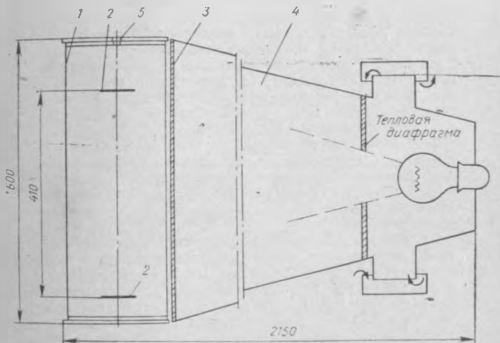
24. Схема прибора для определения скоростей витания обрывков волоконца натурального шелка.
