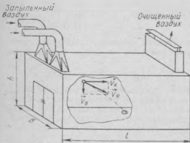
15. Схема устройства пылеосадочной камеры.
