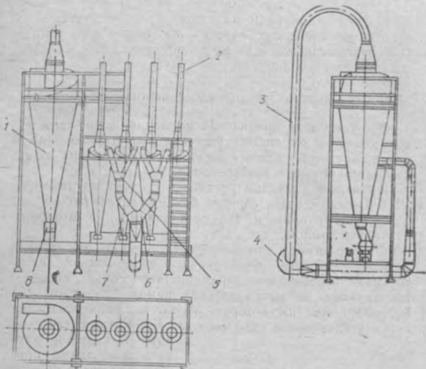
11. Схема двухступенчатой пяти циклонной установки.
