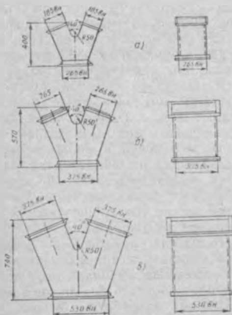
13. Схема тройников.
