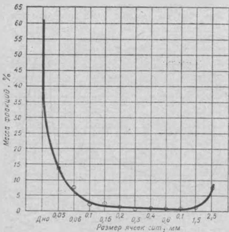
30. Дисперсный состав пыли, выделяющейся в воздухе цеха сухой обработки коконов.
