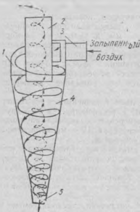
4. Конический циклон.
