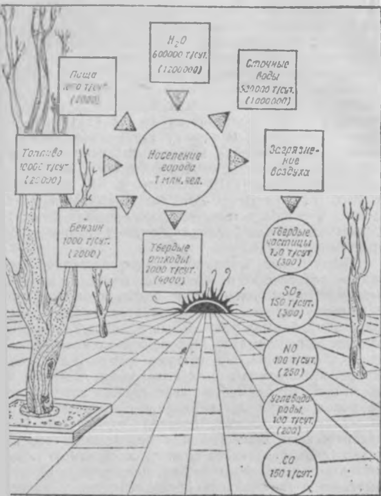
. Массо- и энергообмен современного города за сутки.
