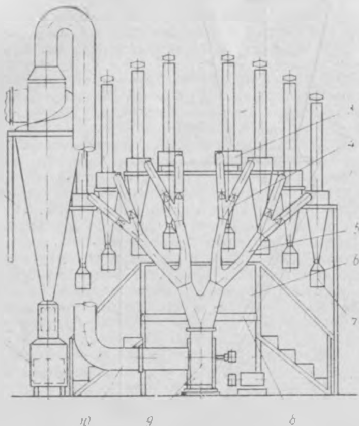
37. Двухступенчатая пылеулавливающая установка.
