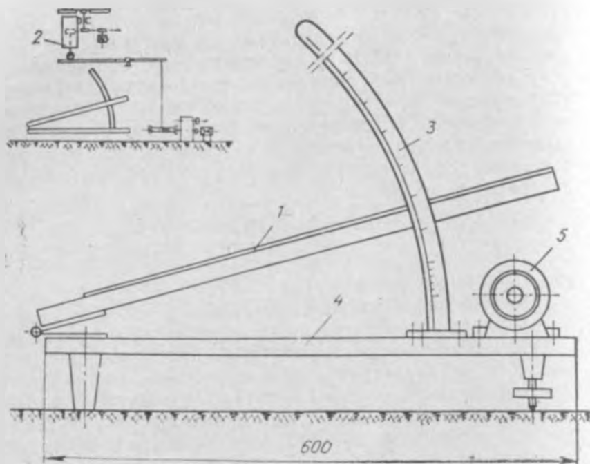
23. Прибор для определения углов трения пыли.
