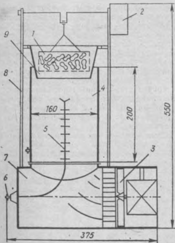
25. Схема прибора для определения количества пыли в массе коконов с использованием коронного газряда для осаждения выделившейся пыли.
