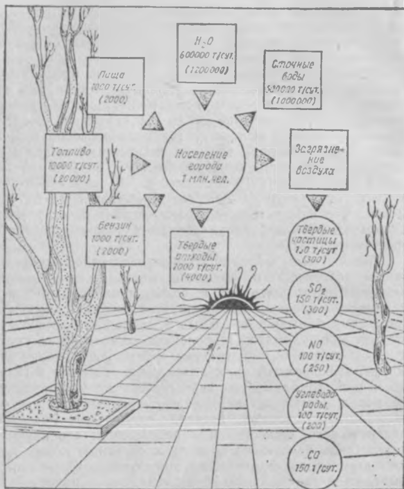
1. Массо- и энергообмен современного города за сутки.
