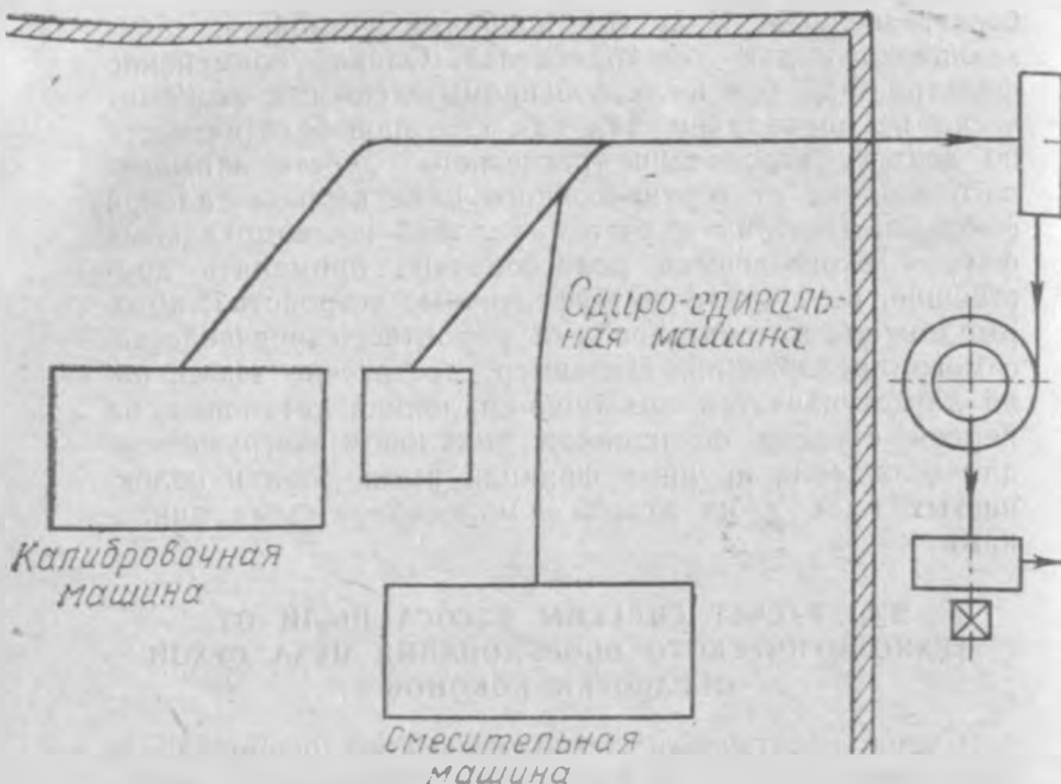
33. Схема расстановки технологического оборудования для обработки сухих коконов на Ферганской шелкомотальной фабрике.
