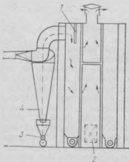
12. Циклон-фильтр-камера:
