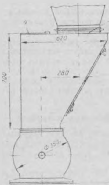
14. Бункер.
