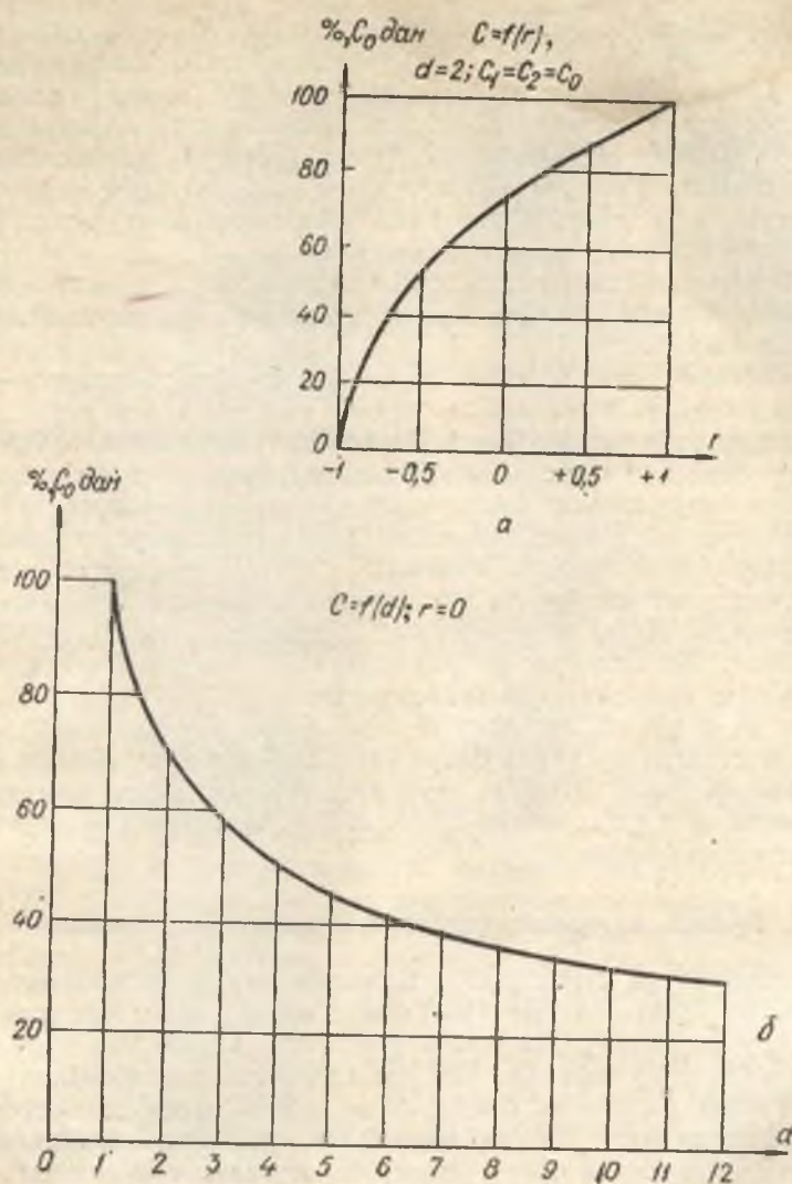
100- расм. Қўшиш процессида маҳсулот нотекислигининг ўзгариши: а — қўшибатган иккита маҳсулотнинг ўртасидаги корреляция коэффициентига қараб; б— қўшишлар сонига қараб, иккита маҳсулотнинг ўртасида корреляция бўлмаган ҳолда.
