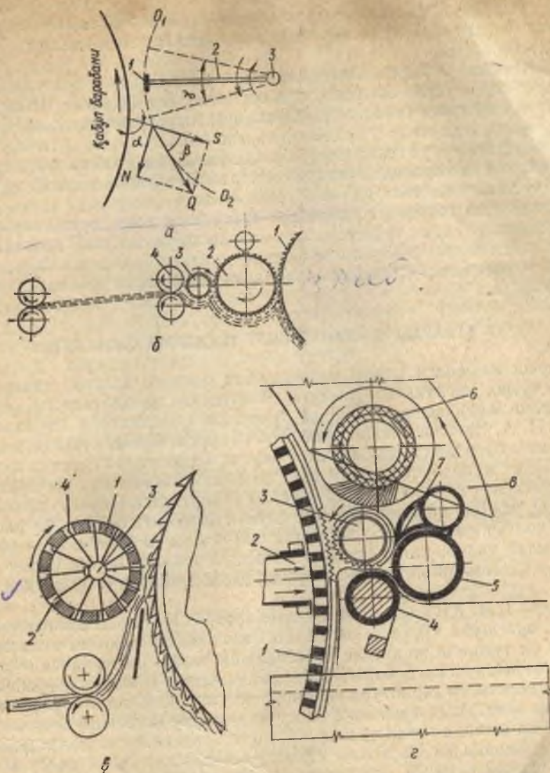
50- расм. Ажратувчи барабан сиртидан тарамни ажратиб олиш: а — тароқли механизм; б — валикли механизм; в — ротацион механизм; г — пневма- тик усулда ажратувчи механизм.
