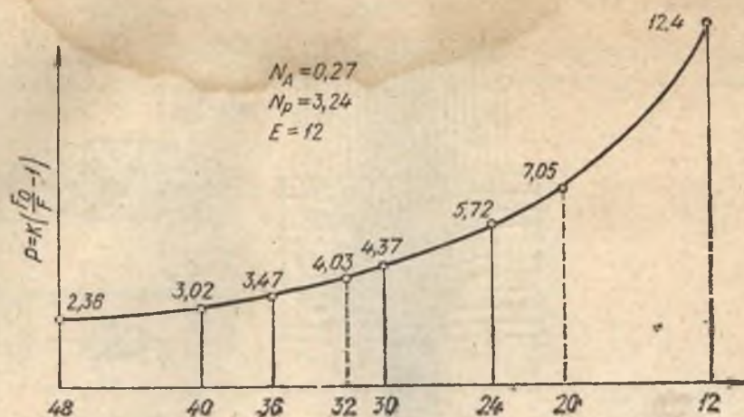
95- расм. Чўзиш асбобига кираётган толалар босимининг ўзгариш диаграммаси.
