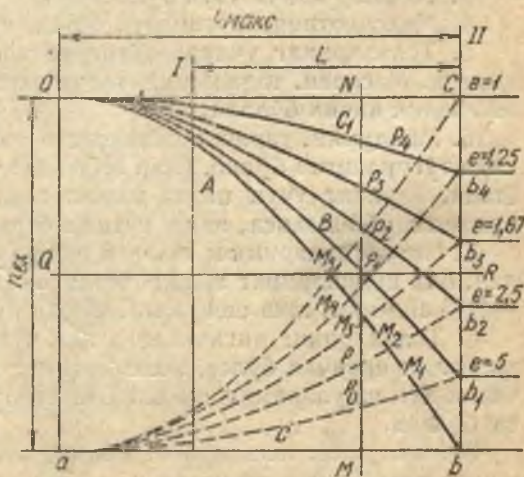
97-расм. Чўзиш эгри чизиғи.
