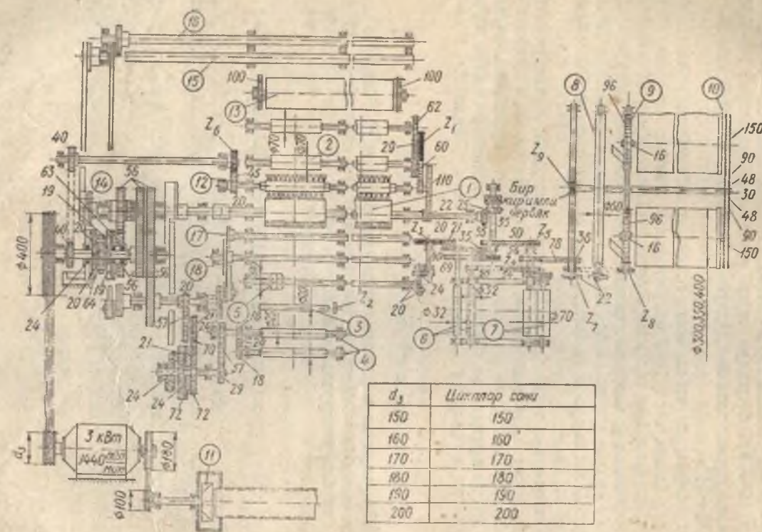
87- расм. Қайта тараш машинасининг кинематик схемаси.
