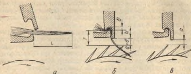
73- расм. Тискиларда холстчанинг сиқилиши.
