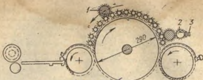
57- расм. Юмалоқ (цилиндрик) шляпкали тараш машини.
