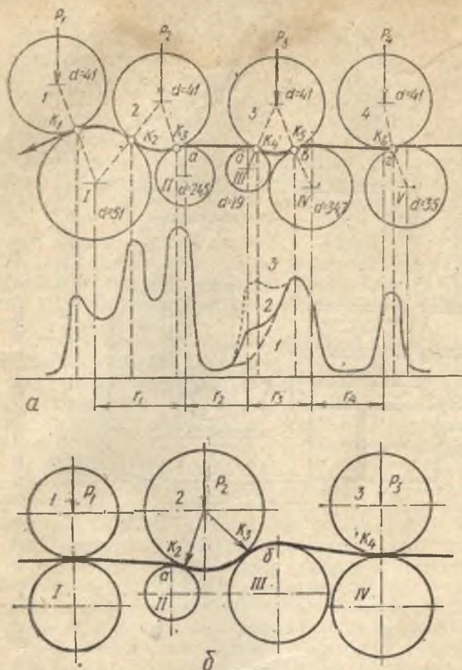
111- расм. Тез ишлай- диган пилта машина- сининг чўзиш асбоби: а — 4 валик; б — цилиндр; б — 3 валик; 4 цилиндр.
