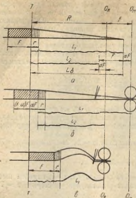
81-расм. Холстча тутамининг ҳар хил иш пайтларидаги ҳолати: а — тароқли барабан тараб бўлгандан кейинги; б — толаларнинг ажрала бошланиши; в — толалар ажралашининг тугалланиши.
