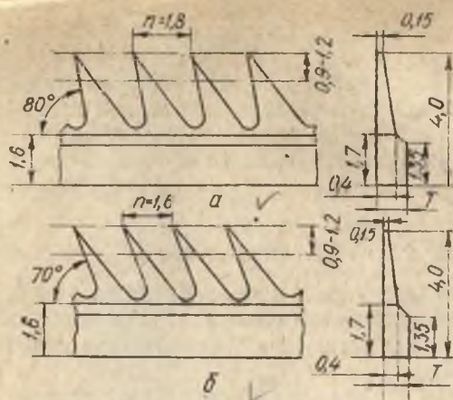
34- расм. Аппарасимон тишли ленталарнинг шакли: а) катта барабан учун, б) ажратувчи барабан учун.
