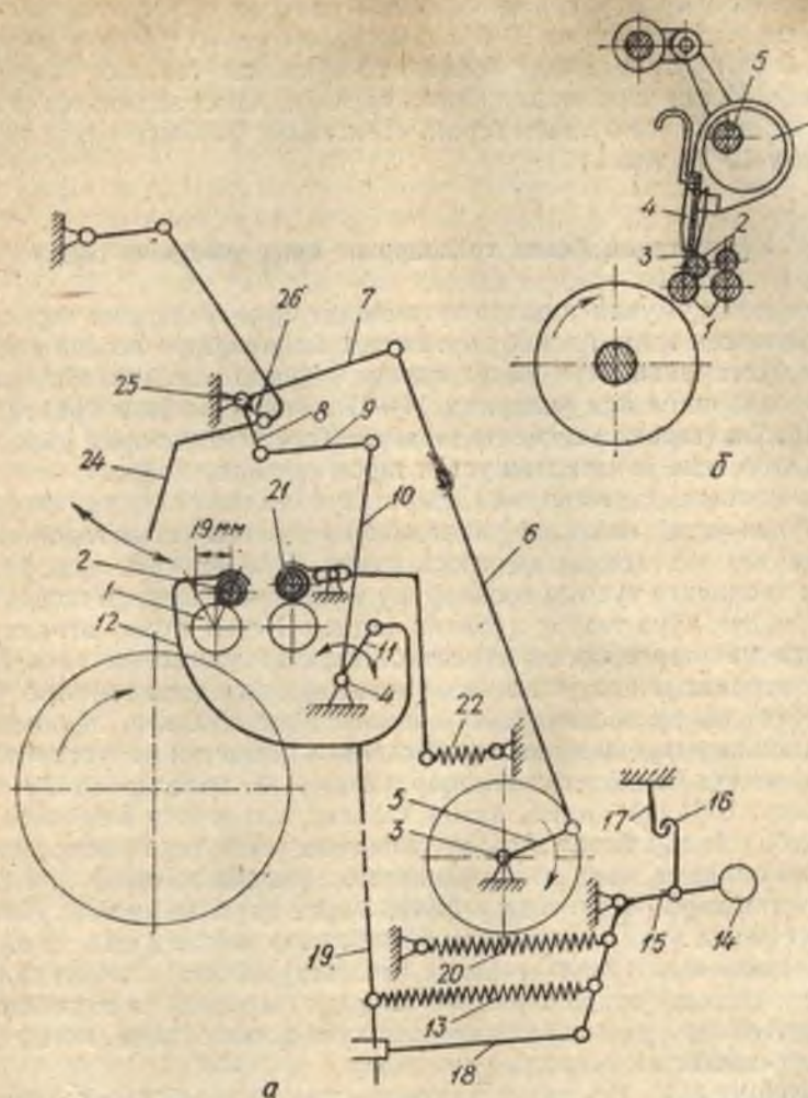
76-рasm. Устки тароқнинг ўрнатилиши.
