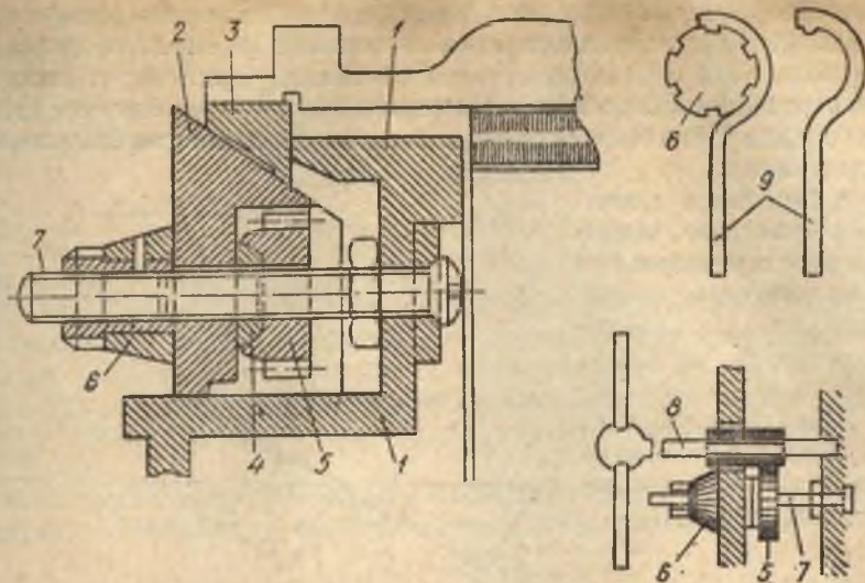
44- расм. Шляпка билан барабан ўртасидаги оралиқ (разводка) ни ростлаш мосламаси.
