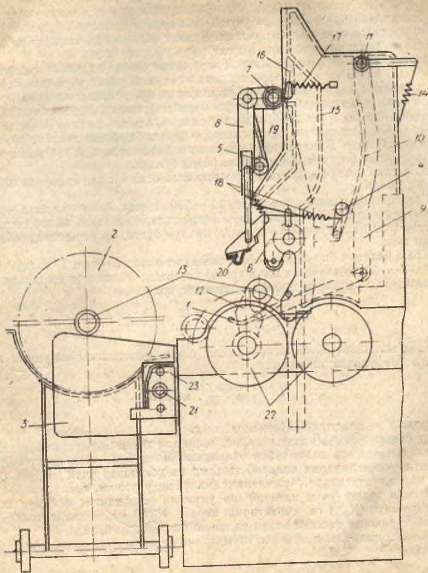
27-рәсм. Холстини автоматик равишда скалкадан чиқазиб олиш ва уни заправка қилиш механизмининг схемаси.
