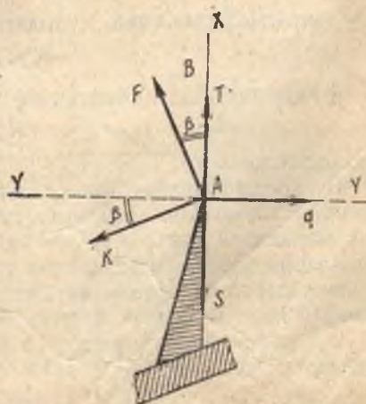
41- расм. Катта барабан тишлари ушлаб турган тола тутамига таъсир қиляётган кучлар.
