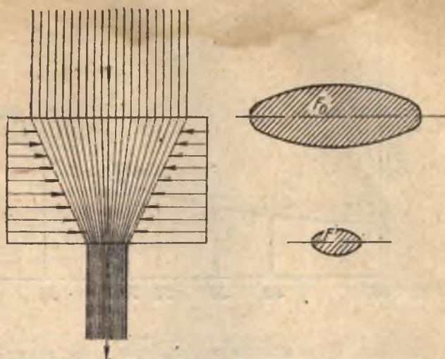
34- расм. Маҳсулотнинг зичланиш схемаси.
