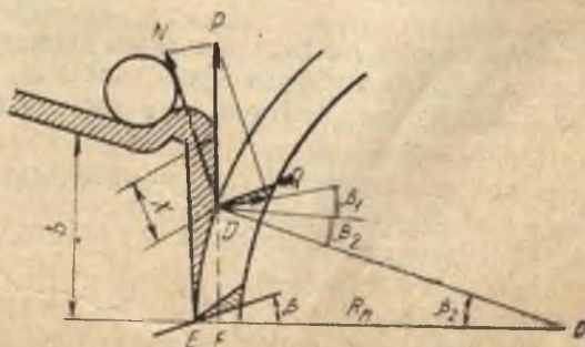
37-расм. Қабул барабани тола тутамининг тара- ётганда, унга таъсир қилаётган кучлар
