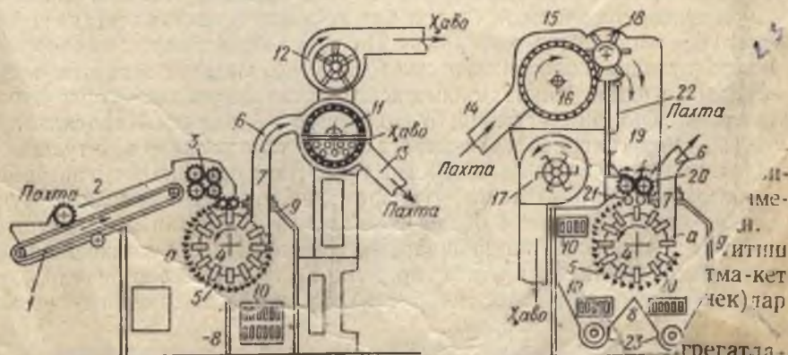
12-расм. Горизонтал пахта титиш машиналари а — чанг тозаловчи барабани; б — таъминловчи барабан
