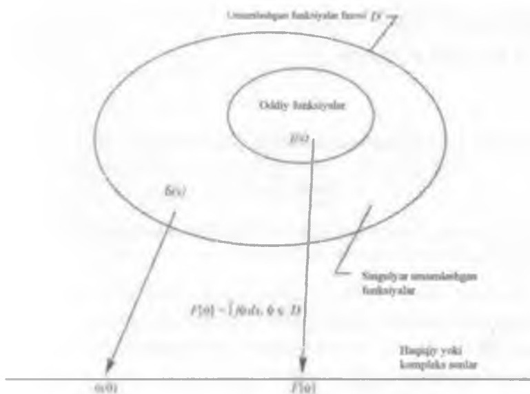
4-chizma. Klassik va umumlashgan funksiyalar to'plamlari.
