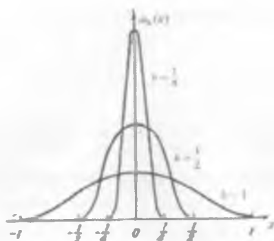
1-chizma. Turli h lar uchun \omega_h(x) funksiyaning grafi.
