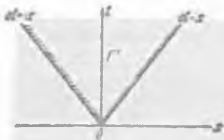
6-chizma. \Gamma_n^1 soha.
