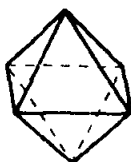
Oktaedr
