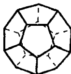
Dodekaedr
