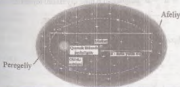
9-rasm. Osmon obyektlarining Quyosh atrofidagi elliptik orbitasi.
