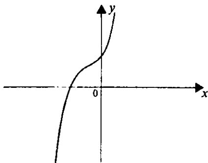
12.14- chizma. y=ax^3+bx^2+cx+d .
