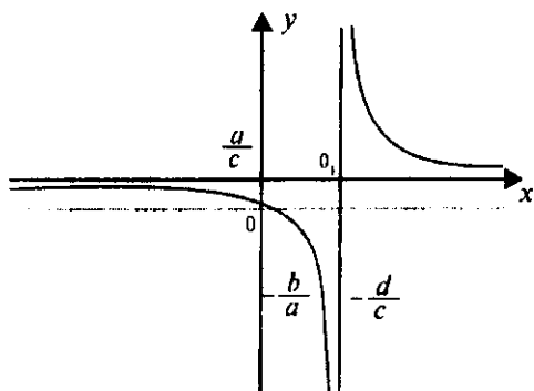
12.23- chizma. k > 0 .
