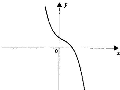
12.13- chizma. y=ax^3+bx^2+cx+d .
